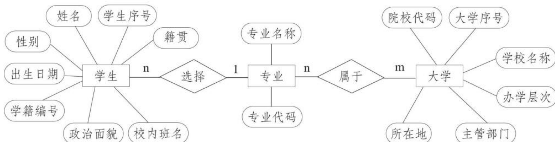
图3.1.8 优化后的E-R图
