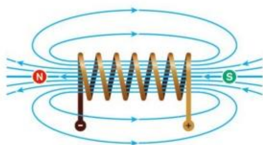
图2.3.3 干扰的出现
