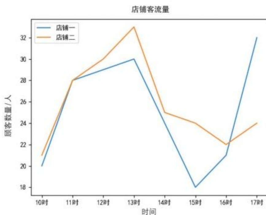
图4.1.2 对比分析图
