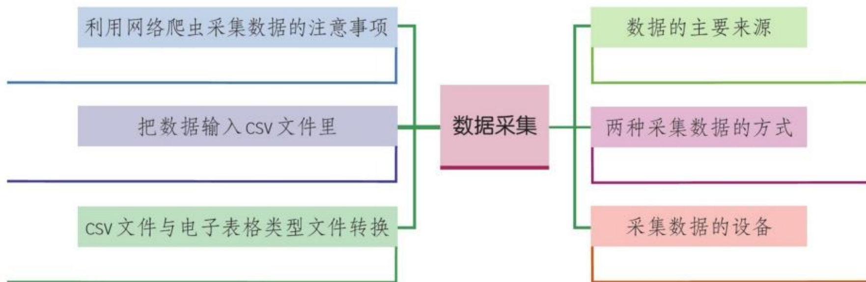
图 2.2.13 知识总结
