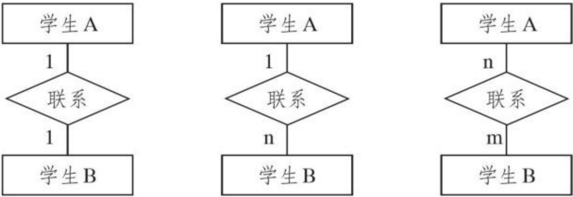
图3.1.6 实体之间的三种联系
