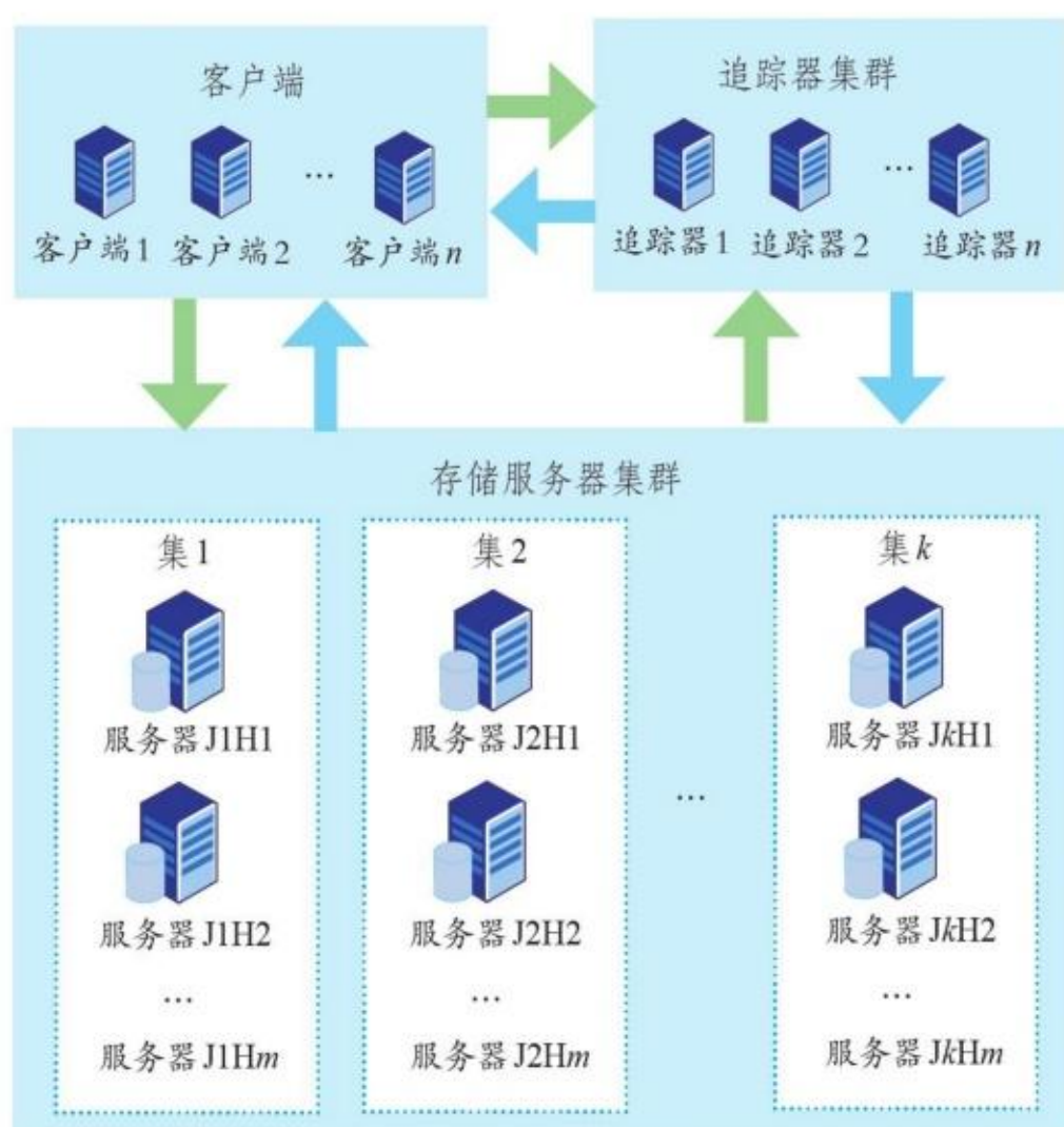
图 1.2.5 分布式文件系统示意图
