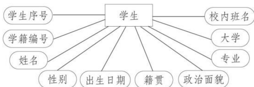
图3.1.7 最初的学生E-R图
