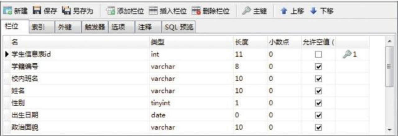
图3.2.5 创建的数据表
