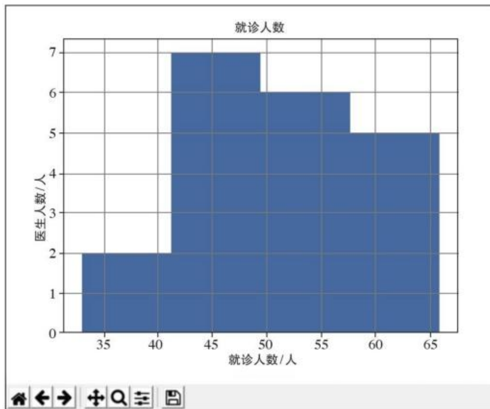
图4.1.4 直方图
