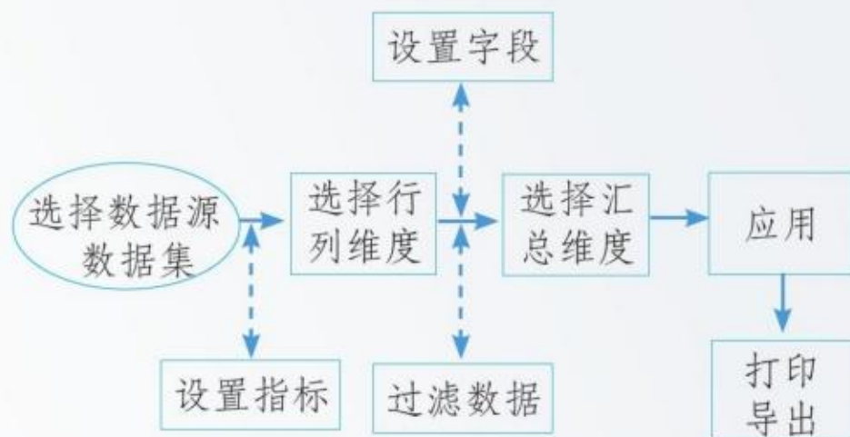
图 4.1.7 交叉分析法
