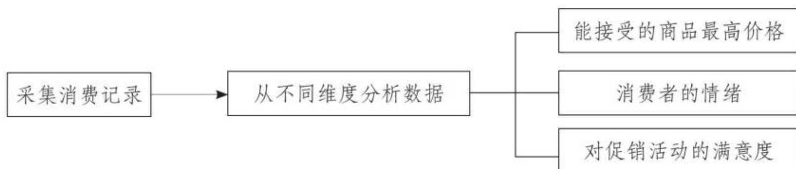
图4.1.1 分析的内容
