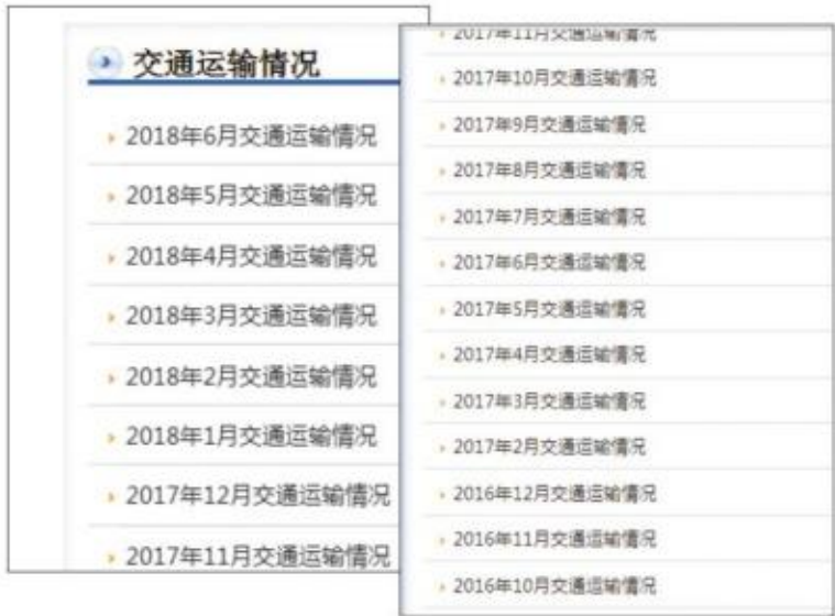
图 2.2.6 网页条目
