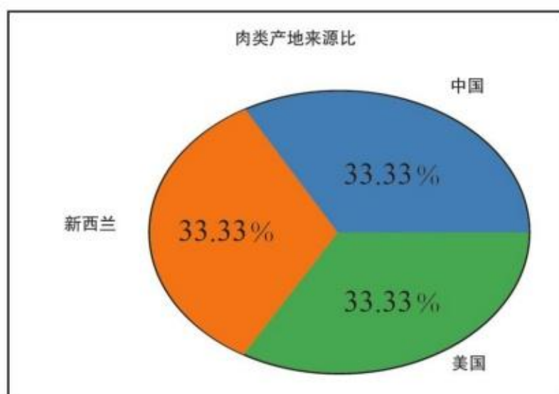
图 4.1.6 饼图
