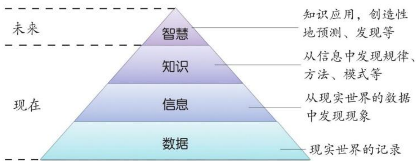
图 1.1.3 DIKW 金字塔
