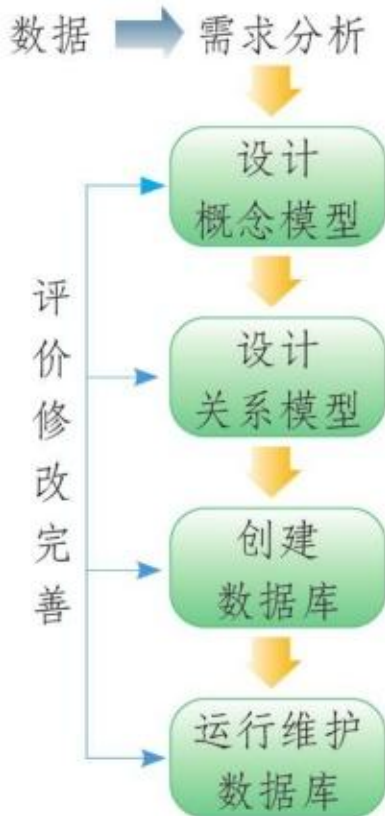
图 3.1.2 大体过程
