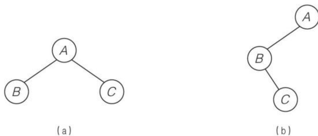
图 3.5.20 3 个节点的二叉树形态
