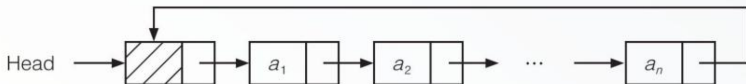
图 3.1.15 具有 n 个节点的单循环链表示意图
