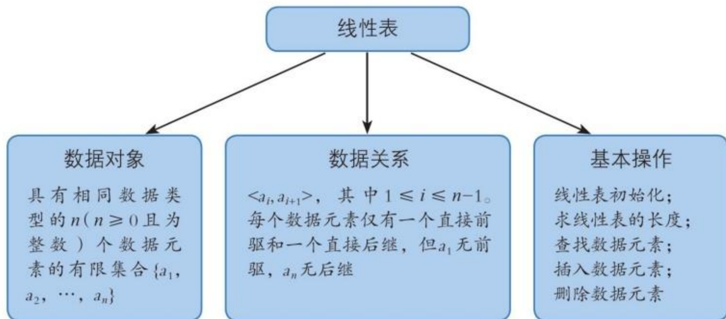
图 3.1.2 线性表的抽象数据类型定义示意图
