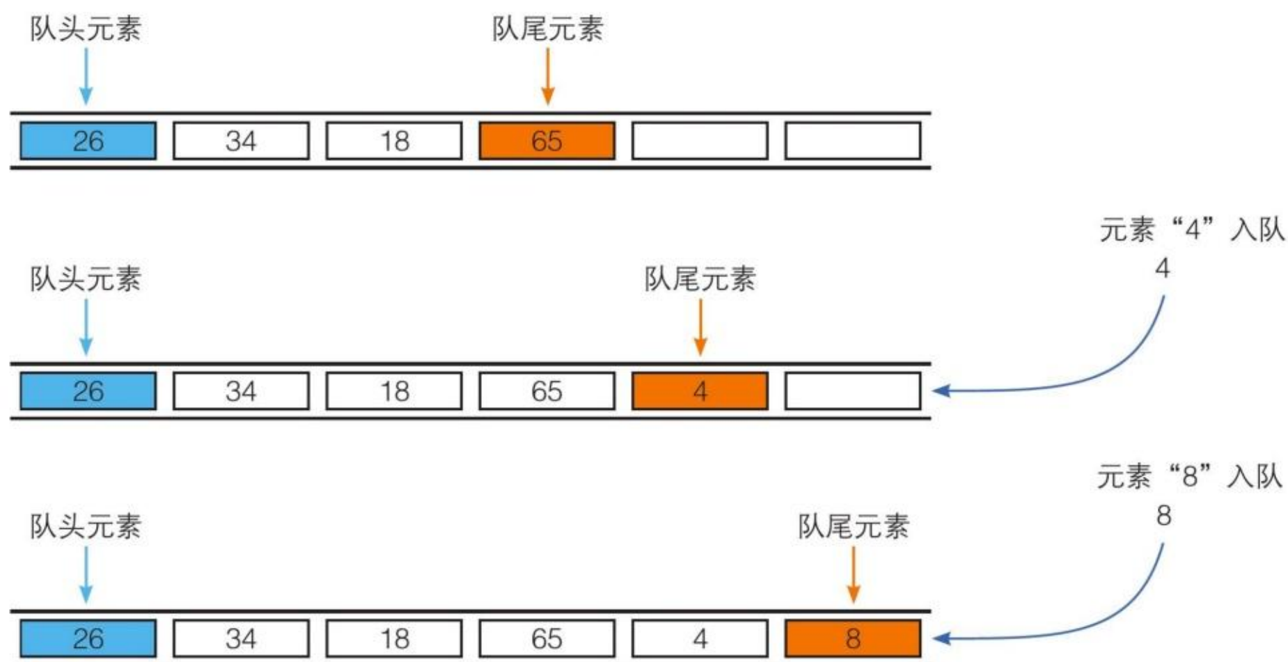
图3.3.6 数据元素连续入队示意图
