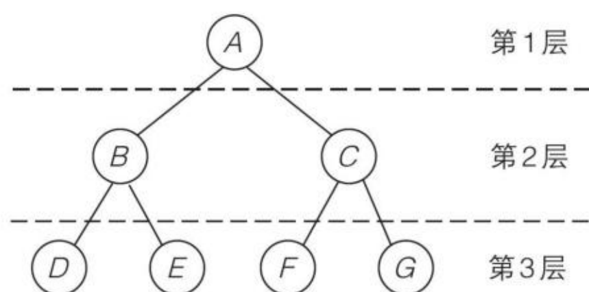
图3.5.6 二叉树的层次示意图
