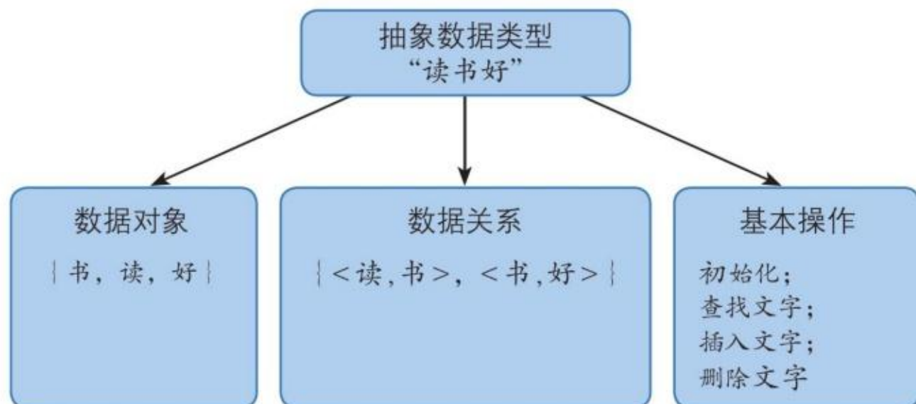
图2.1.11 抽象数据类型“读书好”的定义示意图
