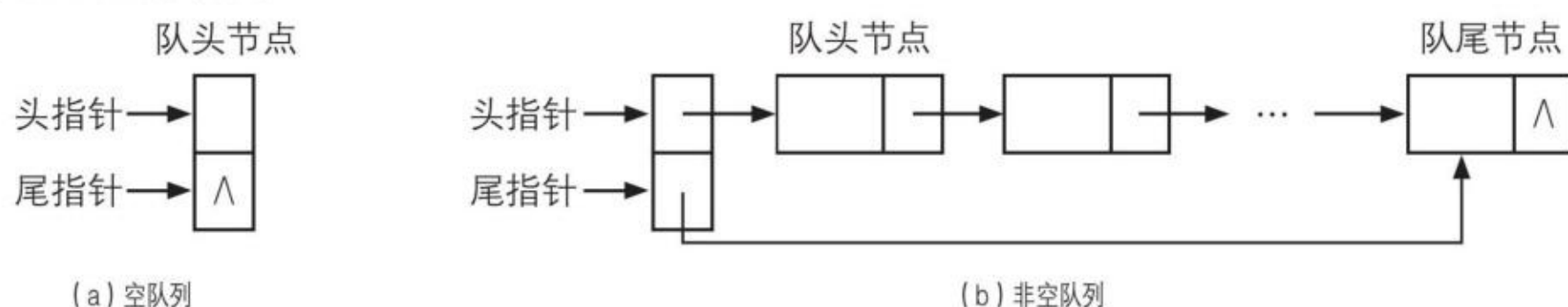
图3.3.12 链式队列示意图
