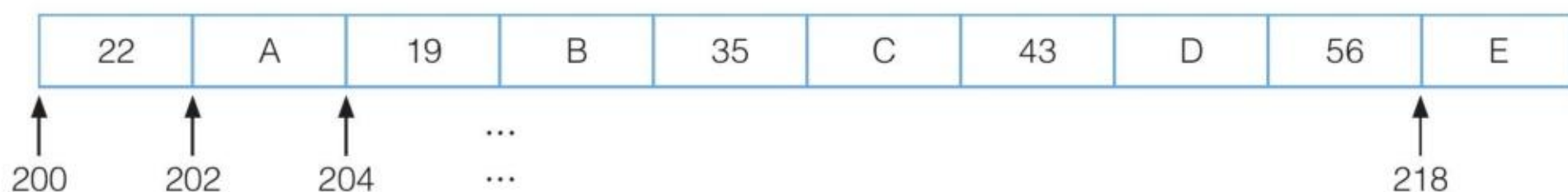
图3.1.19 内存中的某单链表示意图
