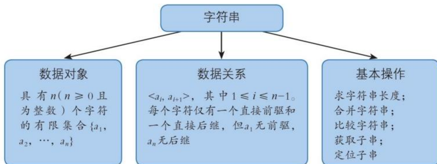
图3.4.2 字符串的抽象数据类型定义示意图
