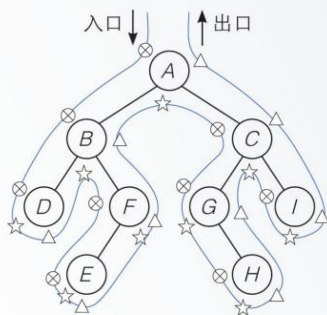
图 3.5.17 动物园馆舍遍历示意图
