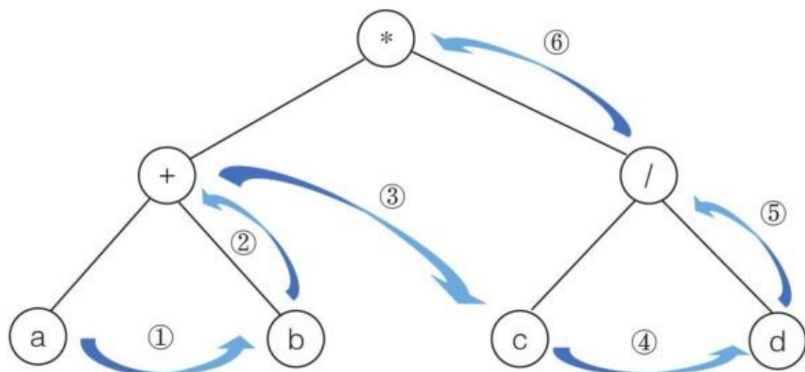
图3.5.16 后根序遍历示意图
