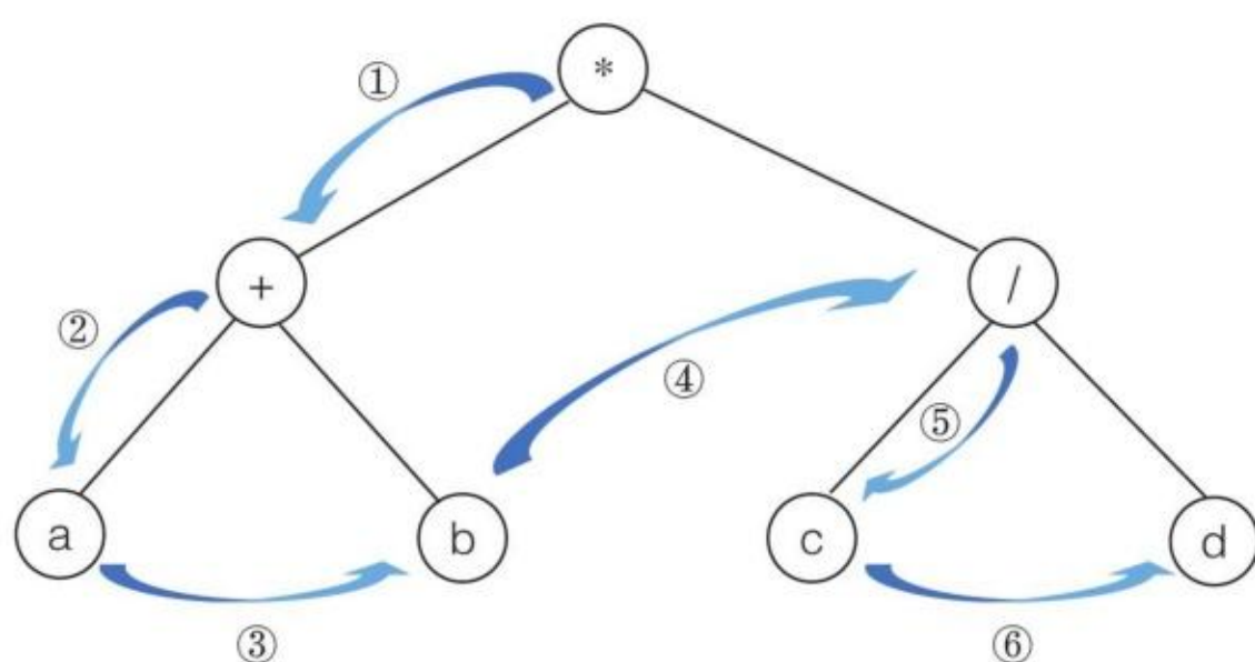
图3.5.14 先根序遍历示意图
