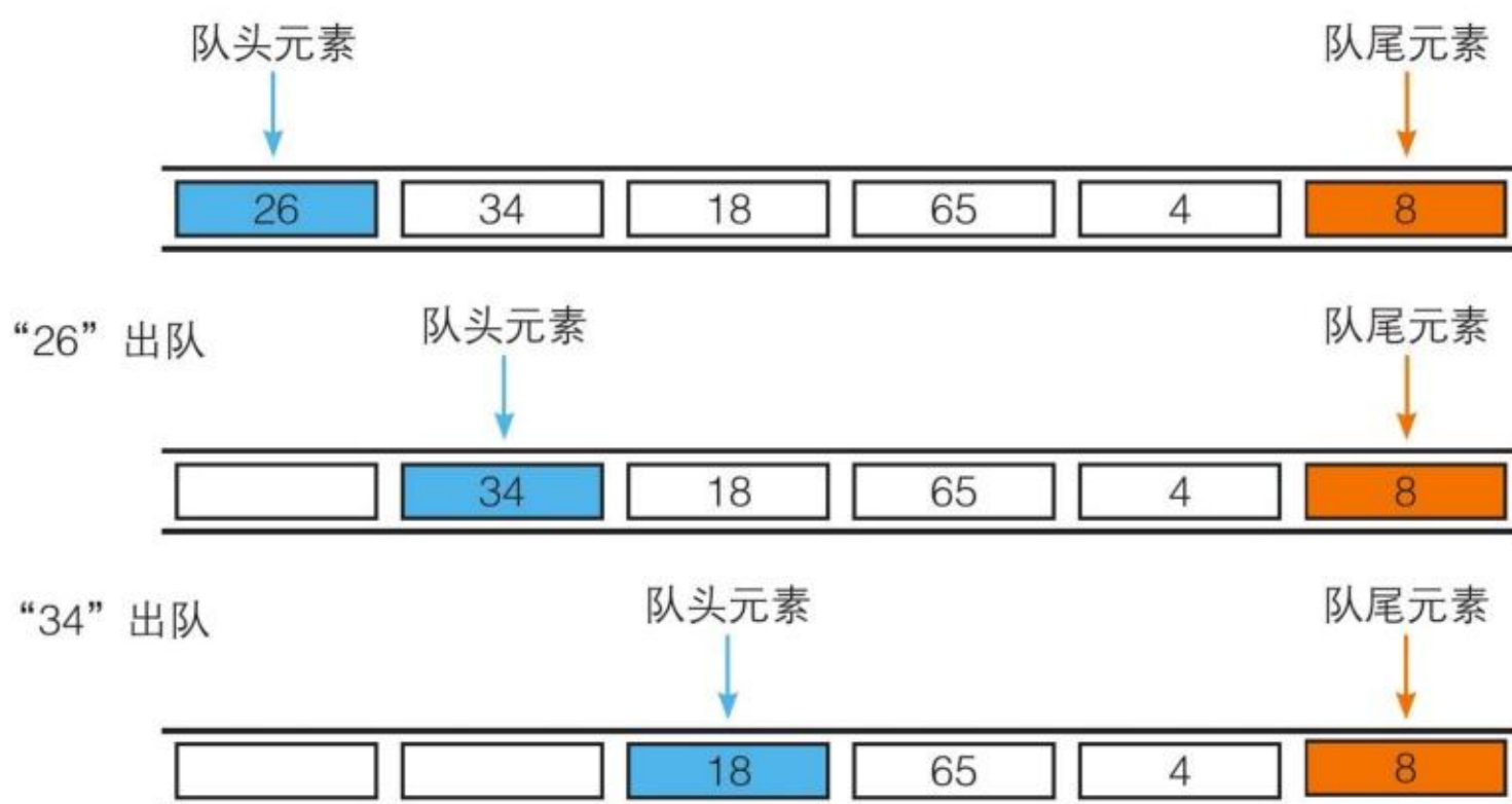
图 3.3.8 队头位置变化时连续出队示意图
