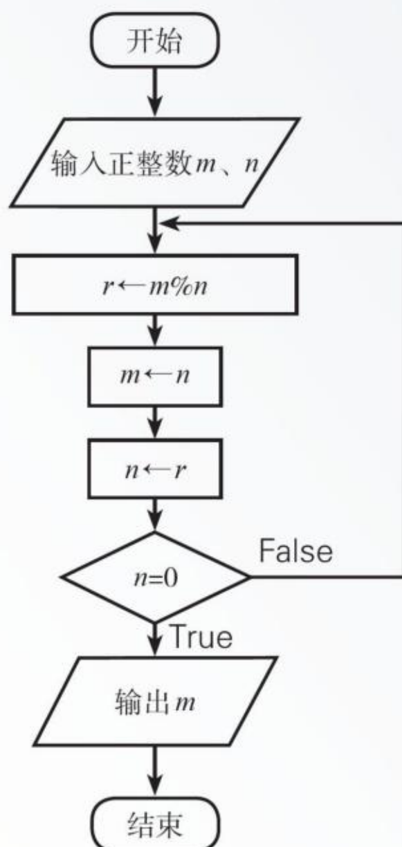
图 4.2.6 求最大公因数的算法流程图
