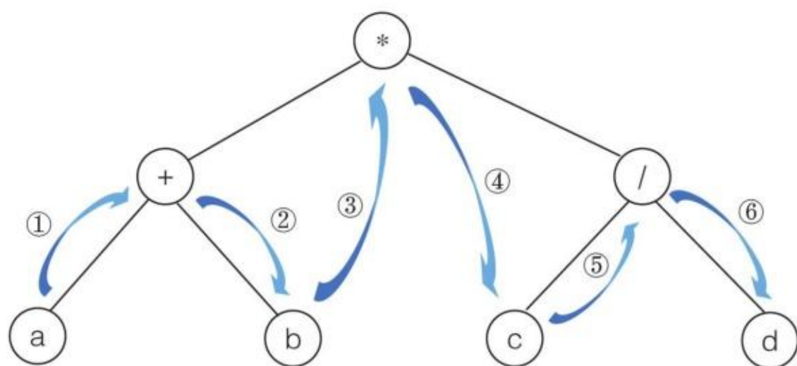
图3.5.15 中根序遍历示意图
