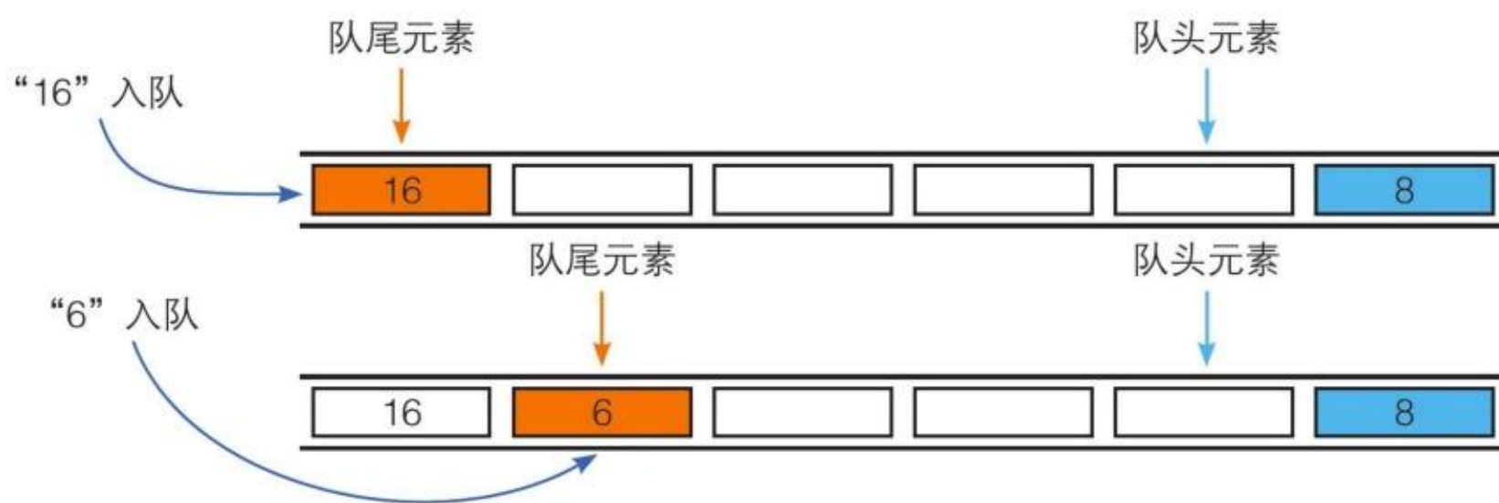
图3.3.10 循环队列连续入队示意图
