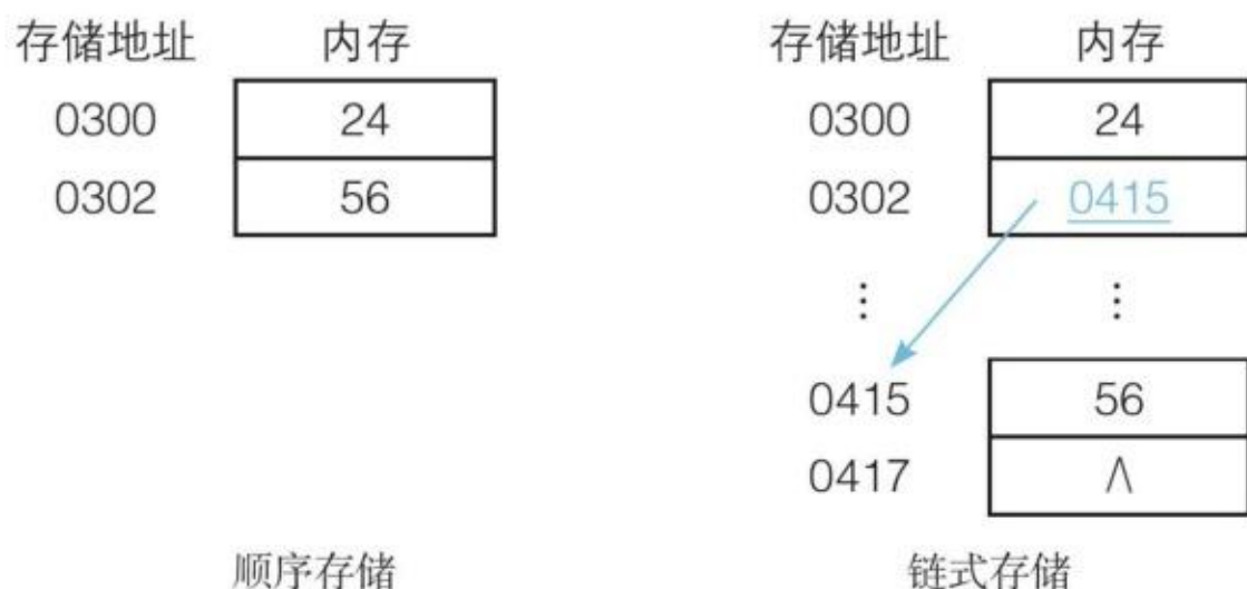
图2.2.2 \langle 24, 56 \rangle 的两种存储方式示意图
