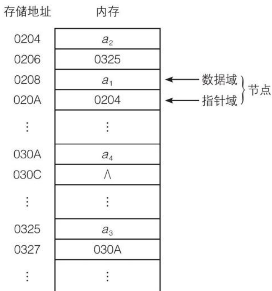
图 2.2.5 链式存储结构示意图
