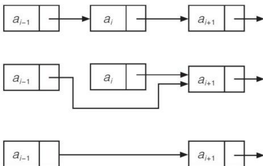
图 2.2.13 删除节点的指针变化示意图
