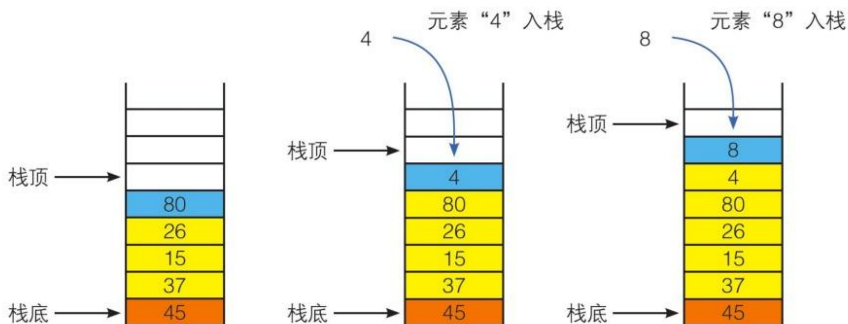
图3.2.9 连续入栈示意图
