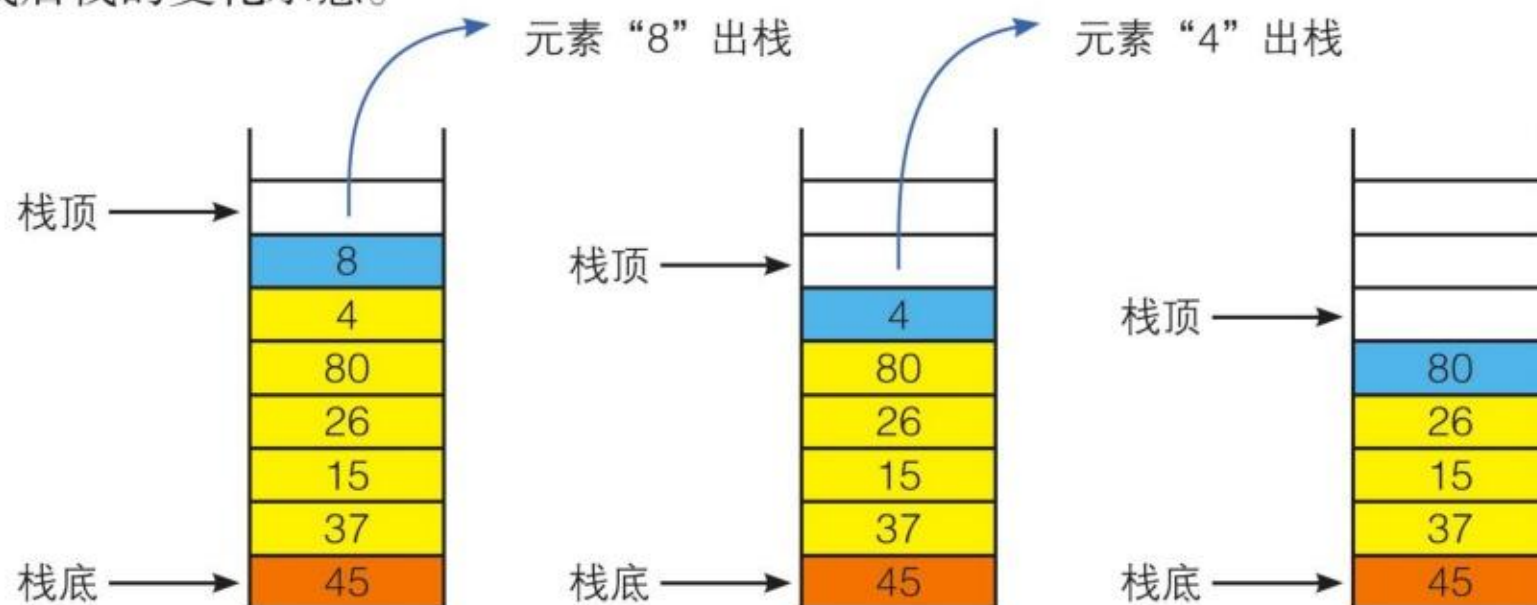
图3.2.10 连续出栈示意图
