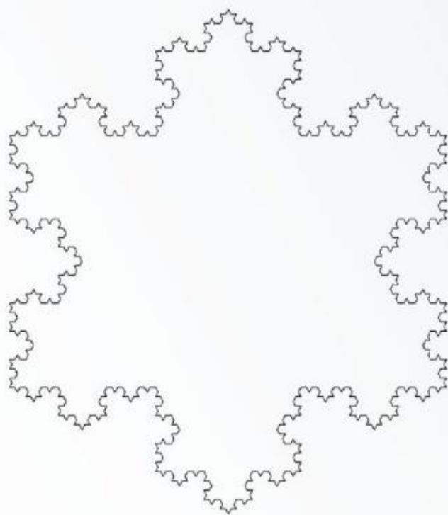
图4.3.9 4阶雪花曲线
