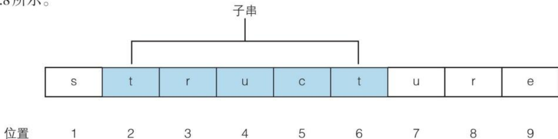
图3.4.8 获取子串
