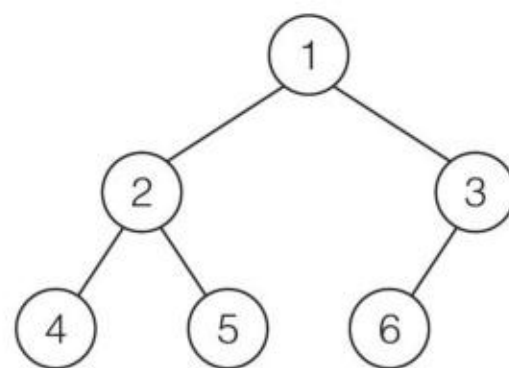
图3.5.10 完全二叉树
