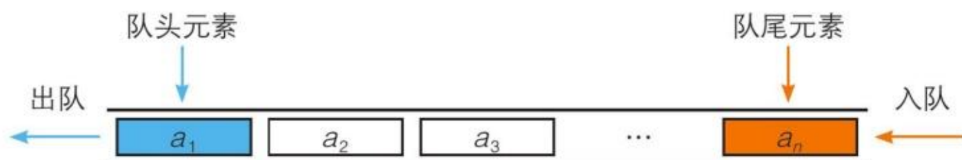
图 3.3.4 队列示意图
