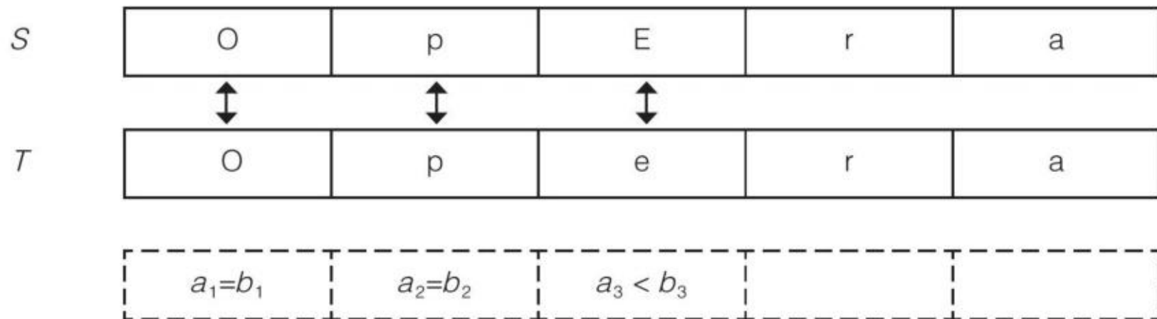
图 3.4.6 字符串比较 (3)
