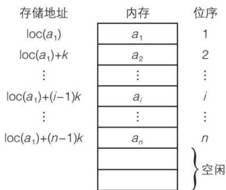
图 2.2.3 顺序存储结构示意图
