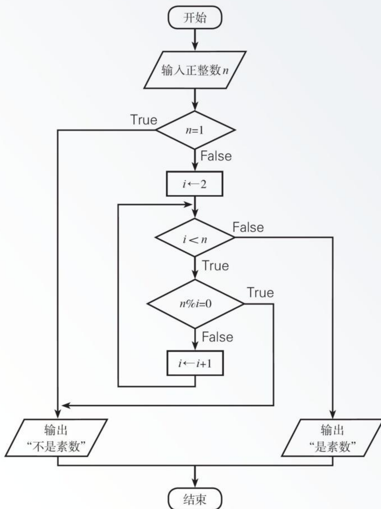
图 4.1.3 素数判断算法流程图
