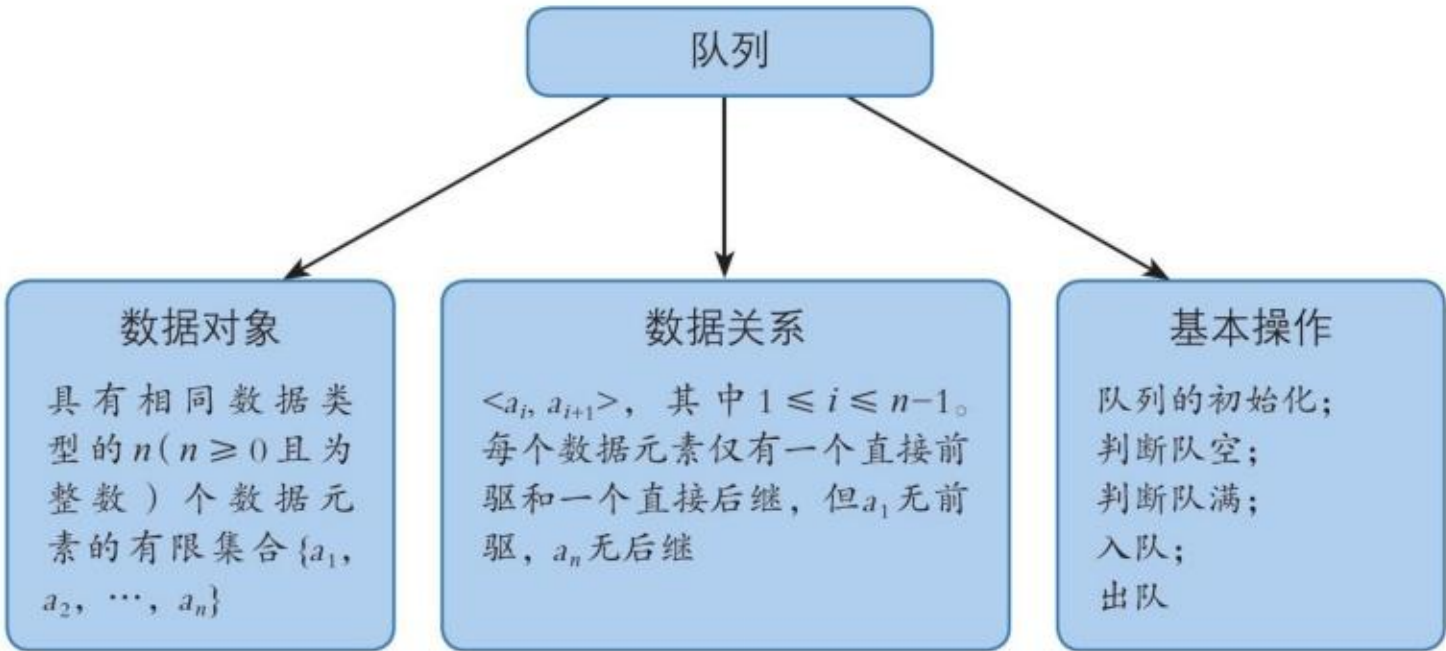
图3.3.5 队列的抽象数据类型定义示意图
