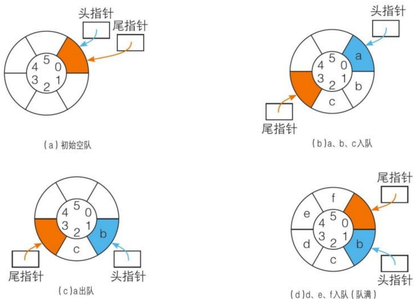
图3.3.11 循环队列示意图
