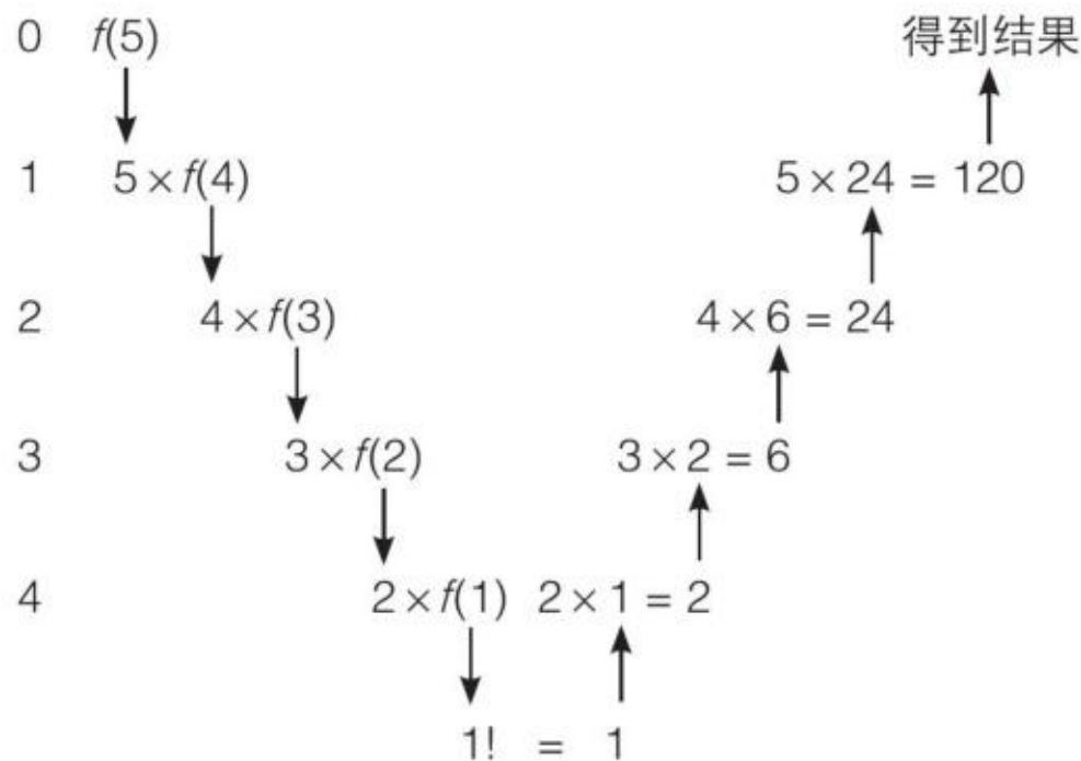
图4.3.2 自然数“5”的阶乘计算过程示意图
