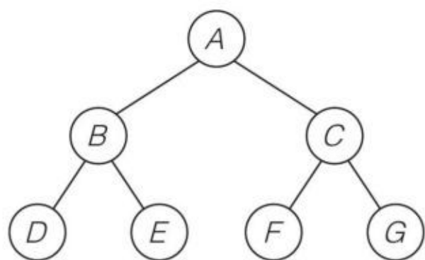
图3.5.8 满二叉树
