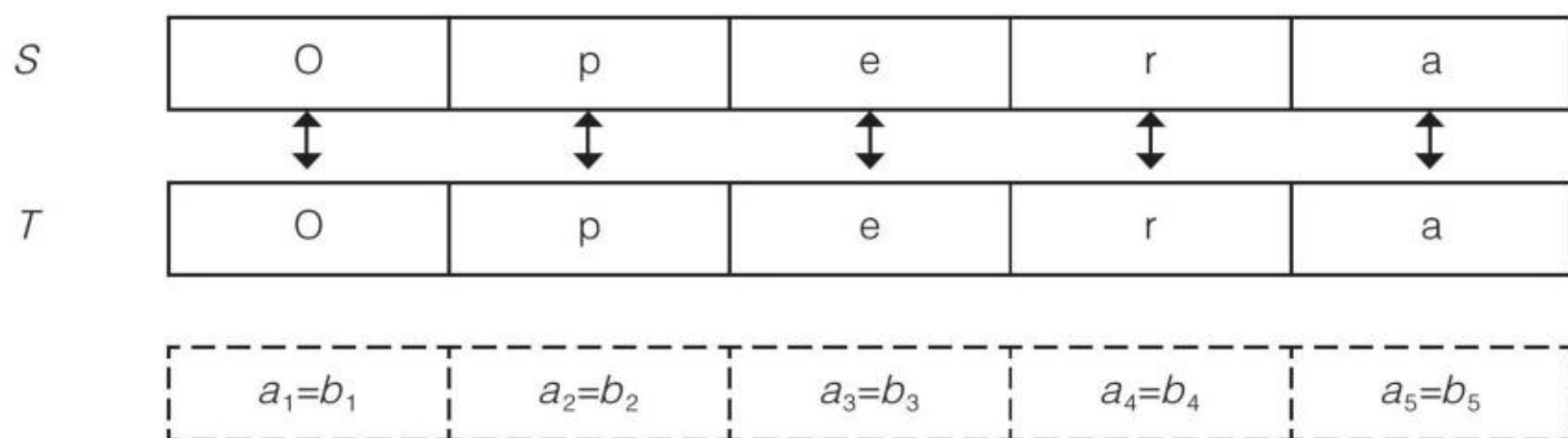
图 3.4.4 字符串比较 (1)
