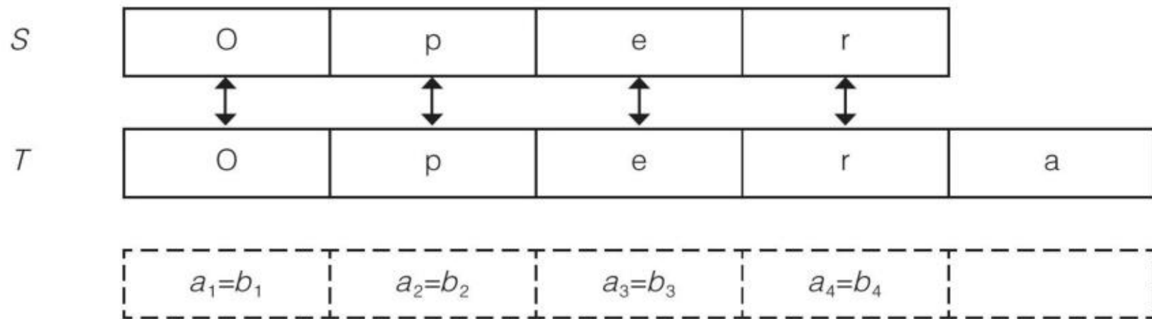
图 3.4.5 字符串比较 (2)
