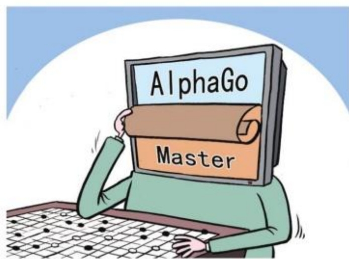
图1.2.2 阿尔法围棋
