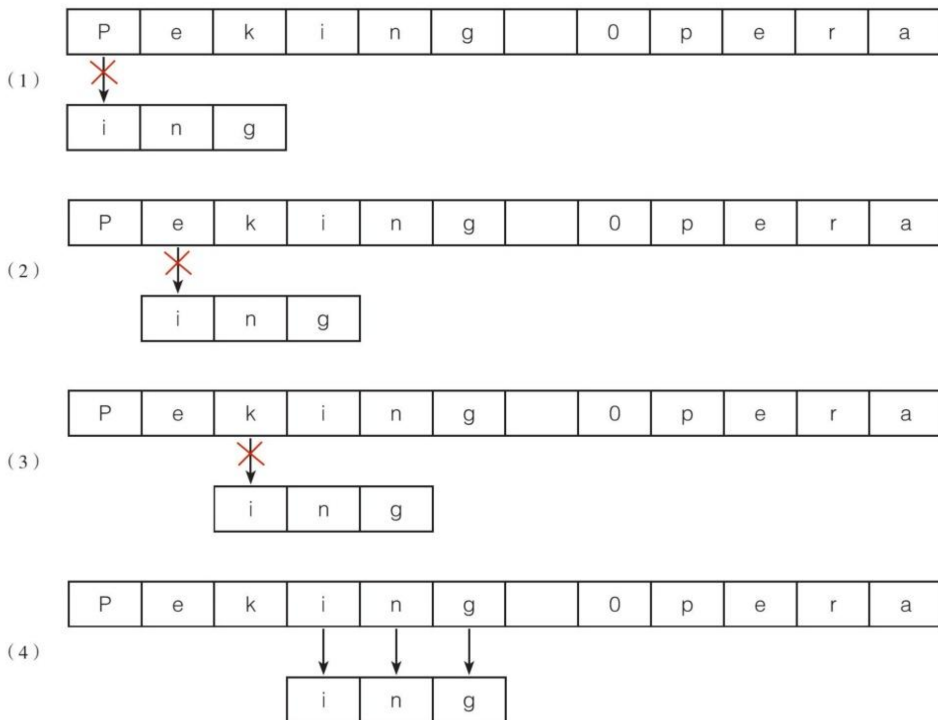
图3.4.9 定位子串
