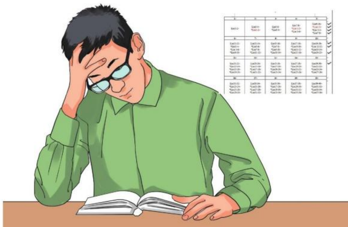
图4.2.1 小明背单词
