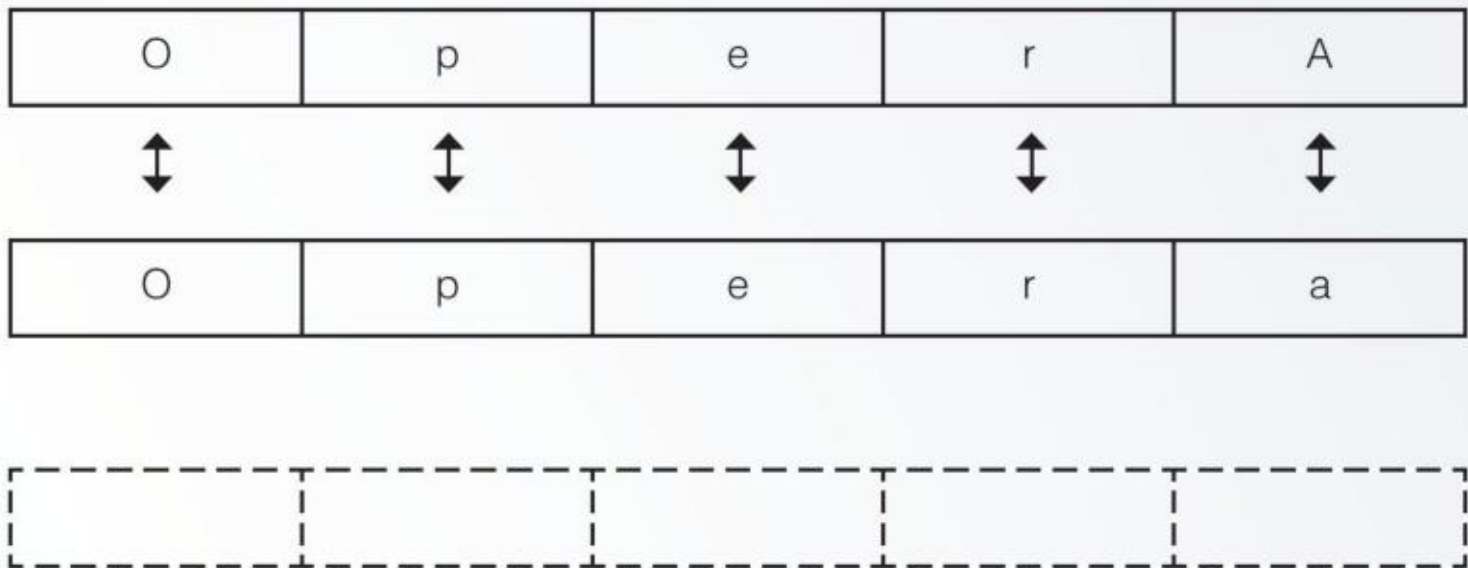
图3.4.7 字符串比较（4）
