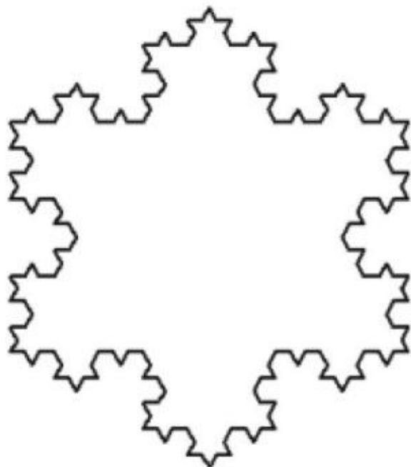
图4.3.7 雪花曲线
