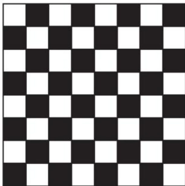
图 1.1.3 棋盘示意图
