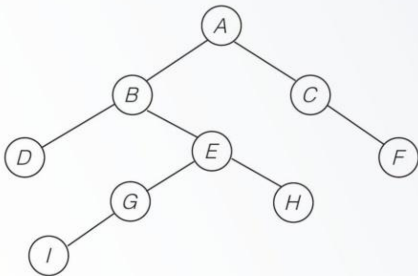
图 3.5.11 二叉树结构
