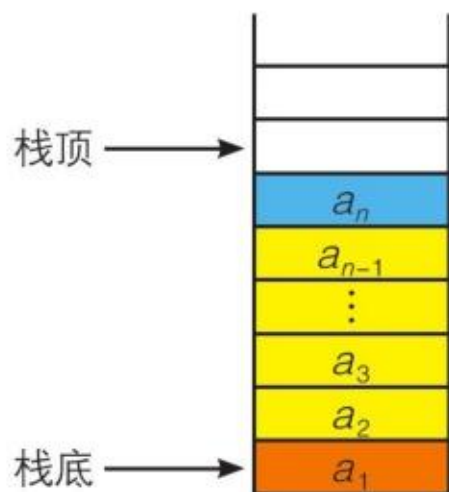
图3.2.4 栈的示意图
