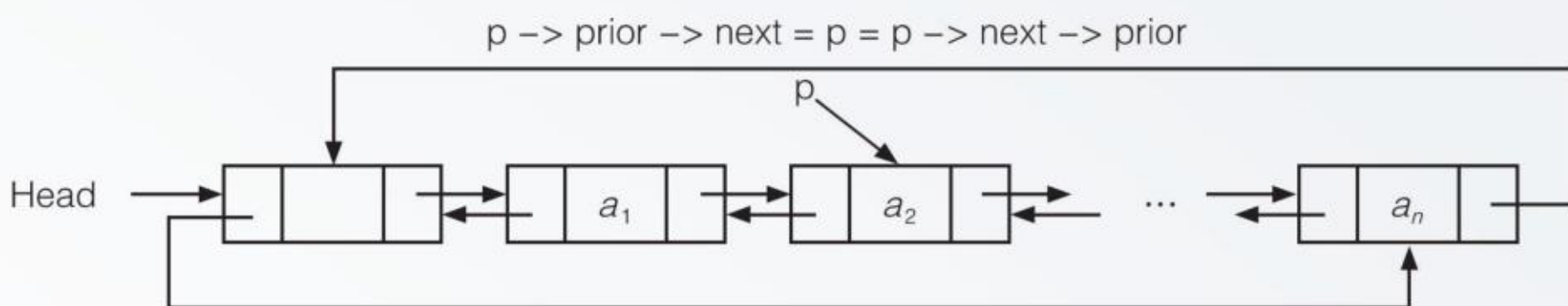
图 3.1.14 具有 n 个节点的双链表示意图
