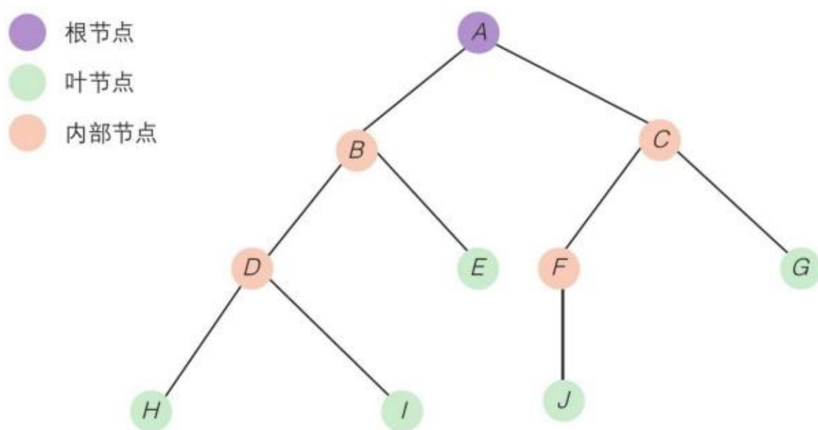
图3.5.4 节点分类示意图
