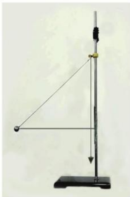
图研-4 水平放置的杆线摆
