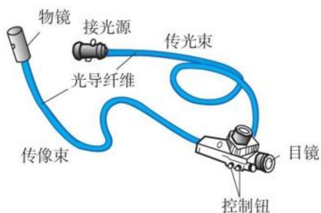
图 4.2-9 内窥镜
