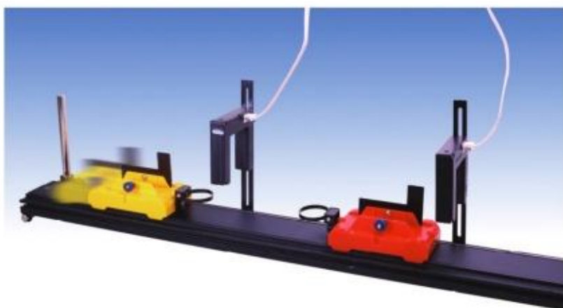
图 1.5-1 研究小车碰撞前后动能的变化
