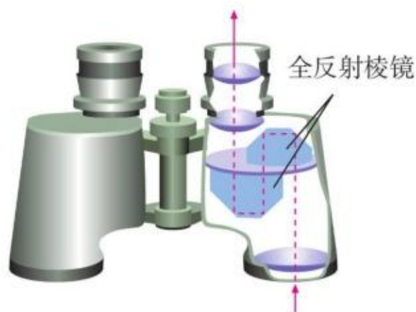
图 4.2-5 双筒望远镜中的全反射棱镜
