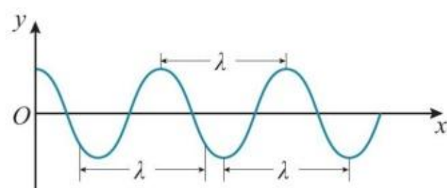
图 3.2-3 波长
