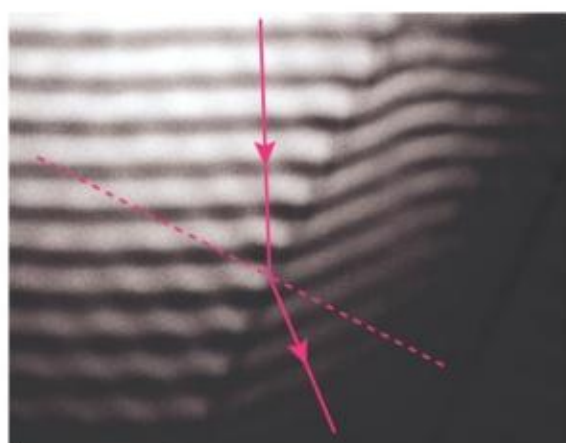
图 3.3-2 水波的折射
