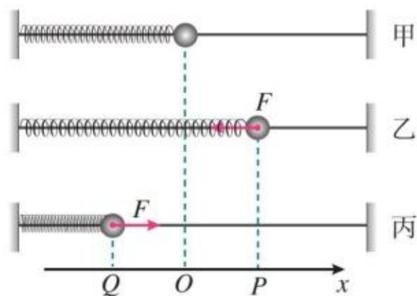
图 2.3-1 简谐运动的回复力
