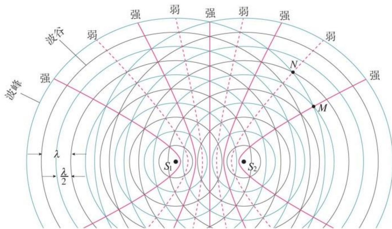
图 3.4-3 波的干涉示意图
