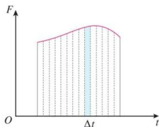
图 1.2-2 变力的冲量
