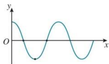
图 3.2-2 横波的图像
