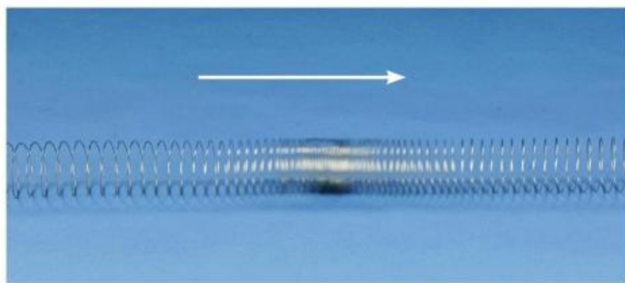
图 3.1-4 弹簧形成的波
