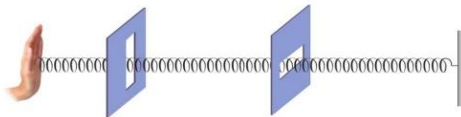
图 4.6-2 纵波可以穿过不同方向的狭缝
