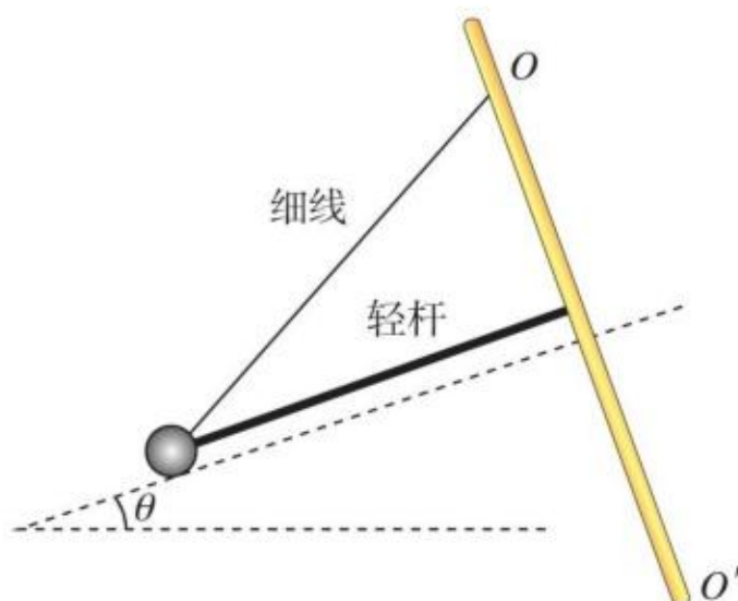
图研-3 杆线摆
