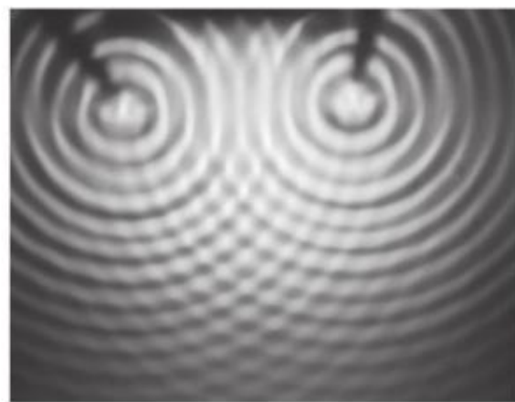
图 3.4-2 水波的干涉图样
