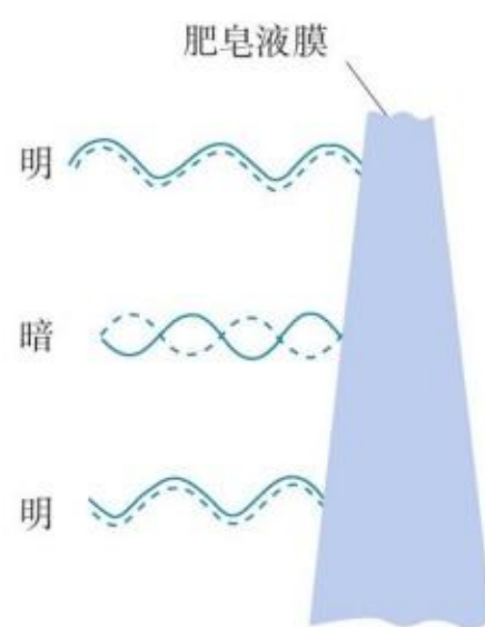
图 4.3-6 薄膜前后两个面的反射光
