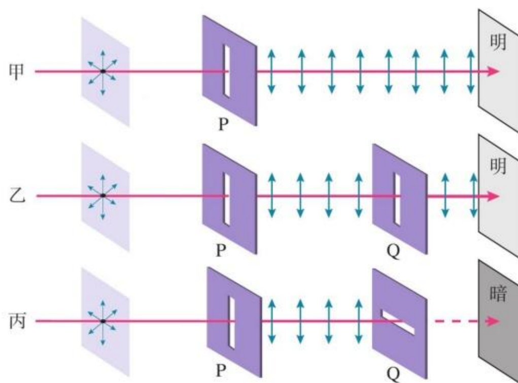
图4.6-3 自然光通过偏振片的实验结果
