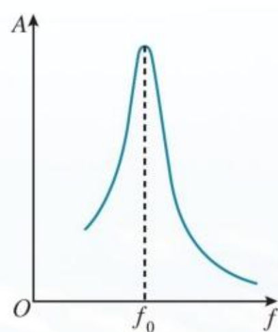
图 2.6-4 受迫振动振幅与驱动力频率的关系
