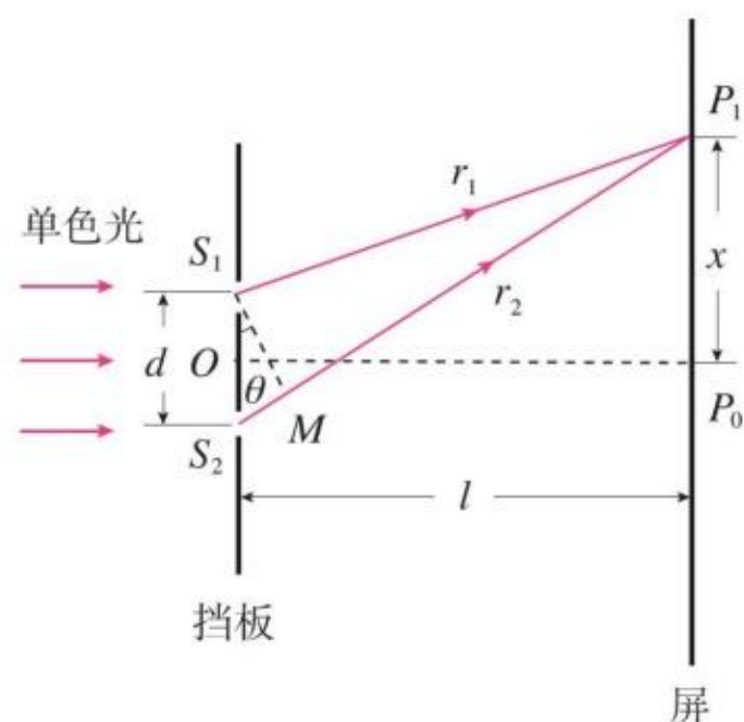
图 4.3-4 导出相邻亮条纹距离的表达式
