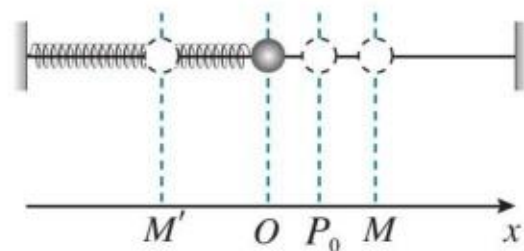
图 2.2-2 简谐运动的振幅
