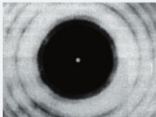
图 4.5-6 泊松亮斑
