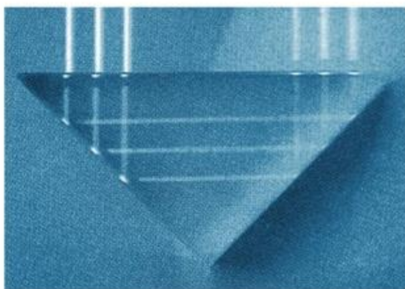
图 4.2-4 全反射棱镜
