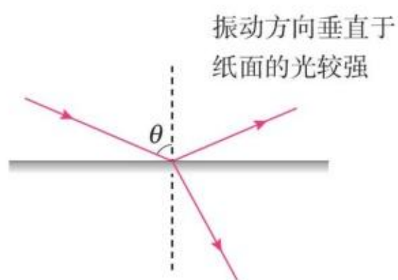
图 4.6-5 反射引起自然光的偏振
