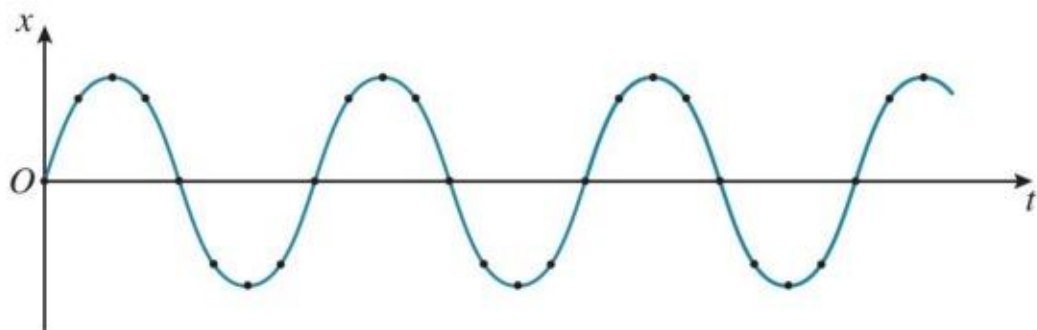
图 2.1-3 振动图像
