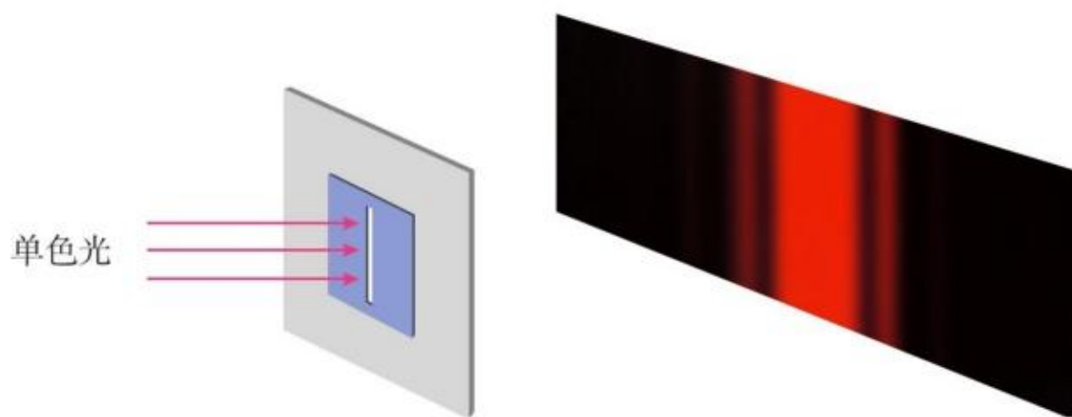
图 4.5-1 单缝衍射示意图
