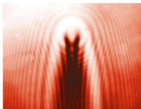
图 4.5-4 光经过大头针尖时的衍射照片
