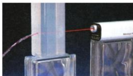
图 4.2-10 水流导光
