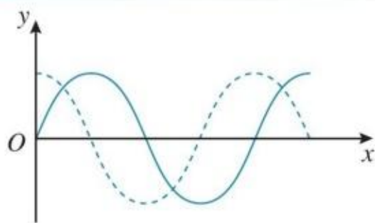
图 3.2-4 不同时刻的波形图
