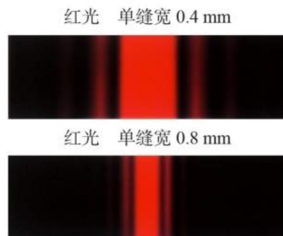
图 4.5-2 单缝衍射产生的图样
