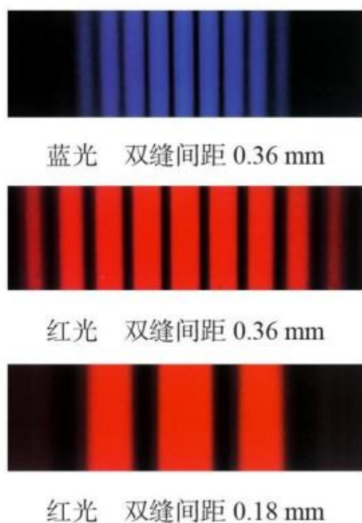
图 4.4-4 不同色光、不同双缝的双缝干涉条纹
