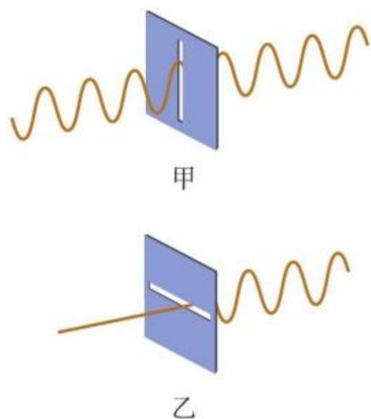
图 4.6-1 狭缝的方向影响横波的传播
