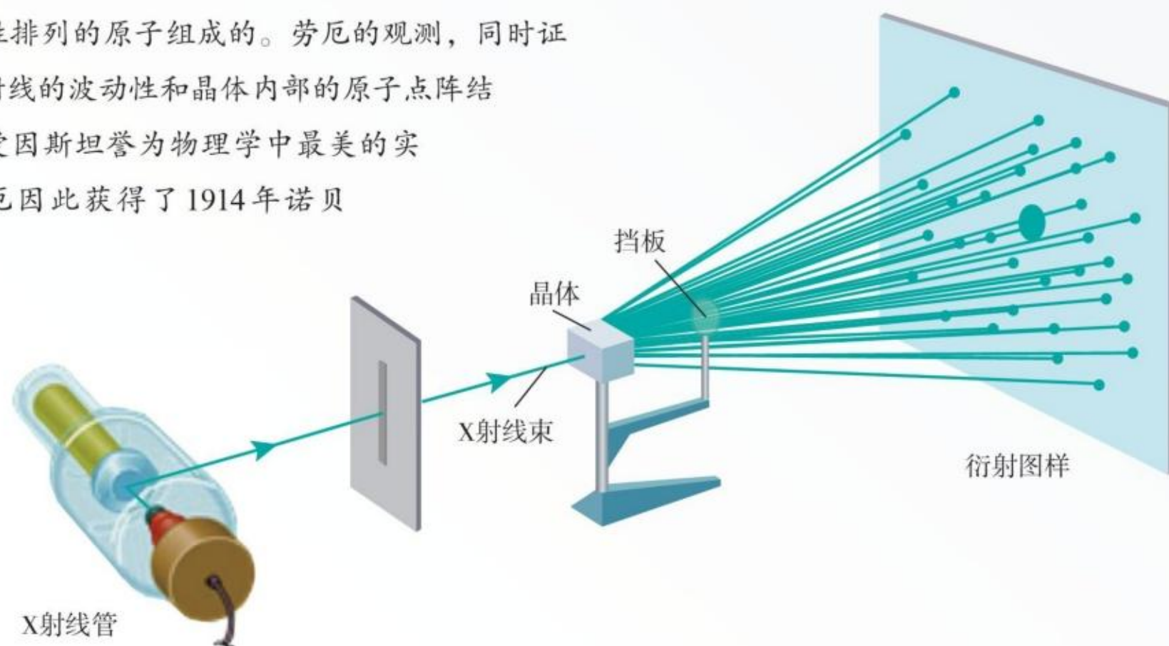
图 4.5-7 X 射线晶体衍射实验示意图
