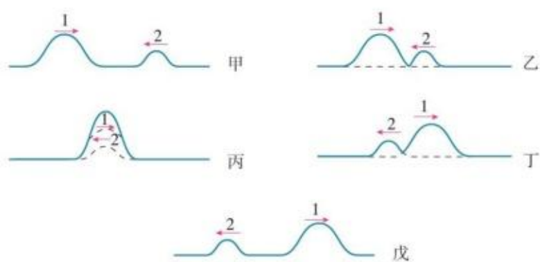
图 3.4-1 波的叠加
