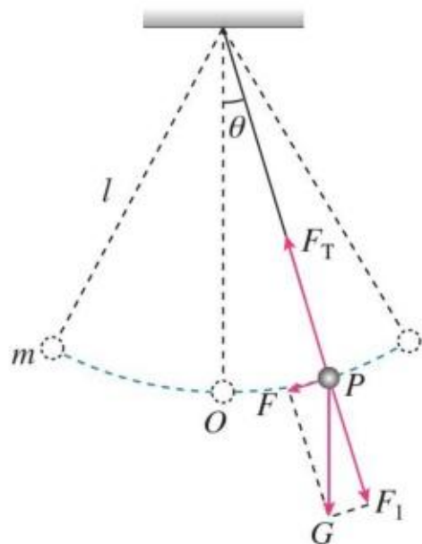
图 2.4-1 分析单摆的回复力
