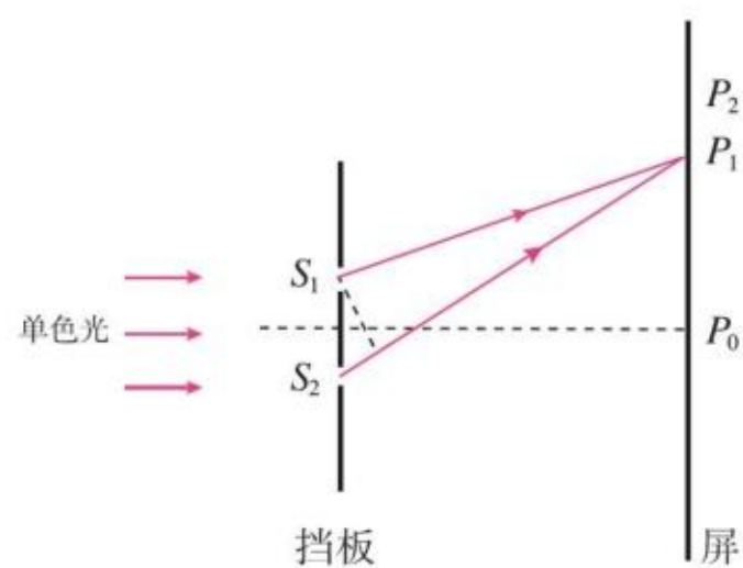
图 4.3-3 双缝干涉的原理图
