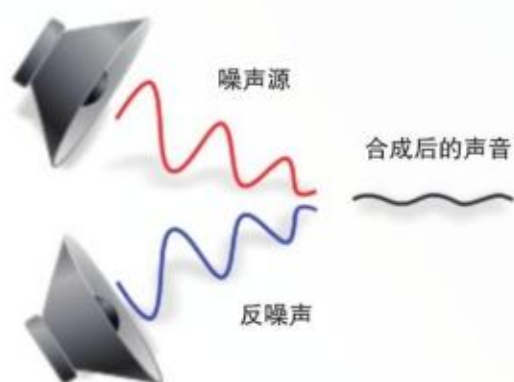
图 3.4-4 消声原理
