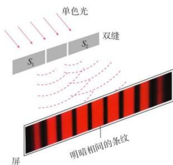
图 4.3-2 双缝干涉的示意图
