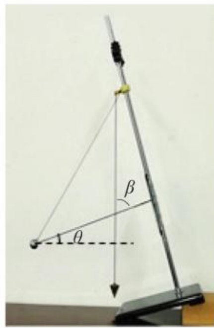
图研-5 倾斜放置的杆线摆
