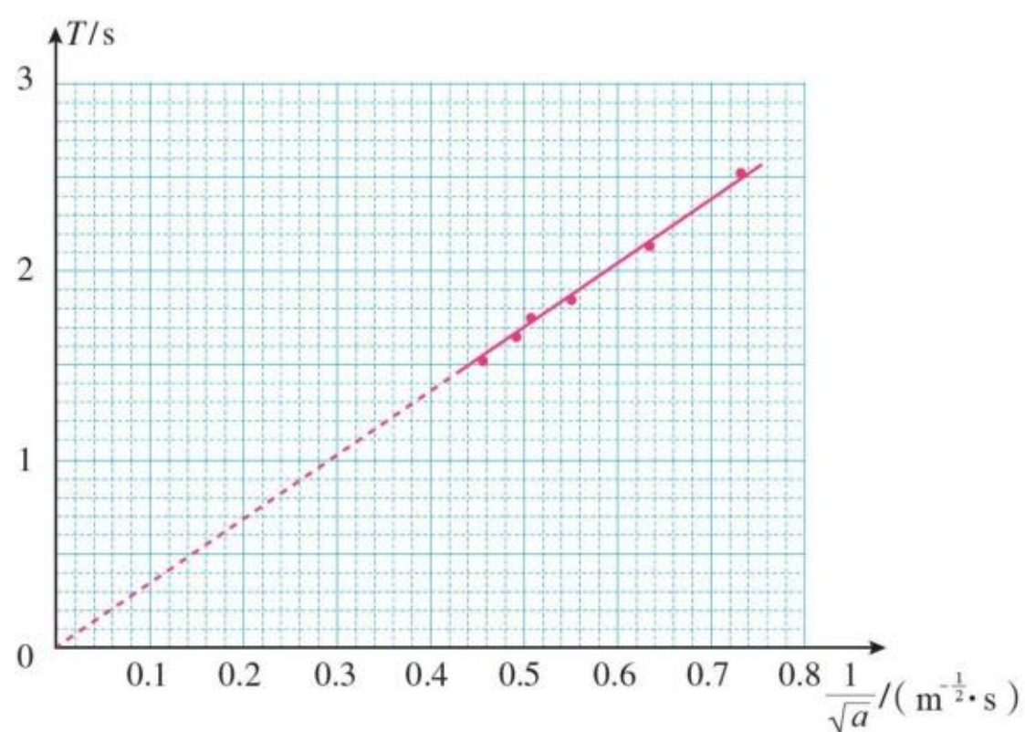
图研-6 T - \frac{1}{\sqrt{a}} 图像
