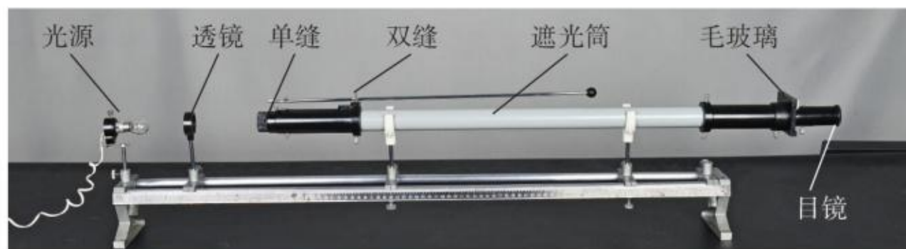
图 4.4-1 双缝干涉的实验装置
