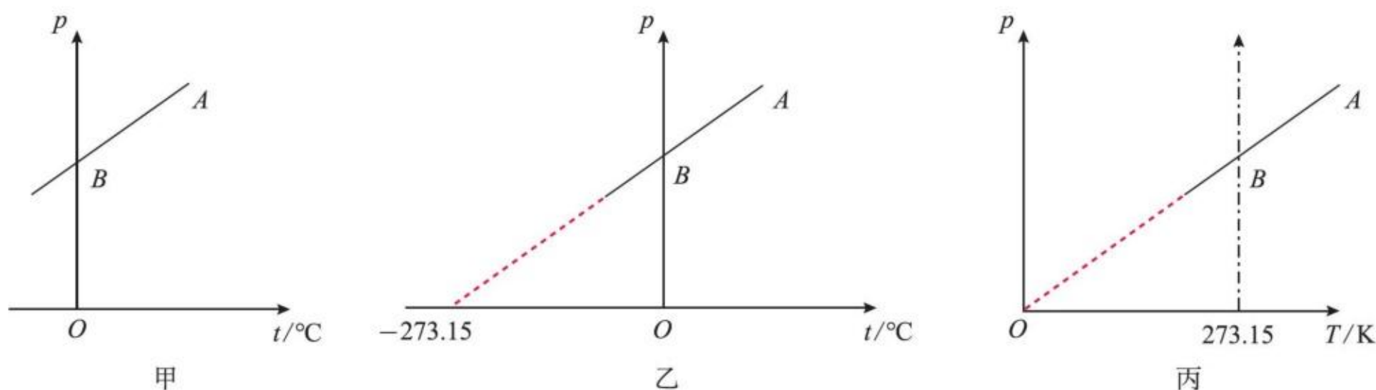
图2.3-2 气体等容变化的 p - T 图像
