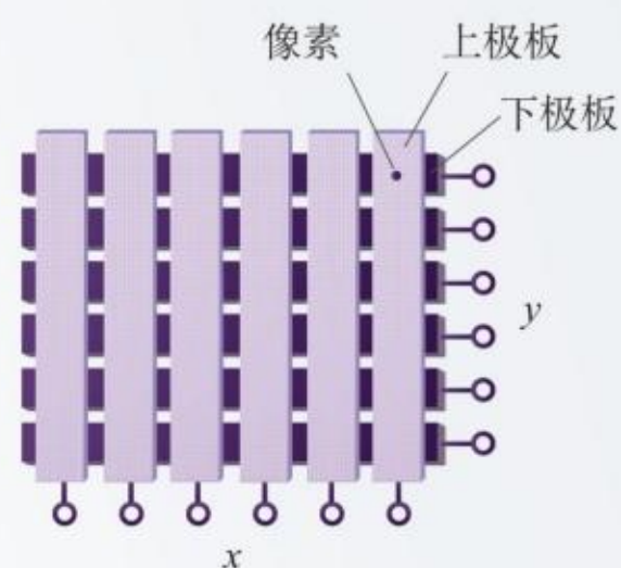
图2.5-11 像素矩阵显示中的条形电极
