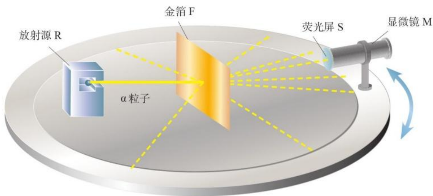
图 4.3-3 \alpha 粒子散射的实验装置示意图
