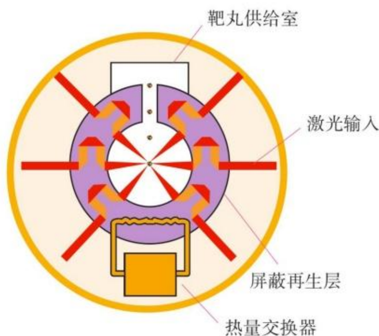
图 5.4-11 惯性约束示意图
