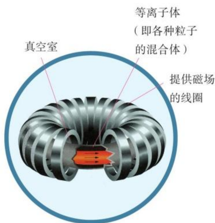
图 5.4-9 环流器的结构示意图
