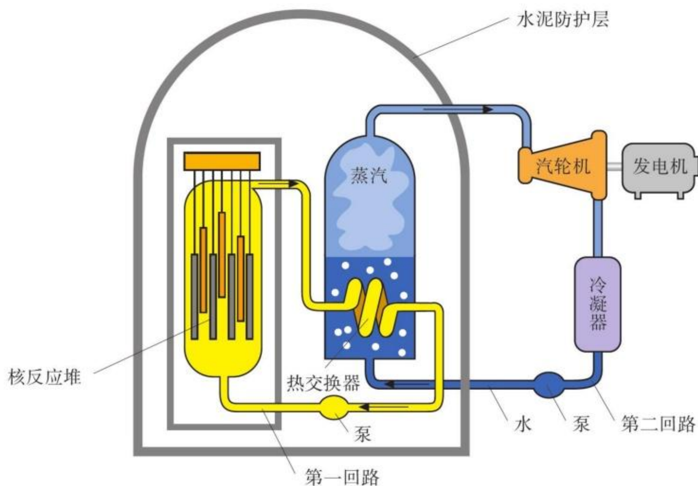
图 5.4-5 核电站工作流程
