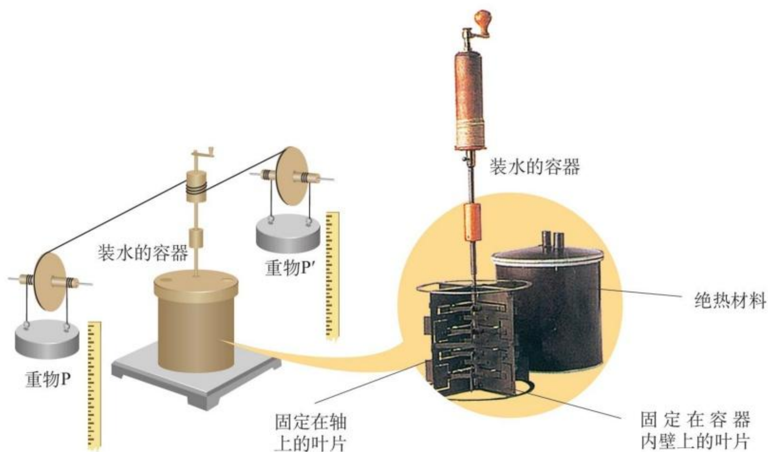
图 3.1-1 焦耳的实验装置
