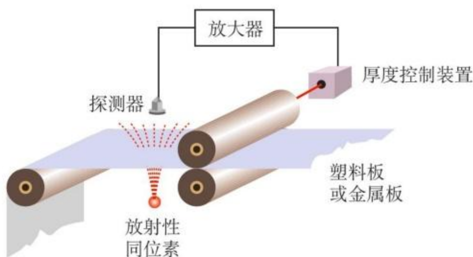
图 5.2-5 射线测厚装置
