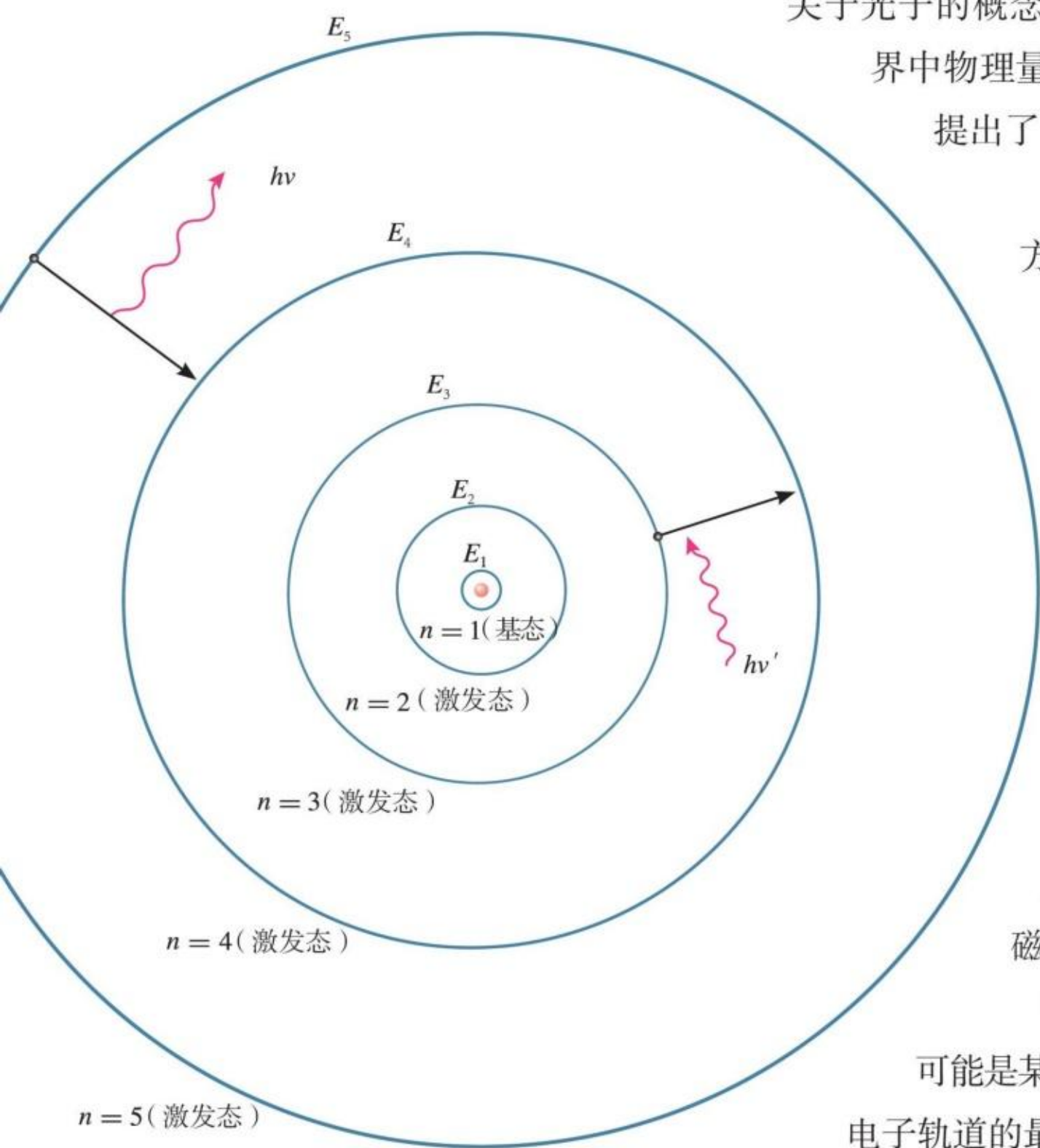
图4.4-5 氢原子的电子轨道示意图
