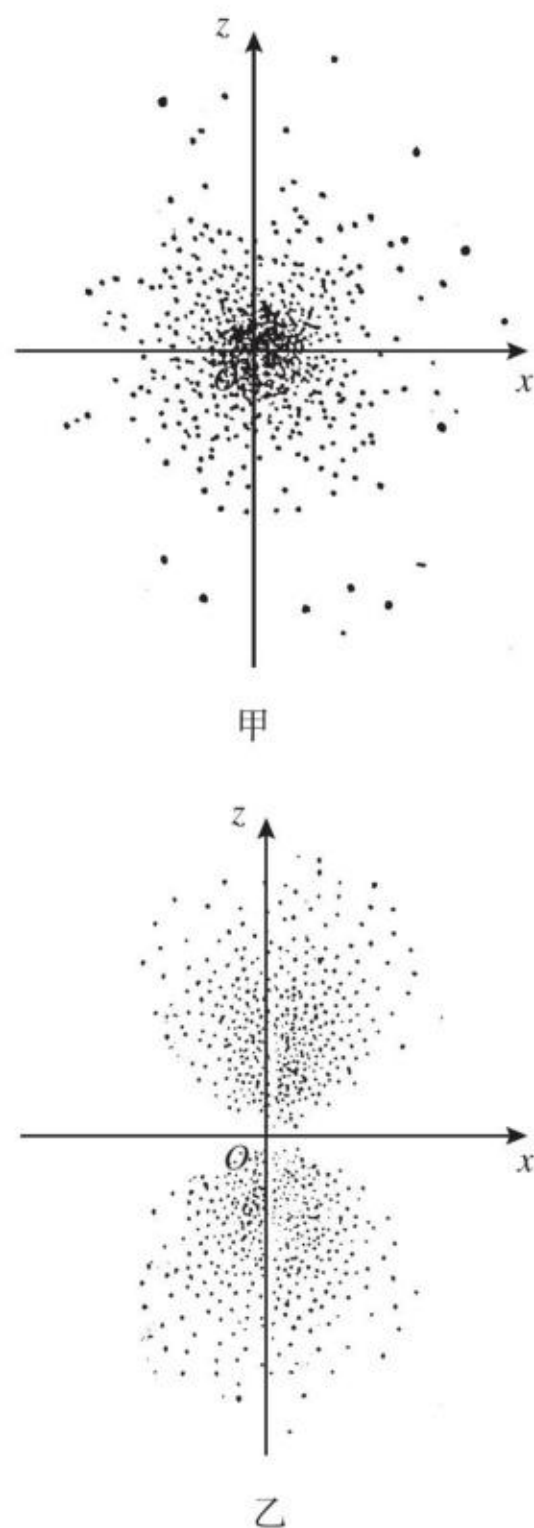
图 4.4-8 氢原子电子云示意图
