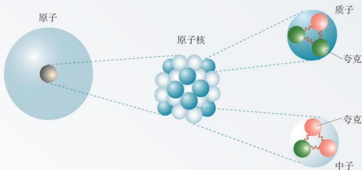
图5.5-2 原子核结构
