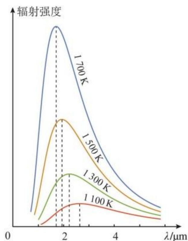
图 4.1-2 黑体辐射的实验规律
