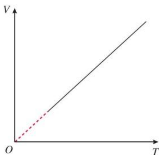
图2.3-1 压强不变时体积与温度的关系
