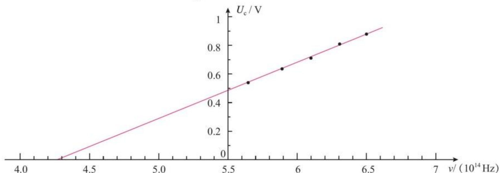
图 4.2-5 某金属的 U_c - \nu 图像
