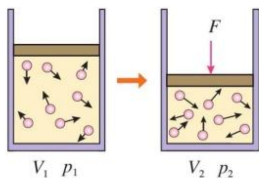
图2.3-3 等温变化
