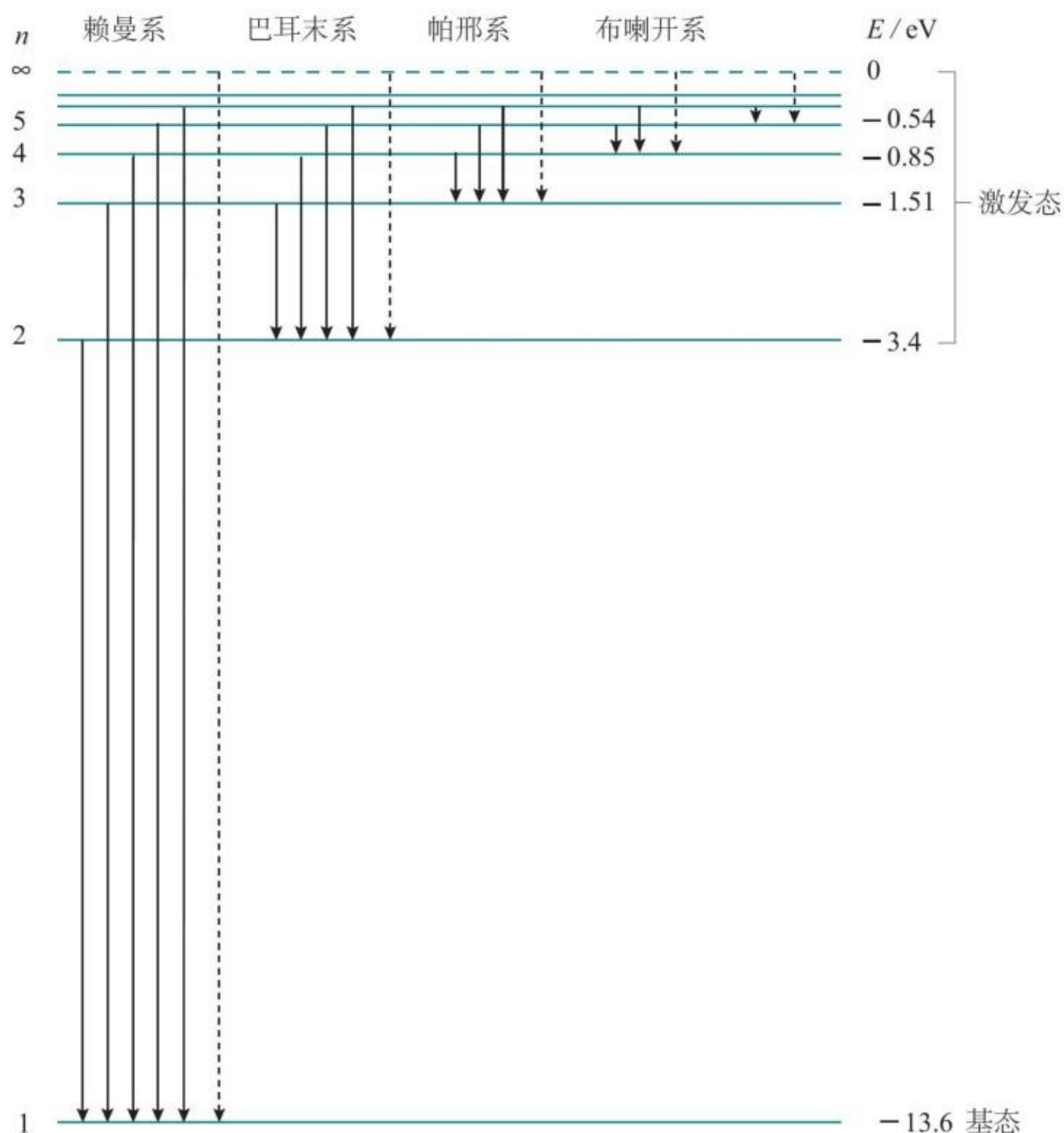
图 4.4-6 氢原子能级图
