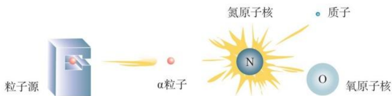
图 5.1-4 \alpha 粒子轰击氮原子核示意图
