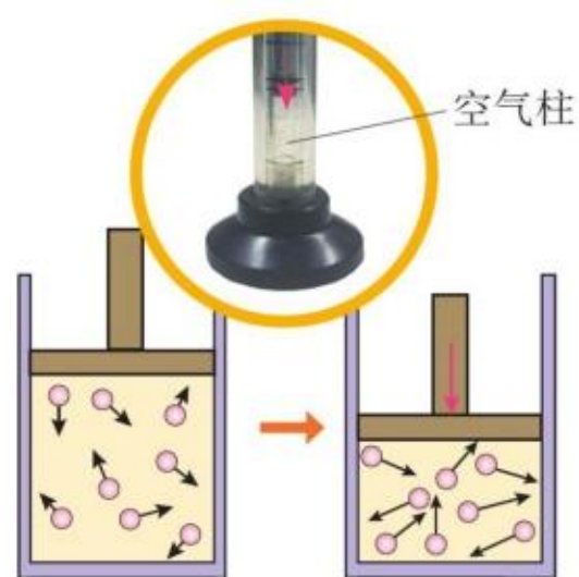
图3.1-3 绝热压缩
