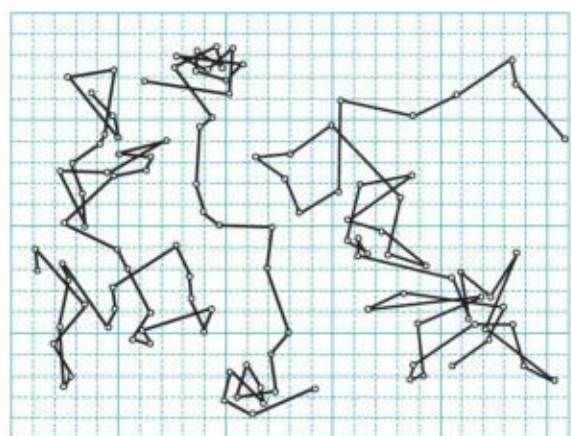
图 1.1-4 三颗微粒运动位置的连线
