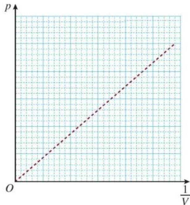
图2.2-3 检验 p 与 \frac{1}{V} 的线性关系
