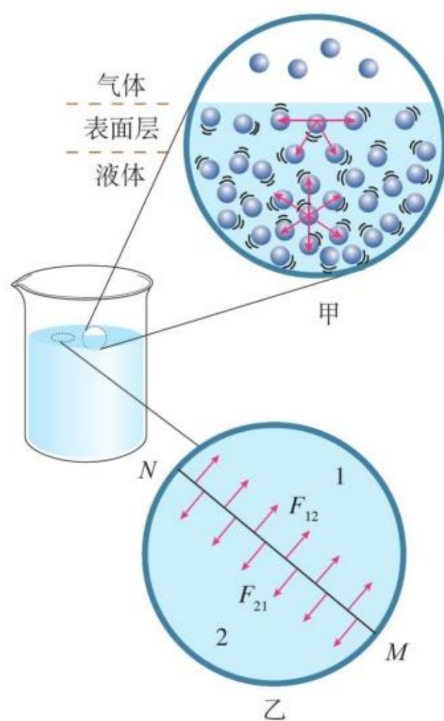
图2.5-3 液体的表面张力
