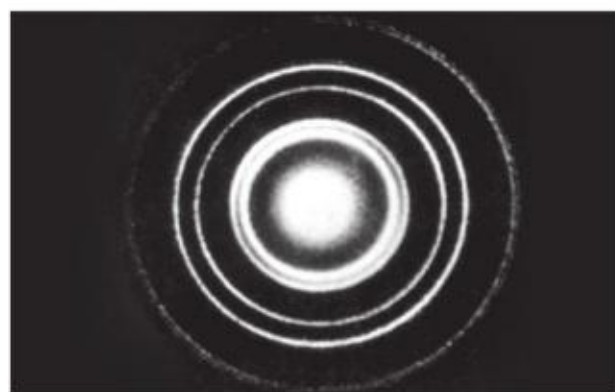
图4.5-1 电子束穿过铝箔后的衍射图样
