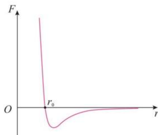
图 1.1-7 分子间作用力与分子间距离的关系
