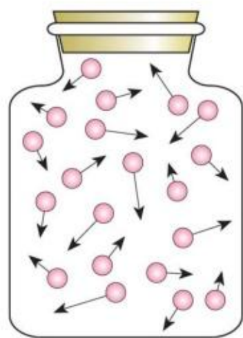
图 1.3-1 气体分子运动的示意图
