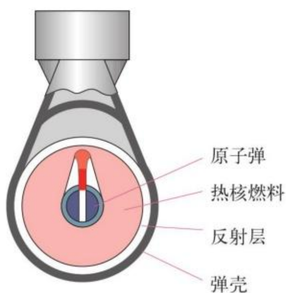
图 5.4-8 氢弹原理图
