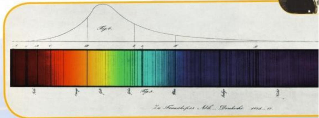
夫琅禾费线
