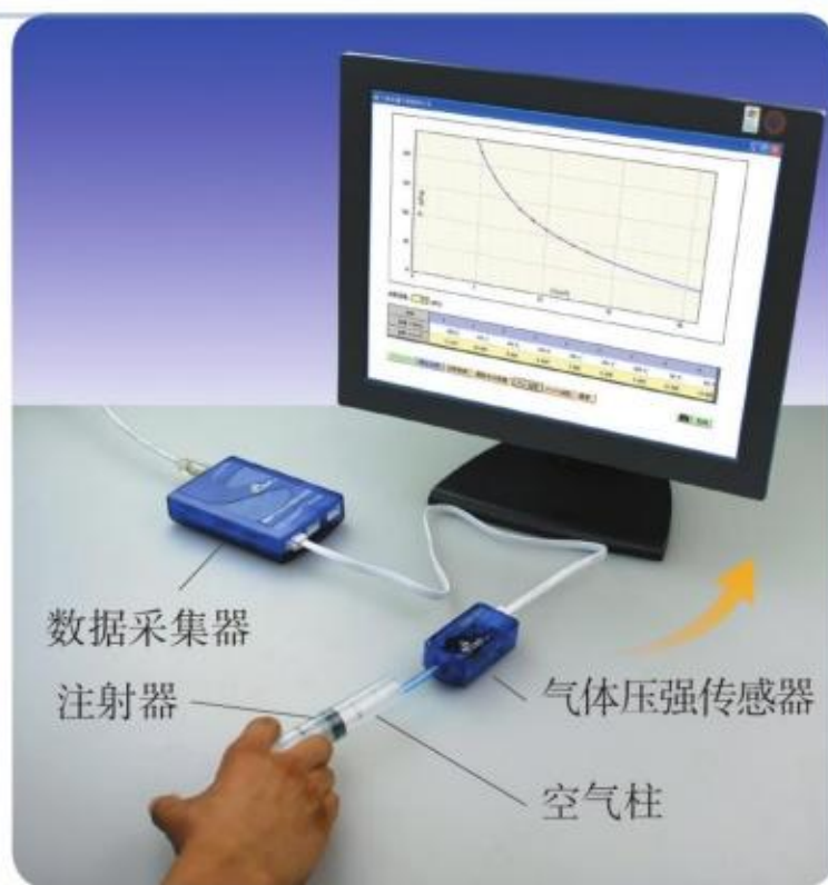
图2.2-4 用传感器探究气体等温变化的规律
