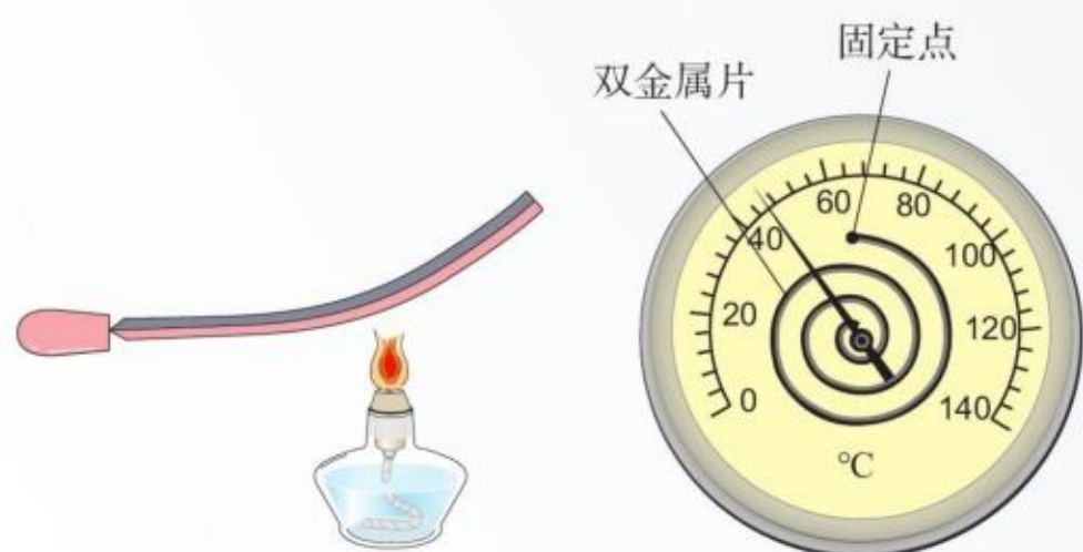
图 2.1-3 双金属温度计
