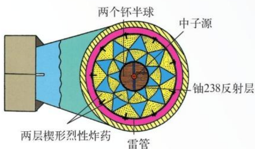
图 5.4-3 内爆式原子弹示意图
