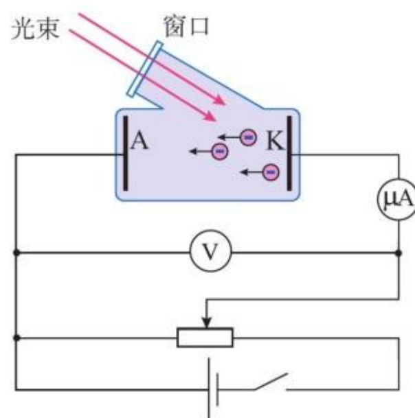
图4.2-1 研究光电效应的电路图
