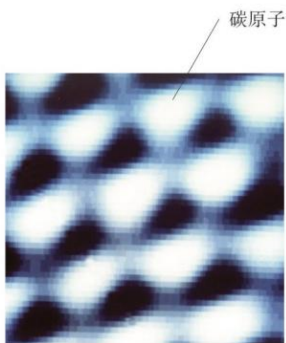
图1.1-1 石墨表面原子的照片
