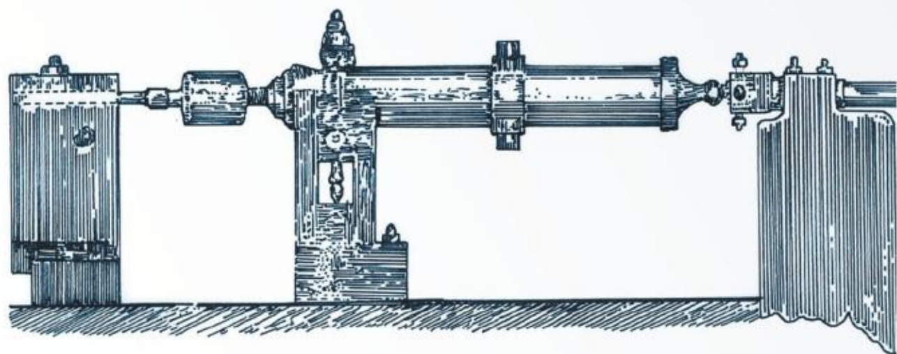
图3.2-3 伦福德的炮筒镗孔实验
