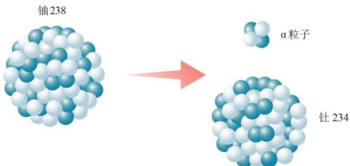
图 5.2-1 \alpha 衰变
