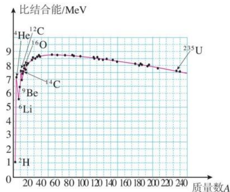
图 5.3-4 原子核的比结合能
