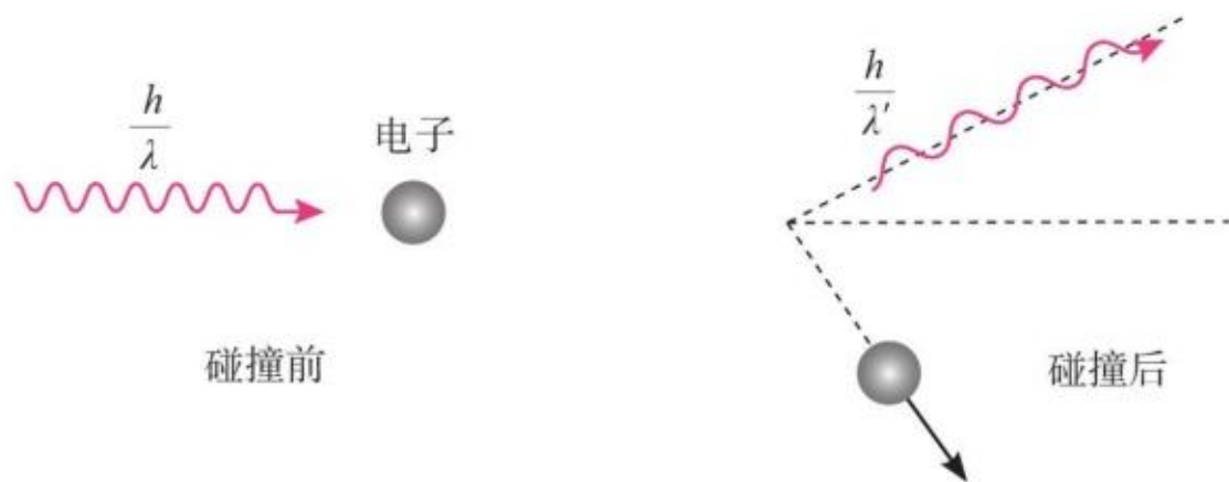
图 4.2-6 光子既有能量也有动量
