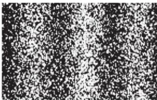
图4.5-2 电子干涉条纹
