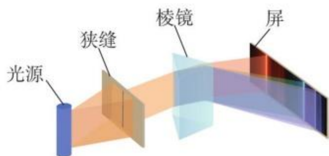
图 4.4-1 光谱的形成
