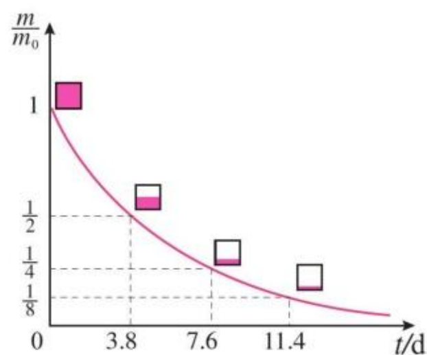
图 5.2-4 氡的衰变
