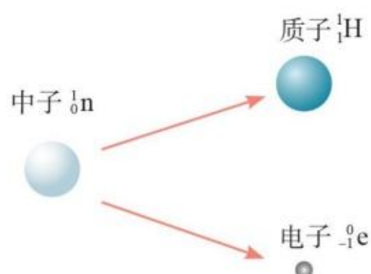
图 5.2-3 中子的转化
