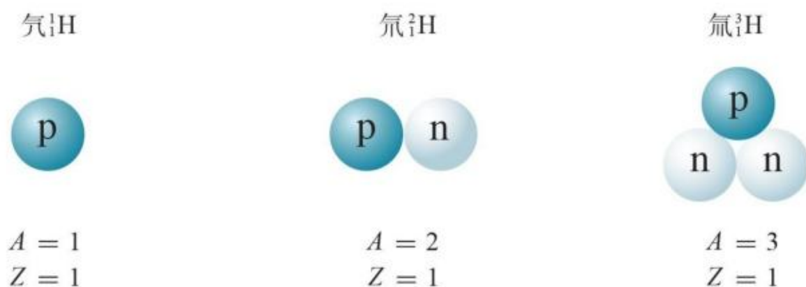
图5.1-7 氢的同位素
