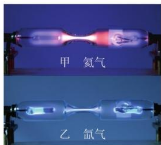
图 4.4-7 气体放电管中的气体导电时会发光
