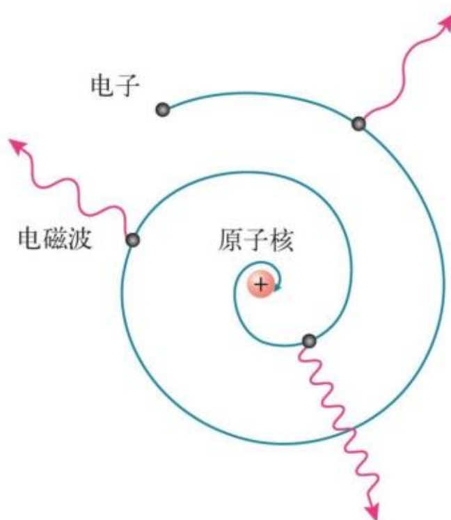
图 4.4-4 电子绕核转动的经典图景
