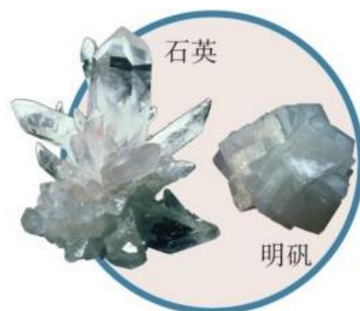
图2.4-3 晶体的外形
