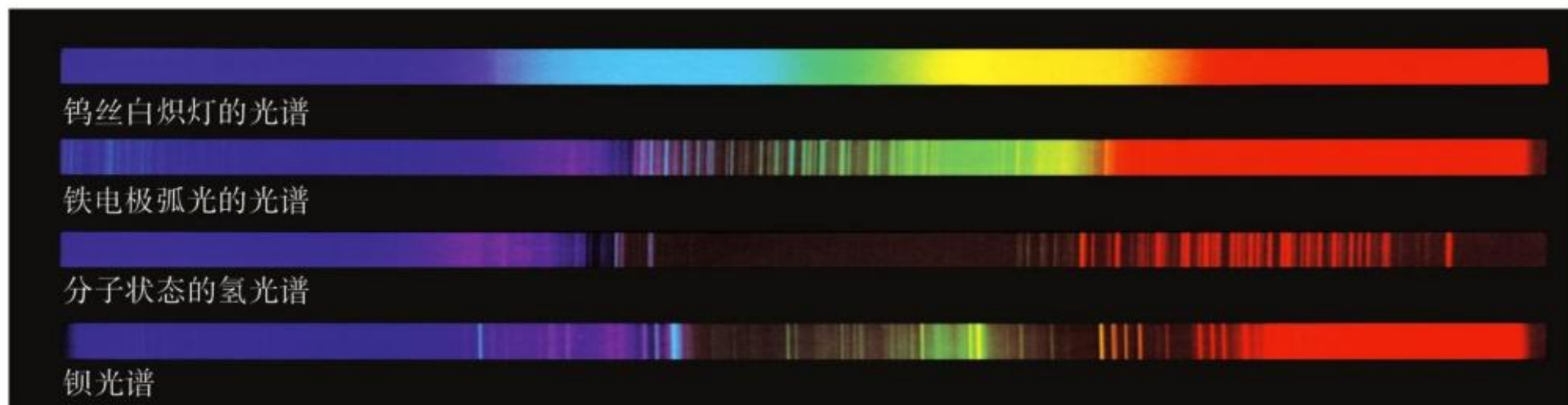
图 4.4-2 几种光谱
