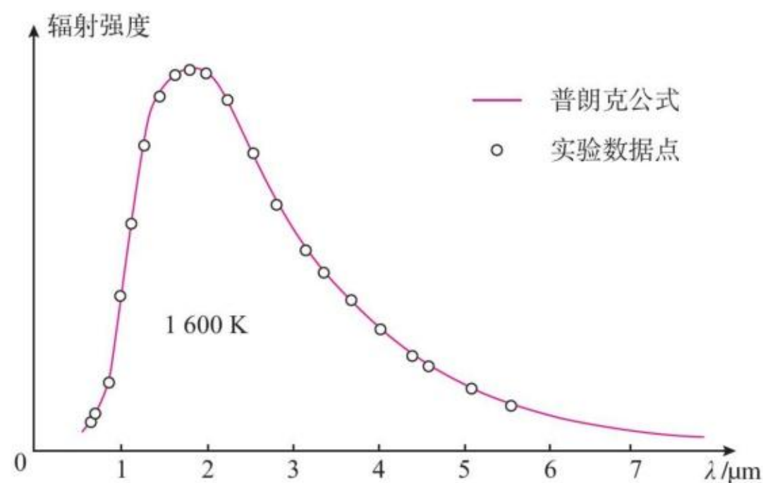
图 4.1-3 普朗克公式与实验结果的比较
