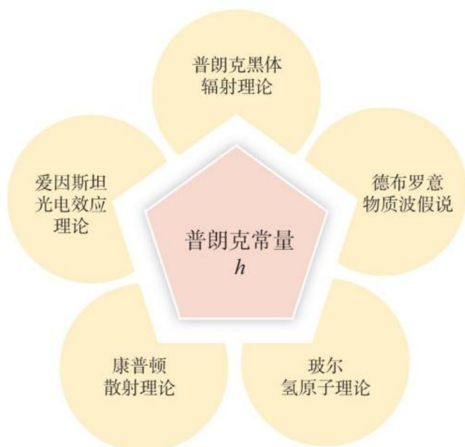
图 4.5-3 一系列理论都和普朗克常量紧密相关 人们需要建立描述微观世界的物理理论。
