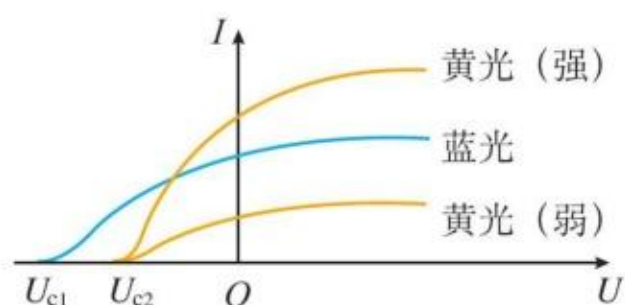
图4.2-2 光电流与电压的关系
