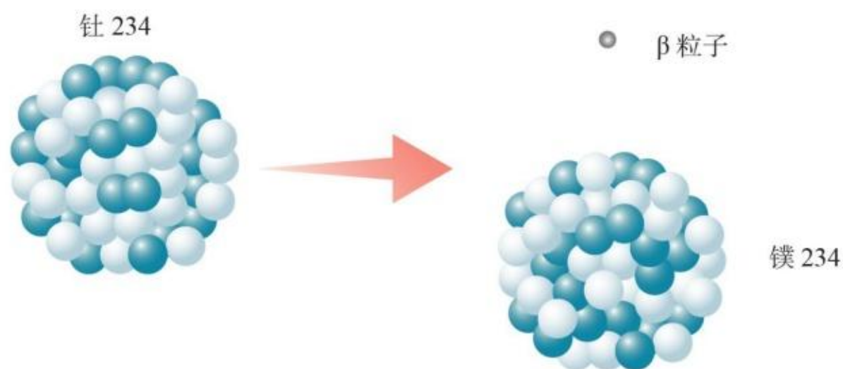
图 5.2-2 \beta 衰变
