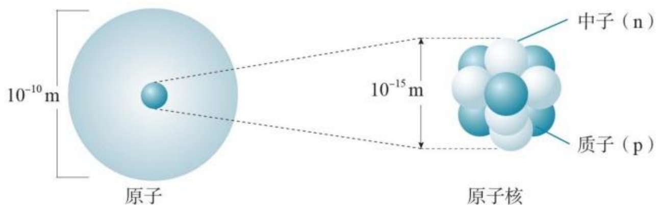
图 5.1-5 原子核的示意图
