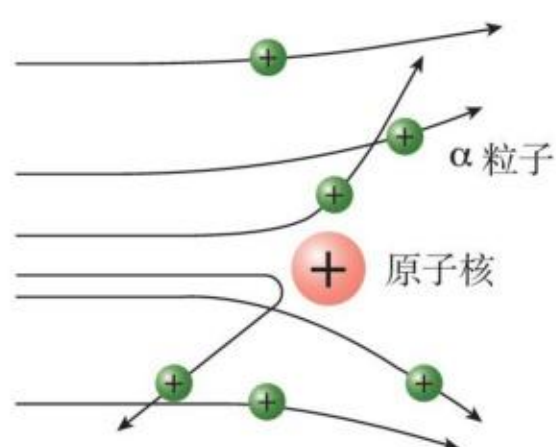
图 4.3-4 \alpha 粒子散射图景
