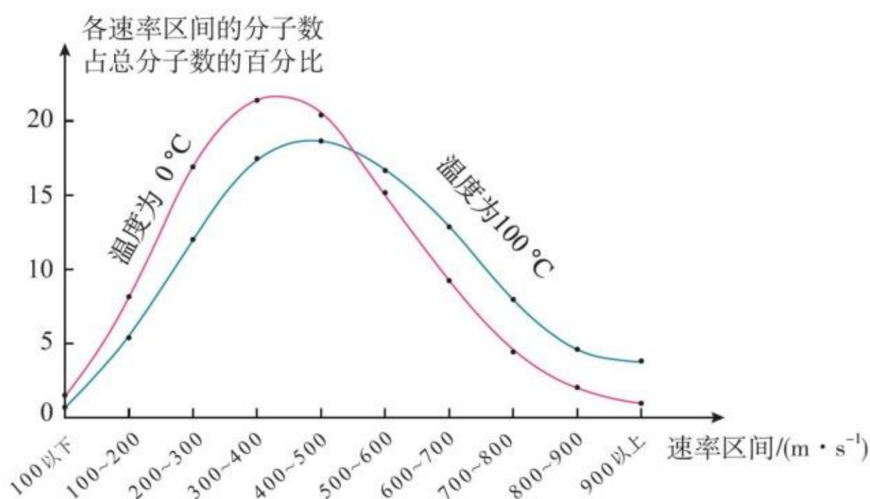
图1.3-2 氧气分子的速率分布情况
