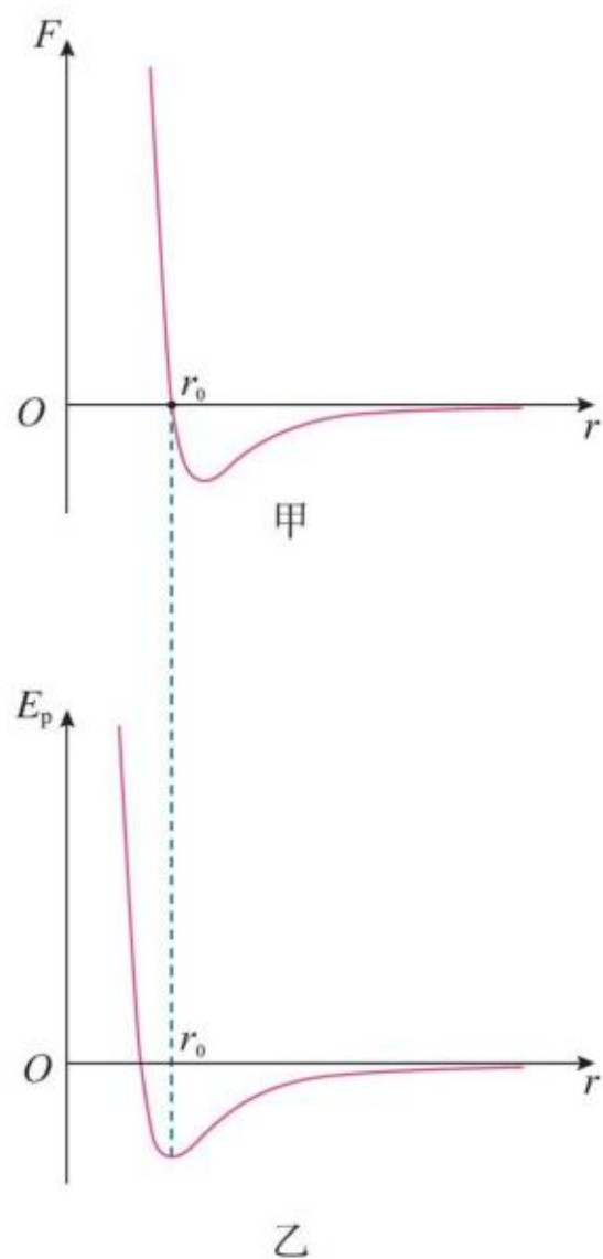
图1.4-2 分子间的作用力与分子势能
