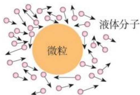
图 1.1-5 液体分子沿各方向对微粒的撞击
