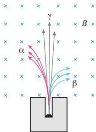
图 5.1-1 三种射线在磁场中的运动径迹不同
