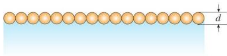
图1.2-1 水面上单分子油膜的示意图
