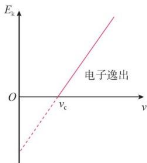
图4.2-4 光电效应的 E_k - \nu 图像
