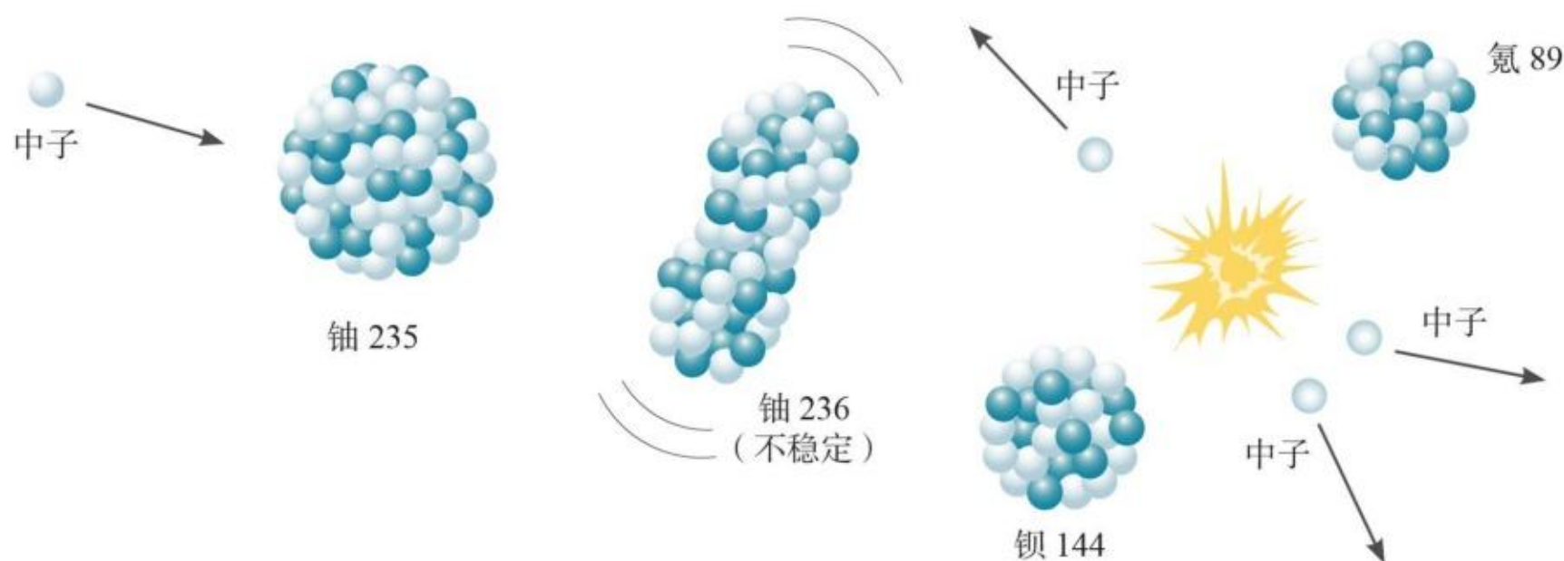
图 5.4-1 核裂变示意图
