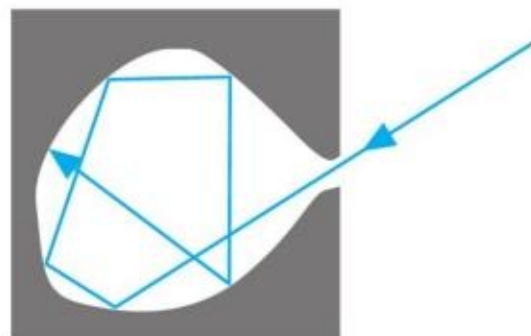
图4.1-1 带小孔的空腔
