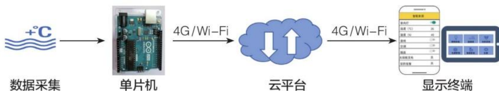
图4-8 数据采集系统示意图
