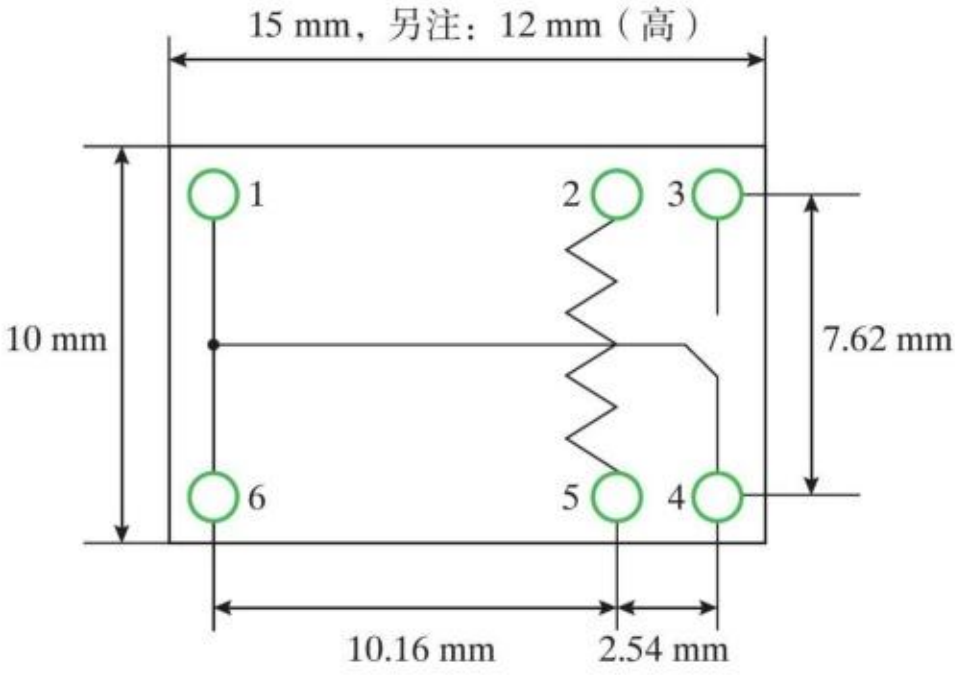
图3-3 继电器封装引脚（底视图）
