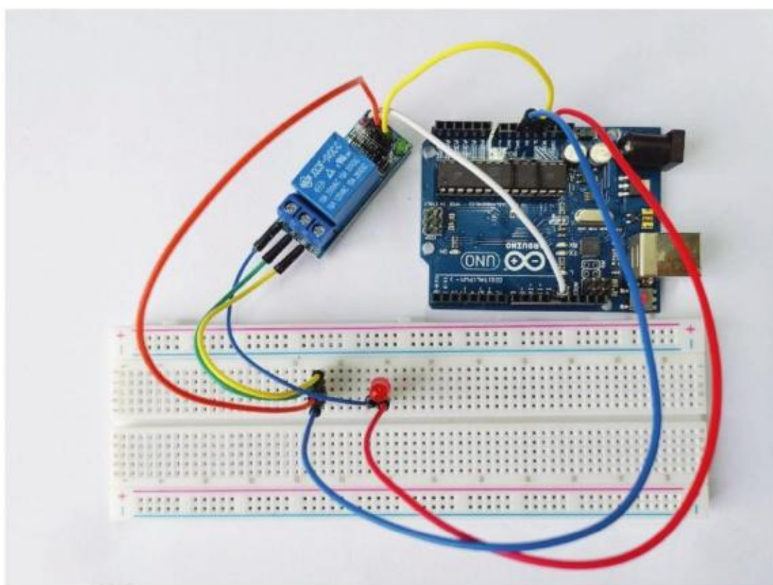
图 3-5 继电器控制 LED 灯连接图
