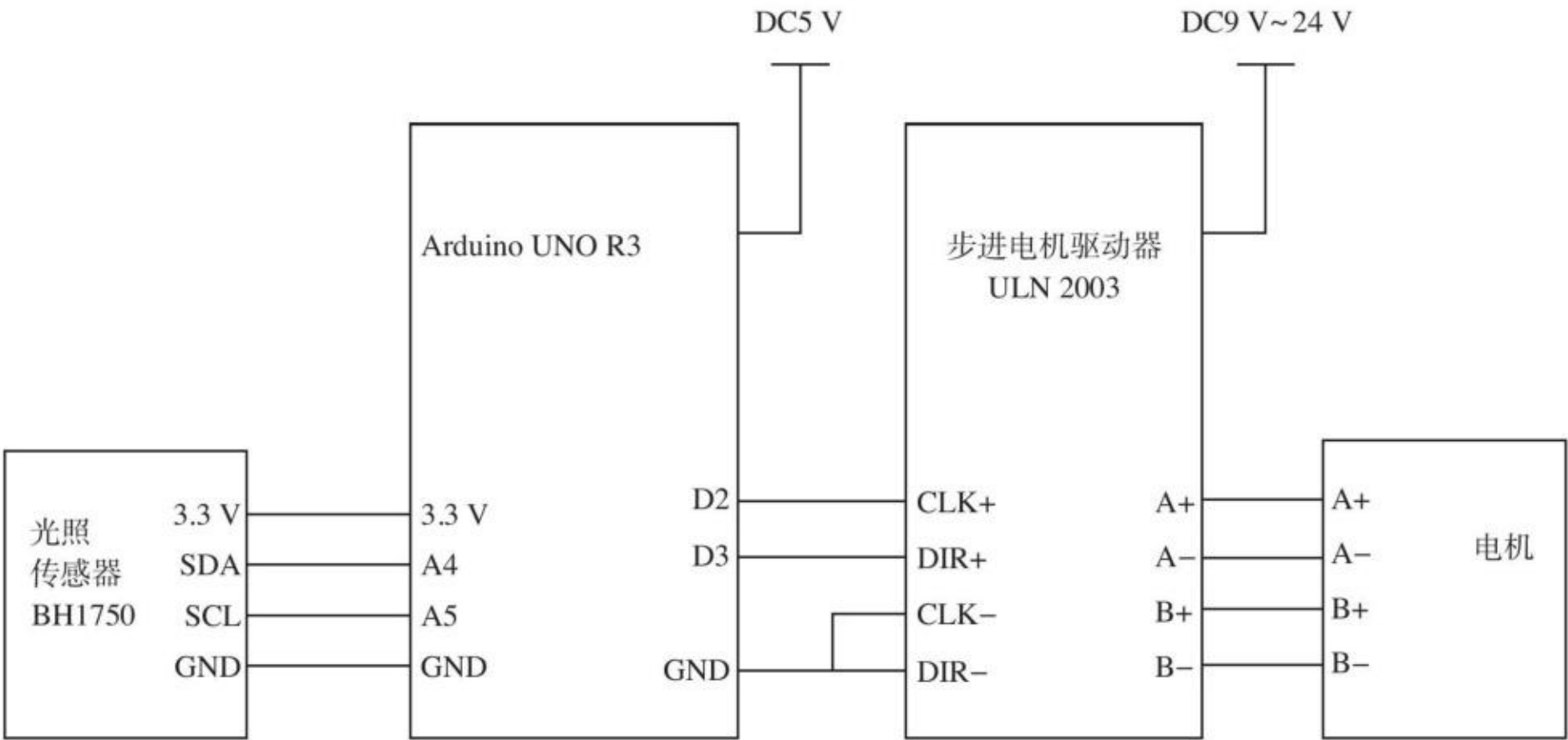
图3-34 闭环智能窗帘系统硬件连接图
