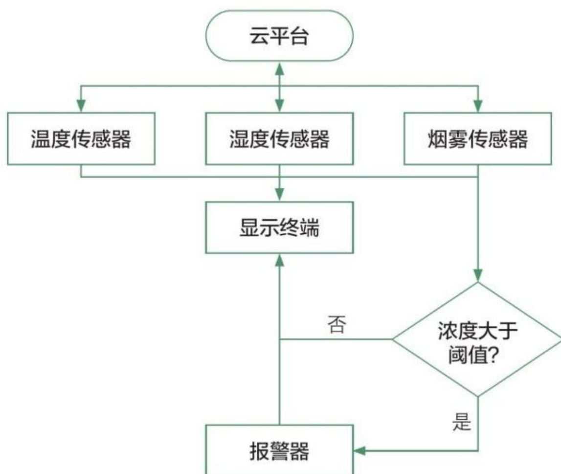
图4-9 数据采集系统设计流程图
