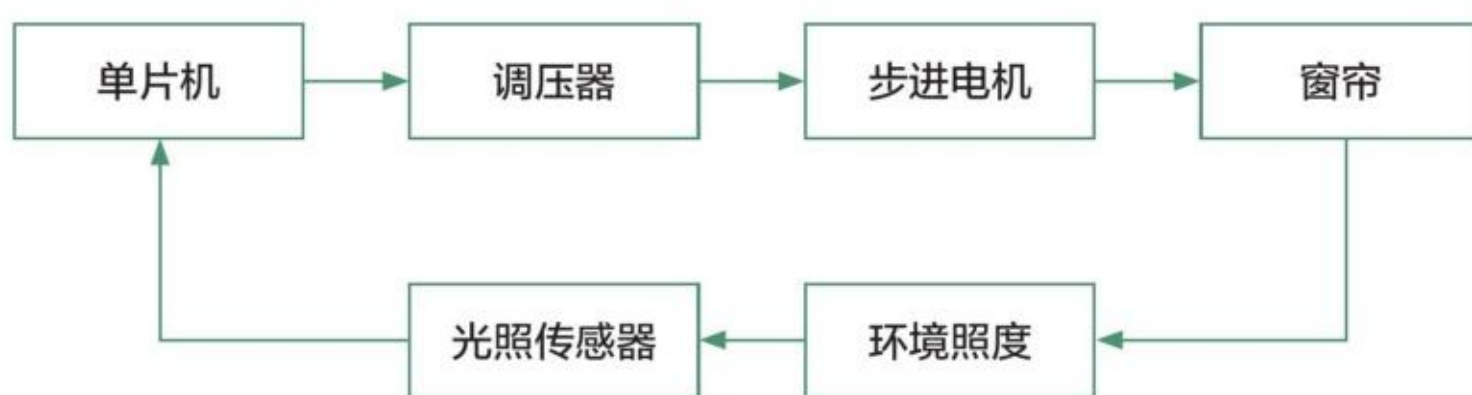
图 3-26 闭环控制的智能窗帘控制系统
