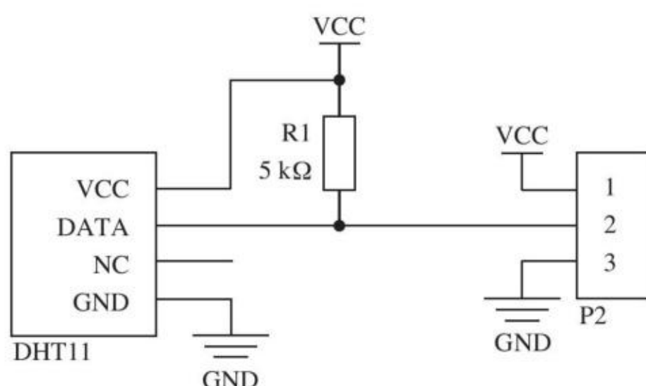
图3-15 DHT11电路连接图
