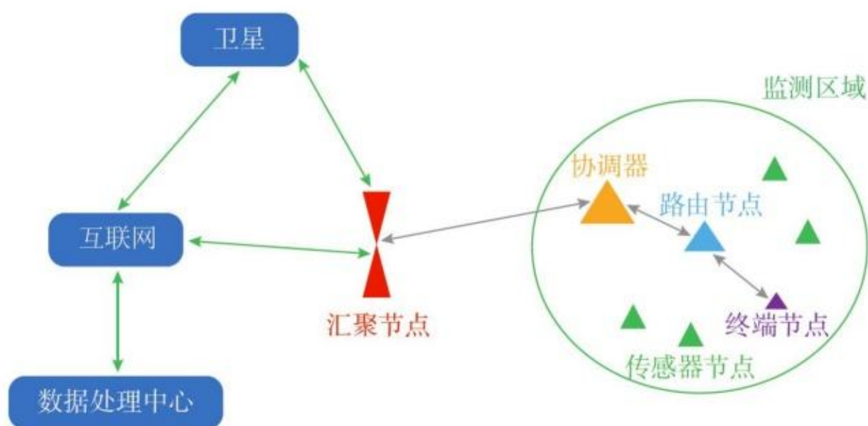
图2-4 无线传感网络系统结构
