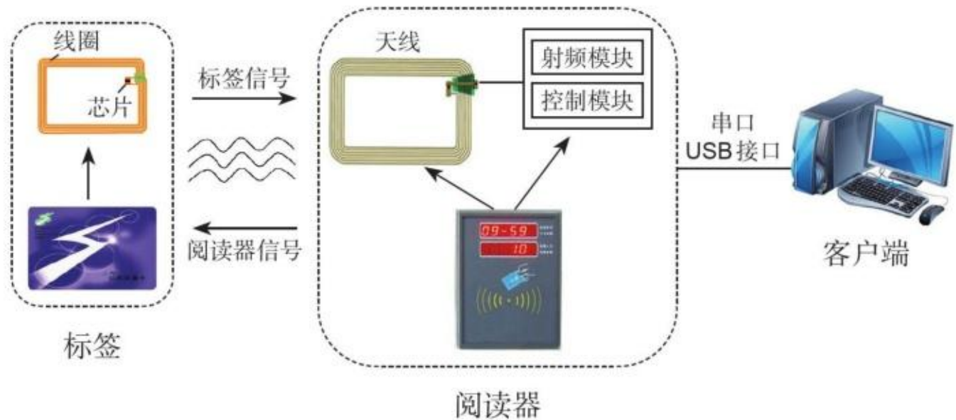
图2-9 射频识别工作原理示意图
