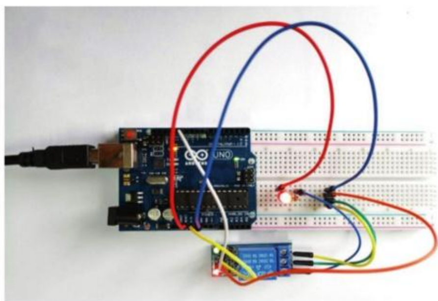
图 3-11 单片机发送高电平控制 LED 灯亮的实物图
