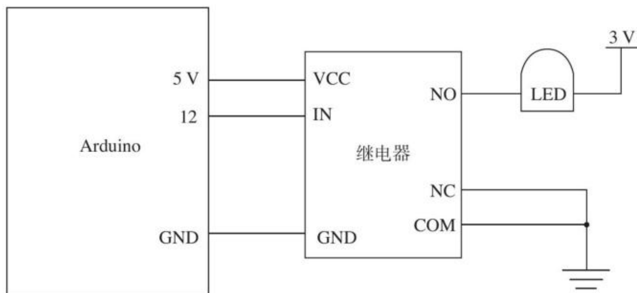
图3-4 继电器与单片机相连控制电路
