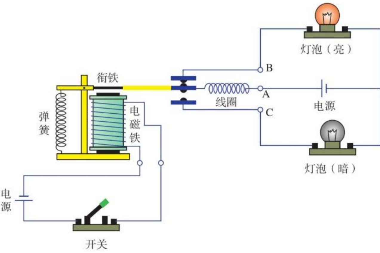
图3-1 继电器原理
