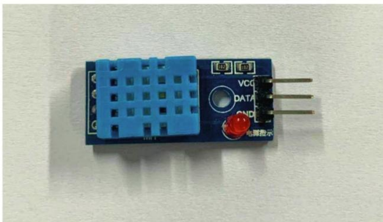
图3-14 DHT11实物
