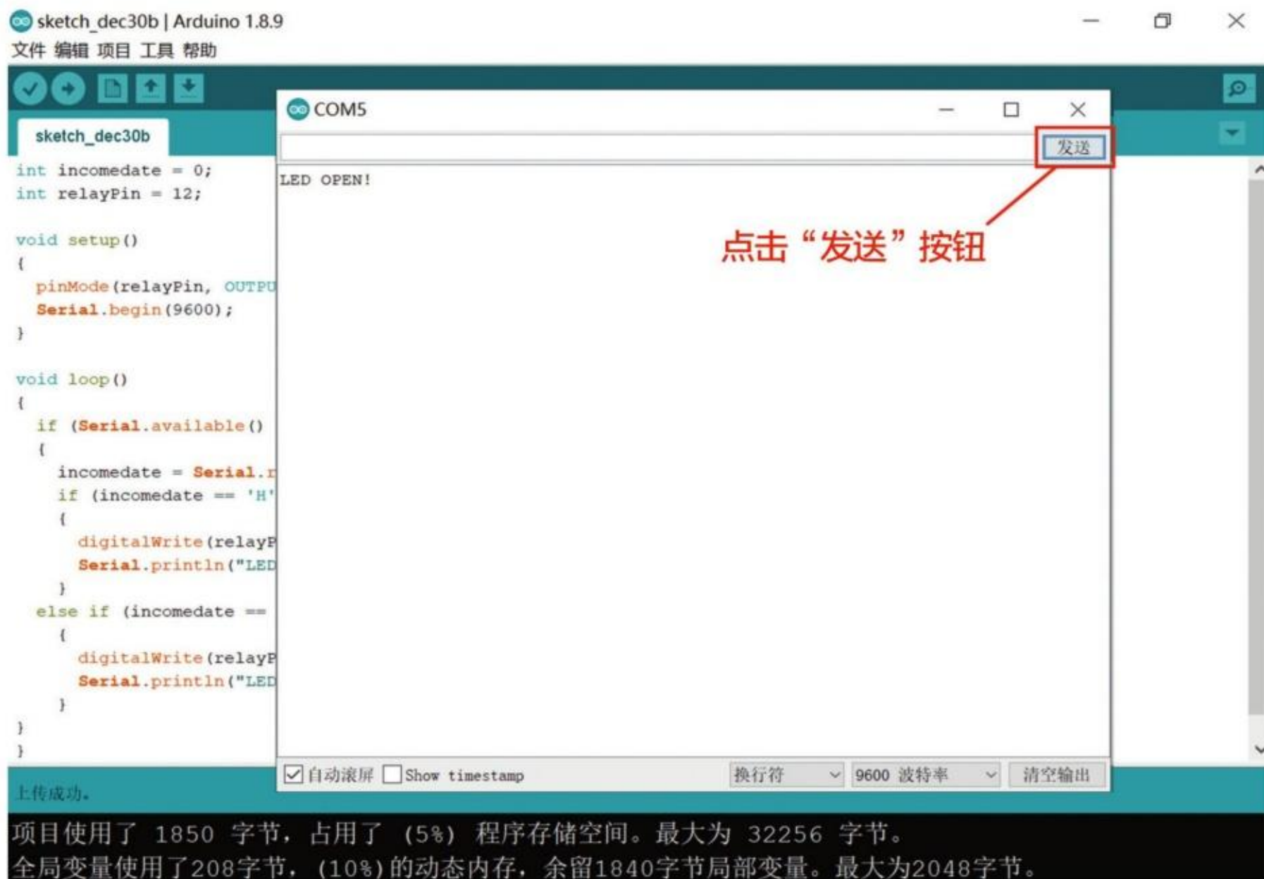
图3-10 实现LED灯控制的软件界面
