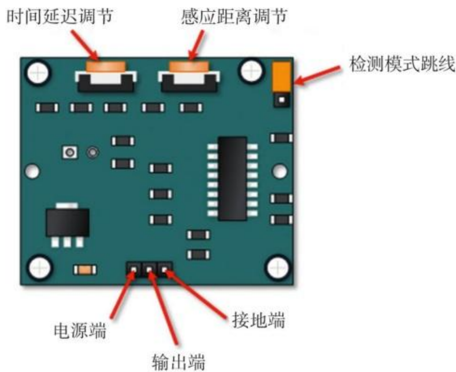
图3-21 HC-SR501模块的主要部分
