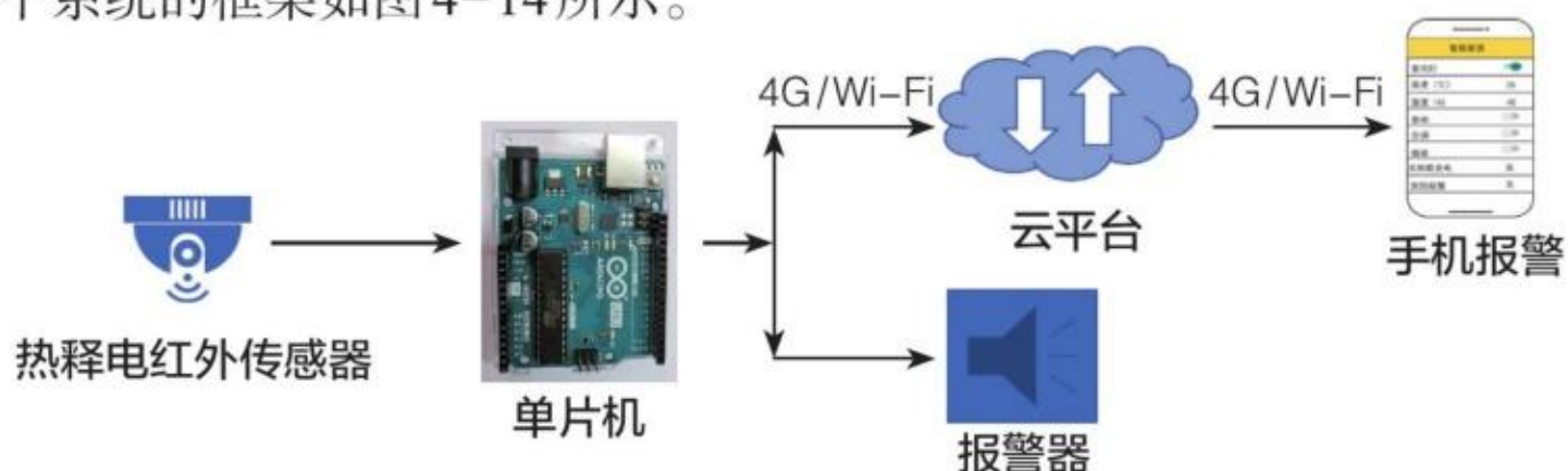
图4-14 智能安防系统框架
