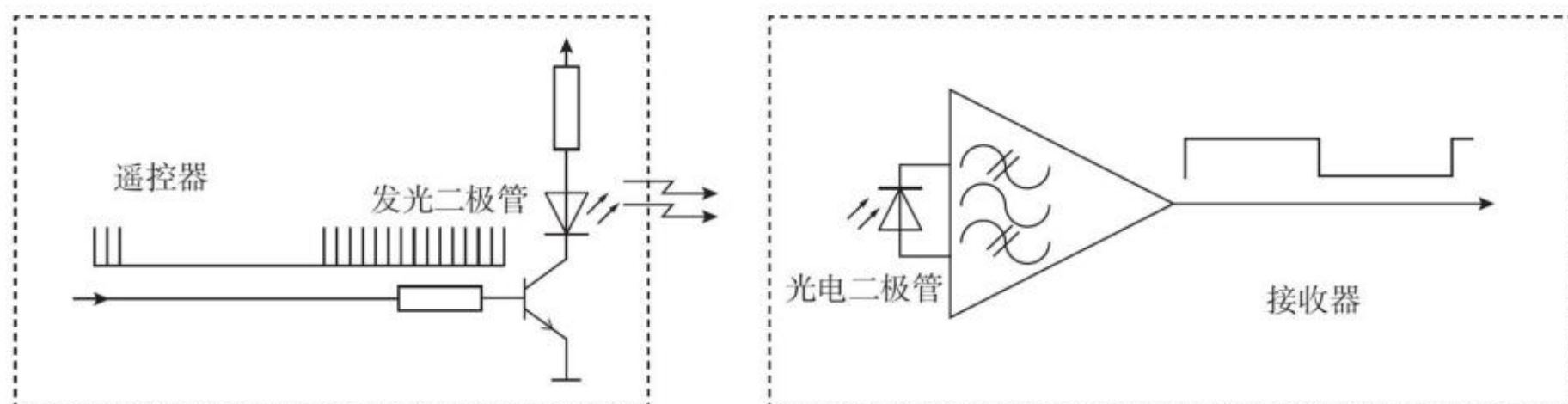
图2-8 红外遥控系统
