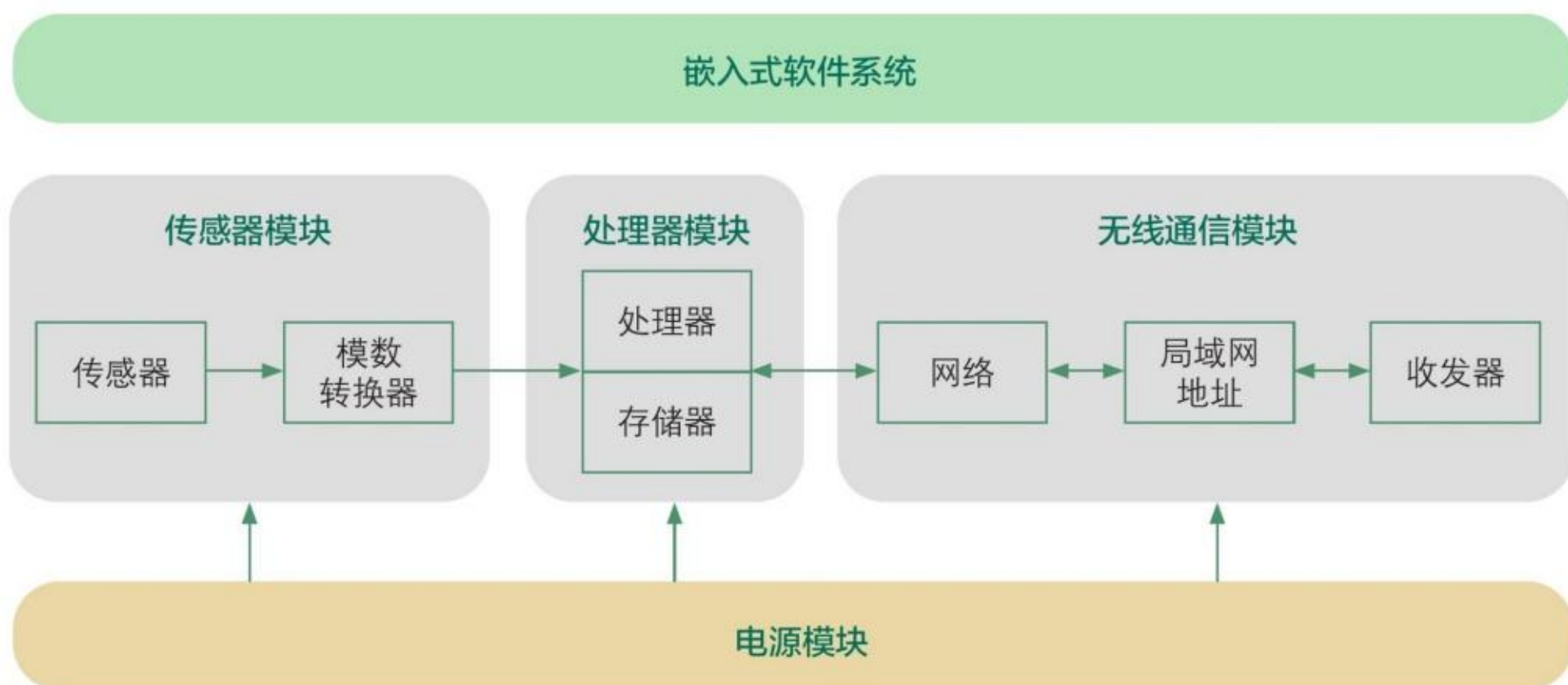
图2-3 无线传感网络节点的体系结构
