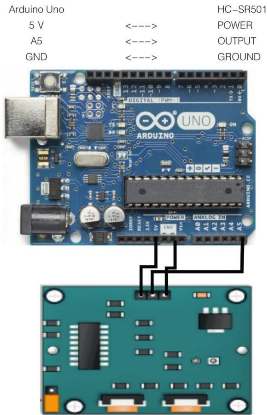
图3-22 系统接法
