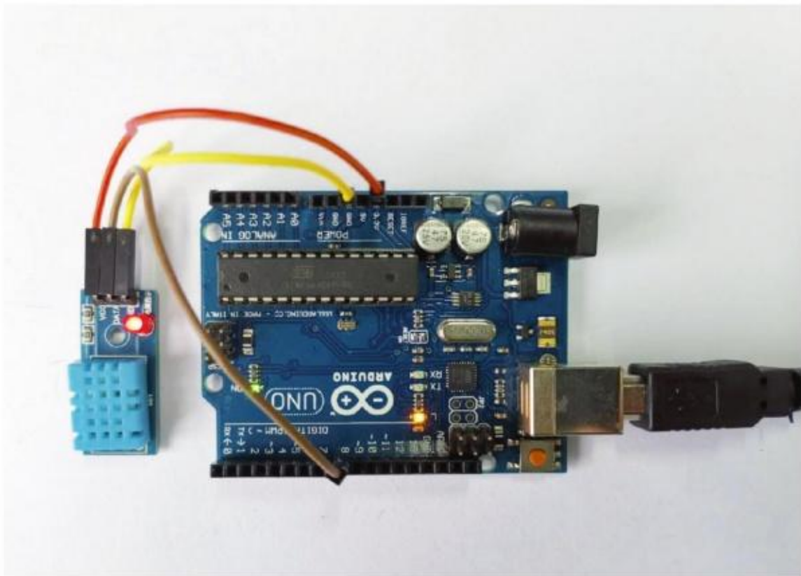
图3-16 数字温湿度计实物连接图
