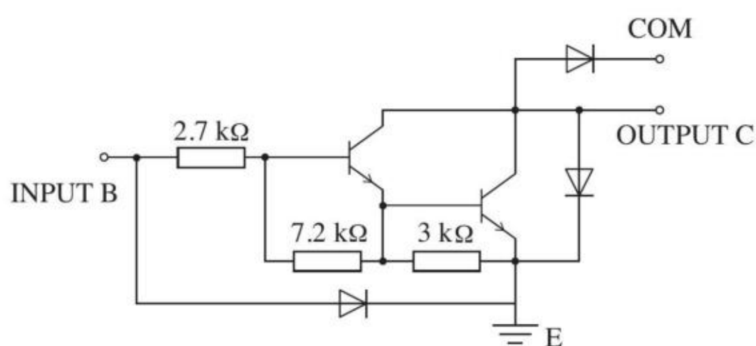
图 3-29 ULN2003 电路示意图
