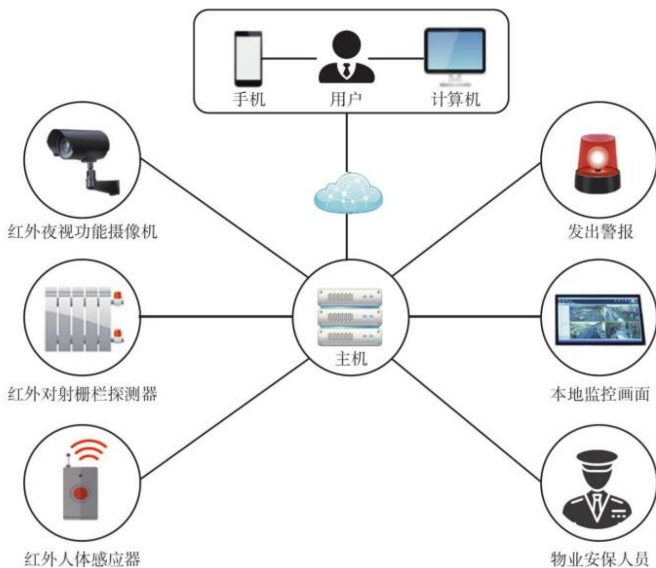
图 1-8 智能家居安防系统架构图
