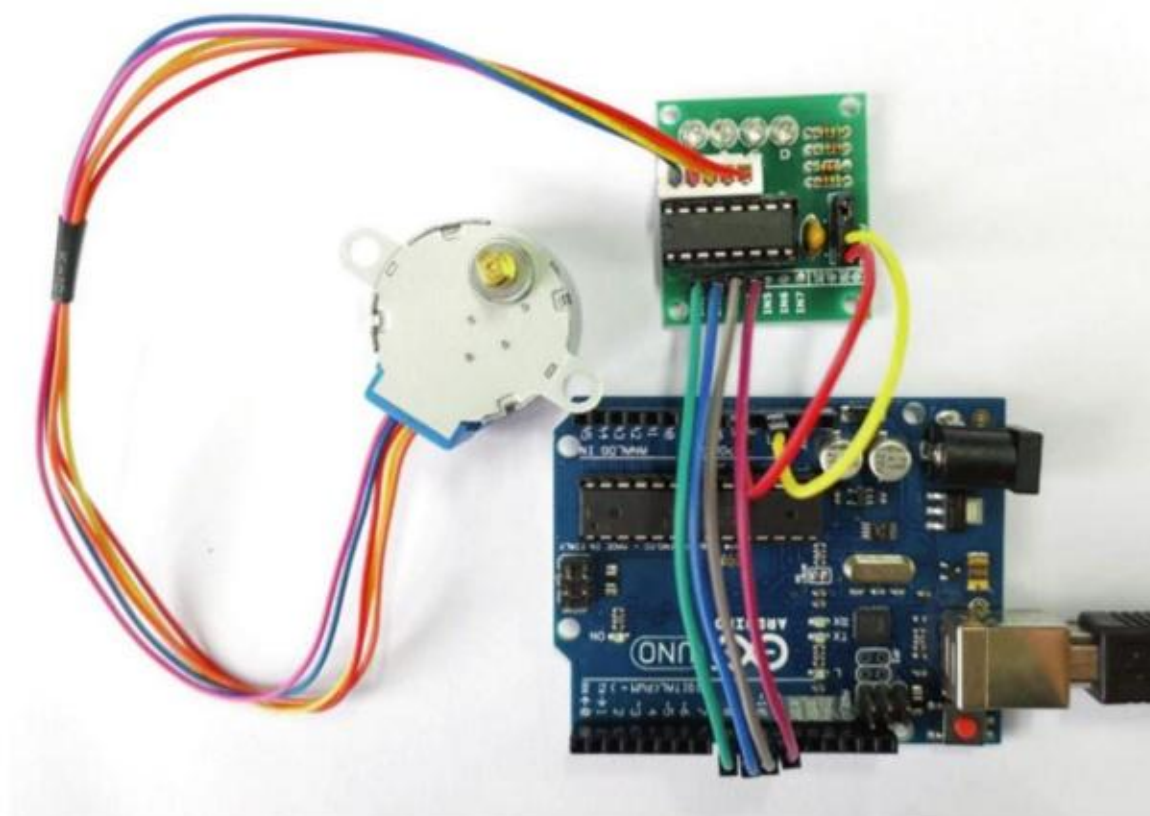
图3-31 系统控制连接实物
