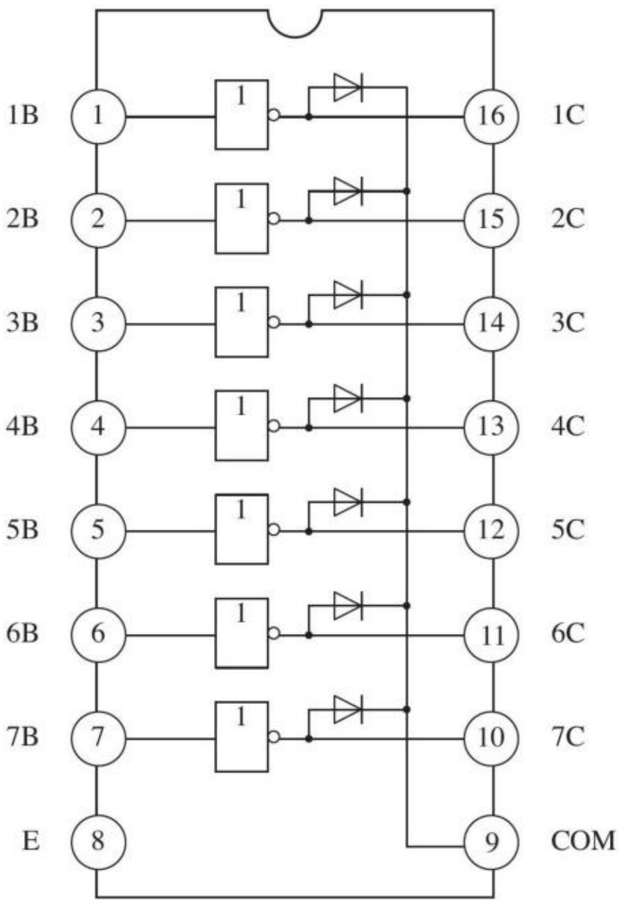
图3-28 ULN2003内部的逻辑框架图
