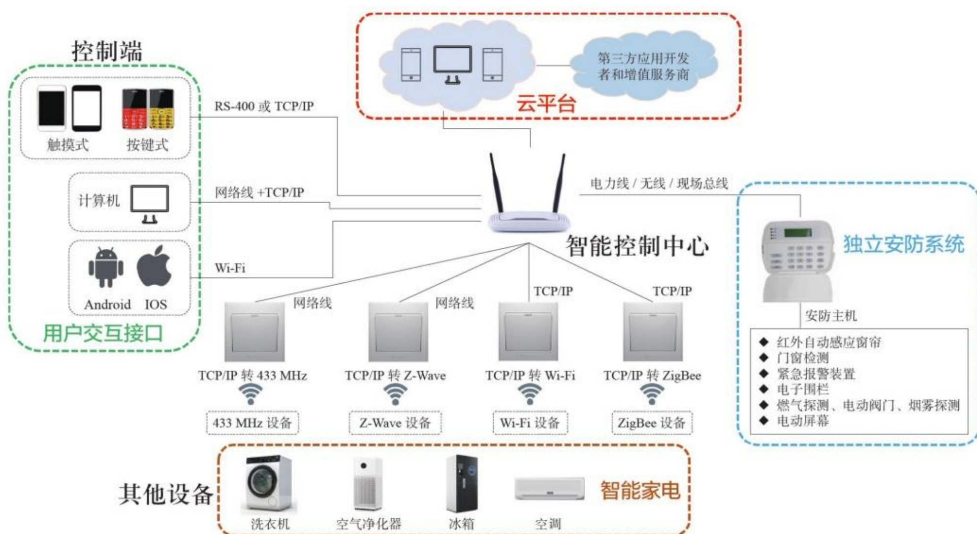
图1-2 智能家居的体系架构
