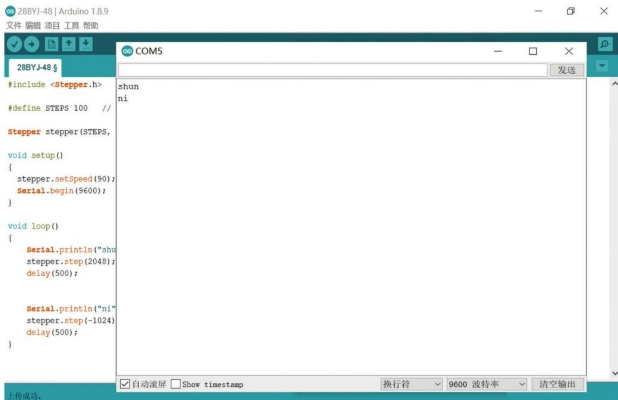
图3-32 电动窗帘实现的软件界面
