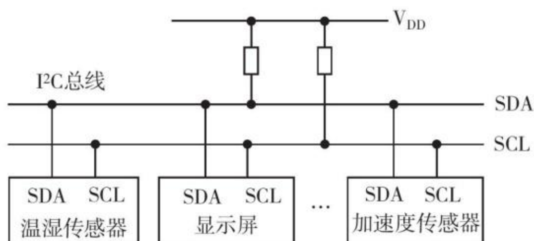
图2.3.5 I 2 C通信示意
