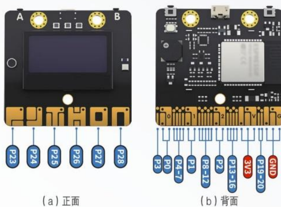
图 2.2.3 B 型板引脚分布图
