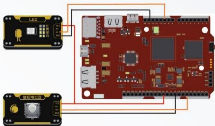
图1.3.5 可调亮度的台灯的接线图
