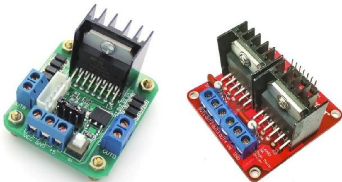
图2.3.10 L298电机驱动模块
