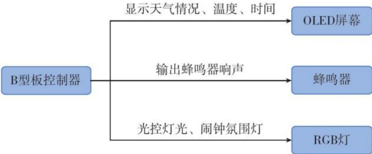
图4.1.9 互联网智能闹钟功能框图
