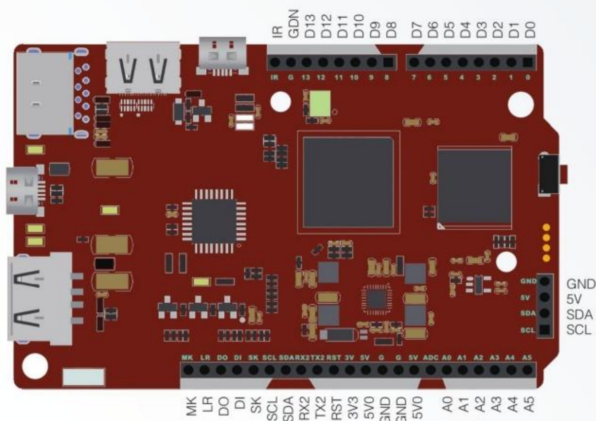
图 2.2.2 V 型板引脚分布图
