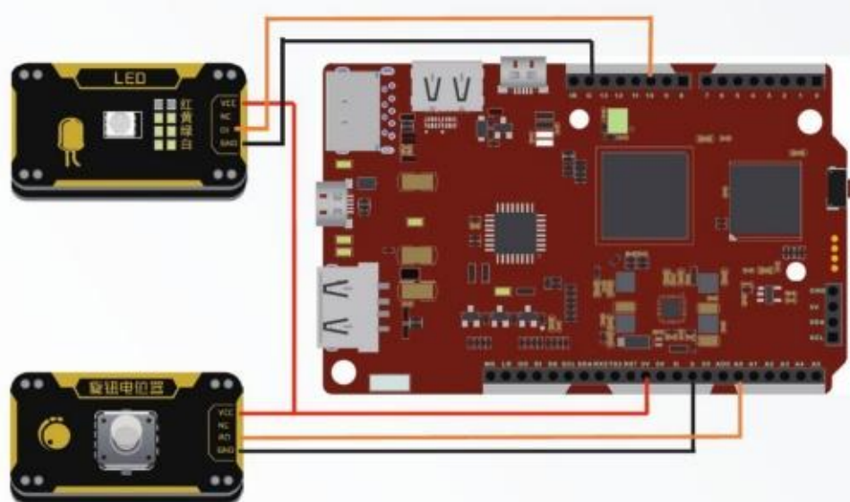
图 2.2.7 V 型板与 LED 和旋钮连接示意
