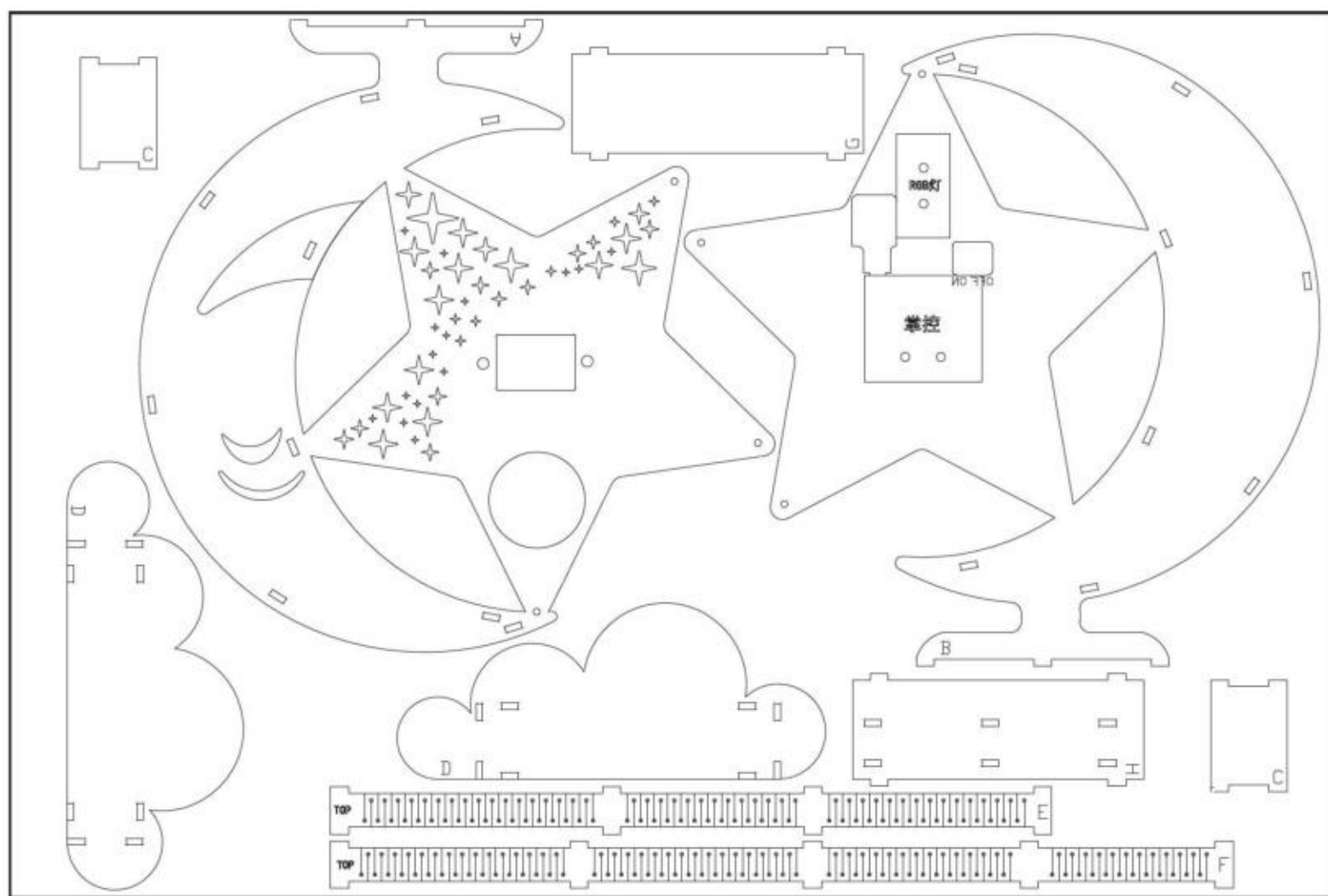
图4.1.3 “互联网智能闹钟”的外形图纸
