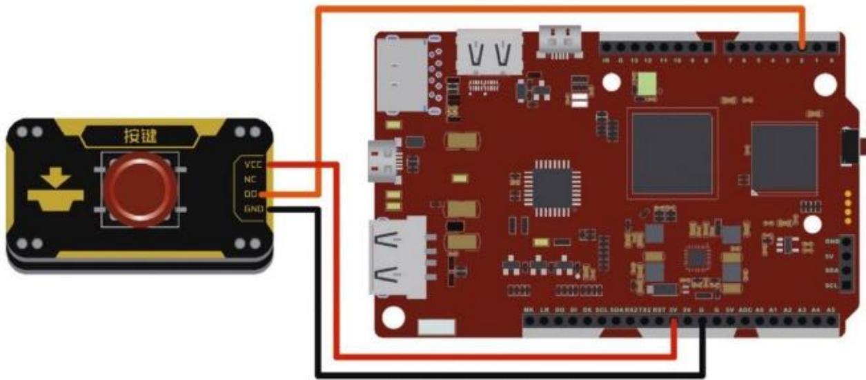
图 2.2.4 V 型板与按键的连接示意
