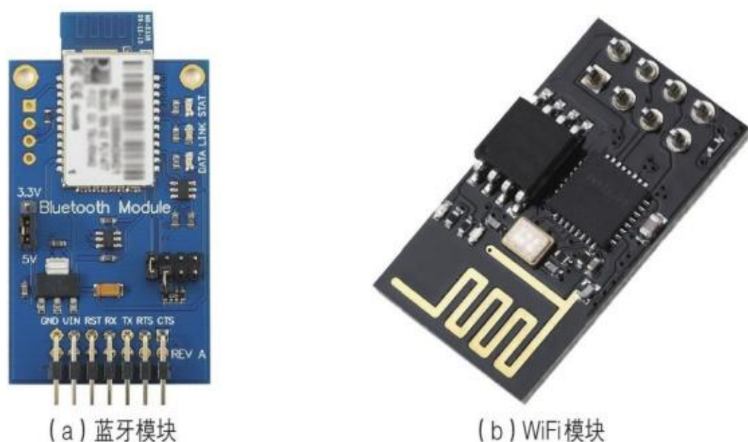
图2.3.2 无线串口通信硬件模块
