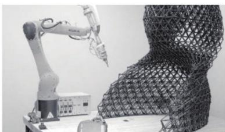
(b) 机械臂3D打印机
