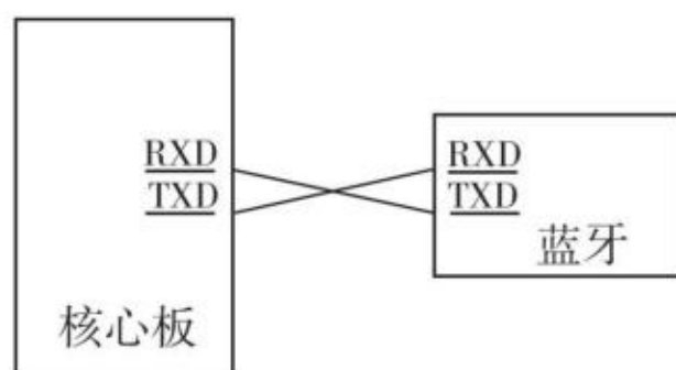
图2.3.4 核心板与蓝牙模块的连接示意
