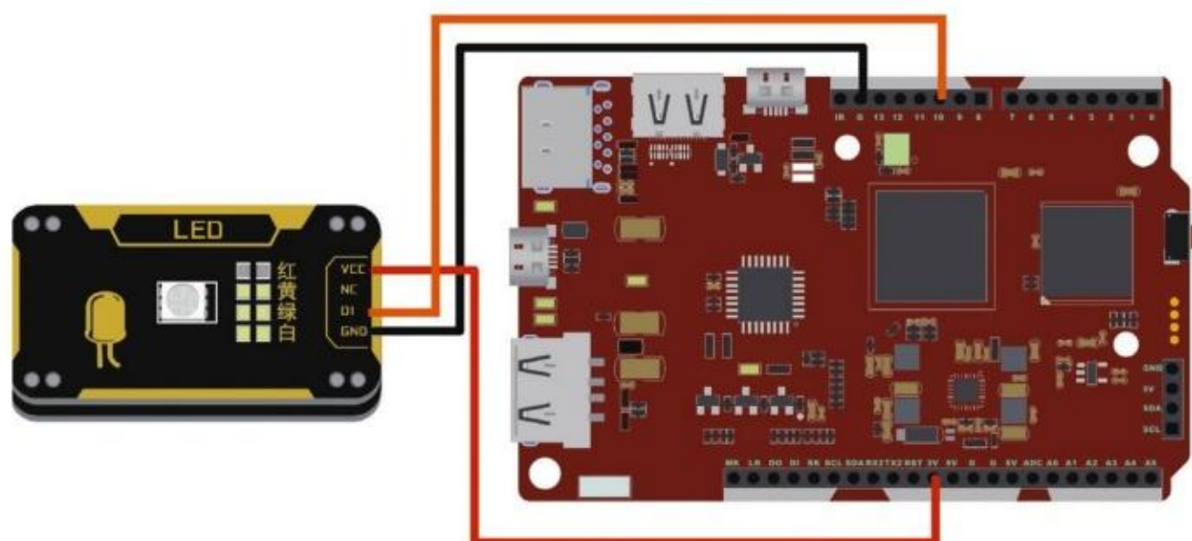
图2.2.6 V型板与LED连接示意
