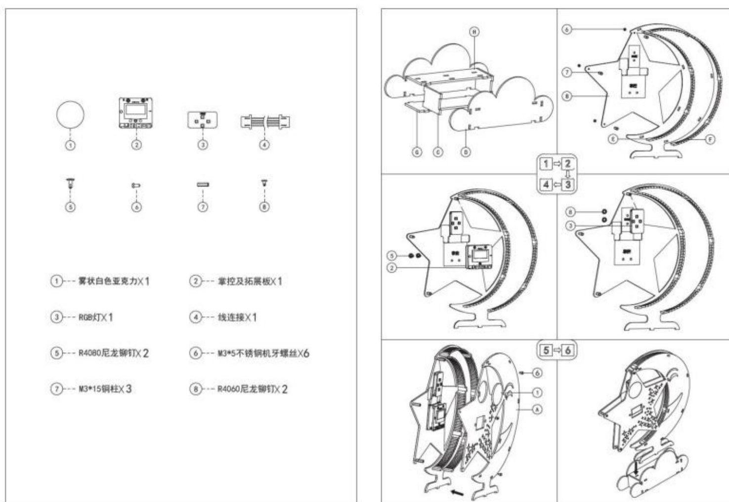
图4.1.5 “互联网智能闹钟”的装配图
