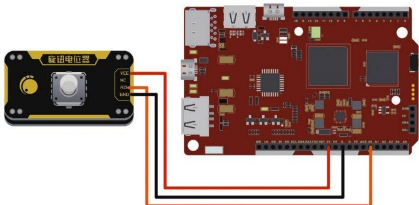
图2.2.5 V型板与旋钮连接示意
