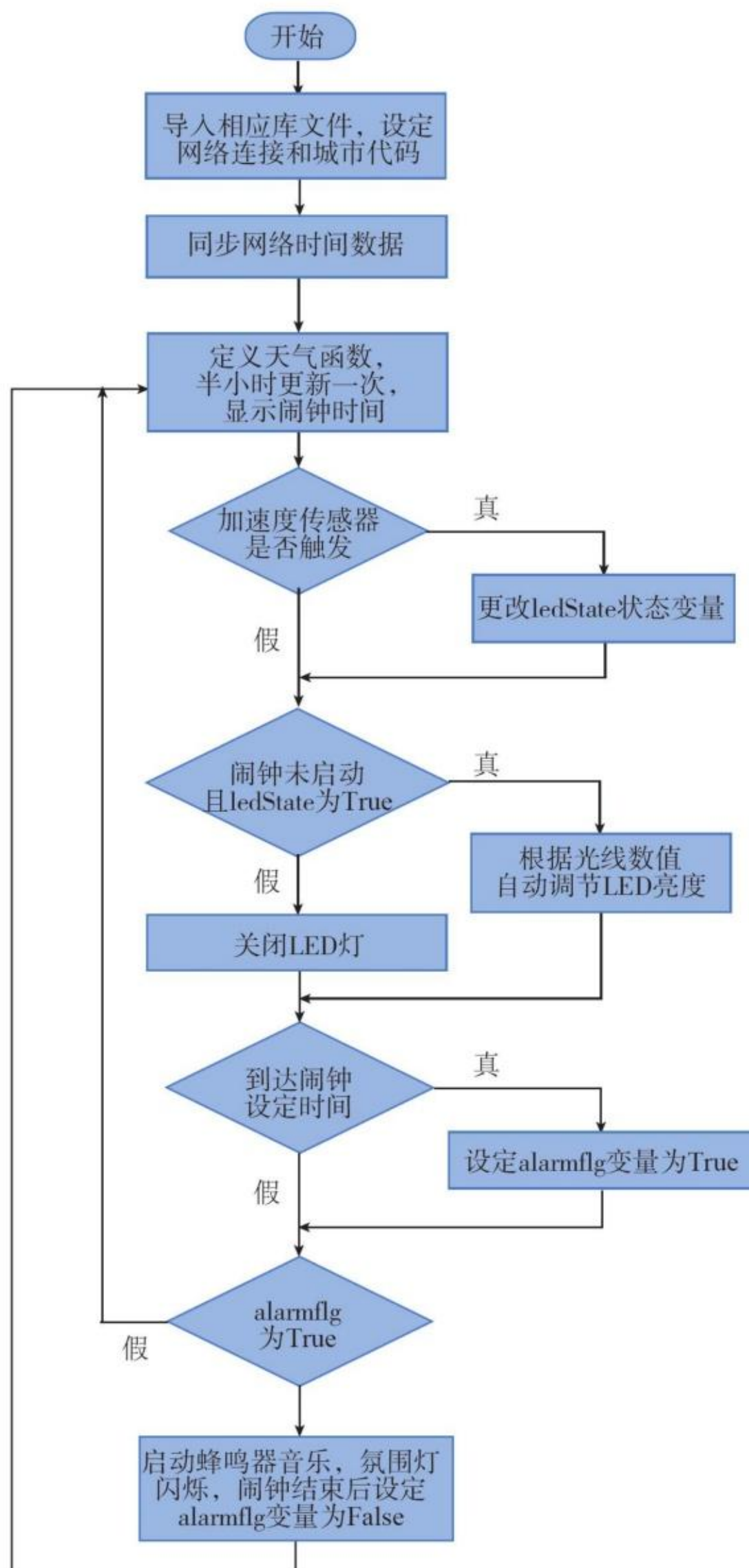
图4.1.11 “互联网智能闹钟”运算处理流程图
