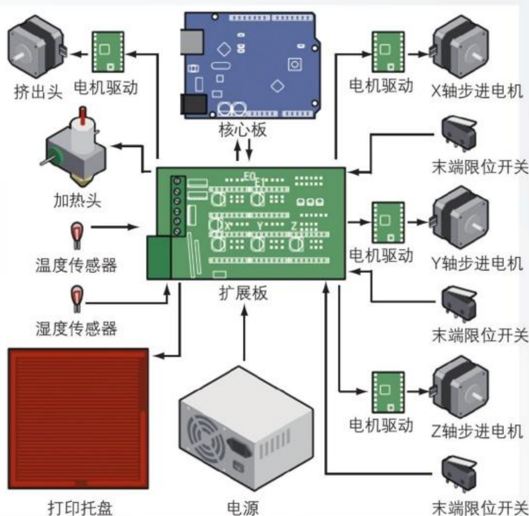
图2.4.4 3D打印机结构示意图
