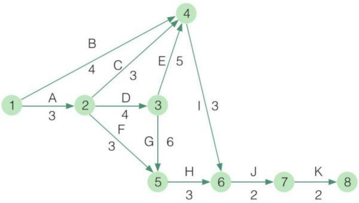
图4-7 热交换器原型测试的关键路径图
