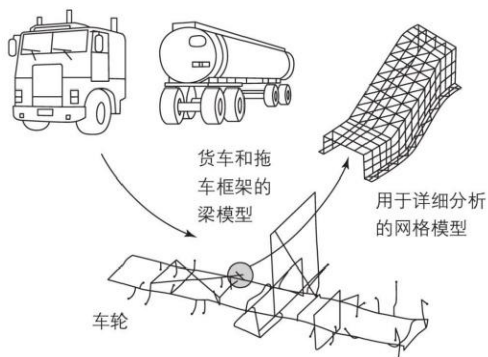
图3-2 有限元分析设计的实例
