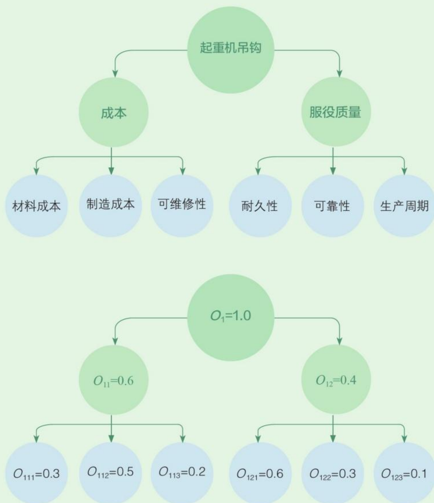
图4-4 起重机吊钩设计评价的层次目标树
