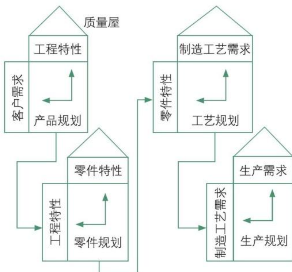
图2-7 完整的质量功能配置流程图
