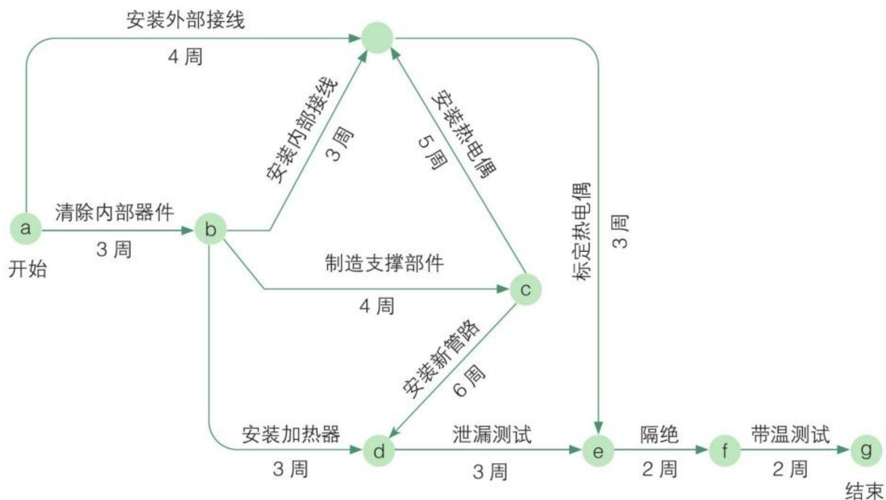
图4-6 热交换器原型安装并测试的网络逻辑图
