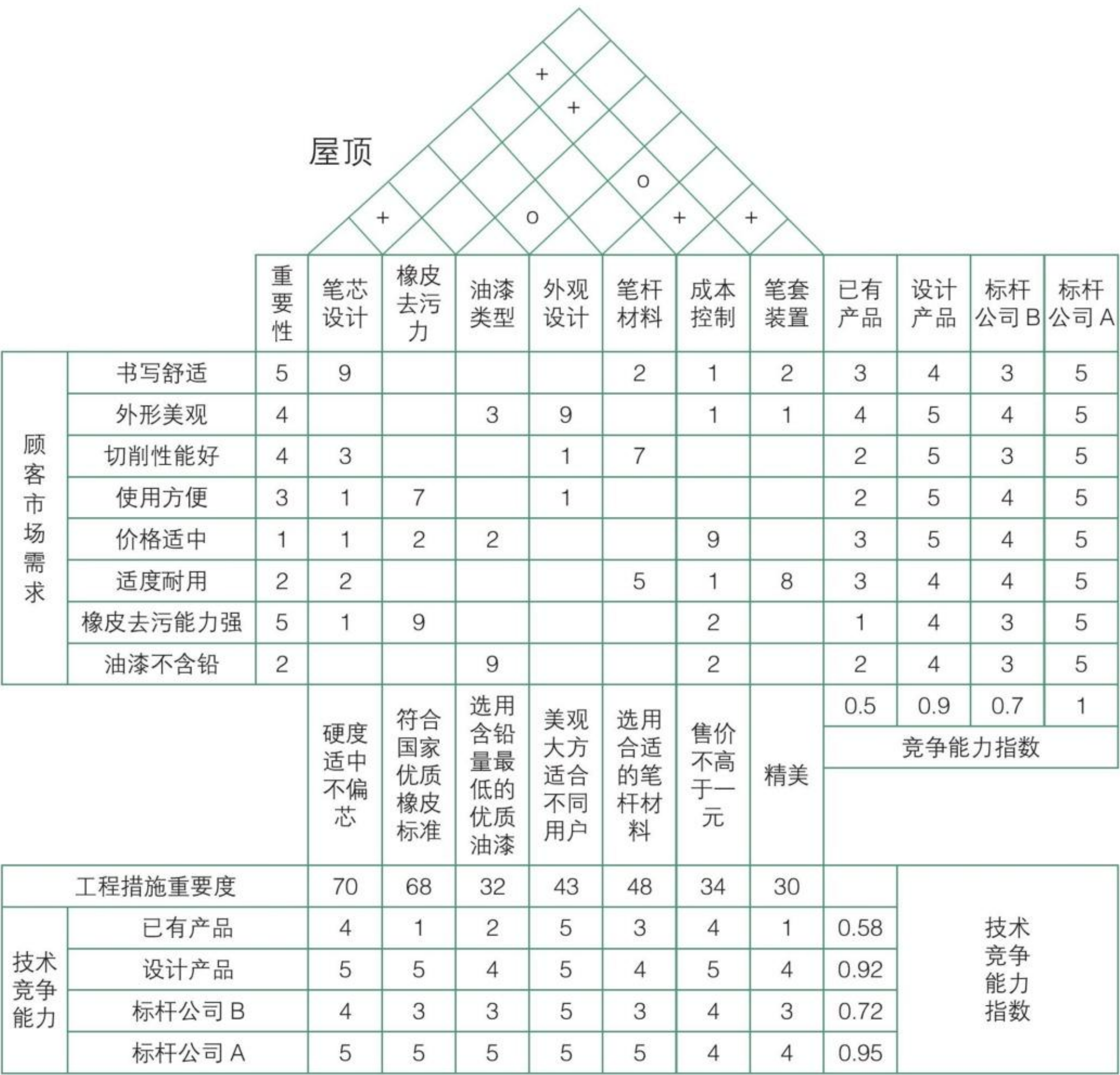
图2-9 铅笔再设计的质量功能配置
