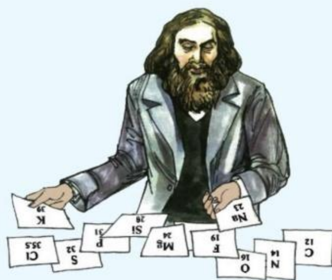
门捷列夫按原子量排列元素的顺序
