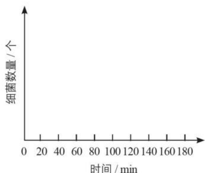
▲ 图 1-4 细菌种群的增长曲线
