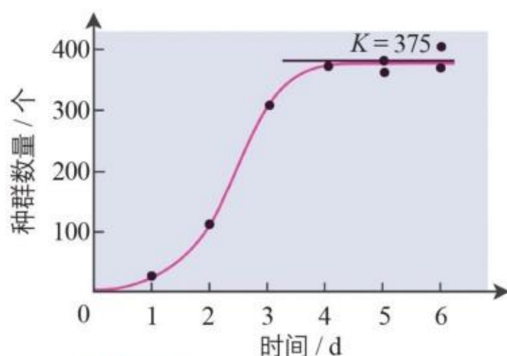
▲ 图 1-5 大草履虫种群的增长曲线
