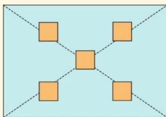
五点取样法
