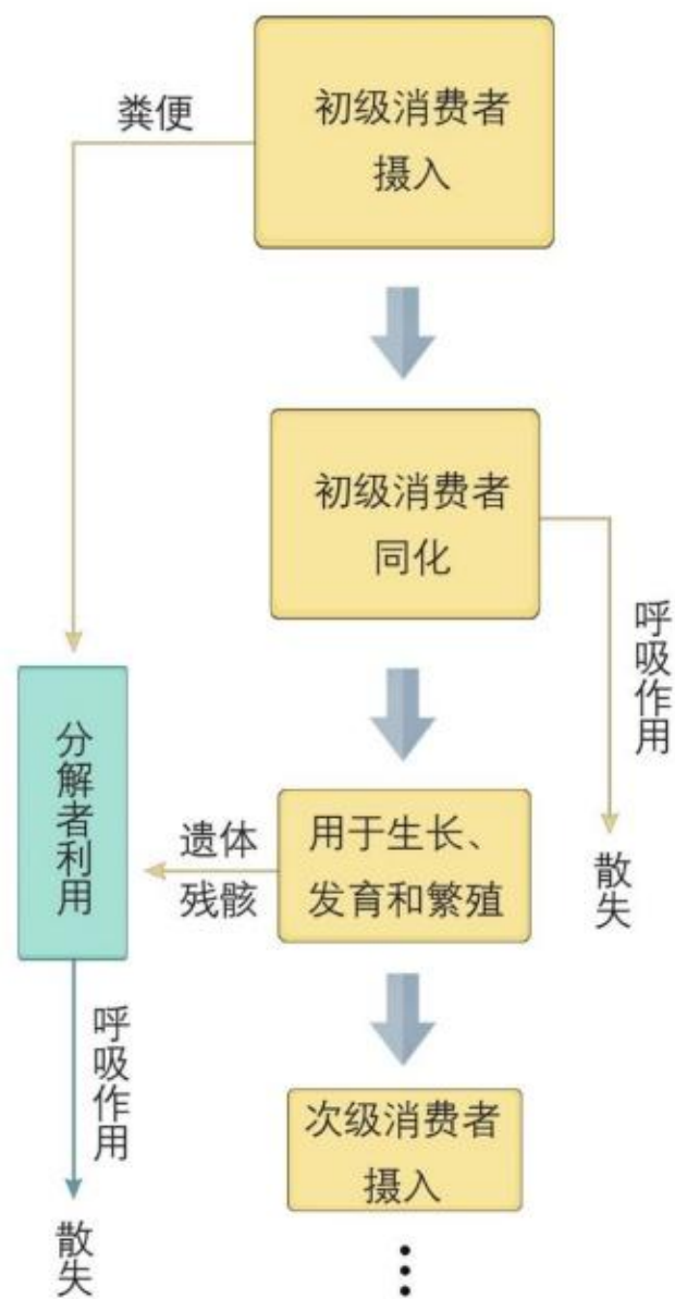
▲ 图 3-5 能量流经第二营养级的示意图
