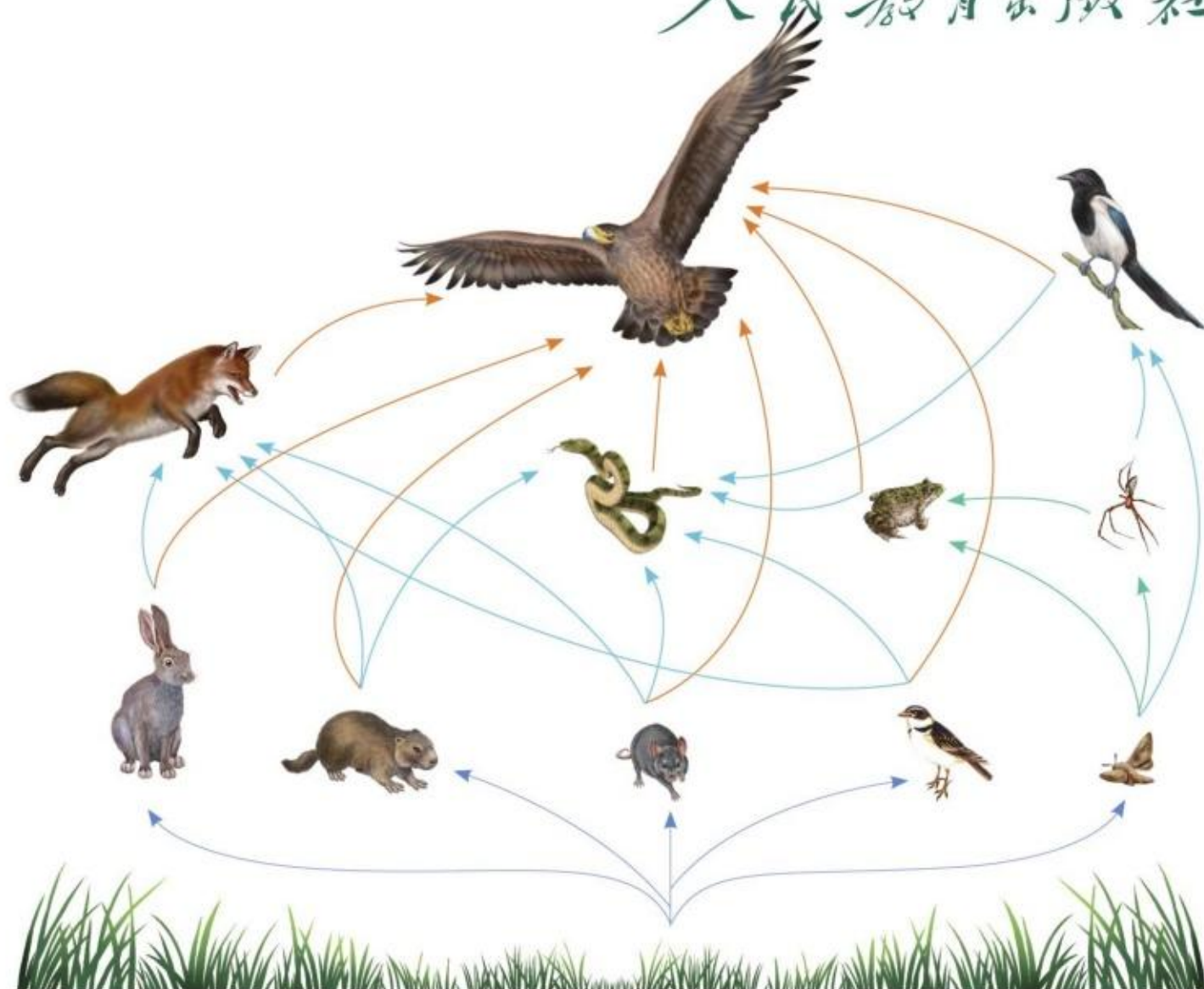
▲ 图 3-4 某陆地生态系统的食物网
