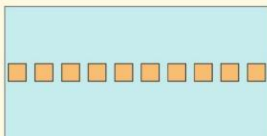
等距取样法
