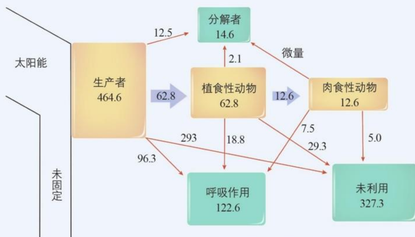
赛达伯格湖的能量流动图解
