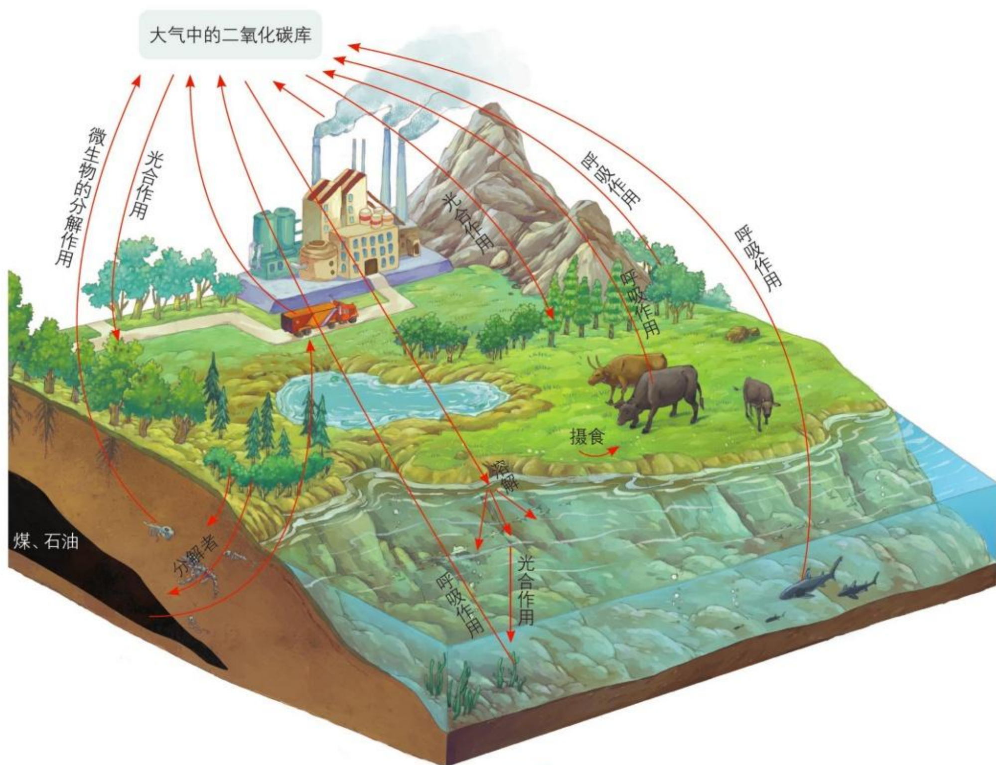
▲ 图 3-10 碳循环示意图
