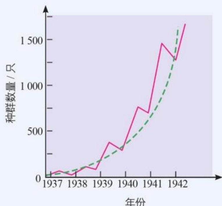
某岛屿环颈雉种群数量的增长曲线
