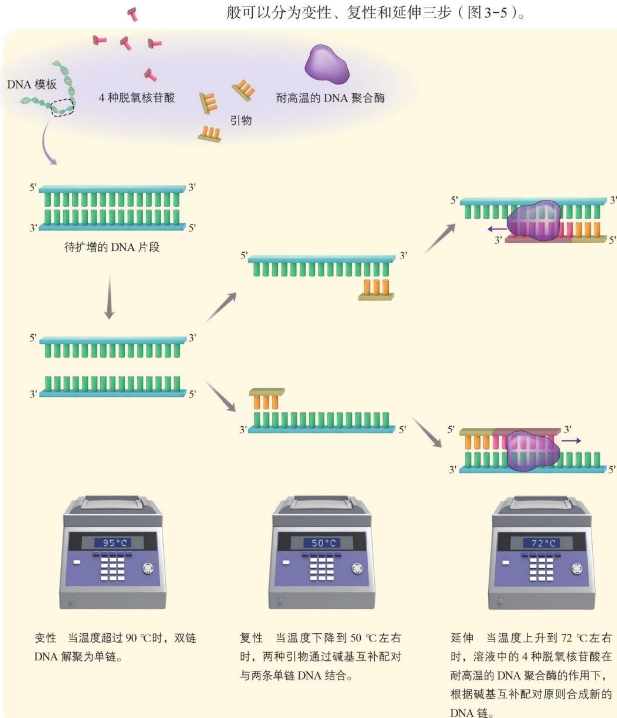
▲ 图3-5 PCR反应过程示意图
