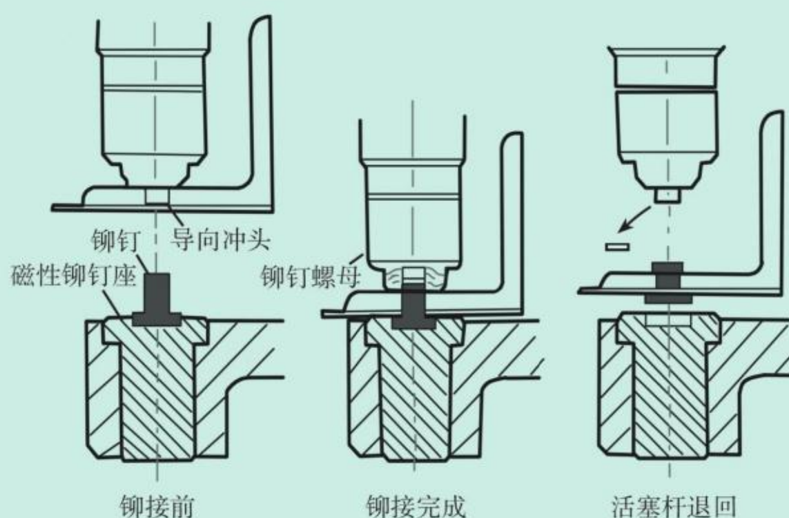
◇ 铆接步骤示意图
