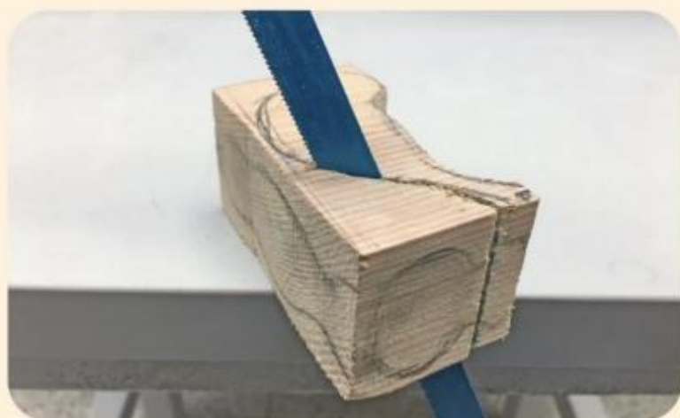
6. 沿着草图的轮廓线锯木块，但不锯透，以确保草图的完整性。
