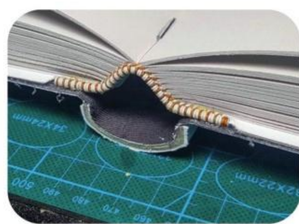
◇ 堵头布和封套结构
