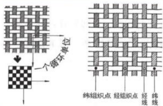
◇ 织物循环单位 ◇ 经纬线组织
