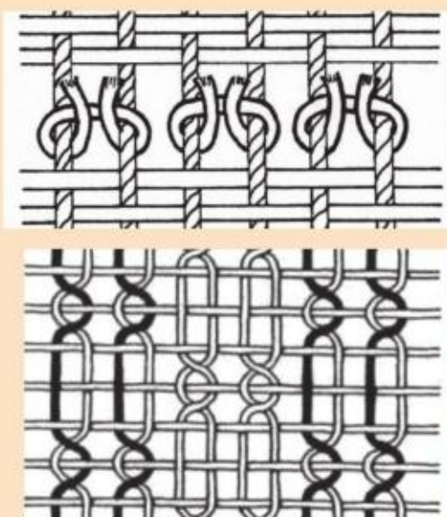
◇ 各种纱罗组织结构
