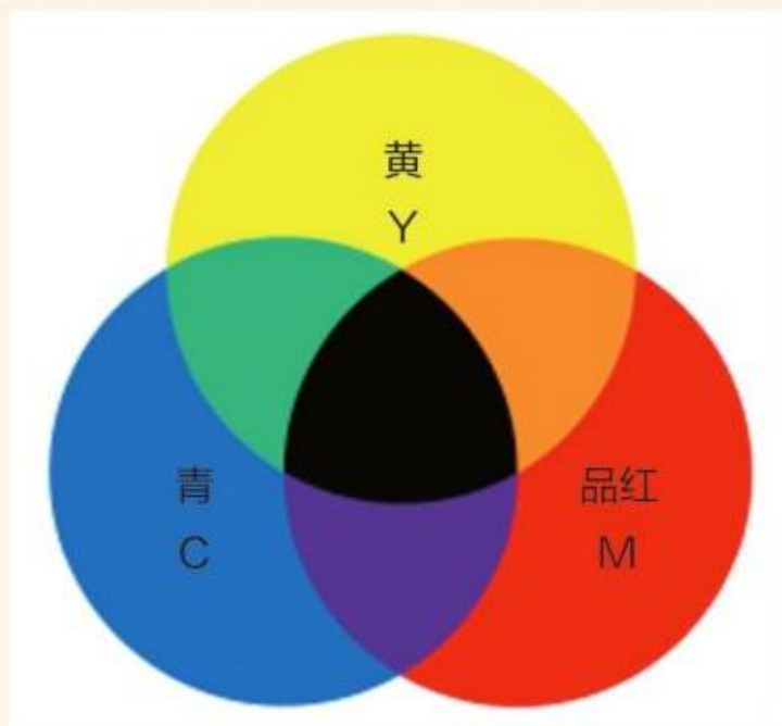
CMY 色彩减法
