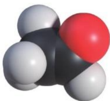
图3-15 乙醛的分子结构模型
