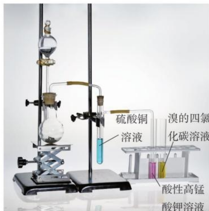
图2-6 乙炔的实验室制取及性质检验
