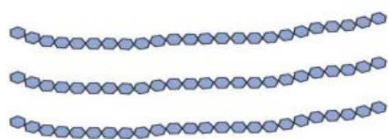
图4-4 纤维素的结构示意图（其中每个小的六边形代表一个葡萄糖的环状结构单元）
