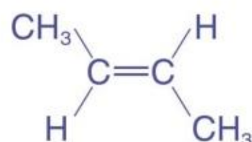
反-2-丁烯
