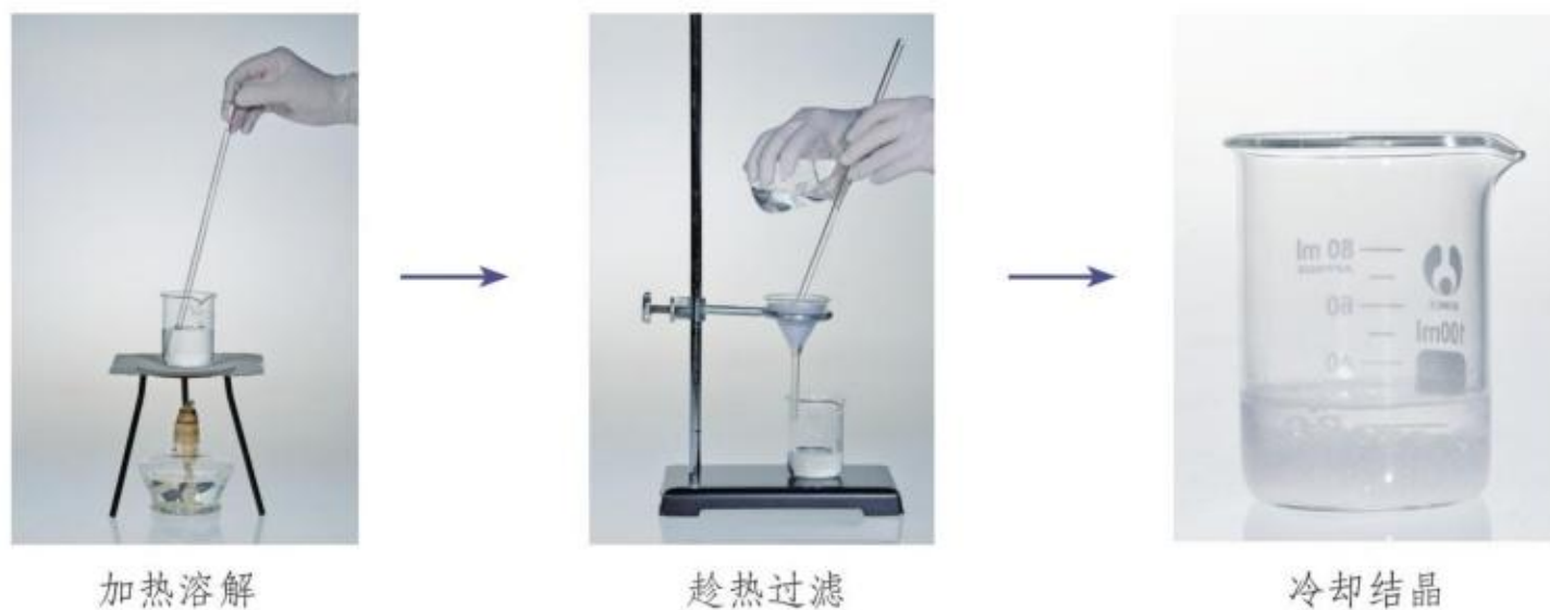
图1-9 重结晶法提纯苯甲酸
