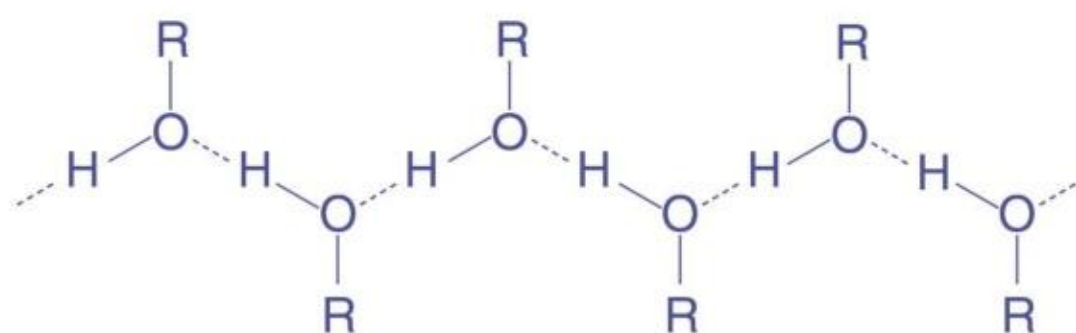
图3-6 醇分子间形成氢键
