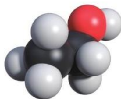
图3-7 乙醇的分子结构模型
