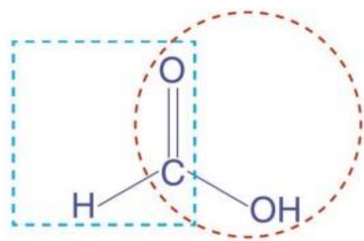
图3-20 甲酸分子的结构
