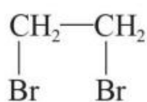
1,2-二溴乙烷
