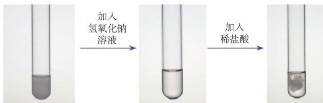
图3-12 苯酚的酸性
