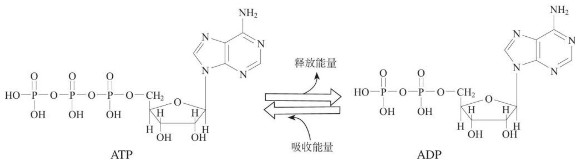
图4-16 生物体内的ATP-ADP循环示意图
