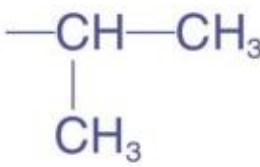
异丙基
