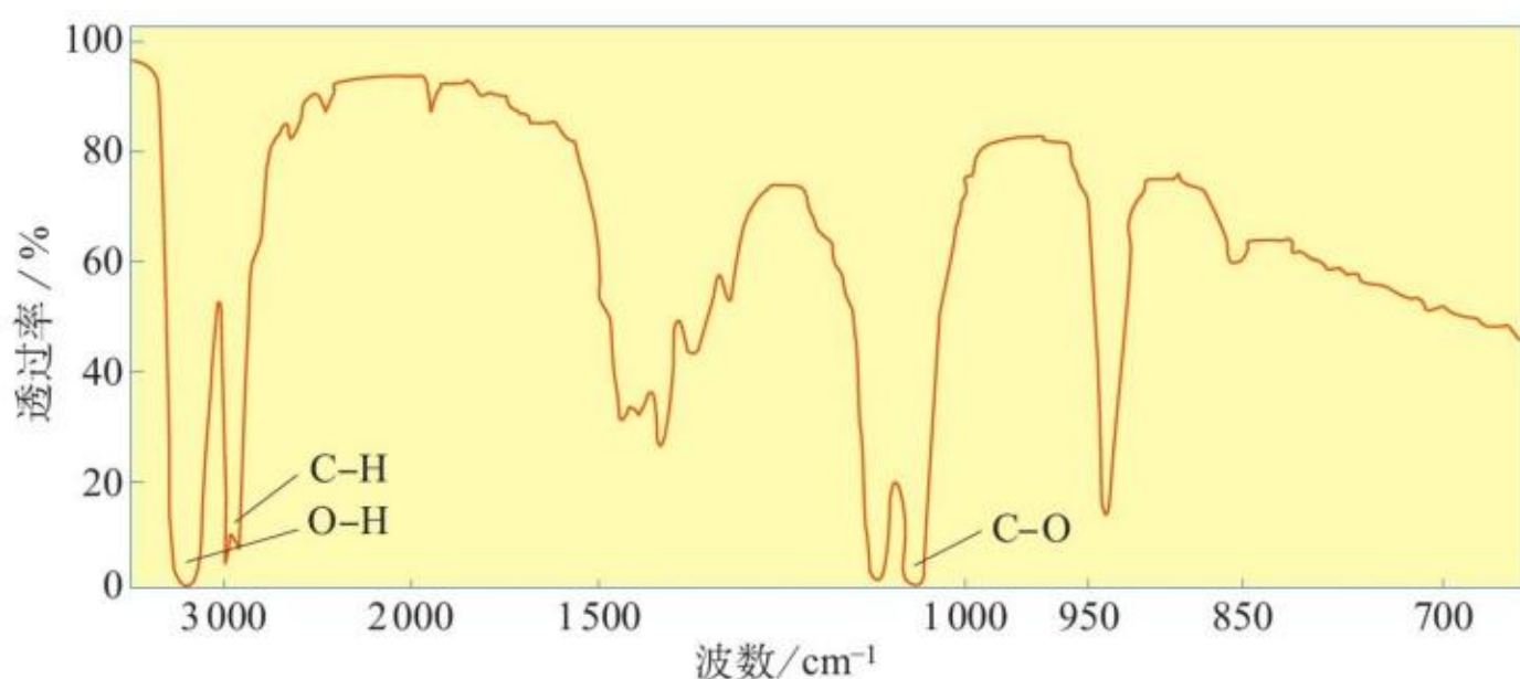
图 1-16 未知物 A 的红外光谱
