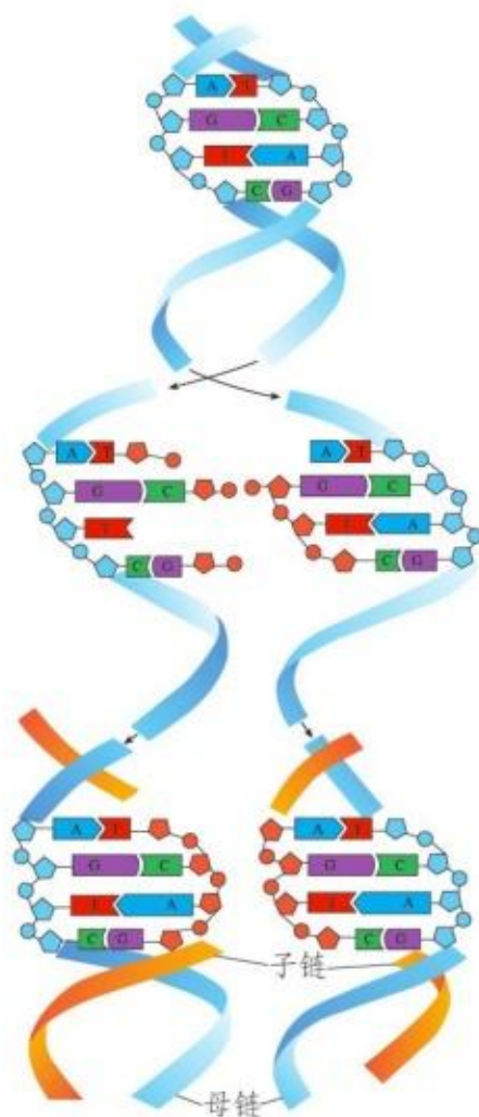
图4-20 DNA分子复制示意图
