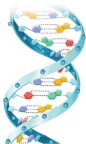
图4-17 脱氧核糖核酸(DNA)的结构示意图
