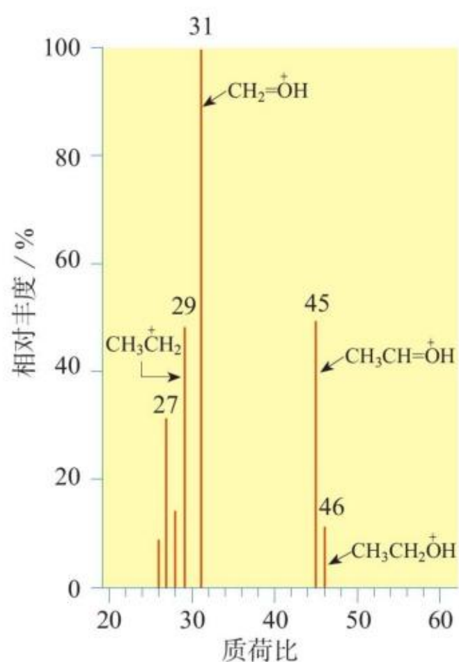
图 1-15 未知物 A 的质谱
