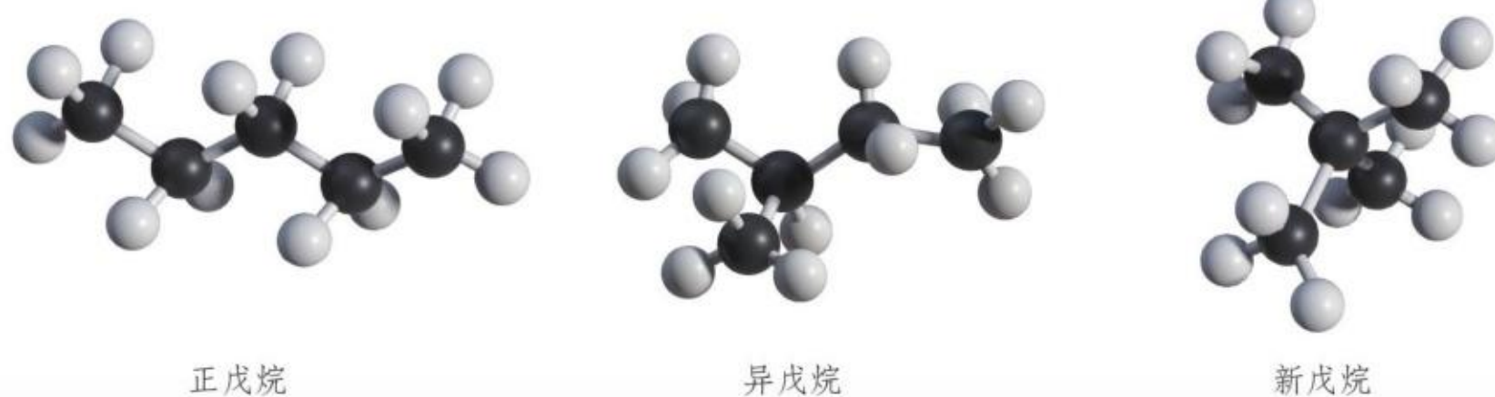
图 1-3 三种戊烷的分子结构模型
