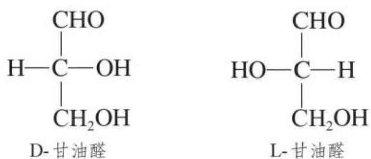
图4-1 甘油醛的对映异构
