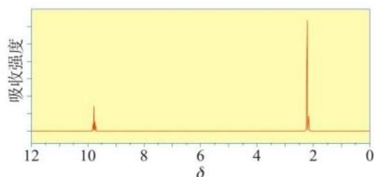
图3-16 乙醛的核磁共振氢谱
