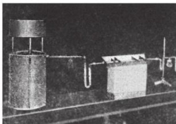
图 1-12 李比希元素分析仪
