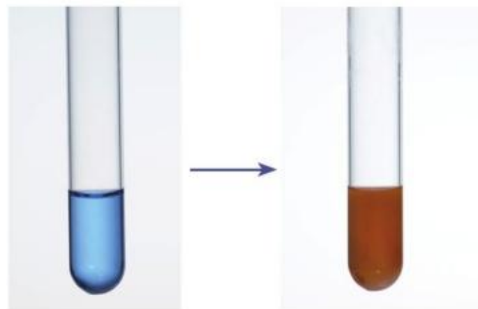
图3-18 乙醛与氢氧化铜反应
