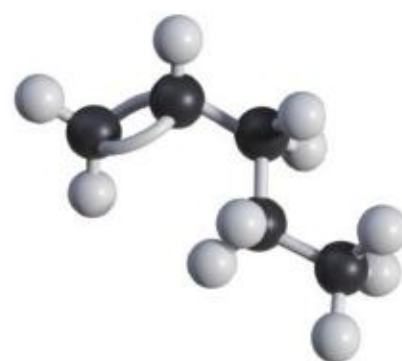
1-戊烯
