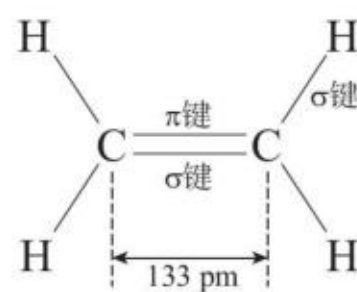
图2-2 乙烯的分子结构示意图
