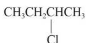
2-氯丁烷
