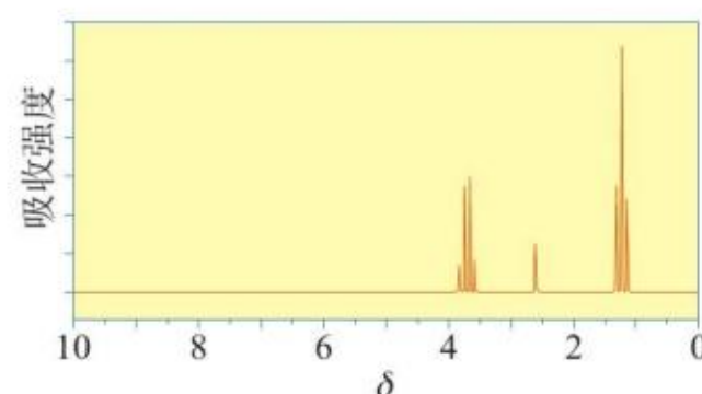
图3-8 乙醇的核磁共振氢谱
