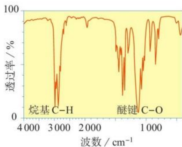
图2 红外光谱
