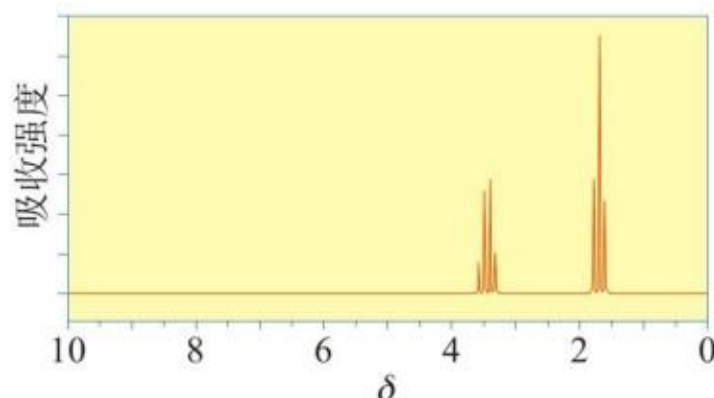
图 3-2 溴乙烷的核磁共振氢谱
