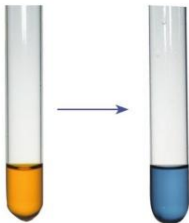
图 3-10 乙醇与酸性重铬酸钾溶液的反应
