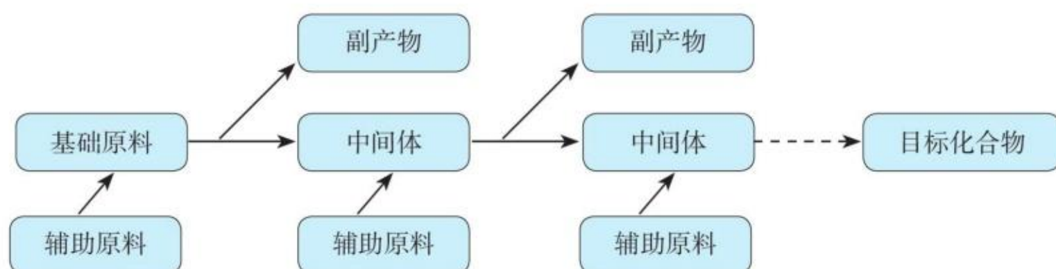
图3-28 有机合成过程示意图
