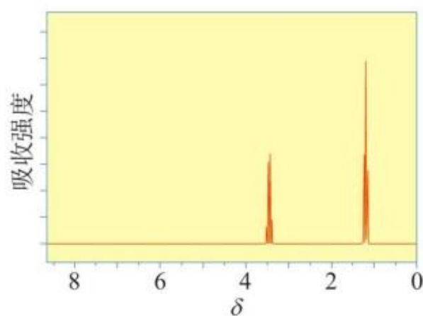
图3 核磁共振氢谱
