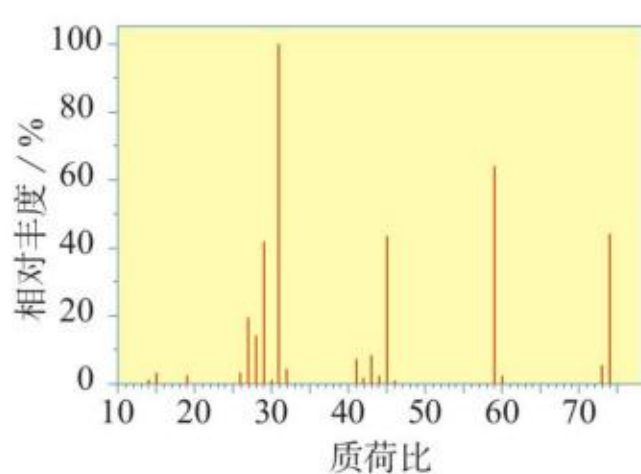
图1 质谱
