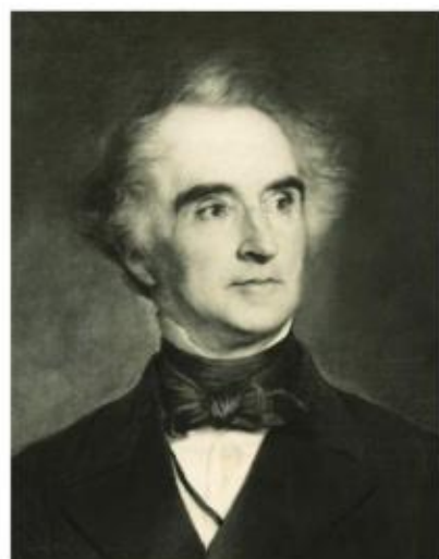
图1-11 李比希
