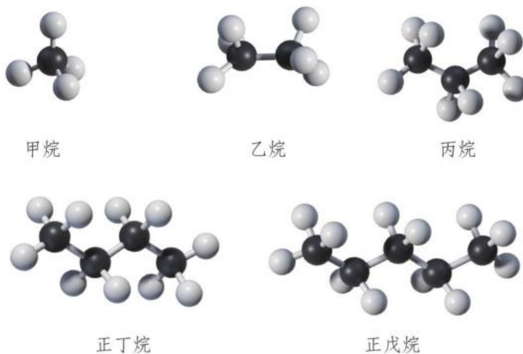
图 2-1 几种简单烷烃的分子结构模型
