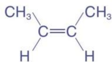
顺-2-丁烯
