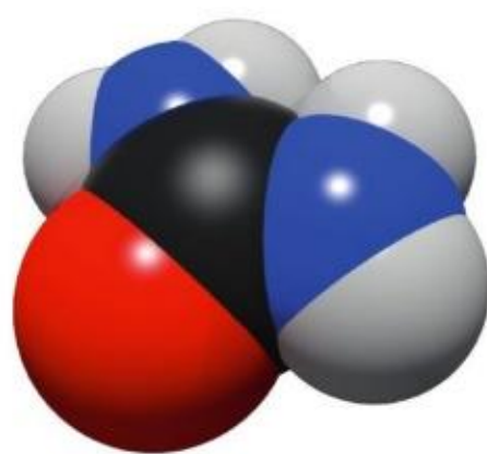
图1 尿素的分子结构模型
