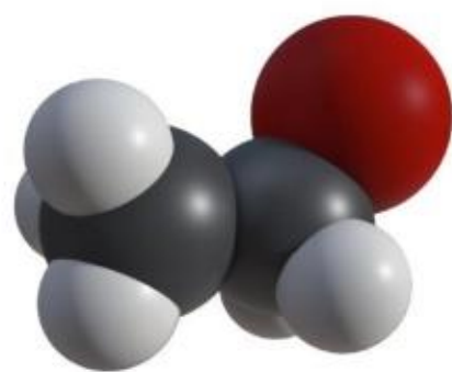
图 3-1 溴乙烷的分子结构模型
