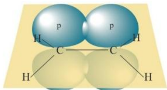
\pi 键
