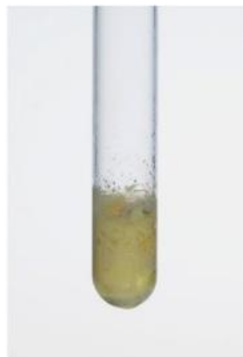
图4-12 蛋白质与浓硝酸的显色反应
