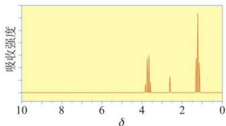
图1-18 未知物A的核磁共振氢谱
