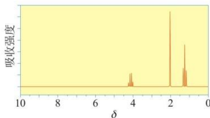
图 3-26 乙酸乙酯的核磁共振氢谱
