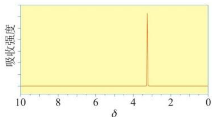
图1-19 二甲醚的核磁共振氢谱
