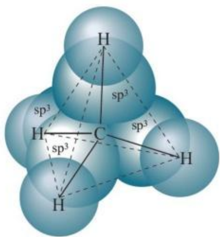
图 1-1 甲烷分子中的 \sigma 键示意图
