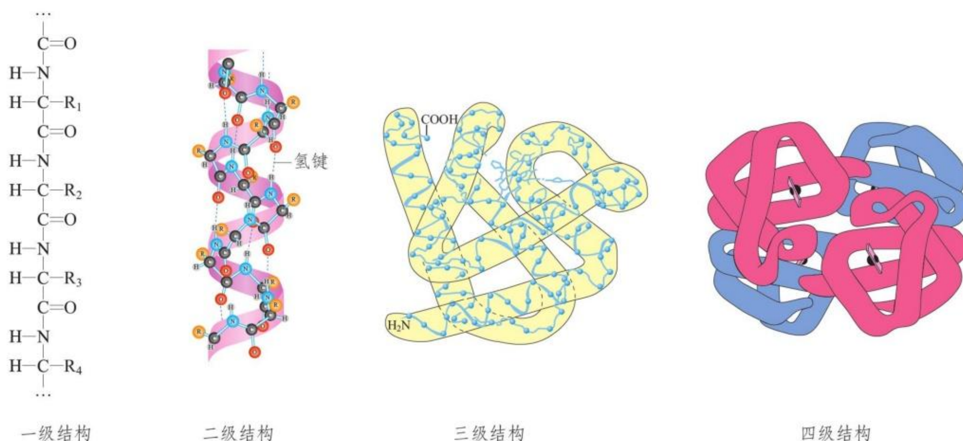
图4-9 蛋白质结构示意图
