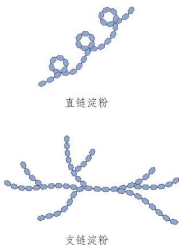
图4-3 直链淀粉和支链淀粉的结构示意图（其中每个小的六边形代表一个葡萄糖的环状结构单元）
