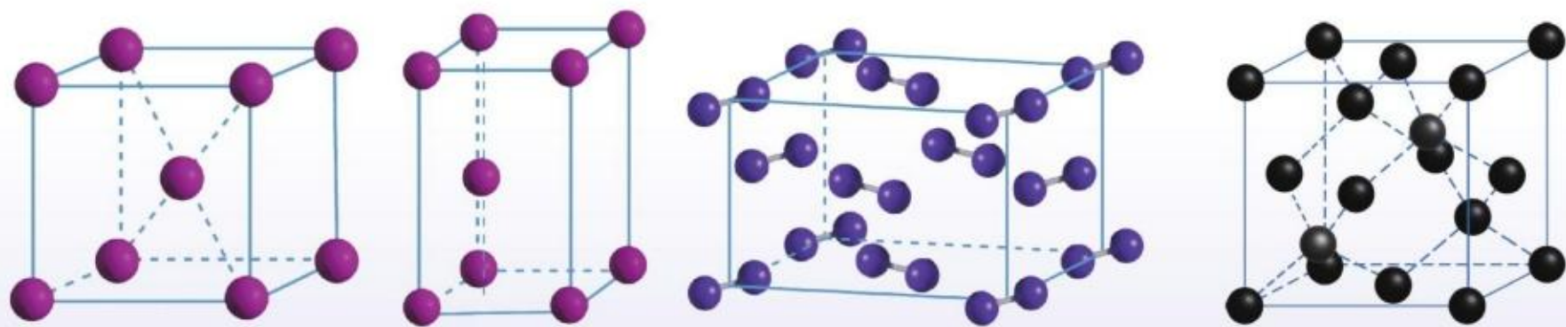
图3-11 钠、锌、碘、金刚石晶胞图
