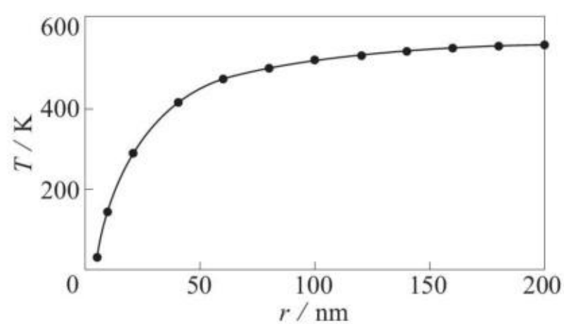
图3-34 金属铅的晶粒大小与熔点的关系
