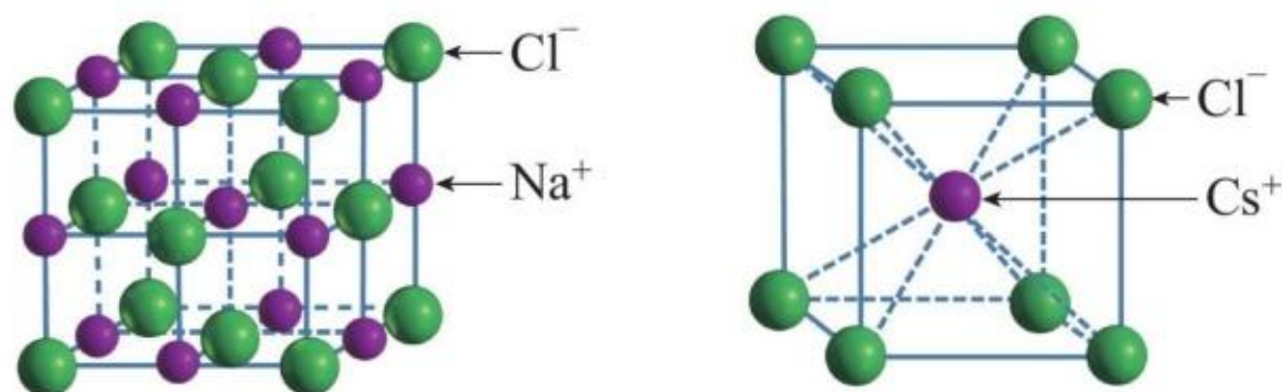
图3-30 NaCl和CsCl的晶胞
