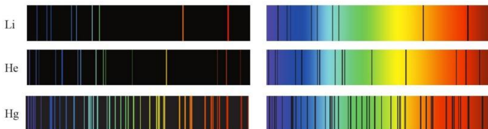
图 1-4 Li、He、Hg 的发射光谱（左）和吸收光谱（右）
