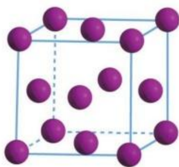
铜晶胞
