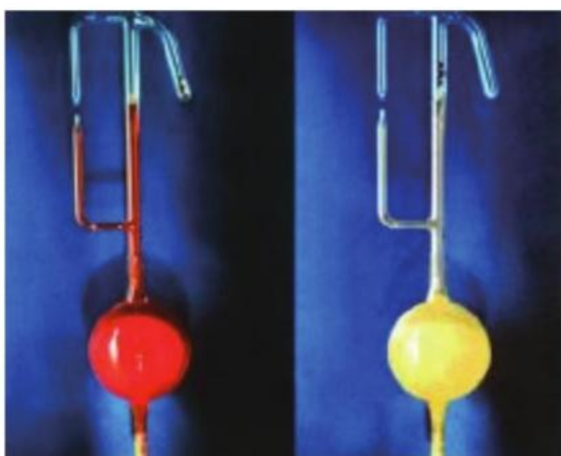
\text{PtF}_6 和Xe反应前后
