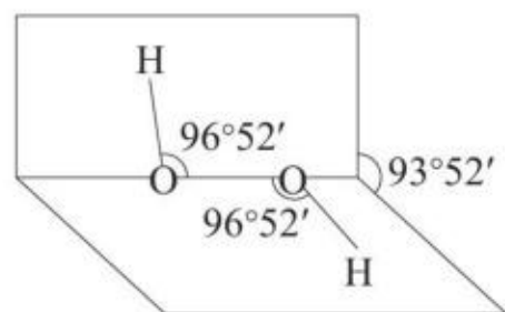
\text{H}_2\text{O}_2 分子结构示意图
