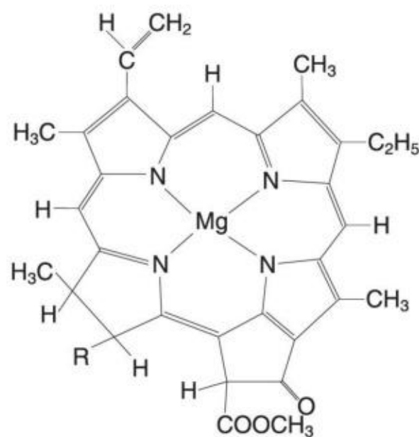
图3-43 卟啉配合物叶绿素的结构示意图
