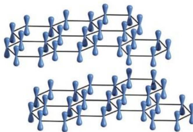
石墨结构中未参与杂化的 p 轨道
