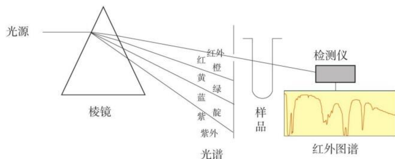
图2-5 红外光谱仪原理示意图
