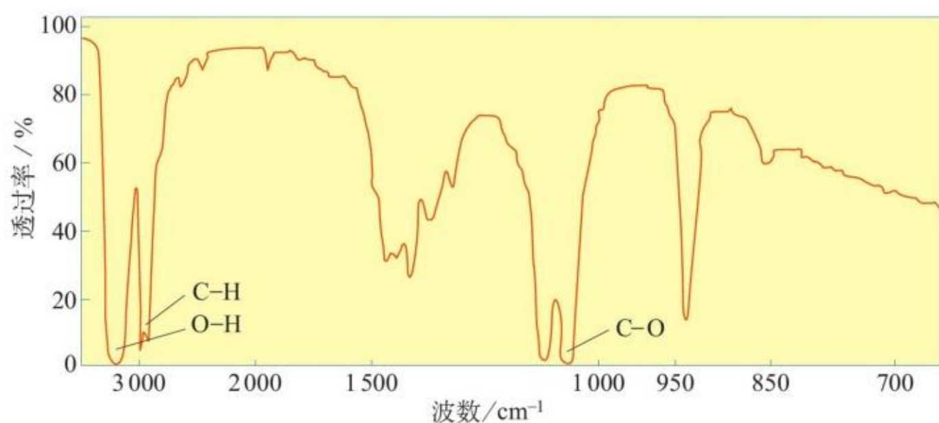
图2-6 某未知物的红外光谱
