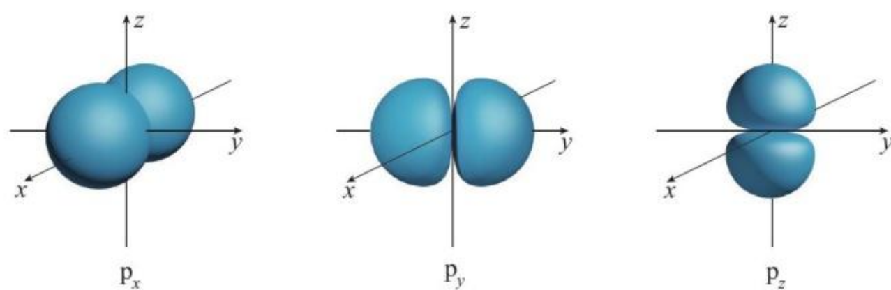
图 1-11 p_x 、 p_y 、 p_z 的电子云轮廓图
