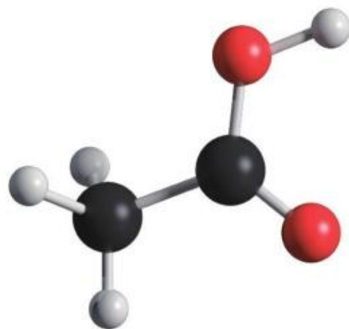
图 3-16 乙酸分子的空间结构
