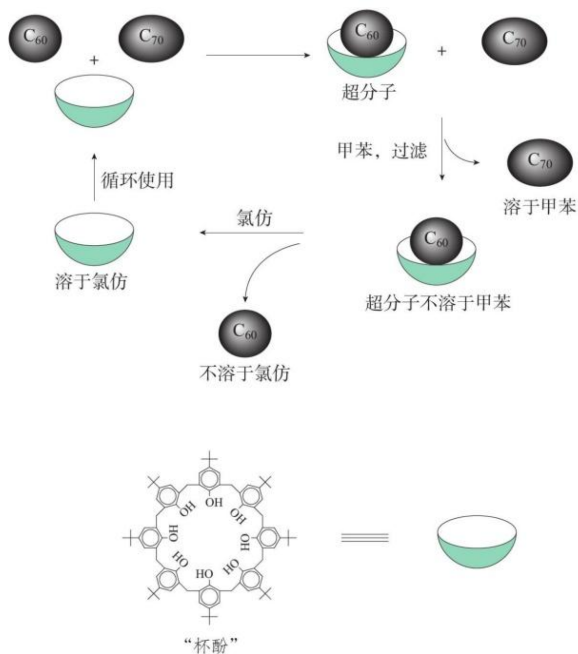
图3-44 分离 C_{60} 和 C_{70} 示意图（注：图中的下部分为“杯酚”）
