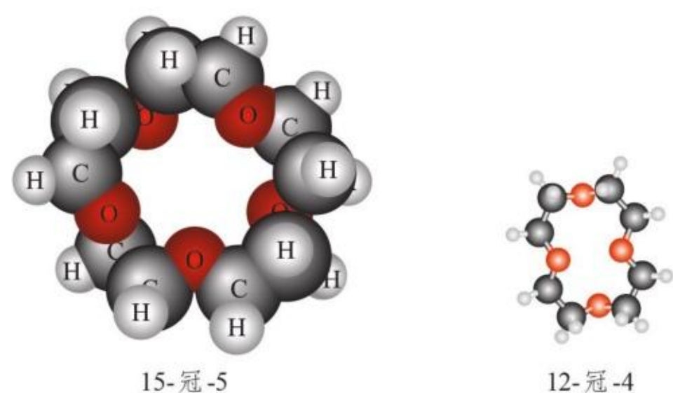
图3-45 冠醚
