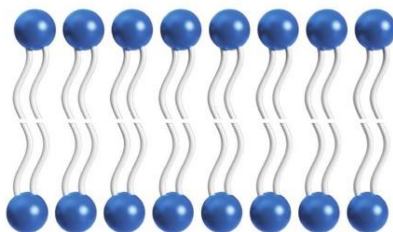
图2-20 细胞和细胞器的双分子膜
