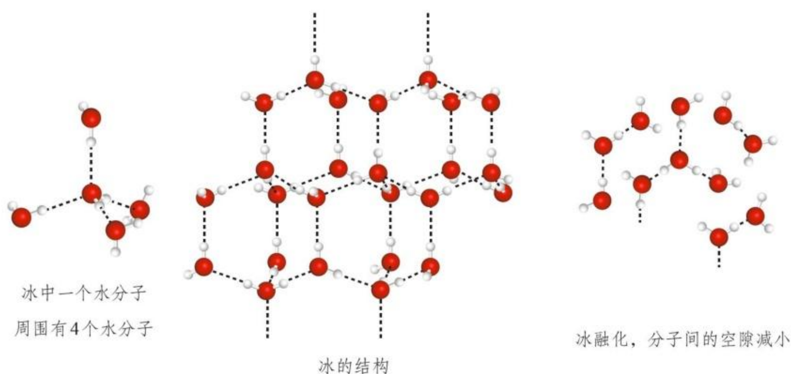
图3-18 冰和液态水的结构对比（虚线表示氢键）
