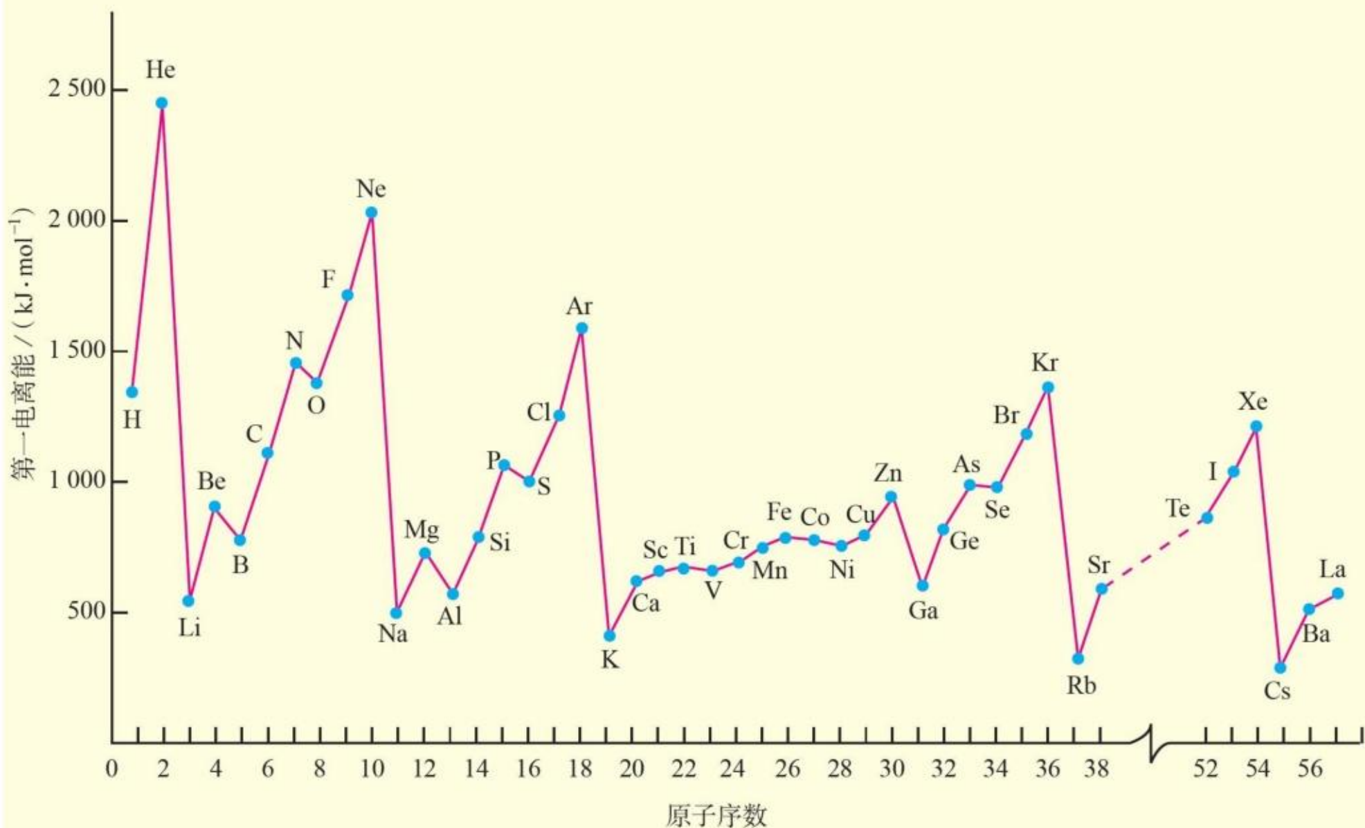
图1-22 元素的第一电离能的周期性
