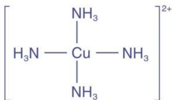
图 3-40 [\text{Cu}(\text{NH}_3)_4]^{2+}
