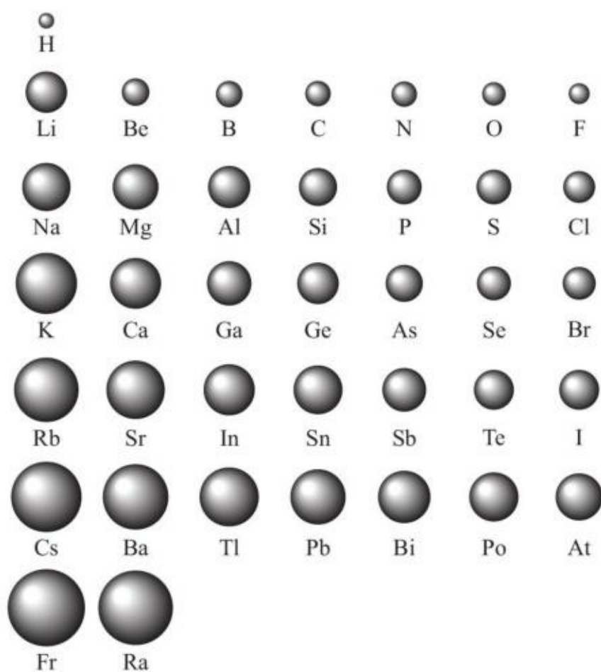
图 1-21 主族元素原子半径的周期性变化
