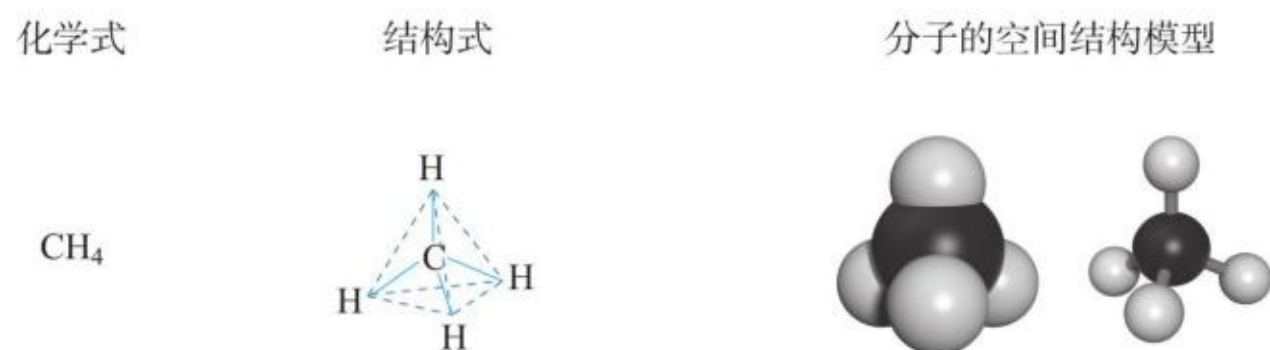
图2-12 \text{CH}_4 的空间结构模型
