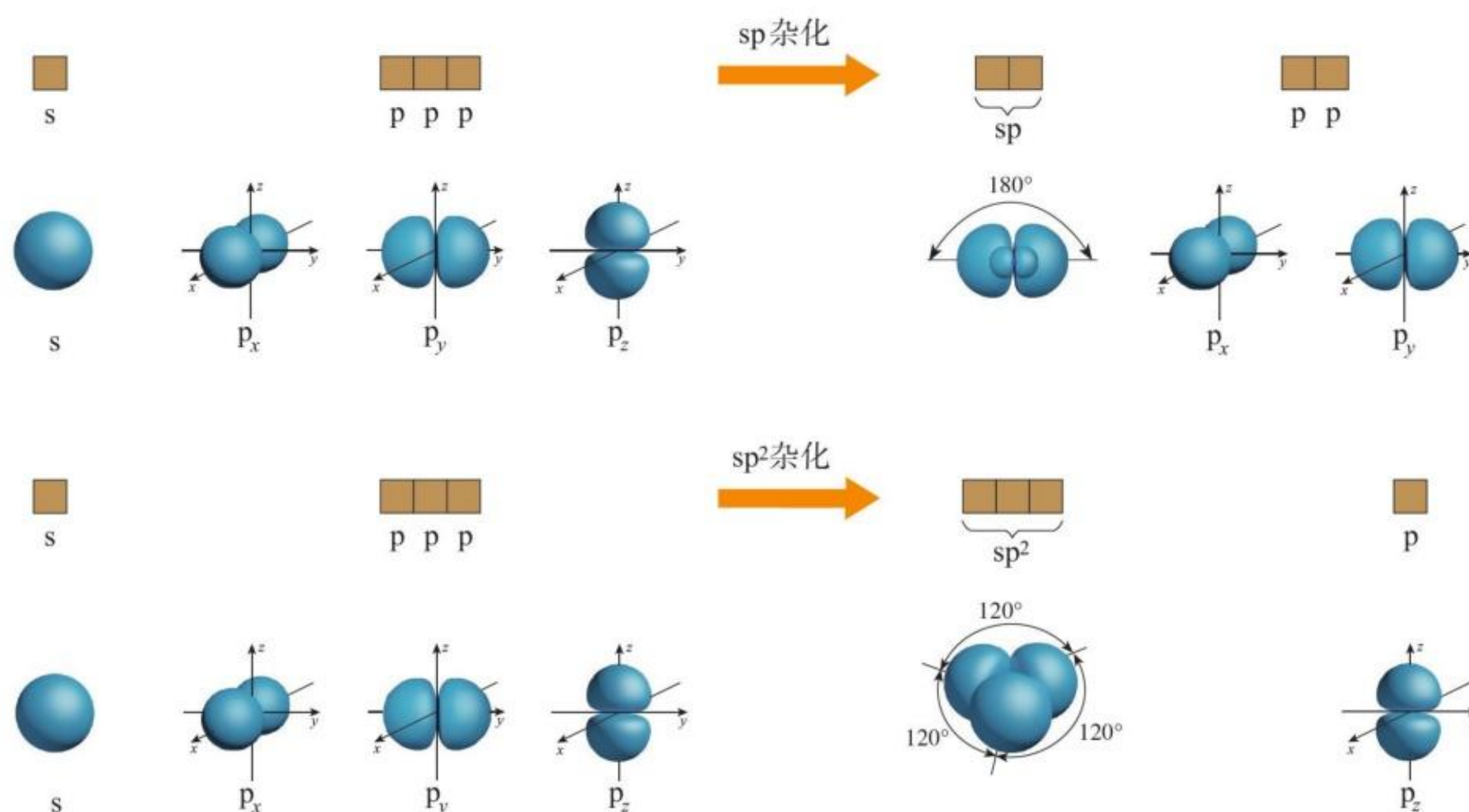
图 2-16 sp 杂化和 sp^2 杂化
