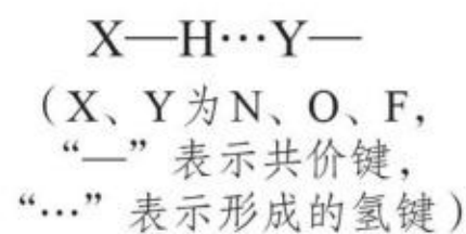
图2-25 常见氢键的类型
