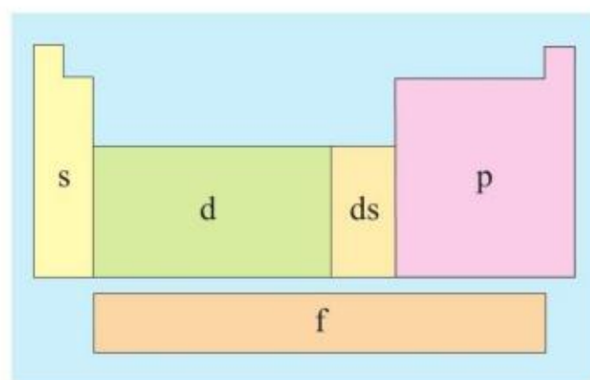
图1-19 元素周期表分区的简图
