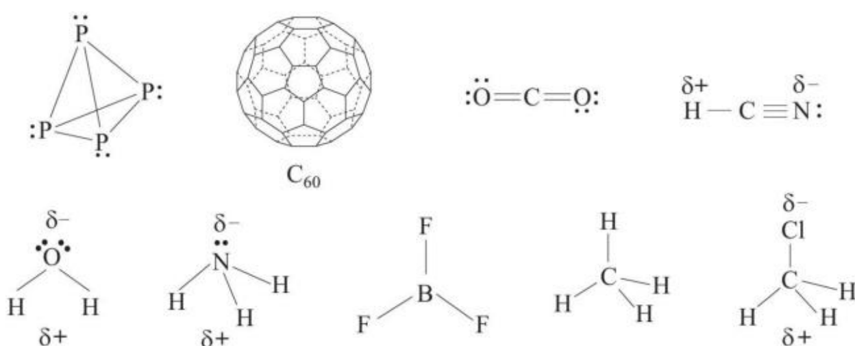
图2-18 常见的极性分子和非极性分子
