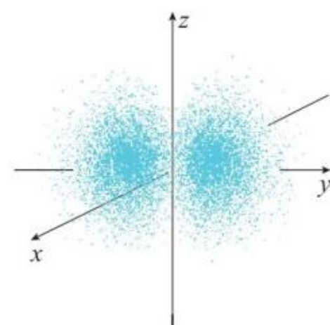
图 1-10 2p_y 电子云
