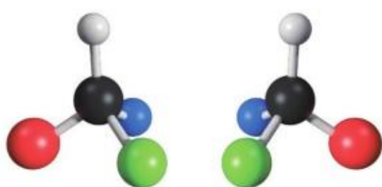
图 2-32 互为镜像的两个分子
