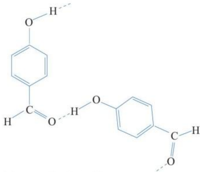
图2-27 分子间氢键
