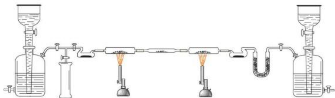
图 1-26 拉姆齐的实验装置图
