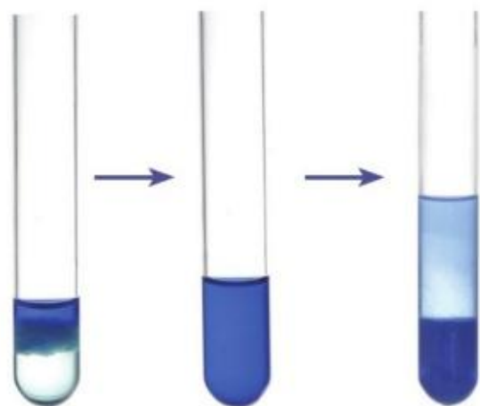
图 3-39 向硫酸铜溶液中加入氨水和乙醇
