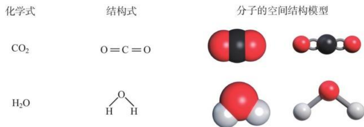
图2-10 \text{CO}_2 和 \text{H}_2\text{O} 的空间结构模型
