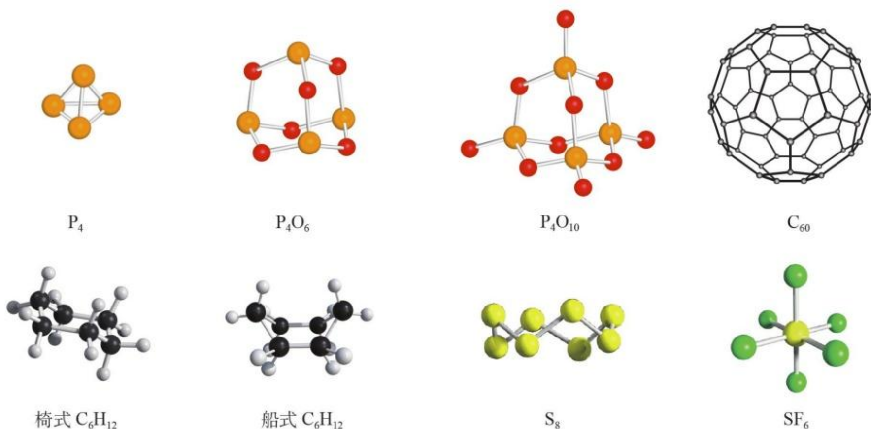
图2-13 一些分子的空间结构模型
