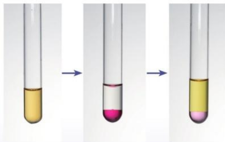
图2-31 碘在水和四氯化碳中的溶解性
