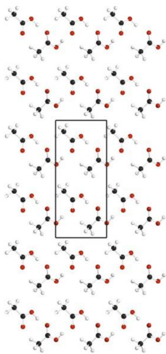
乙酸晶体
