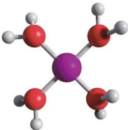
图 3-37 [\text{Cu}(\text{H}_2\text{O})_4]^{2+}
