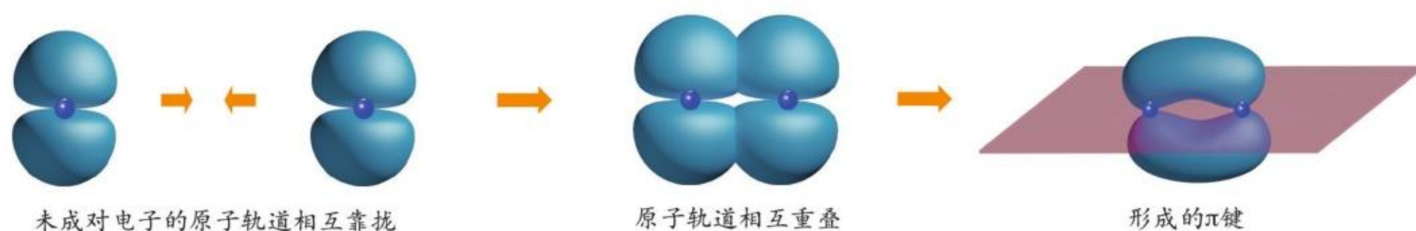
图2-3 p-p \pi 键的形成
