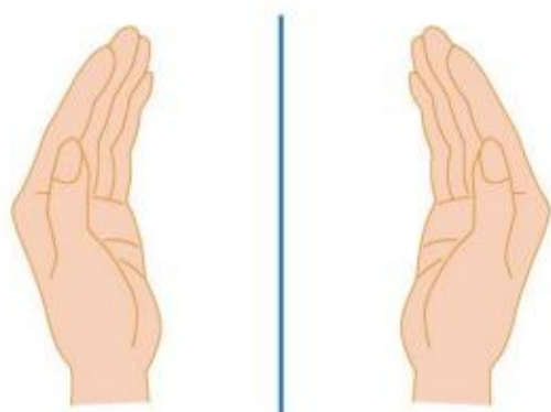
图 2-34 左右手互为镜像
