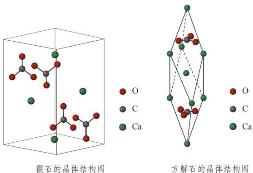
图4 霏石和方解石的晶体结构
