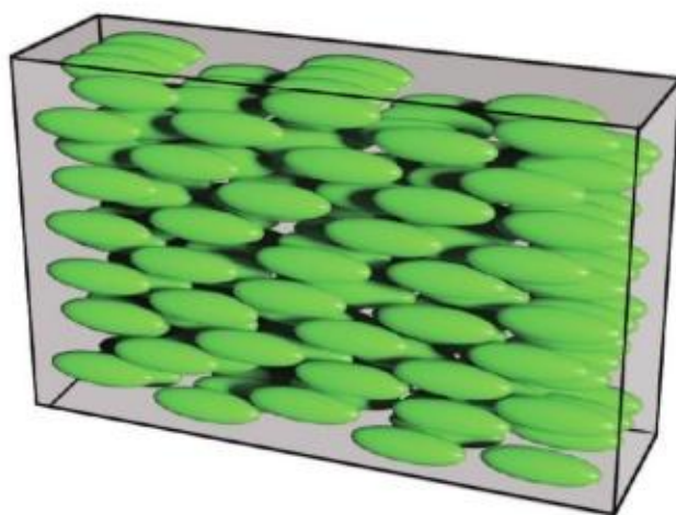
图3-3 棒状分子液晶内部分子排列示意图
