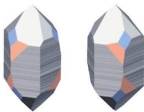
图3-23 石英的左、右型晶体
