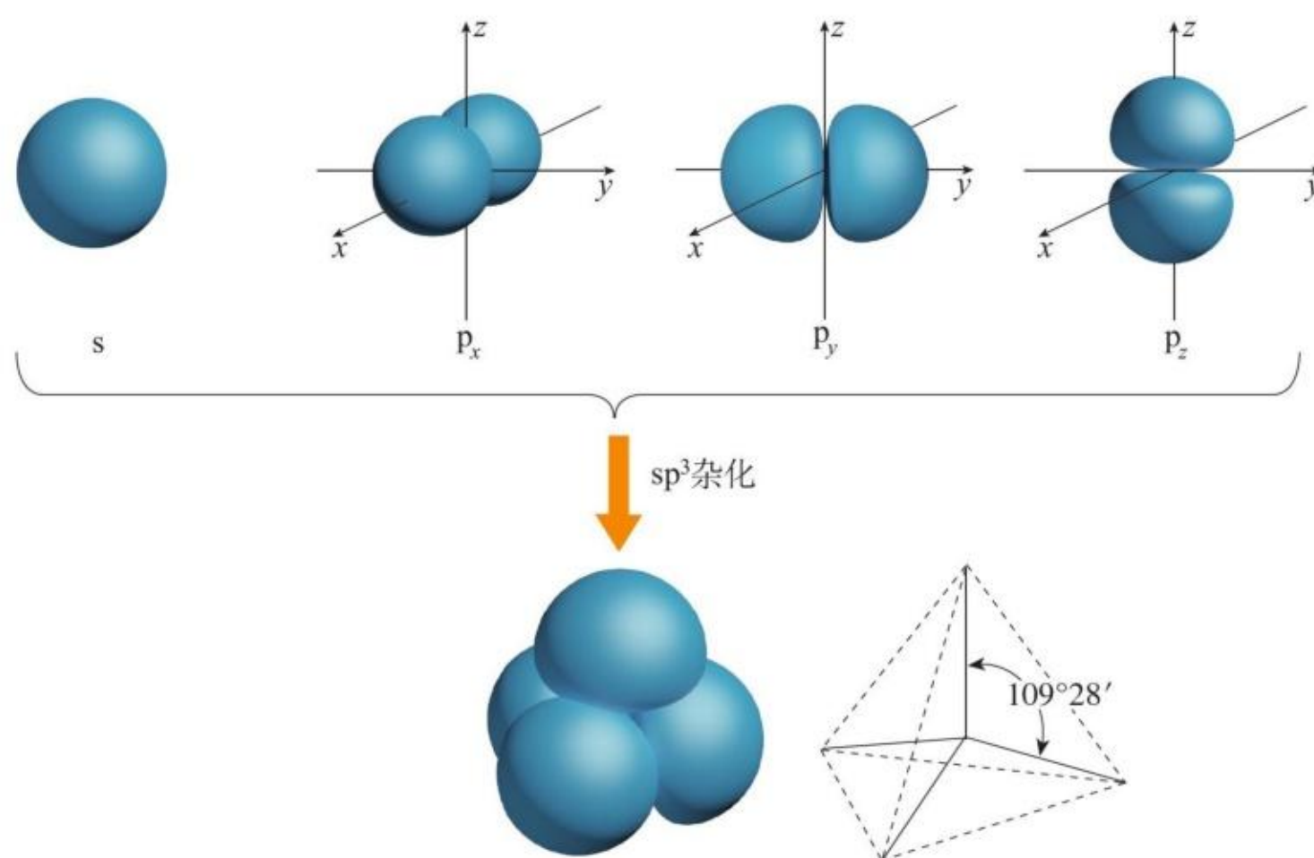
图 2-15 sp^3 杂化轨道
