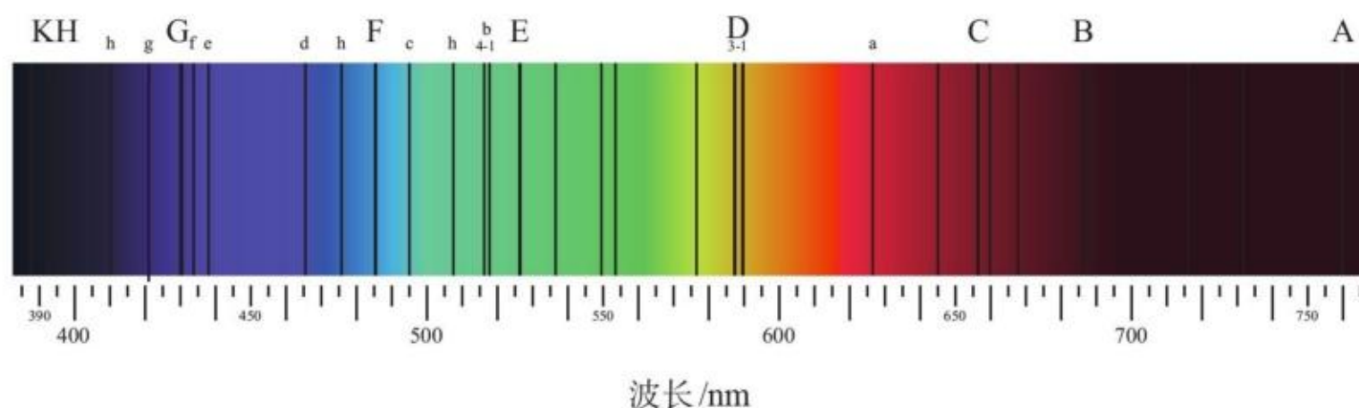
图1-6 太阳光谱里的夫琅禾费线
