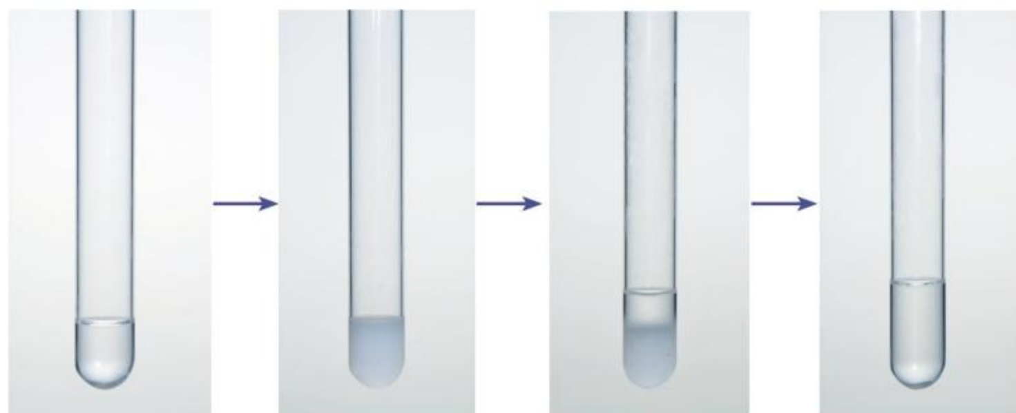
图3-42 向 \text{NaCl} 溶液中滴加 \text{AgNO}_3 溶液和氨水
