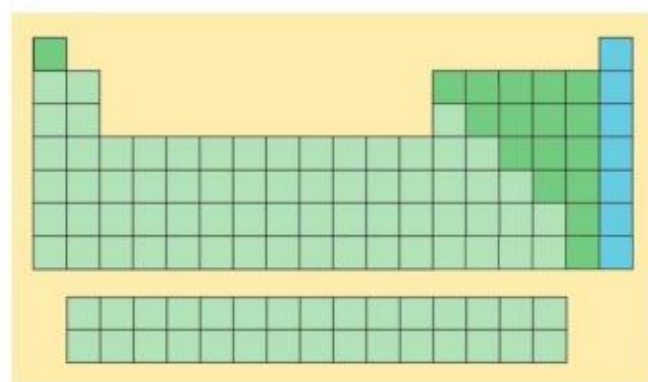
图1-18 元素周期表中的非金属三角区
