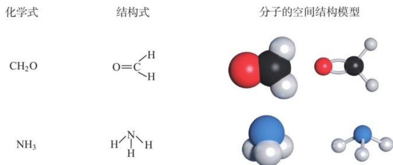
图2-11 \text{CH}_2\text{O} 和 \text{NH}_3 的空间结构模型
