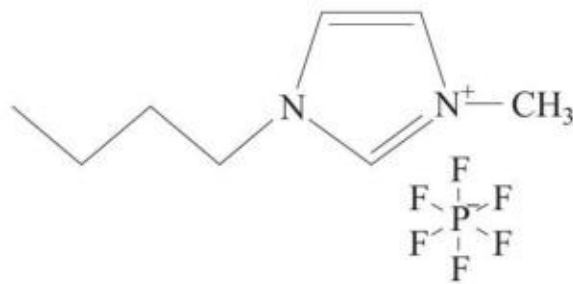
图3-31 1-丁基-3-甲基咪唑六氟磷酸盐
