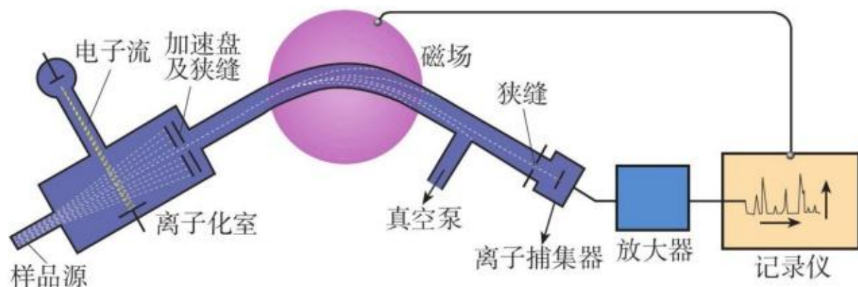
图2-8 质谱仪原理示意图
