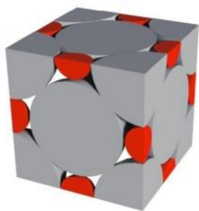
图3-10 NaCl晶胞
