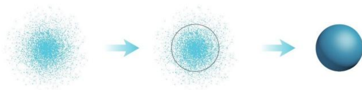
图1-8 电子云轮廓图的绘制过程
