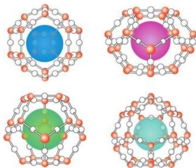
图3-20 天然气水合物示意图
