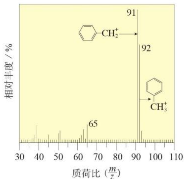
图2-9 甲苯分子的质谱图
