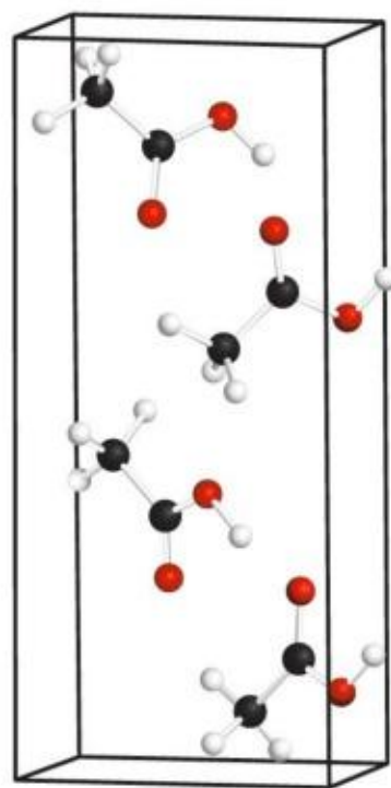
乙酸晶胞
