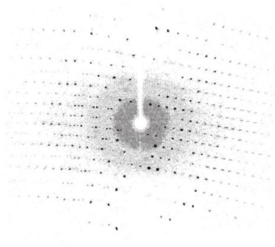
图3-13 单晶衍射图
