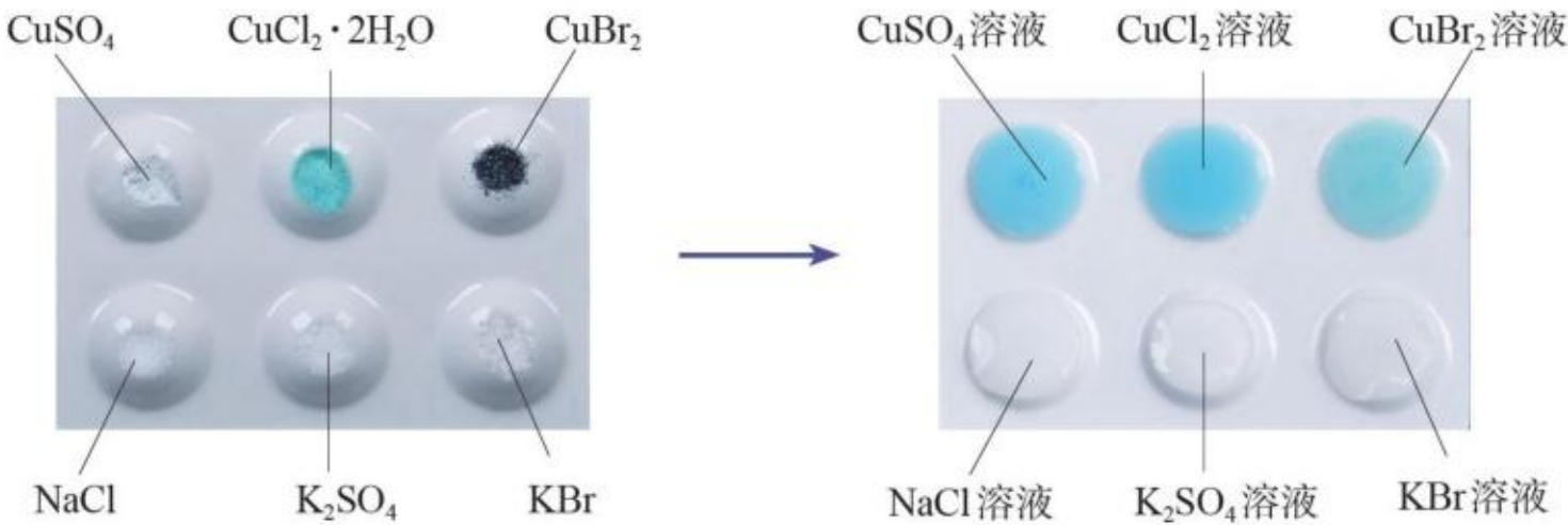
图3-36 几种固体及其溶液的颜色
