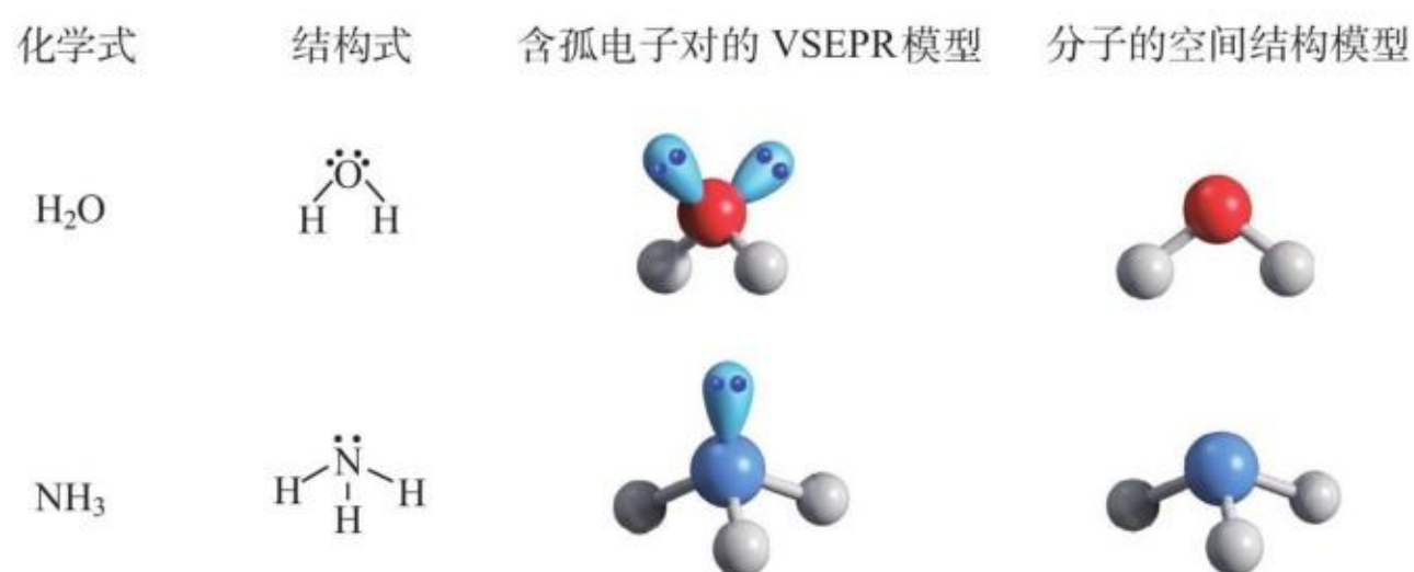
图2-14 \text{H}_2\text{O} 、 \text{NH}_3 的VSEPR模型和空间结构
