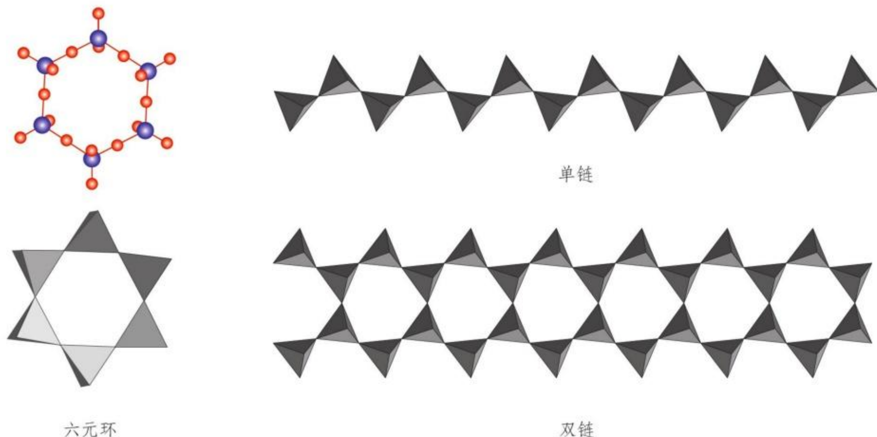
图3-33 硅酸盐晶体中的阴离子举例
