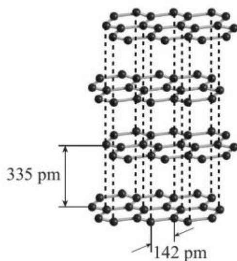
石墨的层状结构
