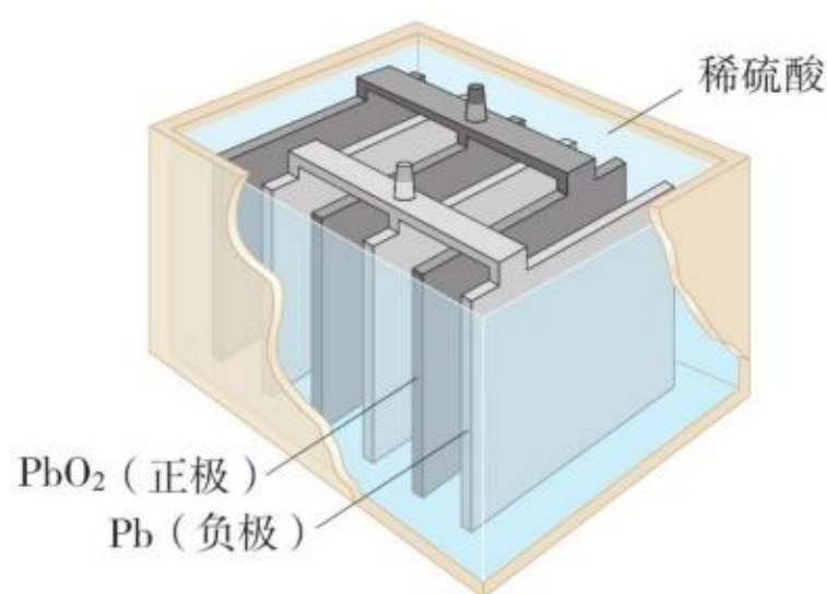
图4-4 铅酸蓄电池的构造示意图
