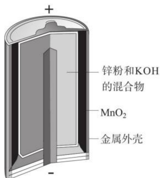
图 4-3 碱性锌锰电池的构造示意图
