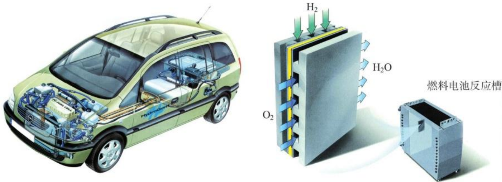
图4-6 车用燃料电池示意图
