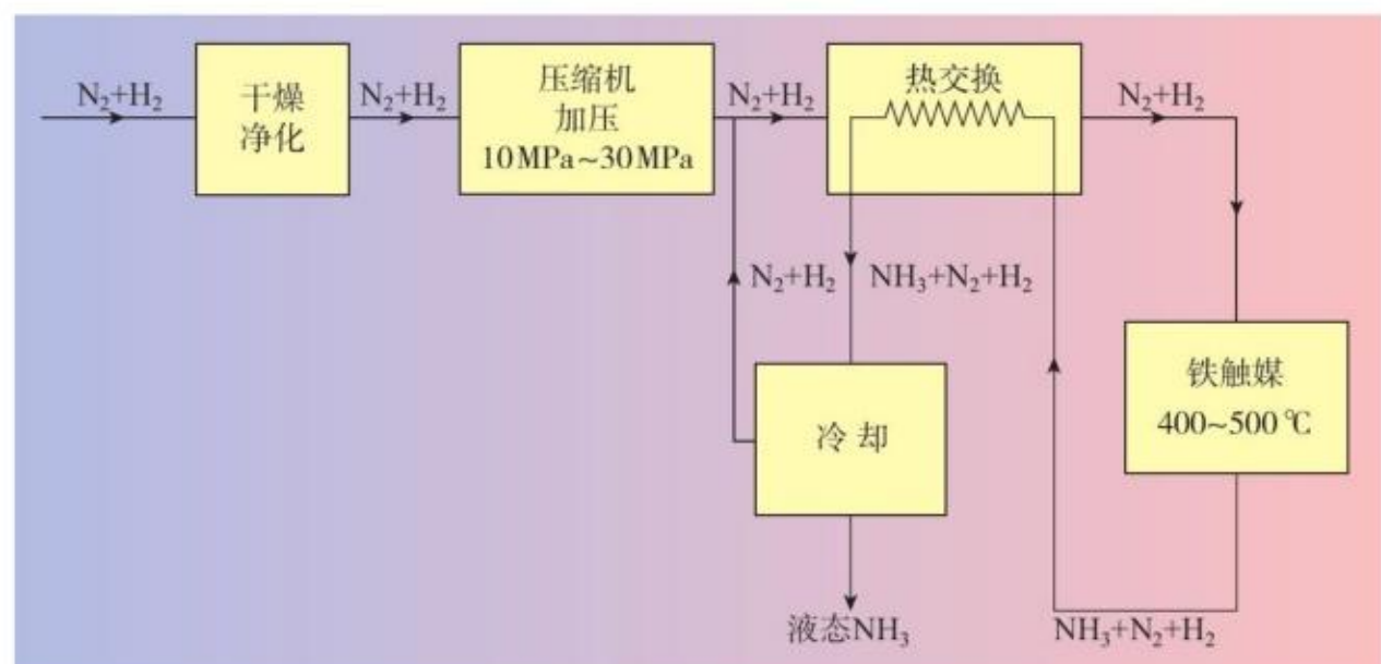
图 2-13 合成氨生产流程示意图
