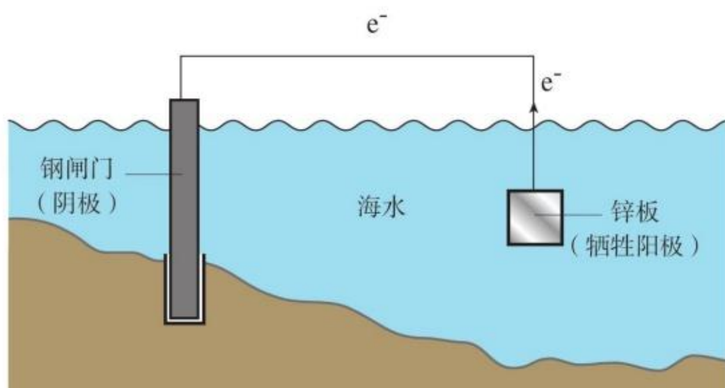
图4-24 牺牲阳极法示意图
