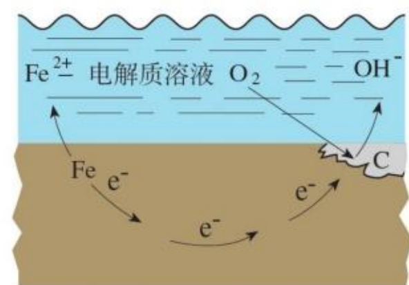
图4-20 钢铁的吸氧腐蚀示意图
