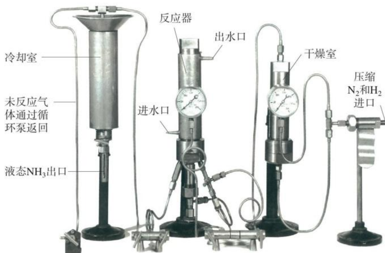
图2-14 哈伯合成氨实验所用的装置
