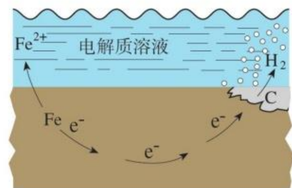
图4-19 钢铁的析氢腐蚀示意图
