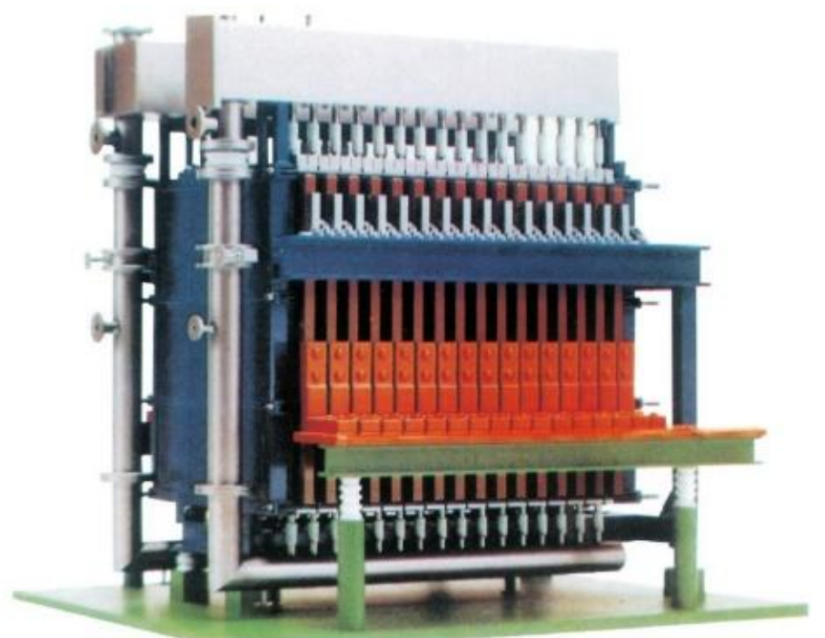
图4-12 离子交换膜电解槽
