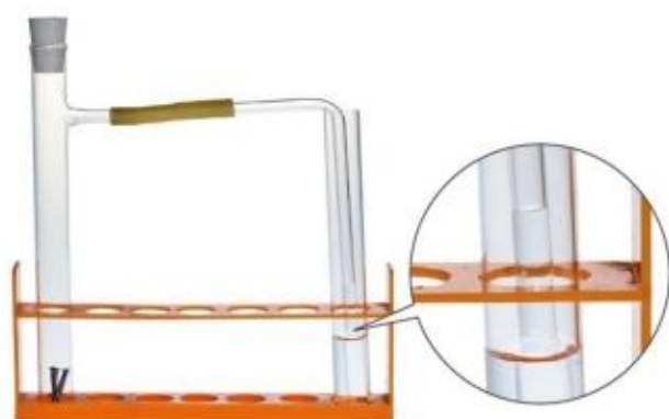
图4-21 铁钉的吸氧腐蚀实验
