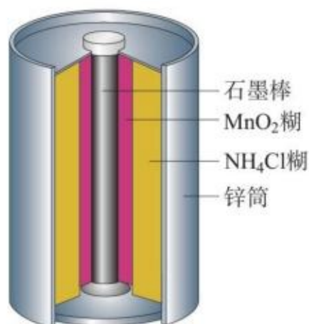
普通锌锰电池构造示意图
