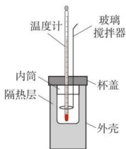
图1-3 简易量热计示意图
