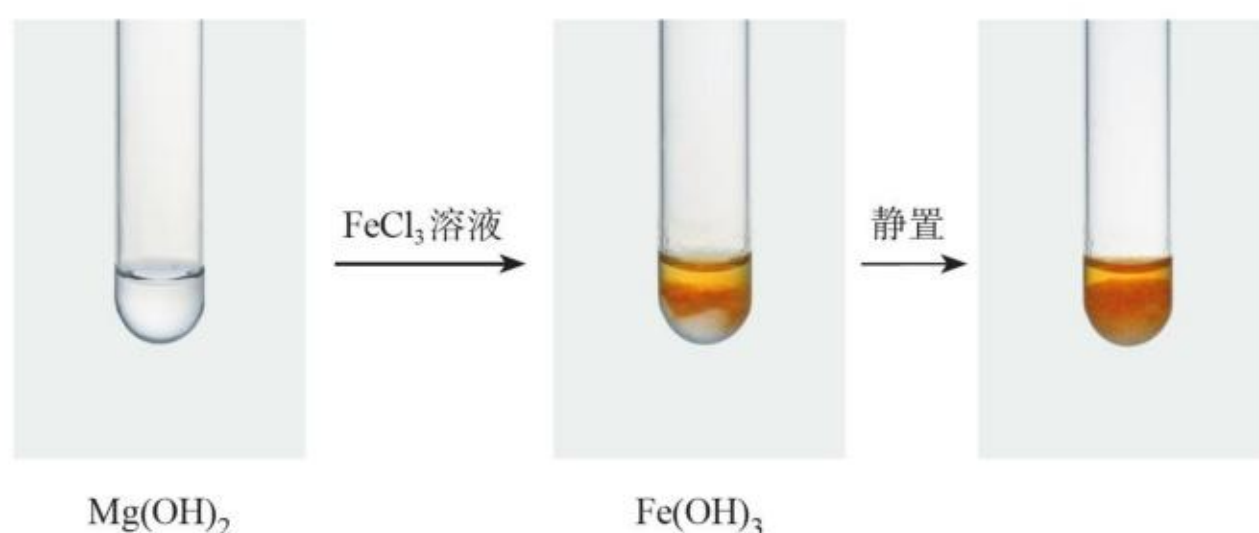
图3-16 沉淀的转化（Ⅱ）
