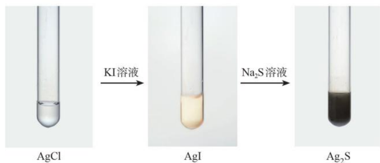
图3-15 沉淀的转化 ( I )
