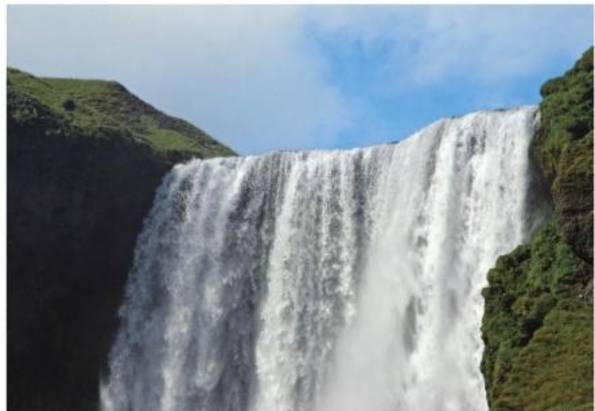
图2-9 水总是自发地从高处流向低处
