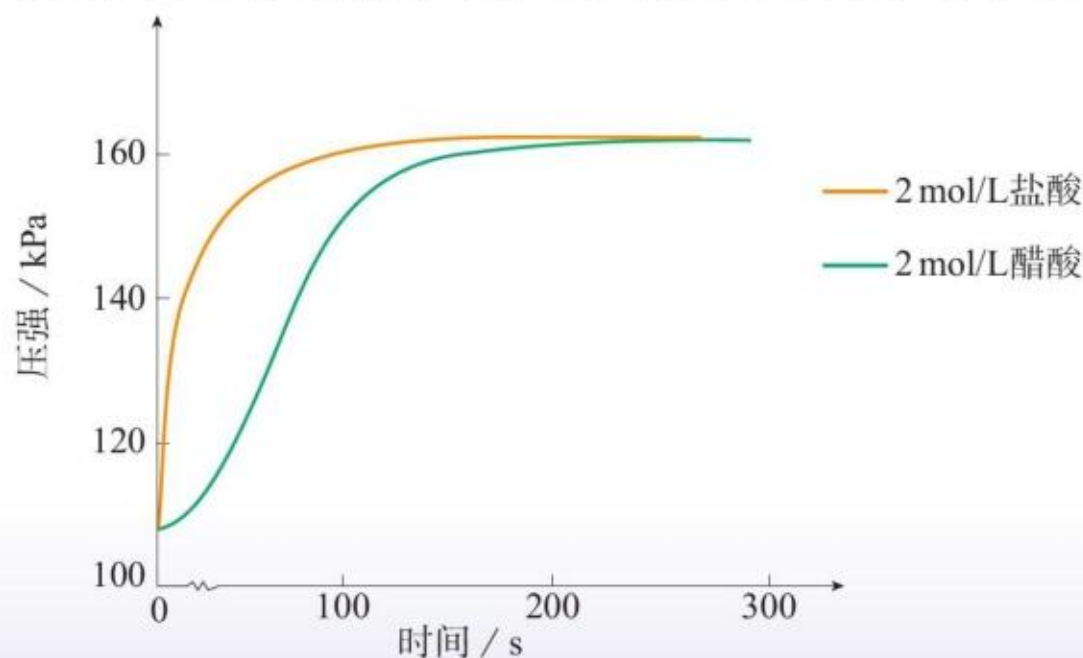
图3-4 镁与盐酸、醋酸反应时气体压强随时间的变化示意图
