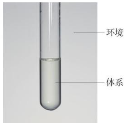
图 1-2 体系与环境示意图
