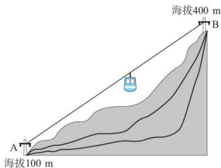
图 1-7 人的势能变化与上山的途径无关
