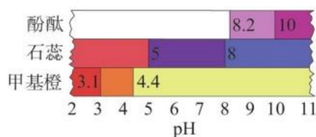
图3-12 几种常用指示剂的变色范围
