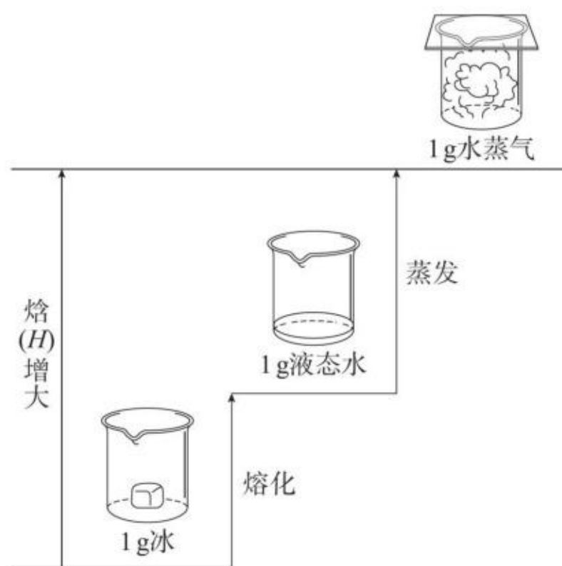
图 1-6 水的聚集状态变化时的焓变示意图
