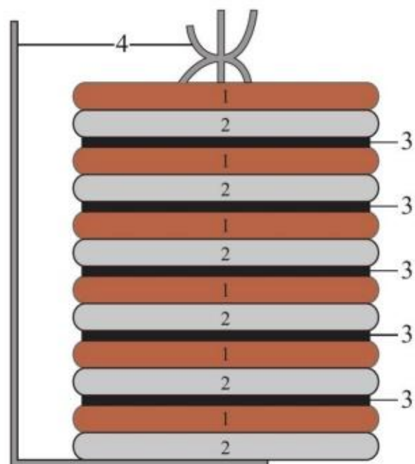
图4-8 伏打电堆示意图
