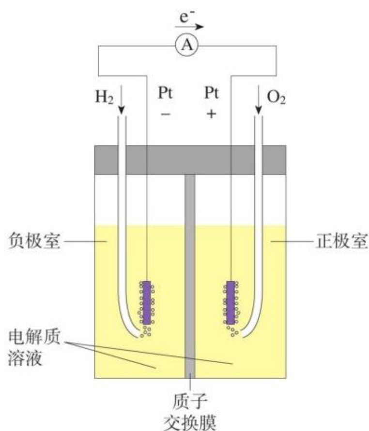
图4-7 氢氧燃料电池工作原理示意图
