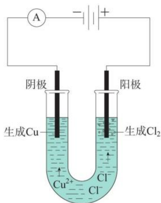
图4-9 氯化铜溶液的电解装置示意图
