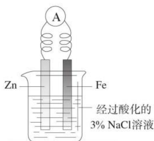
图4-26 牺牲阳极法实验（1）
