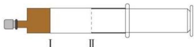
图2-6 压强对化学平衡的影响
