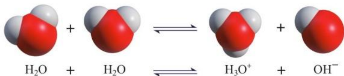
图 3-6 水分子电离过程示意图
