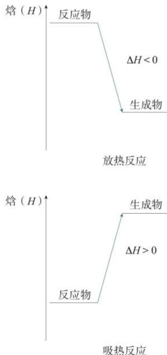
图 1-4 化学反应中焓的变化示意图
