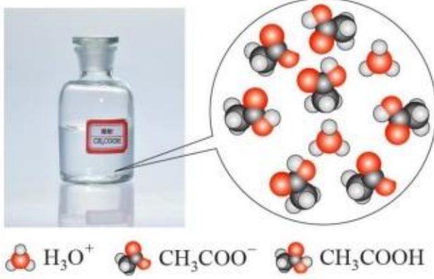
图3-2 CH 3 COOH在水中电离示意图
