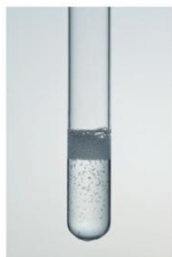
图3-3 向醋酸中滴加碳酸钠溶液
