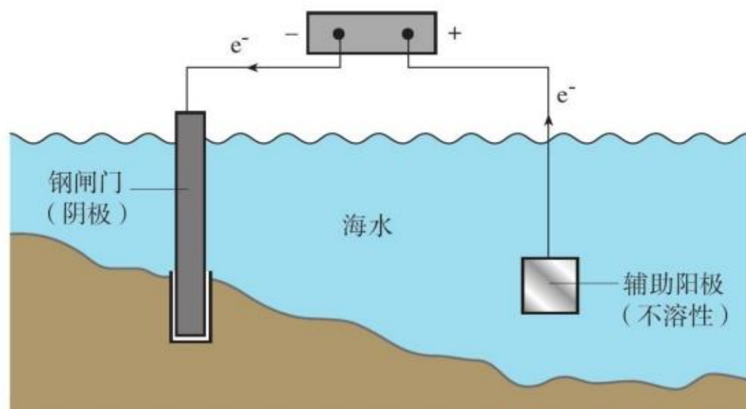
图4-28 外加电流法示意图
