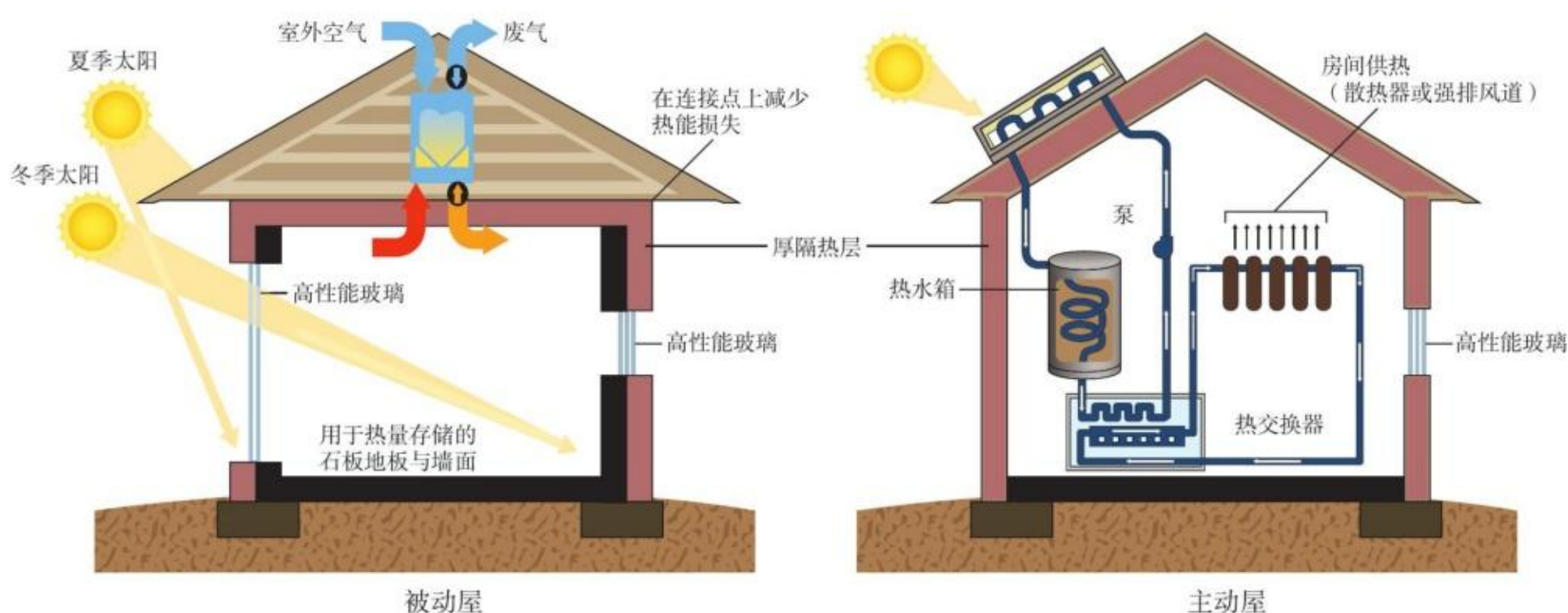
图4.2 被动屋与主动屋加热的对比
