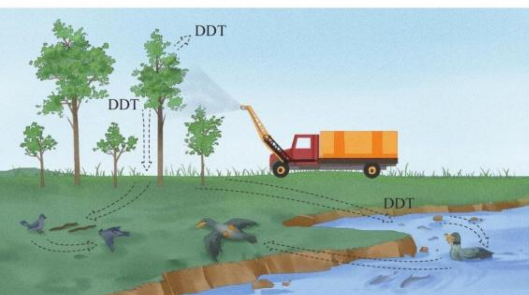
图 1.13 DDT在食物链中的传递
