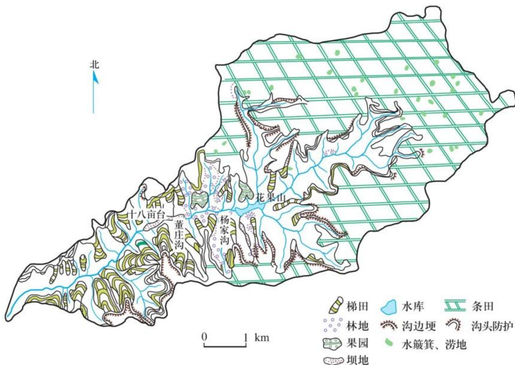
图4.8 南小河沟小流域综合治理措施示意
