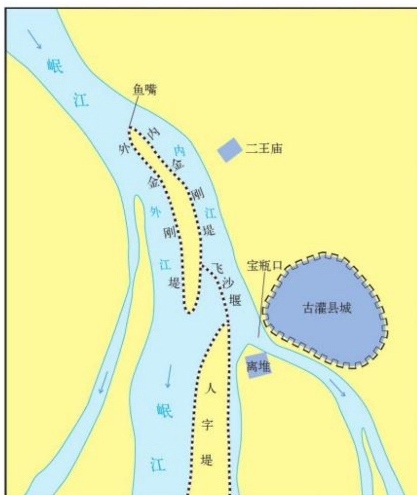
图2.4 都江堰水利工程示意
