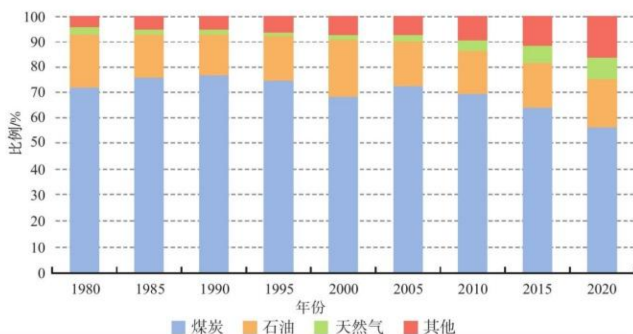
图4.18 1980—2020年我国能源消费结构
