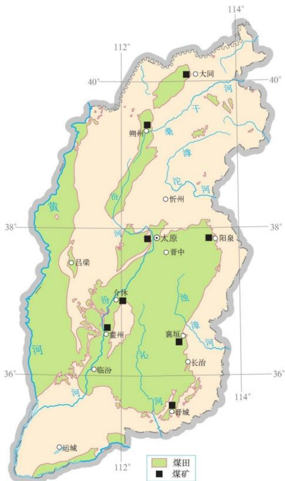
图2.7 山西省煤炭资源的分布
