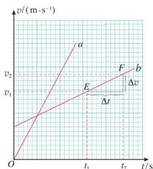
图1.4-2 从 v-t 图像看物体的加速度
