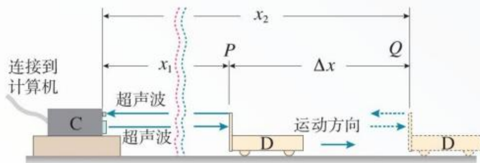
图1.3-7 另一种位移传感器测速度的原理
