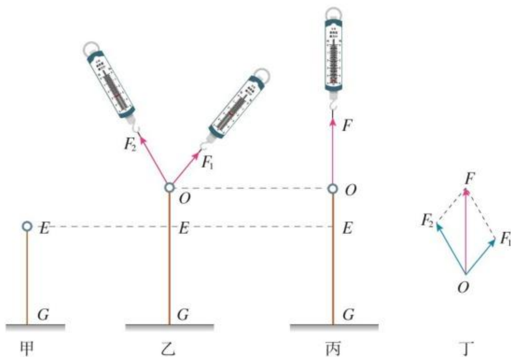
图 3.4-3 探究二力合成规律实验示意图
