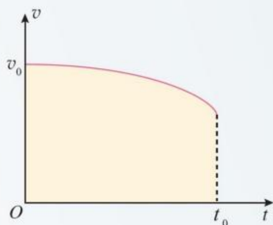
图2.3-5 位移等于 v-t 曲线下面的面积
