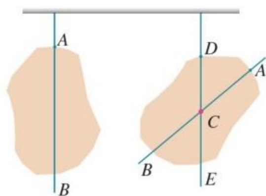
图 3.1-3 确定薄板的重心
