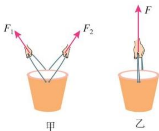
图3.4-1 水桶所受拉力示意图
