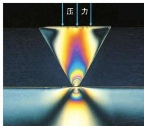
图 3.1-5 有机玻璃的形变
