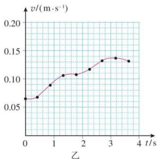
图 1.3-4 某同学手拉纸带运动的 v-t 图像
