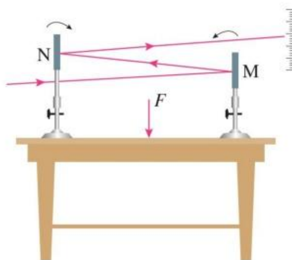
图 3.1-6 观察微小形变示意图
