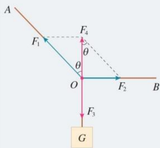
图3.5-3 绳索连接点受力示意图
