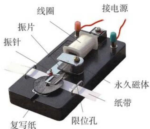
图 1.2-7 电磁打点计时器
