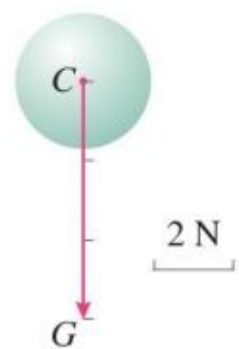
图 3.1-4 力的图示
