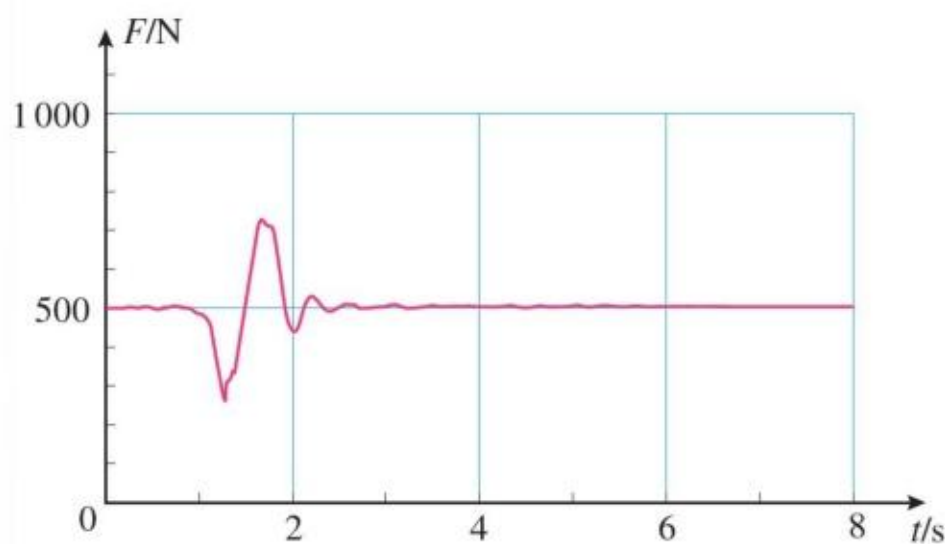
图 4.6-4 下蹲过程
