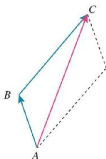
图 3.4-8 人的位移
