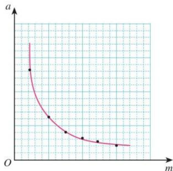
图4.2-4 双曲线
