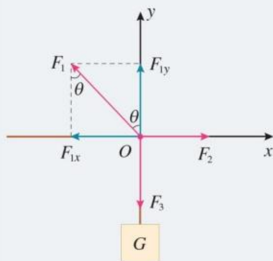
图3.5-4 正交分解法
