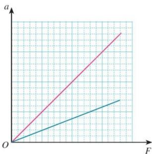
甲 猜想中的 a - F 图像
