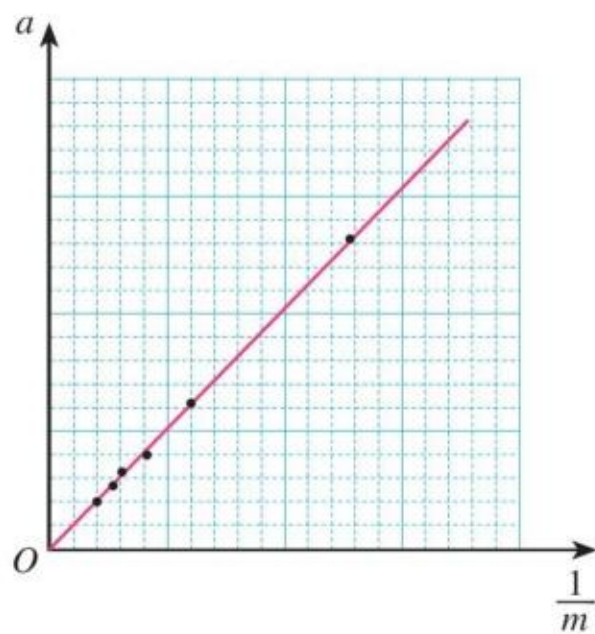
图 4.2-5 过原点的直线
