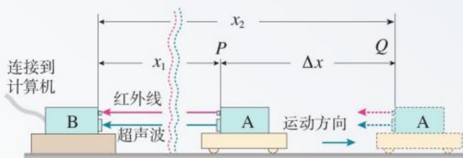
图1.3-6 位移传感器测速度的原理
