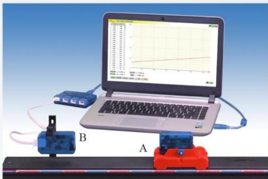
图1.3-5 实验室用位移传感器测速度的装置
