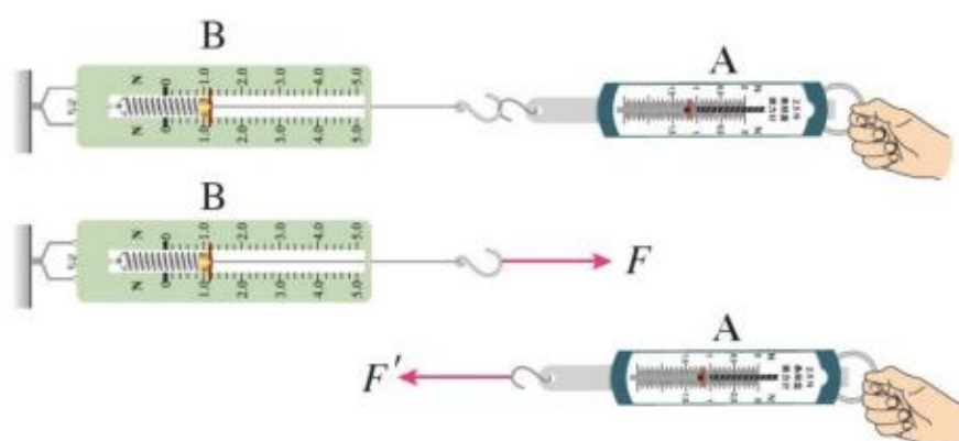
图3.3-3 实验装置
