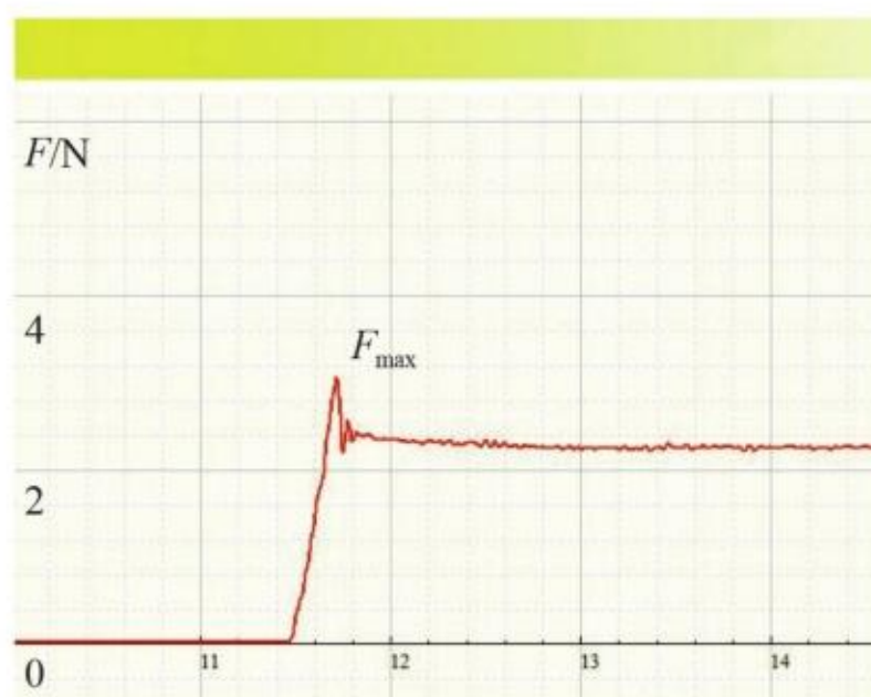
图 3.2-5 F-t 图像
