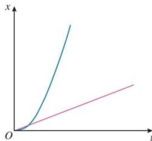
图 1.2-6 x-t 图像
