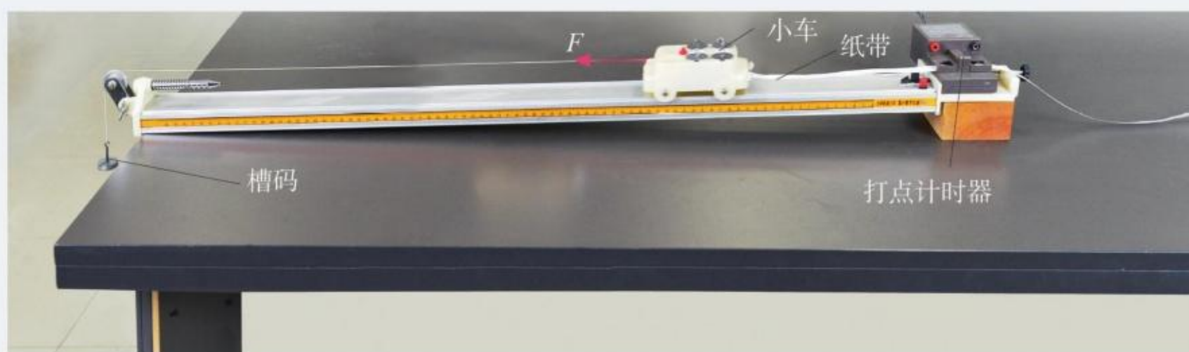
图4.2-2 实验装置
