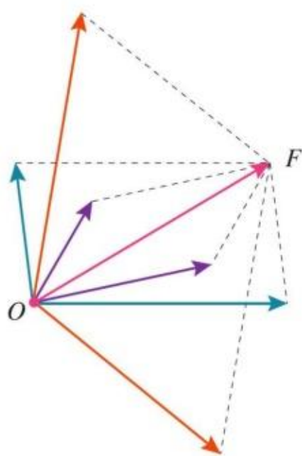
图 3.4-5 力的分解
