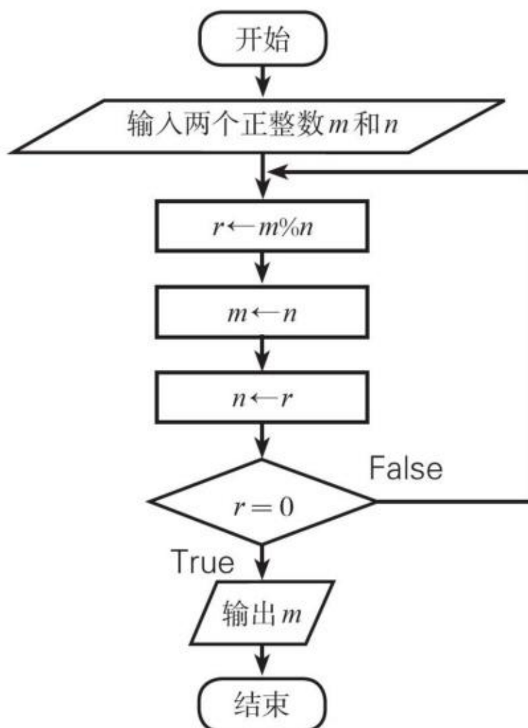
图 2.2.5 欧几里得算法流程图
