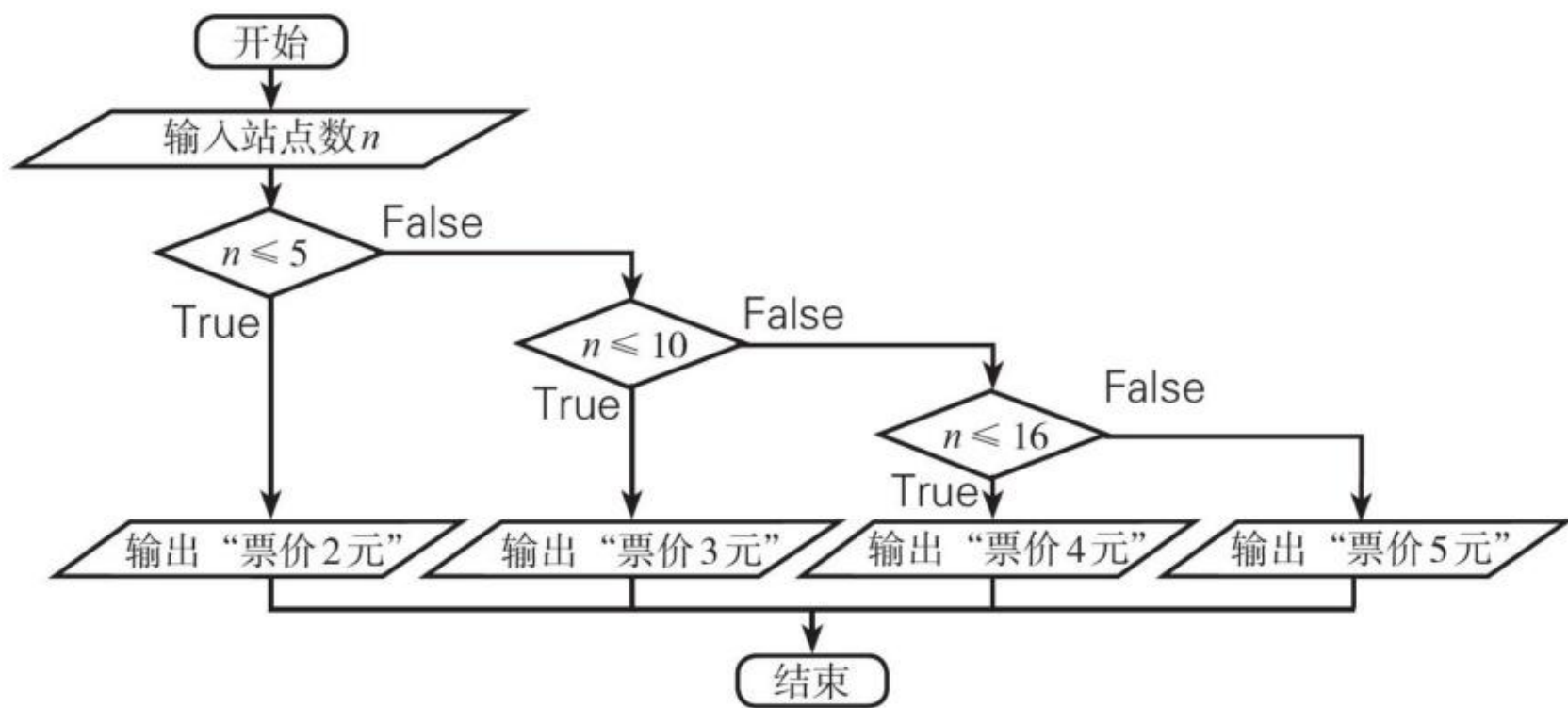
图2.3.4 分段计程票价的多分支算法流程图
