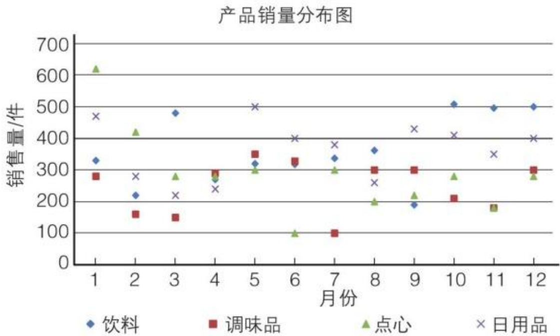
图3.3.20 散点图示例
