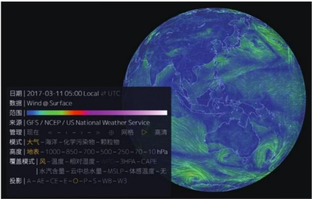
图3.3.25 地球大气环流可视化地图
