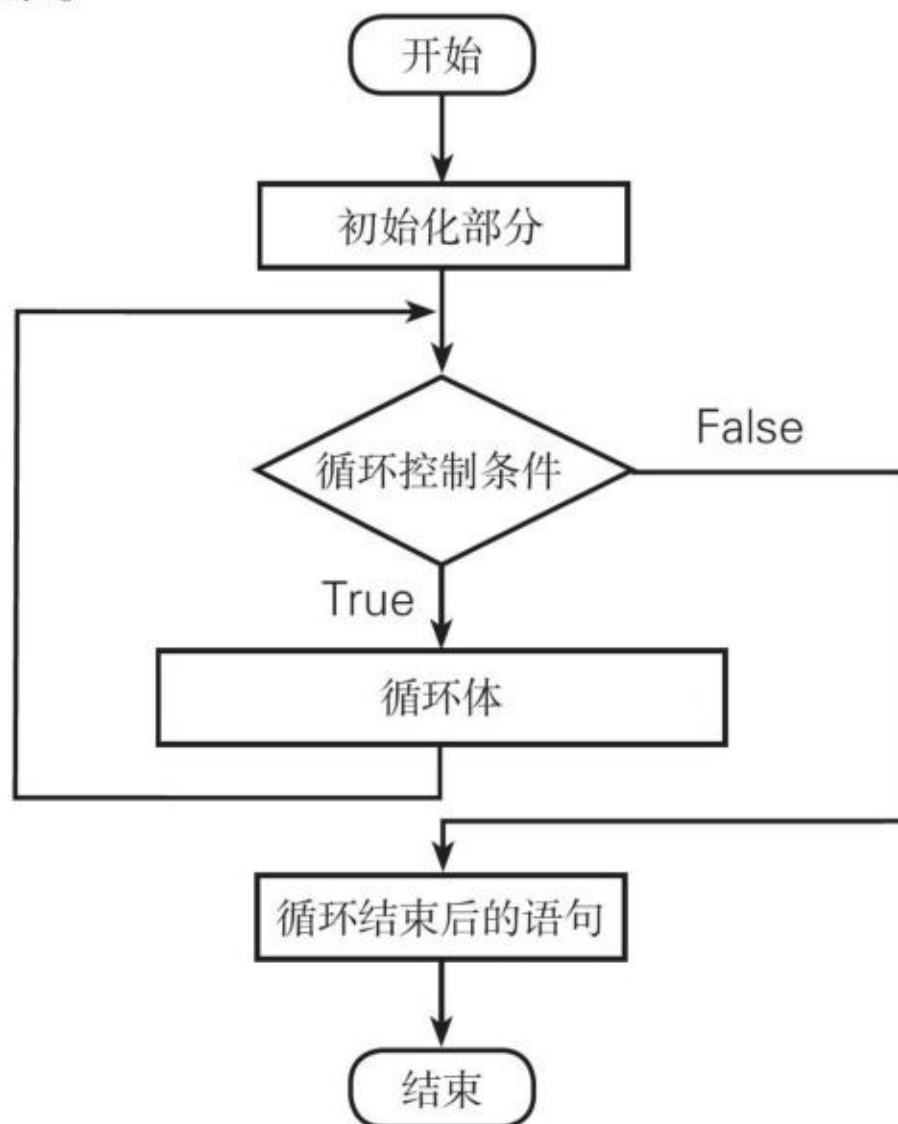
图2.3.5 循环结构流程图
