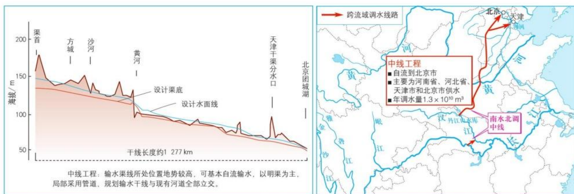
图3.1.2 南水北调中线工程示意
