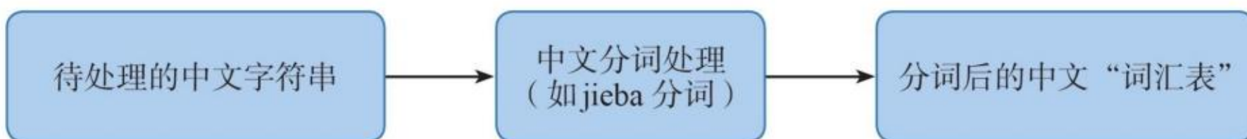
图 2.4.6 中文分词过程示意图
