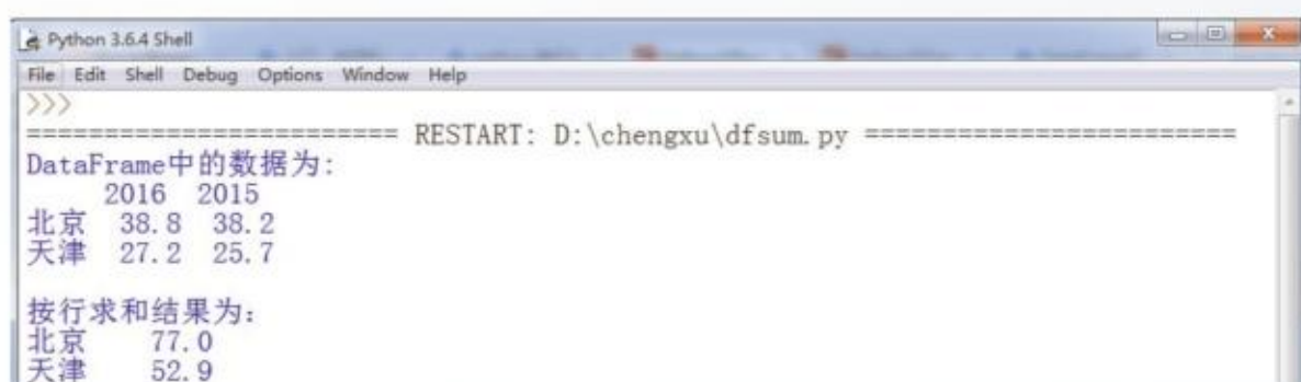
图 3.3.13 DataFrame 按行求和
