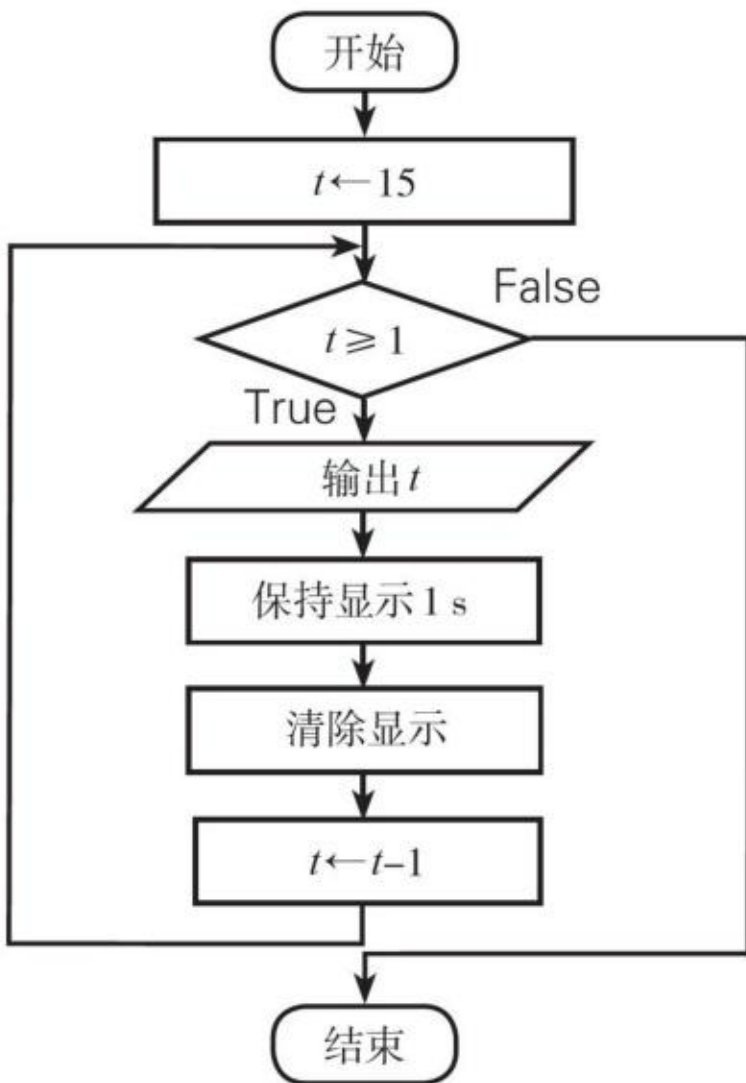
图 2.2.3 “倒计时 15 s”算法流程图
