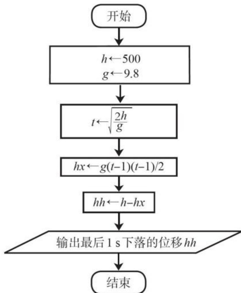
图2.4.2 自由落体运动问题求解流程图
