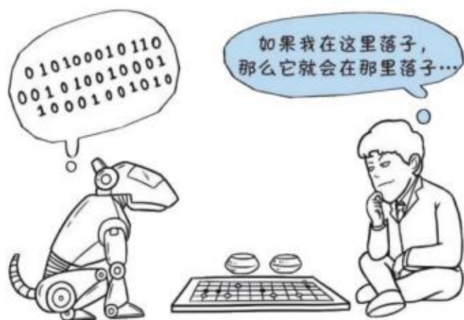
图4.1.1 人机博弈
