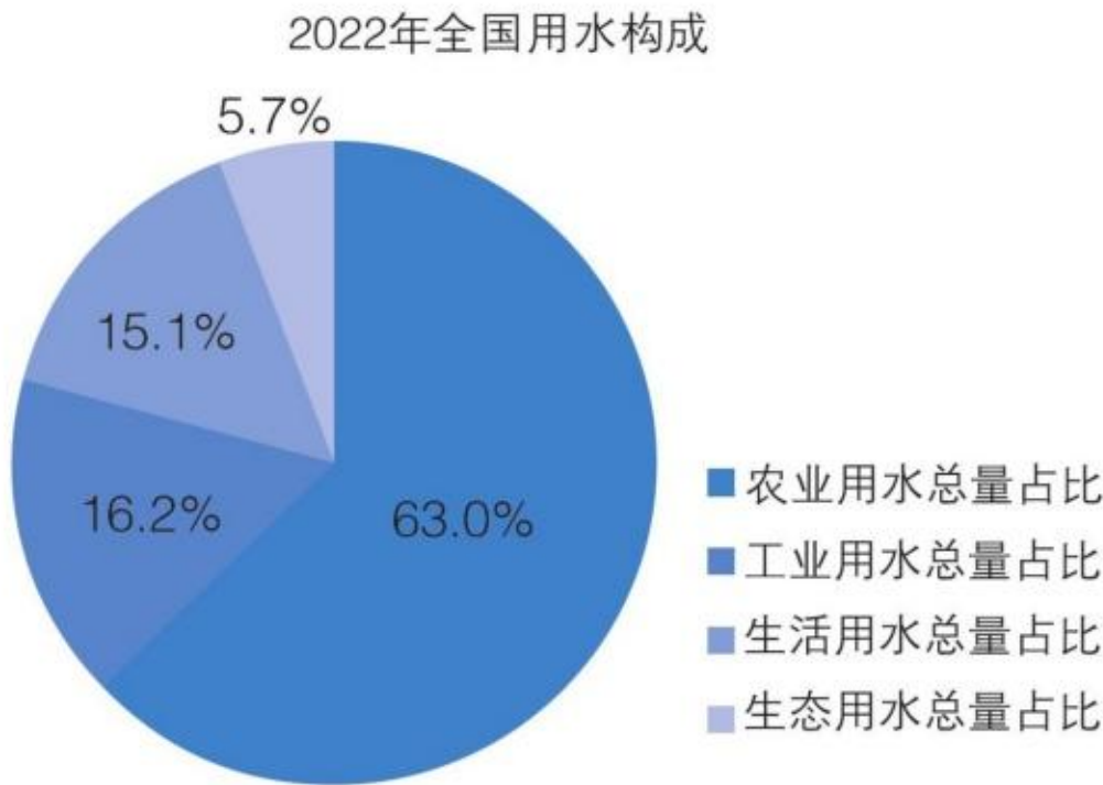
图3.3.19 饼图示例
