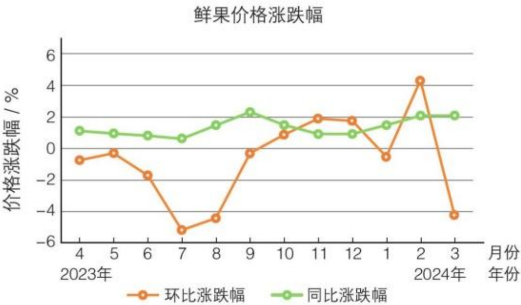
图3.3.17 折线图示例
