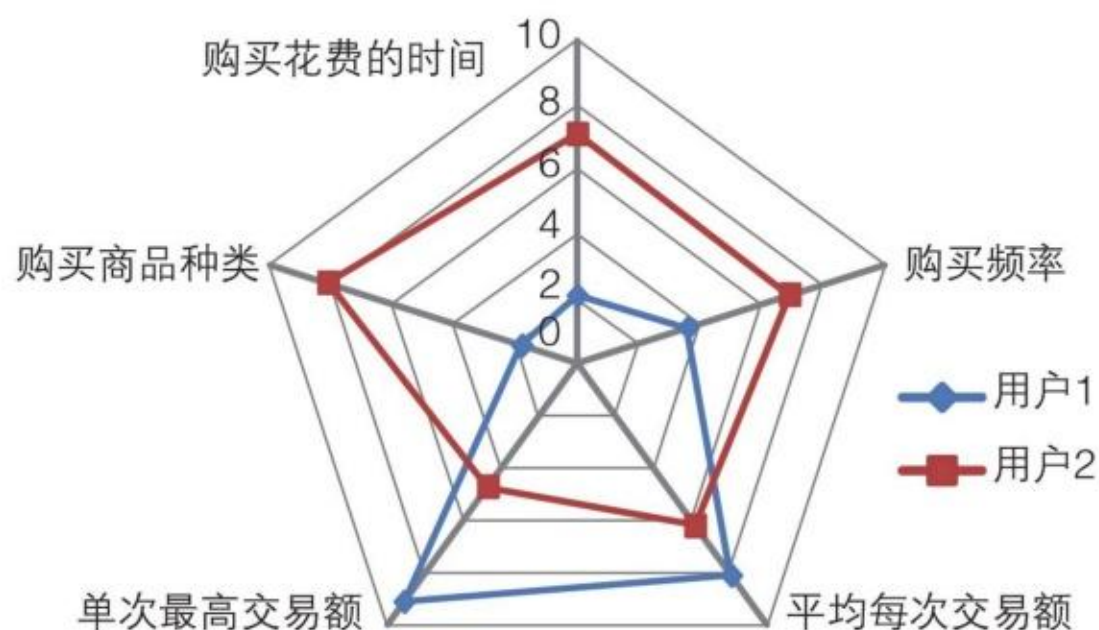
图3.3.21 雷达图示例
