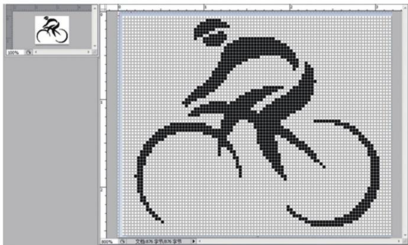
图 1.2.9 图像与像素
