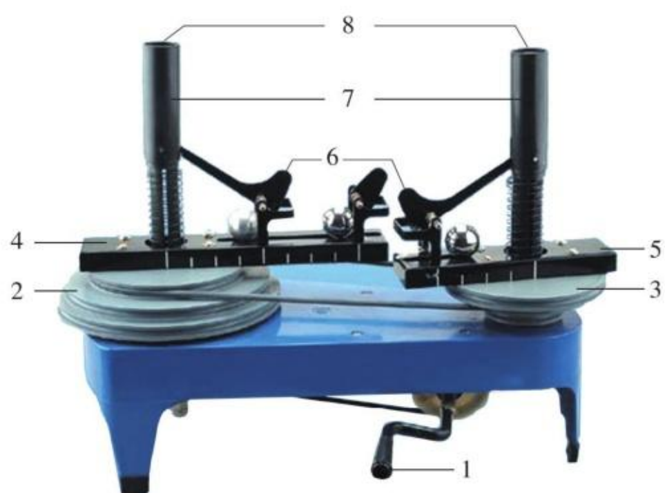
图 6.2-4 向心力演示器
