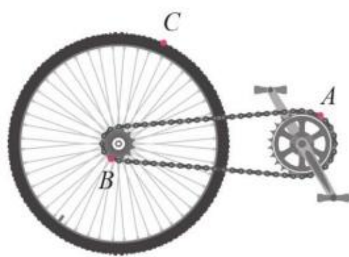
图6.3-2 自行车的大齿轮、小齿轮与后轮
