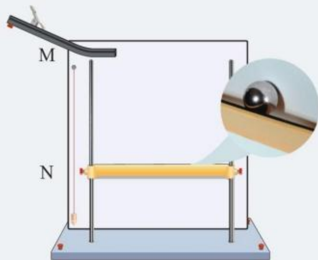
图 5.3-3 绘制小球做平抛运动的轨迹
