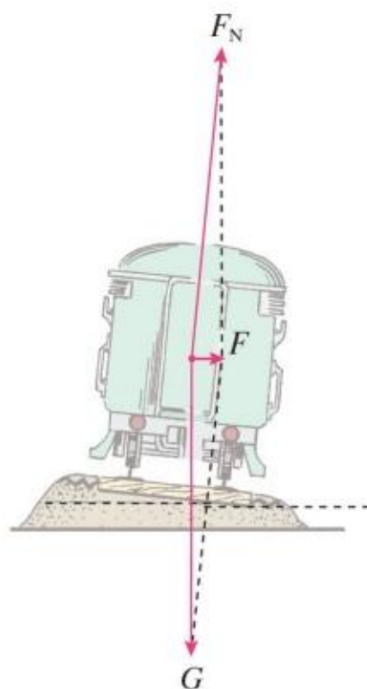
图6.4-3 重力 G 与支持力 F_N 的合力 F 提供了向心力
