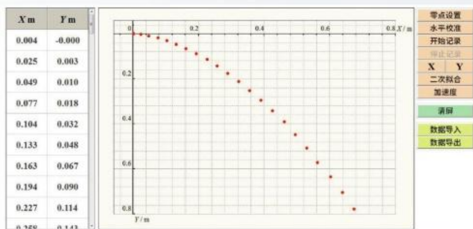
图5.3-6 计算机描绘的平抛运动的轨迹
