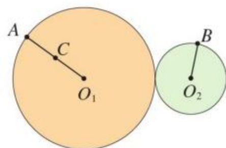
图 6.1-6
