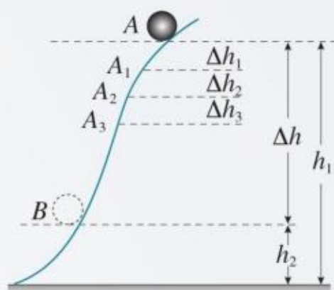
图 8.2-4 研究物体沿曲面运动时重力做的功
