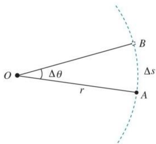
图 6.1-3 曲线运动的角速度
