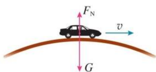
图 6.4-4 汽车通过拱形桥
