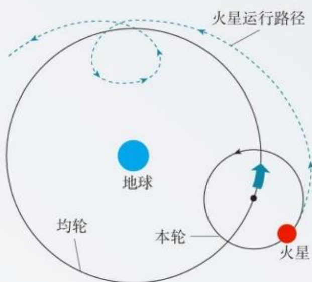
图 7.1-5 本轮和均轮
