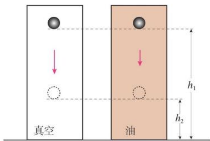
图8.4-2 小球在真空和油中的下落
