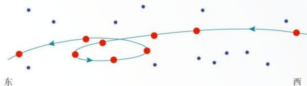
图 7.1-4 火星的逆行
