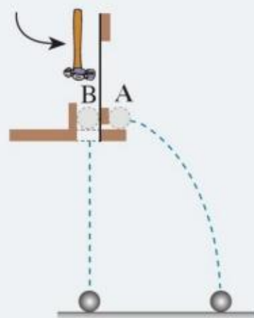
图 5.3-2 研究平抛运动的竖直分运动
