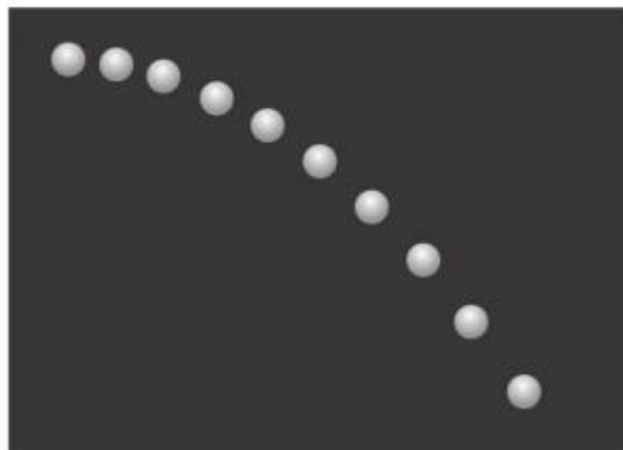
图5.3-1 小球做平抛运动的频闪照片
