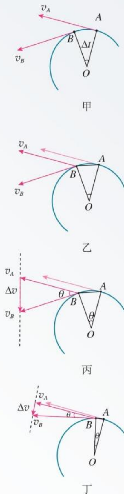
图 6.3-4 推导向心加速度公式
