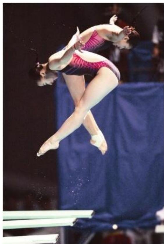
图8.4-1 跳板跳水
