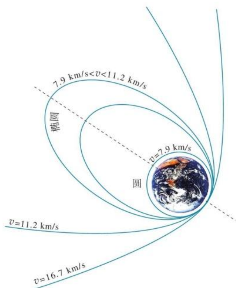
图 7.4-1 三个宇宙速度
