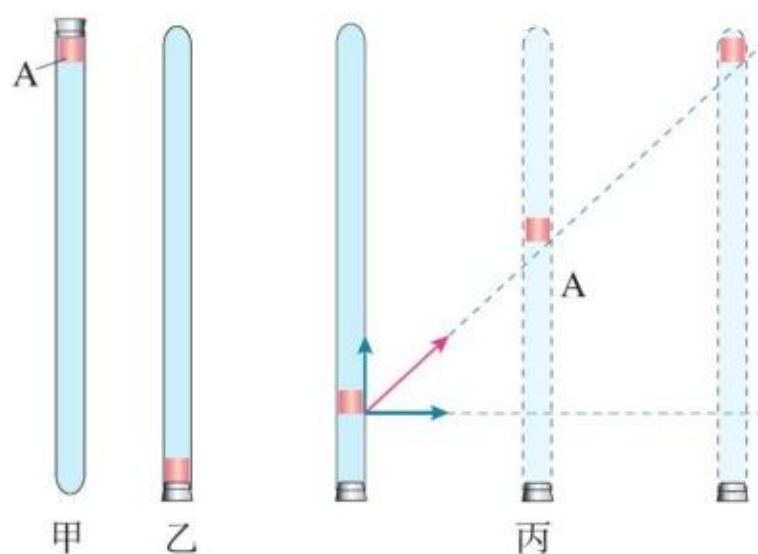
图 5.2-1 蜡块的运动
