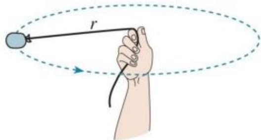
图 6.2-3 感受向心力
