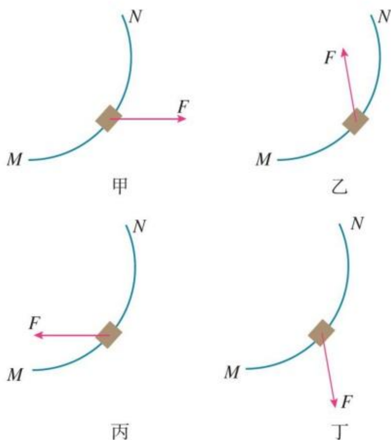
图 6.2-10
