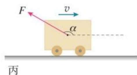
人的拉力做负功 ( \frac{\pi}{2} < \alpha \leq \pi )
