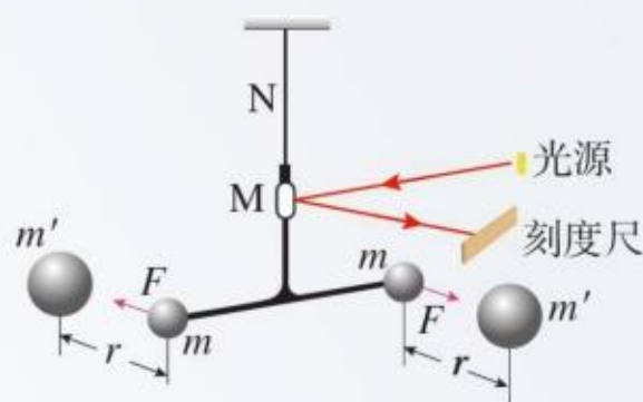
图7.2-3 卡文迪什实验示意图
