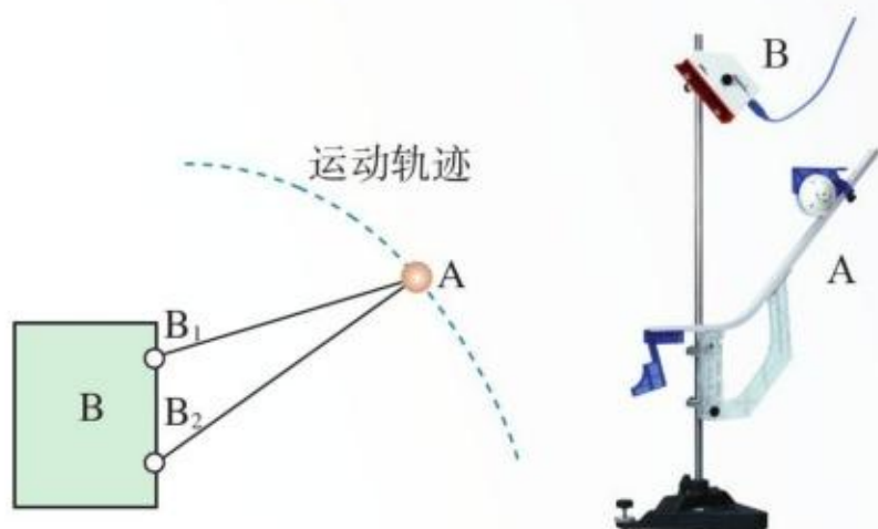
图5.3-4 用传感器研究平抛运动的原理图
