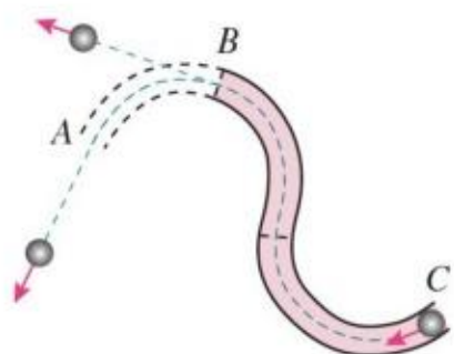
图 5.1-1 钢球离开轨道时速度的方向
