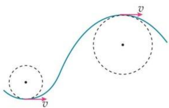
图 6.2-6 一般曲线运动的研究方法
