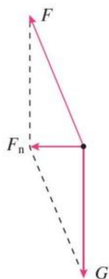
图 6.2-2 飞椅与人受到的力
