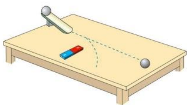
图 5.1-3 钢球的运动轨迹
