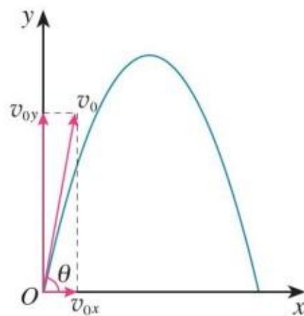
图 5.4-5 斜抛物体的轨迹
