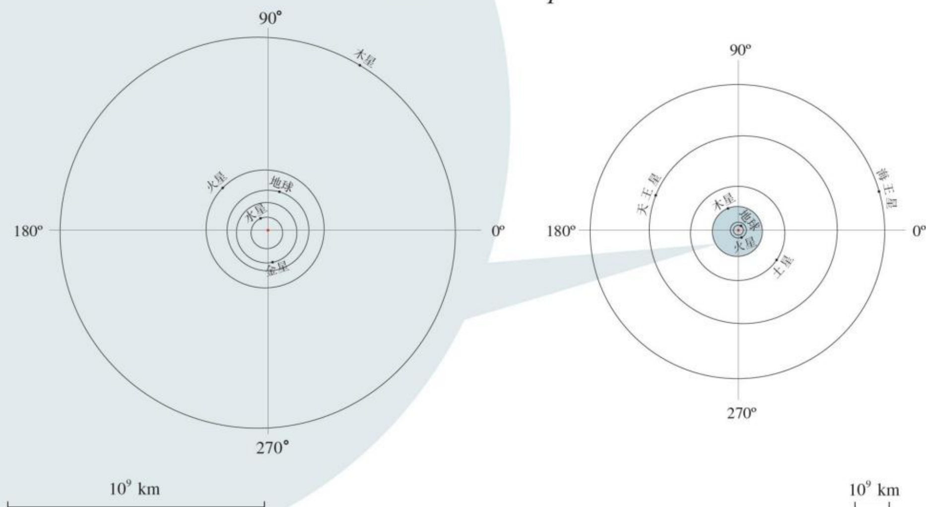
图 7.1-3 太阳系八颗行星的轨道示意图
