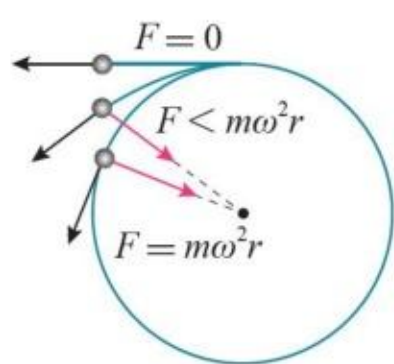
图 6.4-7 物体的离心运动与受力情况
