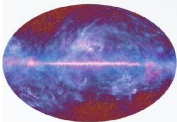
图 7.5-2 普朗克探测器记录下的微波天空
