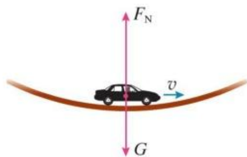
图 6.4-5 汽车通过凹形路面
