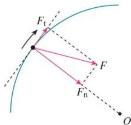
图 6.2-5 做变速圆周运动的沙袋所受的力
