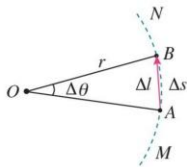
图 6.1-1 曲线运动的线速度
