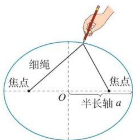
图 7.1-1 用图钉和细绳画椭圆
