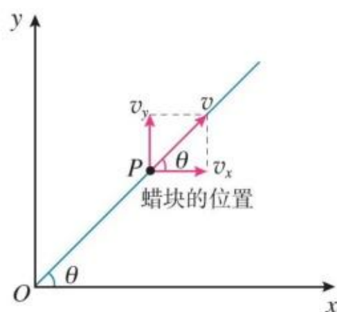
图 5.2-2 研究蜡块的运动
