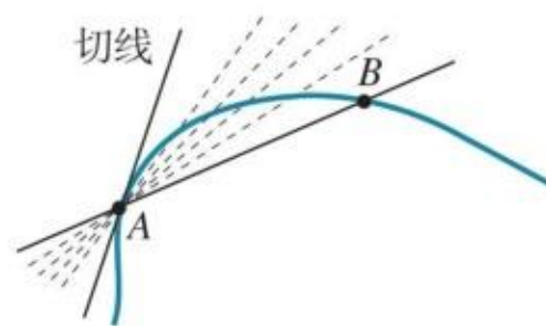
图 5.1-2 曲线的切线
