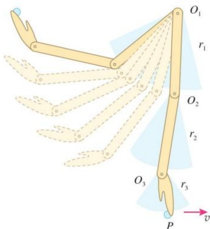
图研-2 甩手过程分析图
