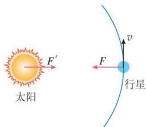
图 7.2-1 太阳与行星间的引力
