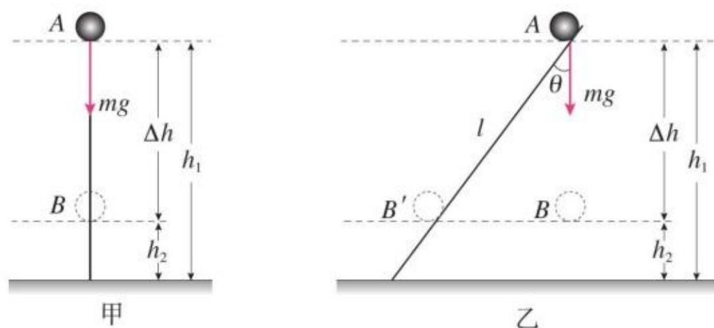
图 8.2-1 研究物体运动时重力做的功
