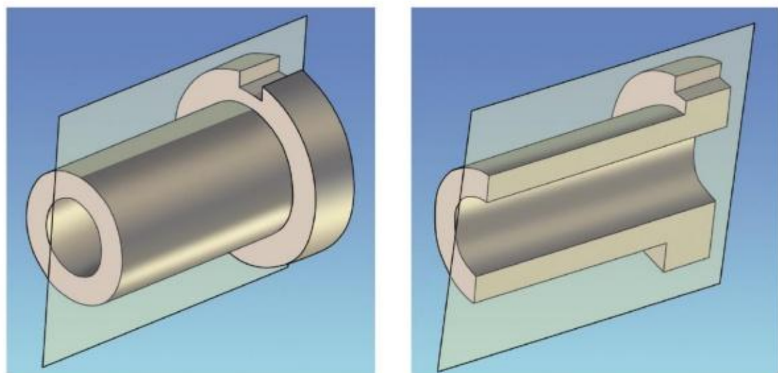
图2-60 剖视图形成过程
