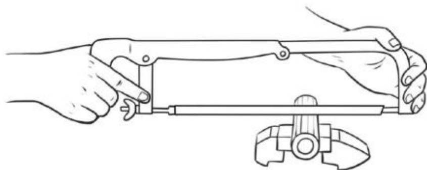
图3-27 握锯姿势
