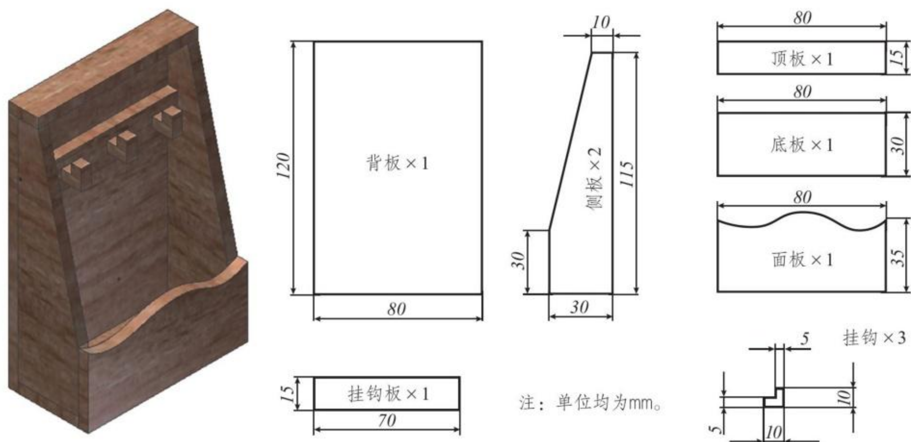
图 3-11 钥匙收纳盒
