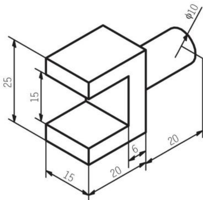
图2-68 物件形体图
