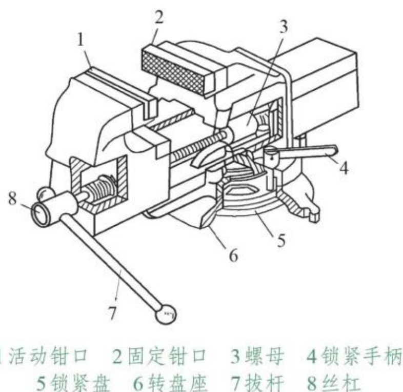
图 3-20 台虎钳构造图
