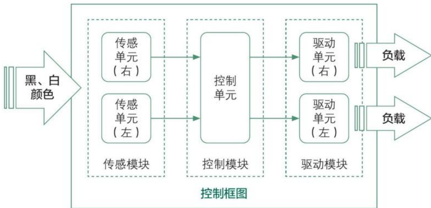
图3-59 循迹小车电路控制板
