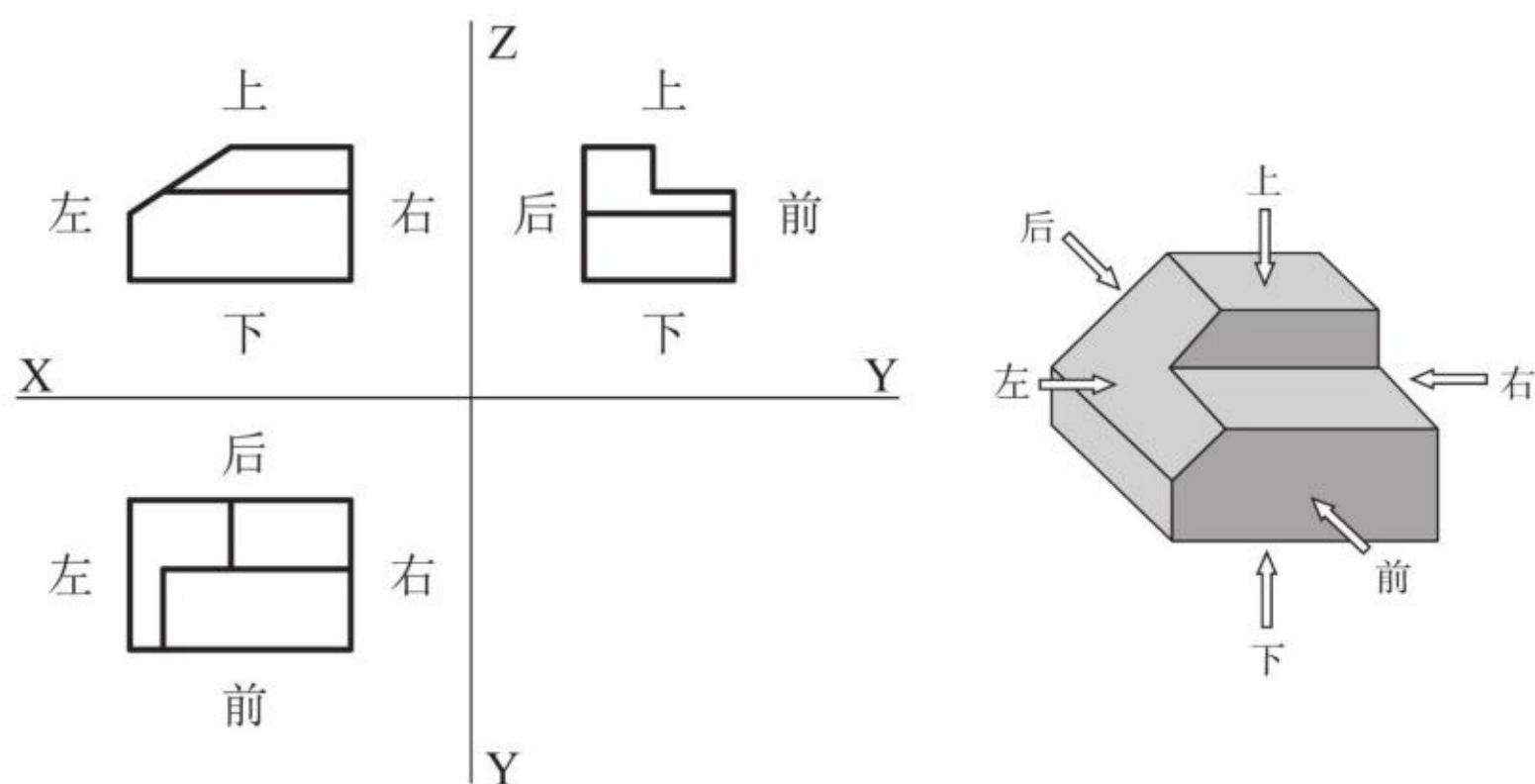
图2-48 平面图中的空间方位体现
