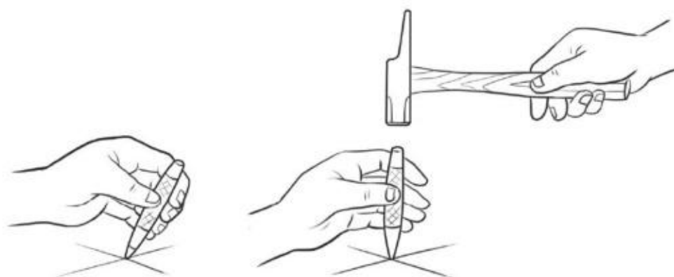
图3-17 样冲的用法
