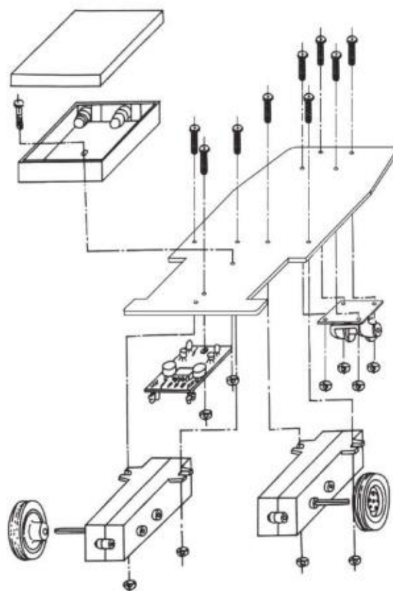
图3-57 循迹小车装配示意图
