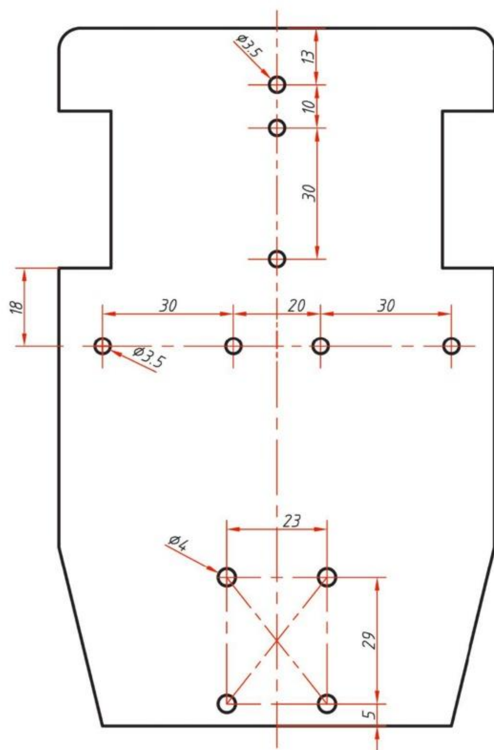
图2-75 循迹小车底板圆孔绘制图
