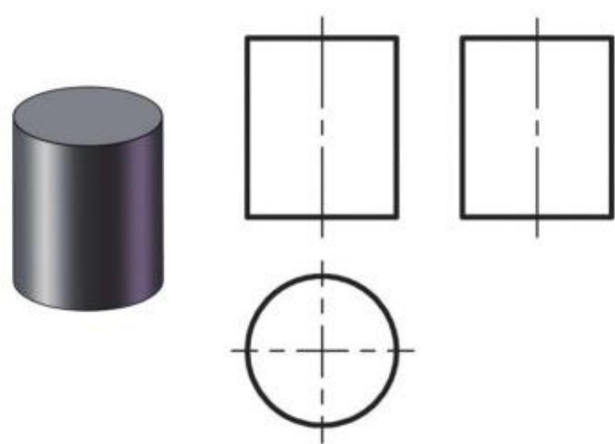
图2-51 直立圆柱体三视图
