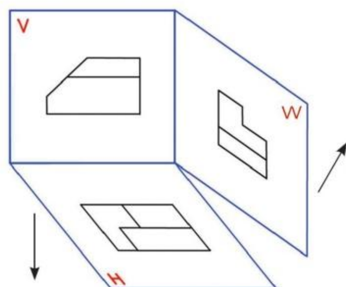
图2-47 三视图的平面展开
