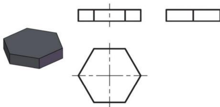
图2-52 平放六棱柱三视图
