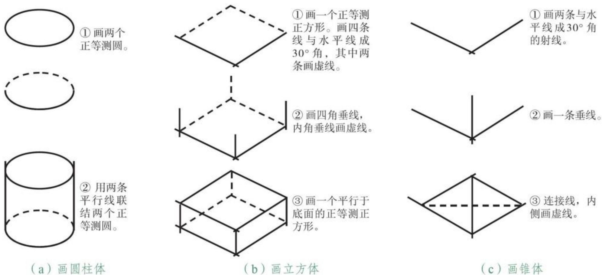
图2-40 基本立体图形的绘制
