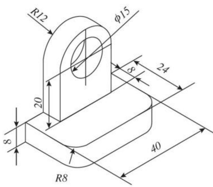
图2-55 物件形体图2
