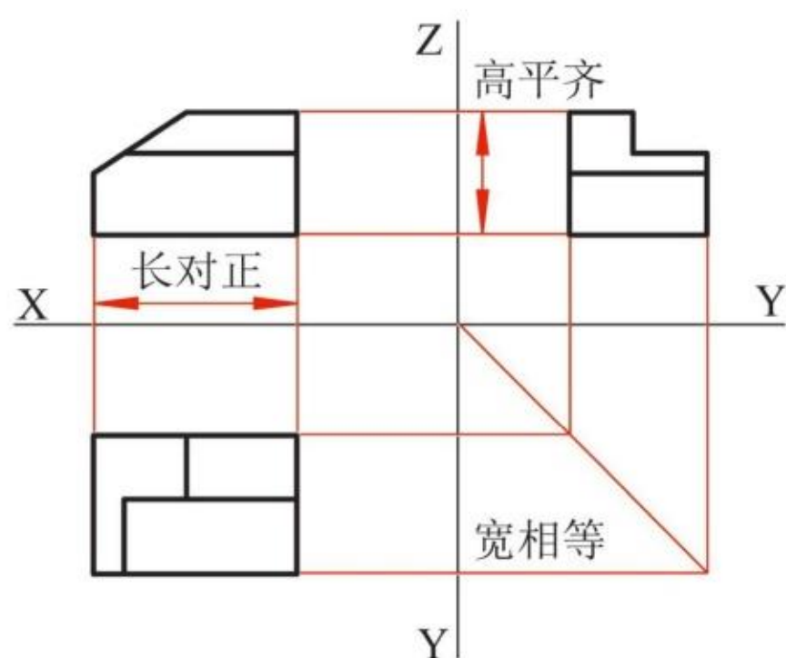
图 2-49 三视图投影规律
