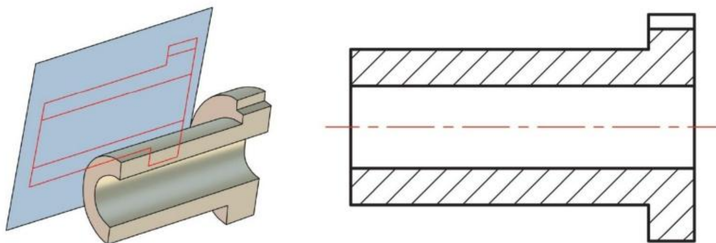
图2-61 剖视图
