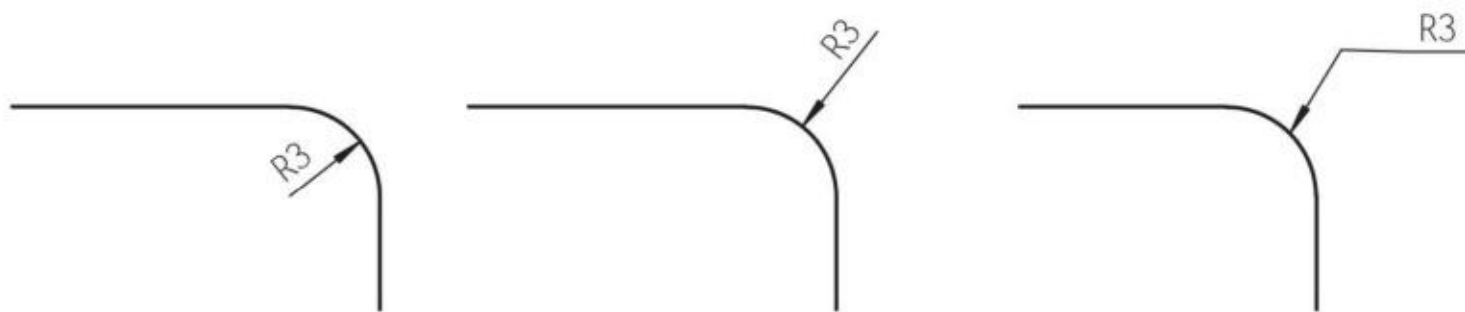
图2-65 半径标注
