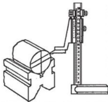
(d) 立体划线
