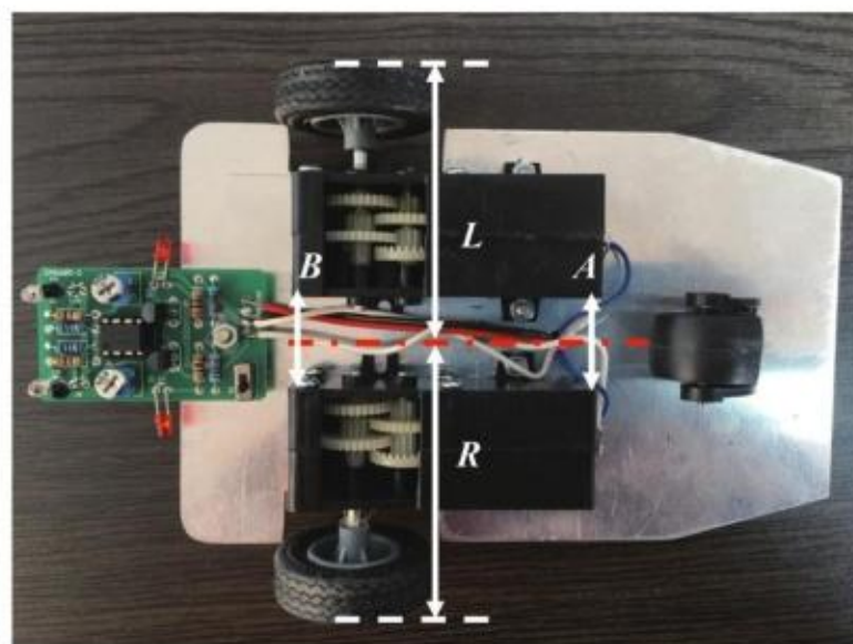
图4-11 循迹小车反面结构图
