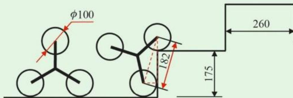
图 2-5 车轮示意图
