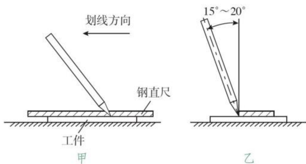
图3-16 针尖位置
