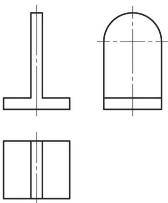
图2-57 组合体三视图
