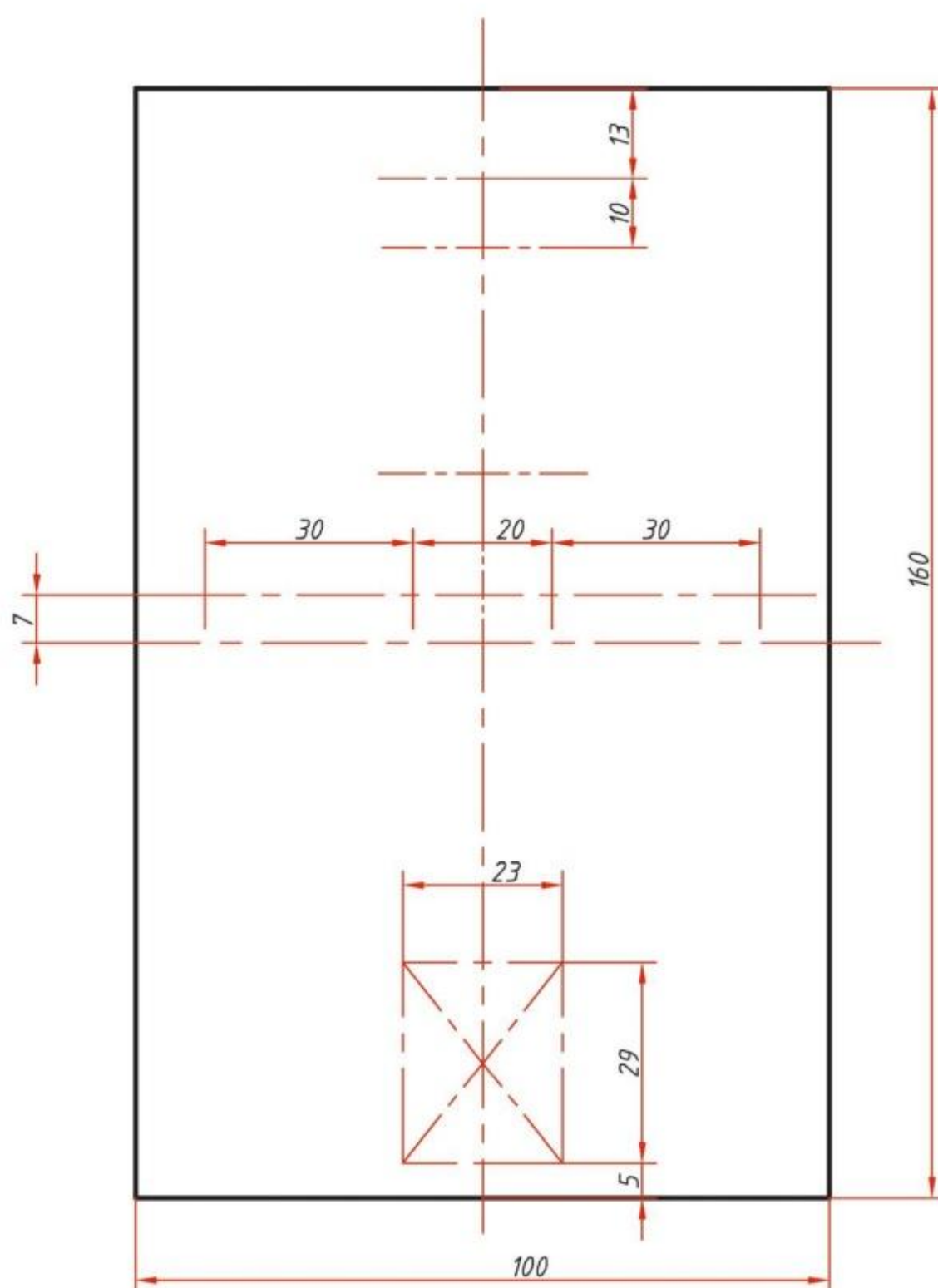
图 2-71 循迹小车底板中心线
