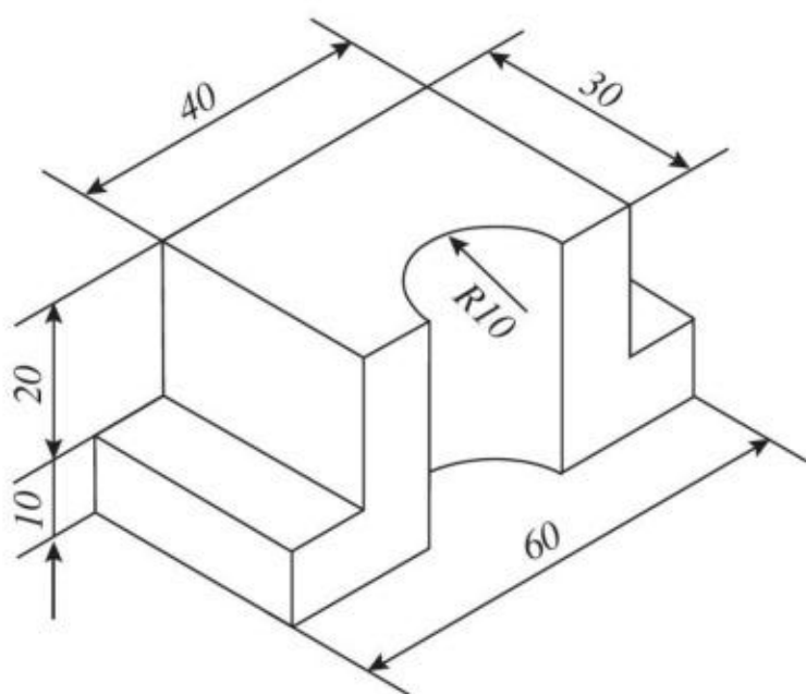
图2-54 物件形体图1
