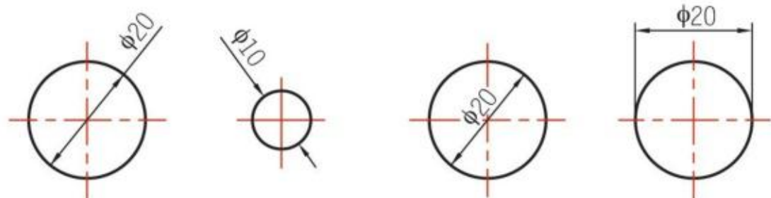
图2-66 直径标注
