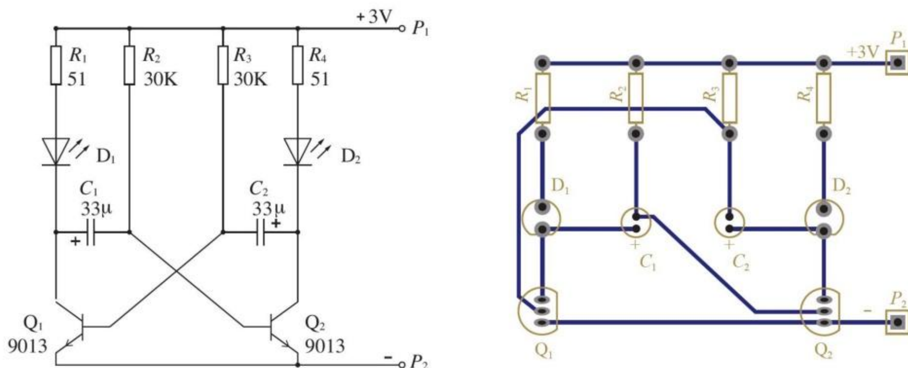
图3-51 简易双闪灯电路
