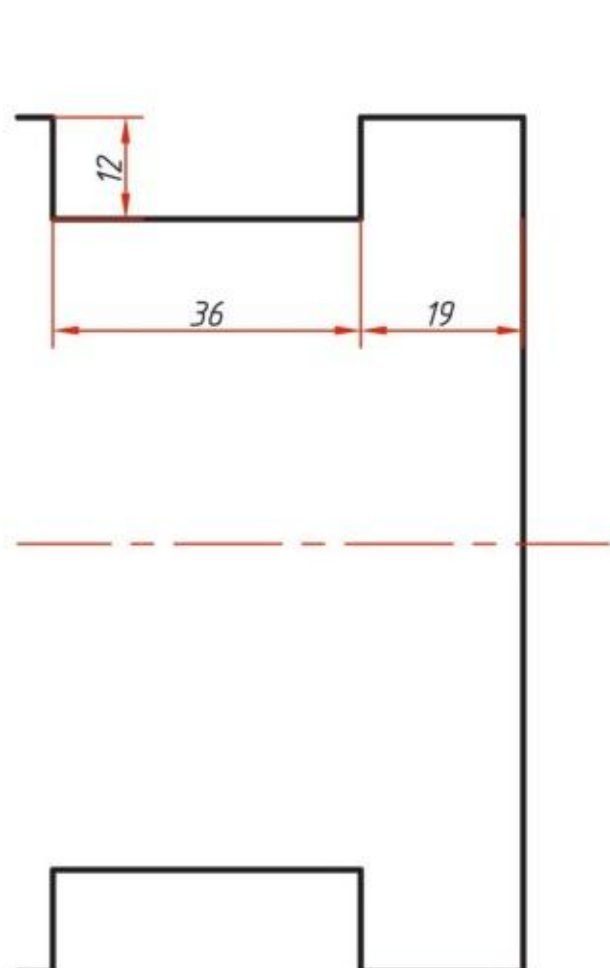
图 2-72 循迹小车底板左右侧缺口
