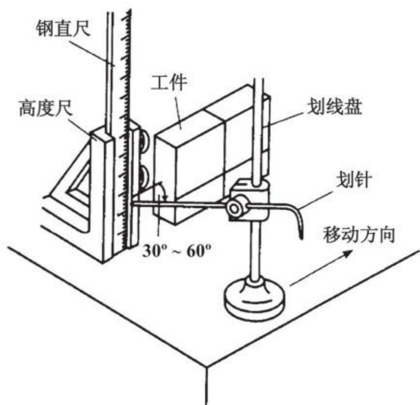
图3-14 划线盘和工件安放
