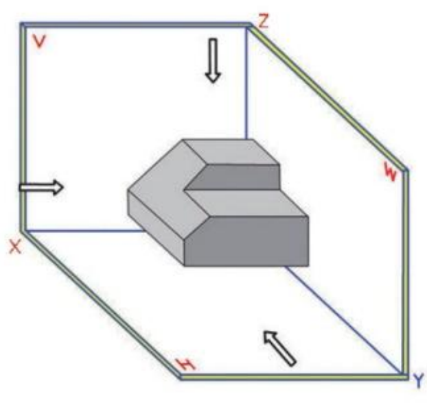
图2-46 第 I 视角内的三视图
