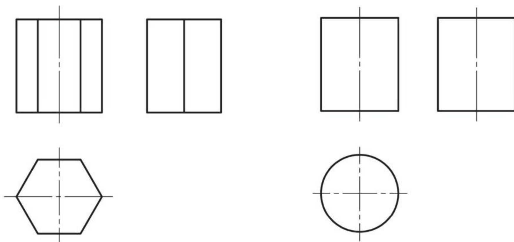
图2-56 六棱柱和圆柱体的三视图
