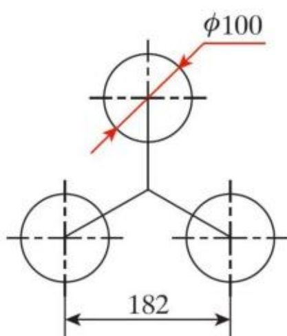
图 2-6 草图
