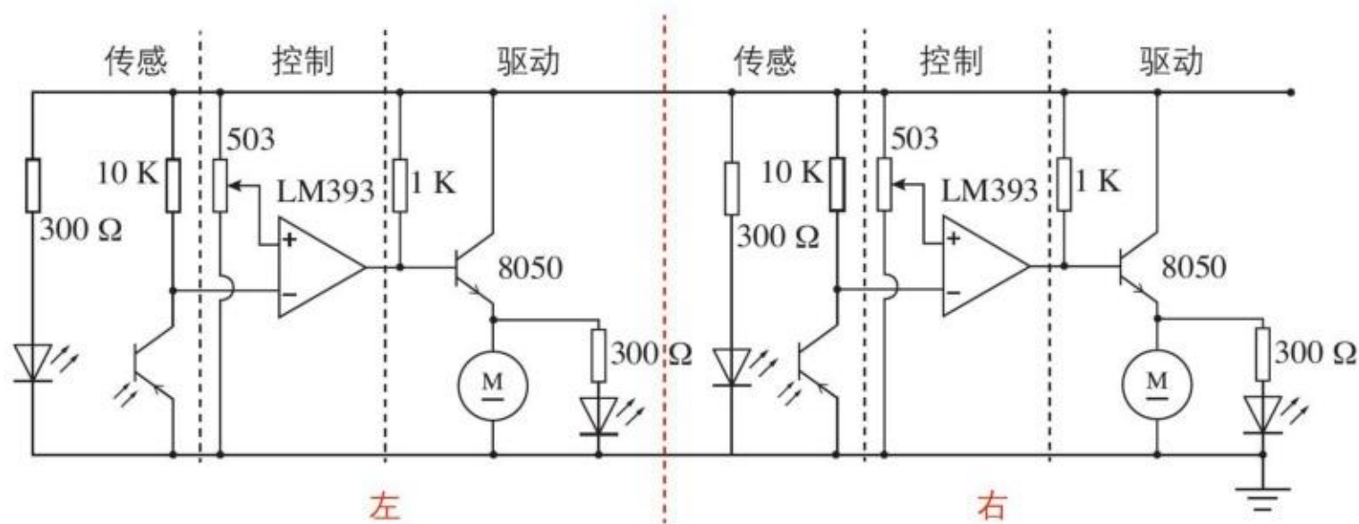
图 2-35 循迹小车电路原理图
