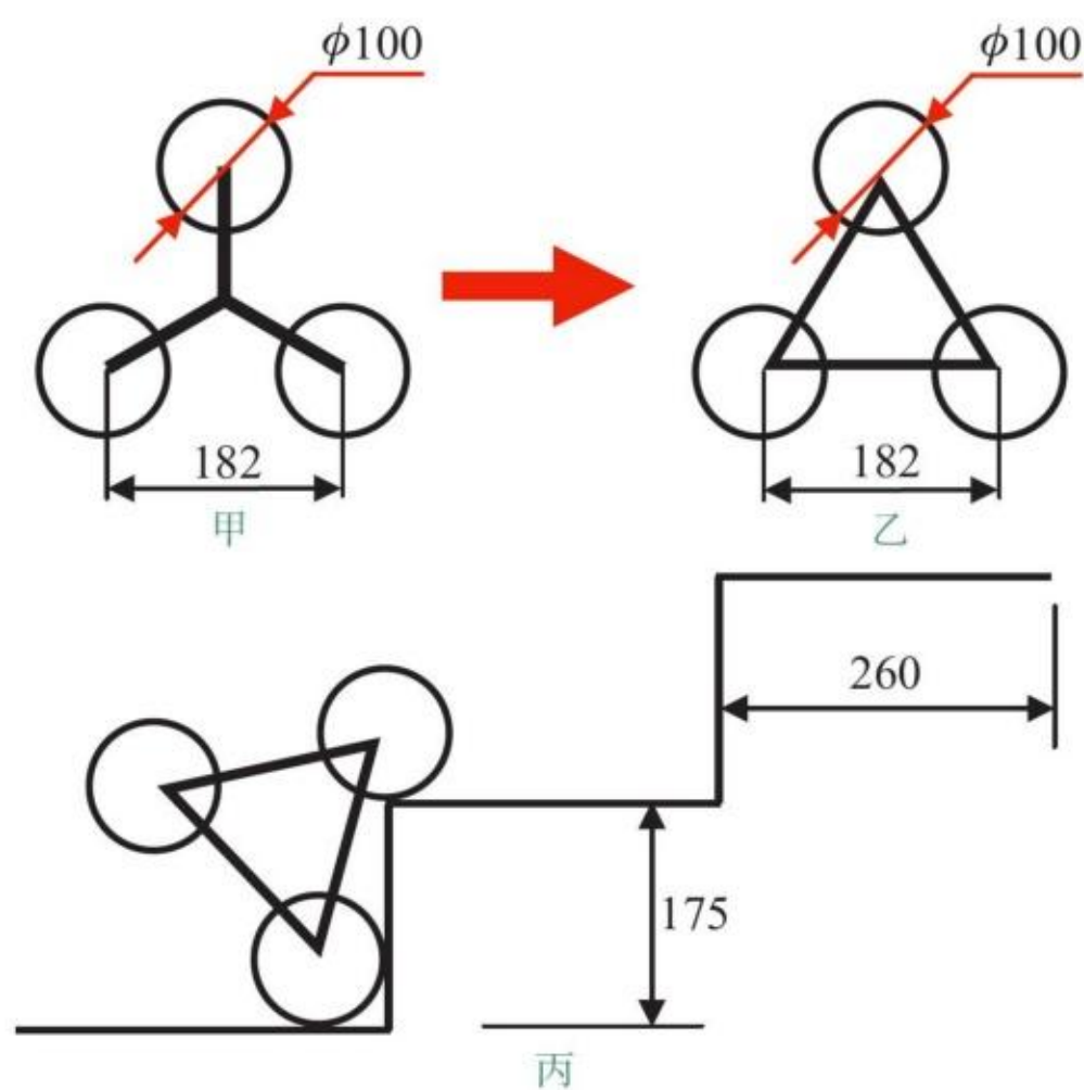
图2-29 完善构思方案
