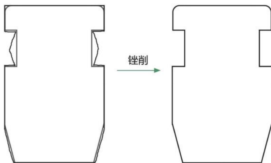
图3-36 循迹小车底板的锉削操作
