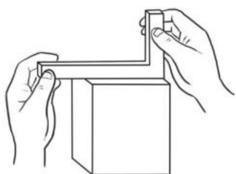
平直度检查
