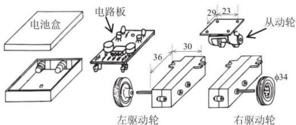
图2-12 循迹小车底板安装部件
