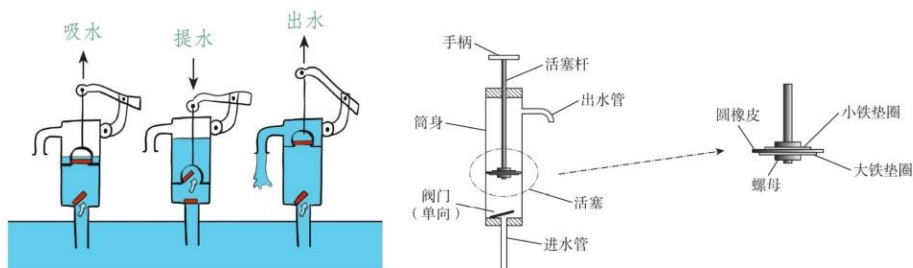
图1-16 活塞式抽水机
