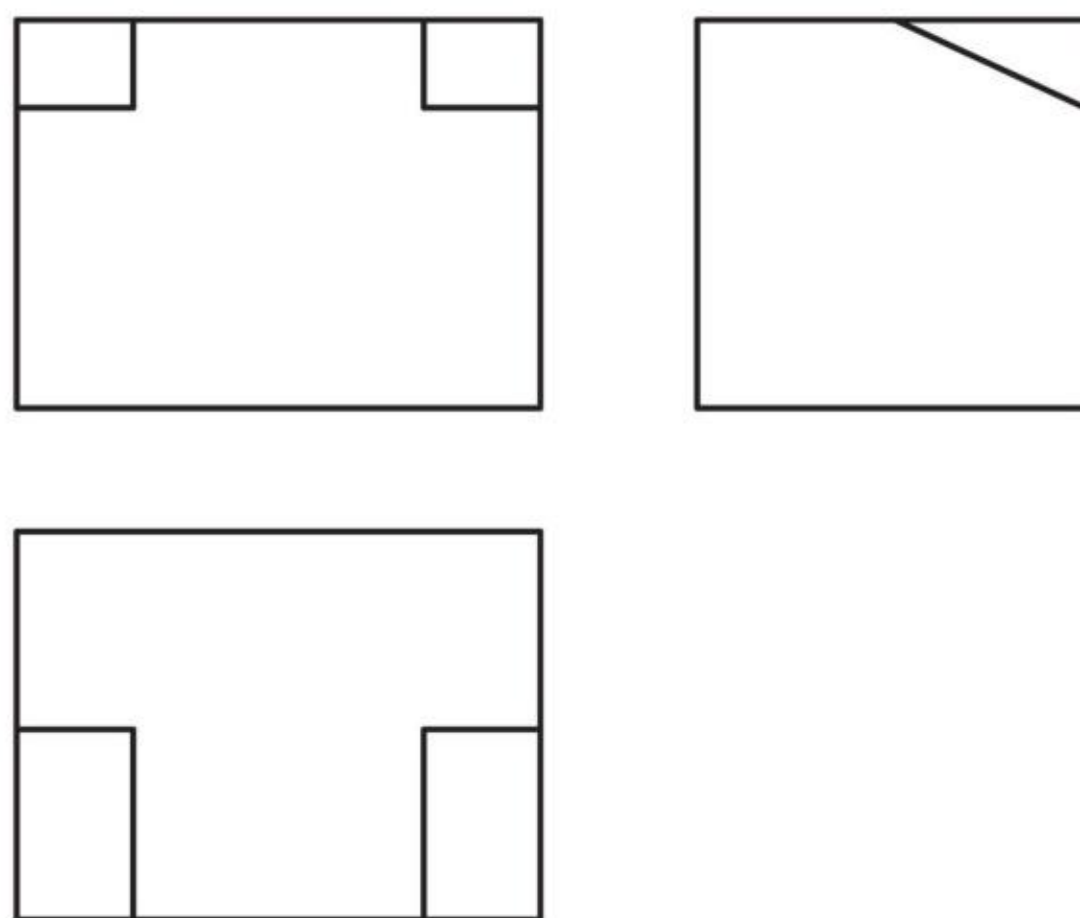
图2-59 三视图
