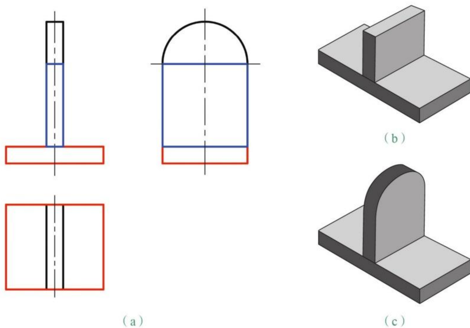
图2-58 识读三视图
