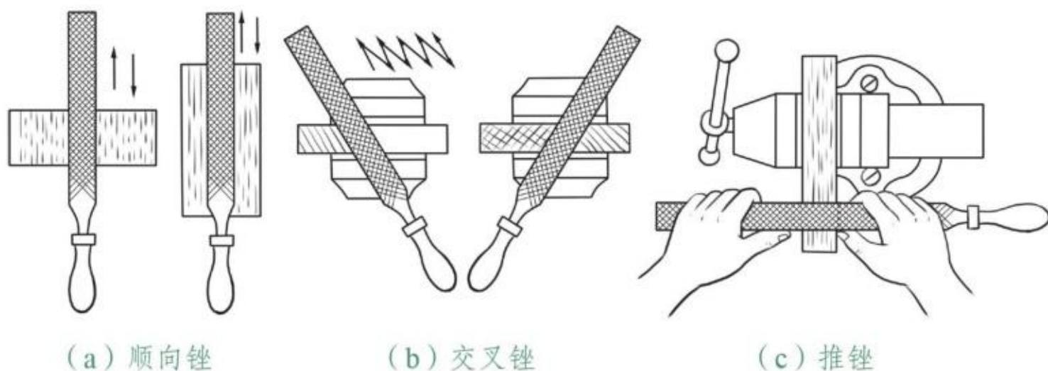
图3-33 平面锉削的方法
