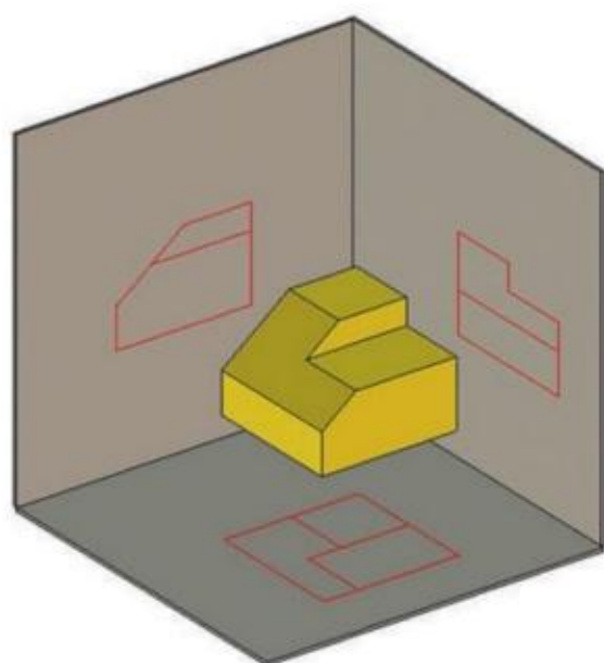
图2-46 第 I 视角内的三视图
