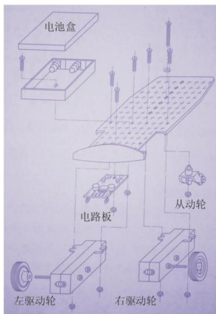
图2-37 循迹小车装配示意图
