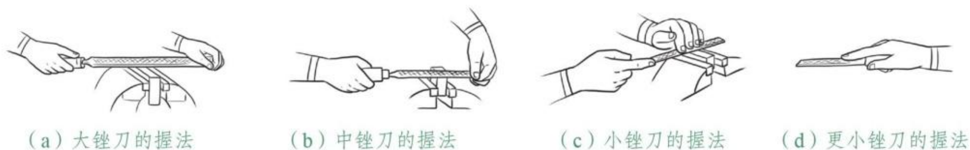
图3-31 锉刀的握法
