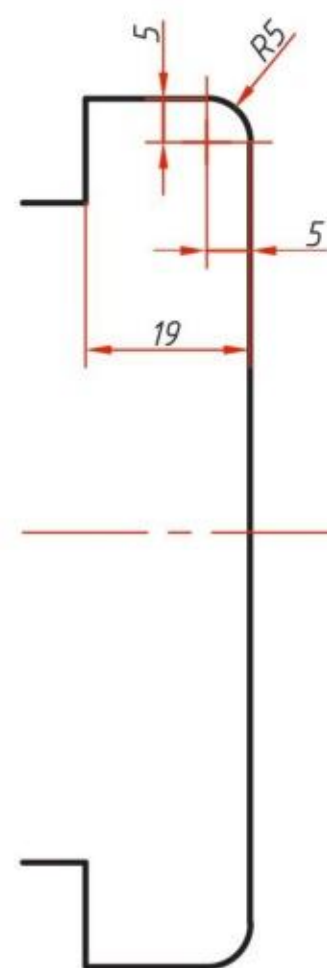
图 2-73 循迹小车底板左右上侧圆角
