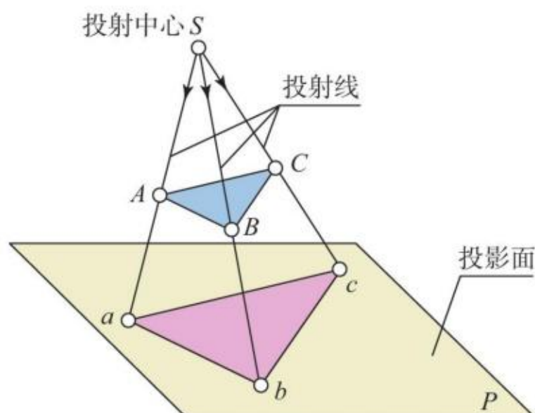
图 2-44 中心投影法示意图
