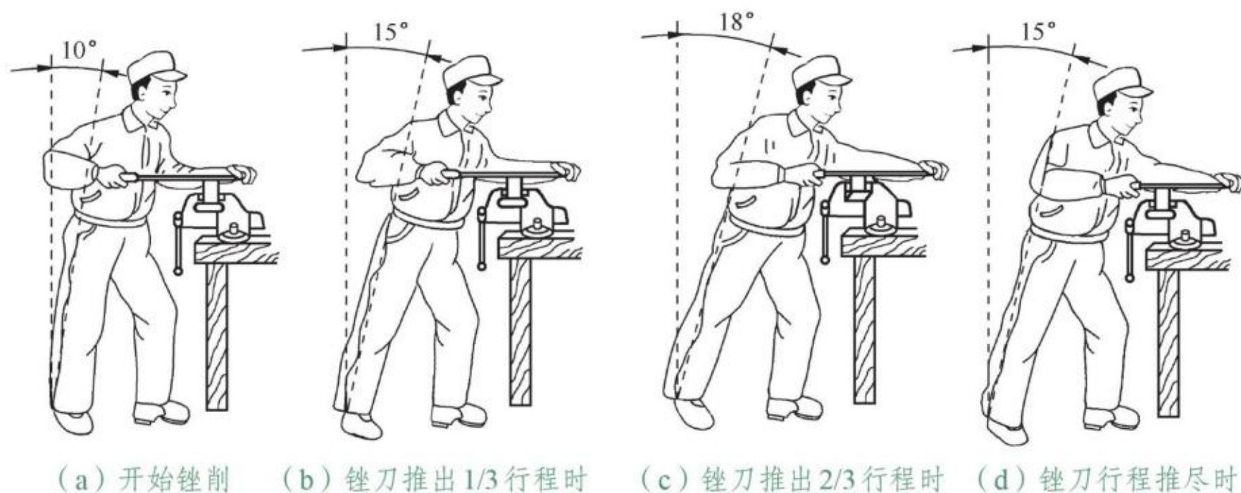
图3-32 锉削过程身体的姿势
