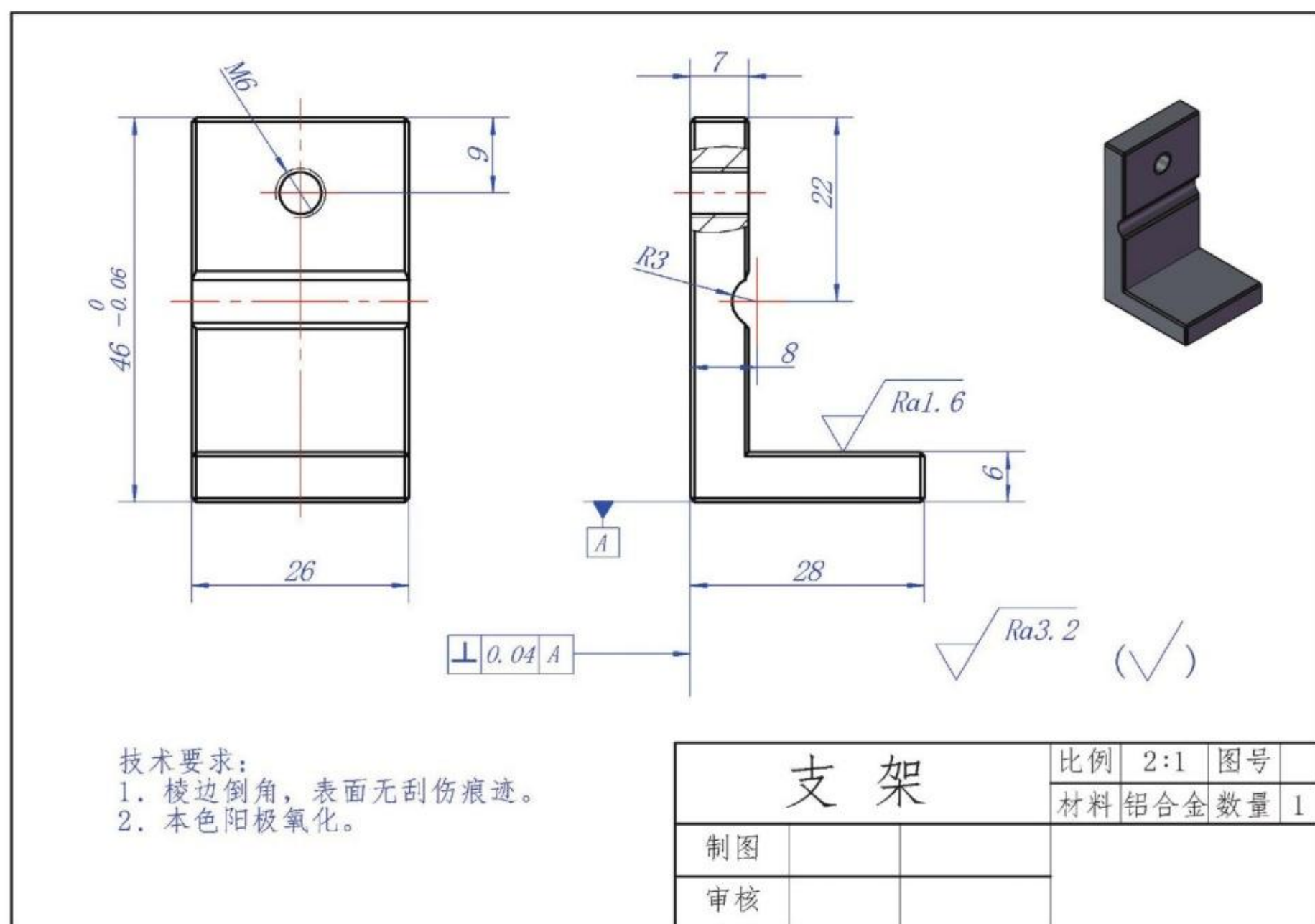
图2-34 支架零件图
