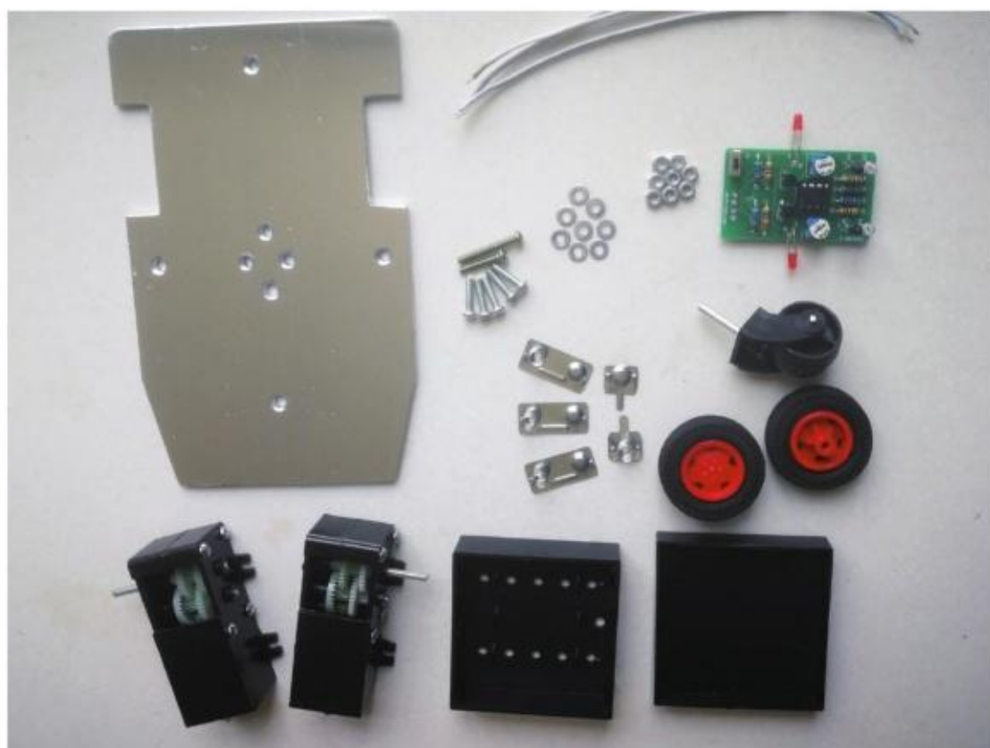
图3-56 循迹小车零件
