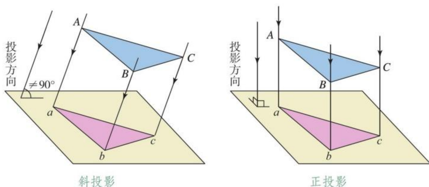
图2-45 平行投影法示意图
