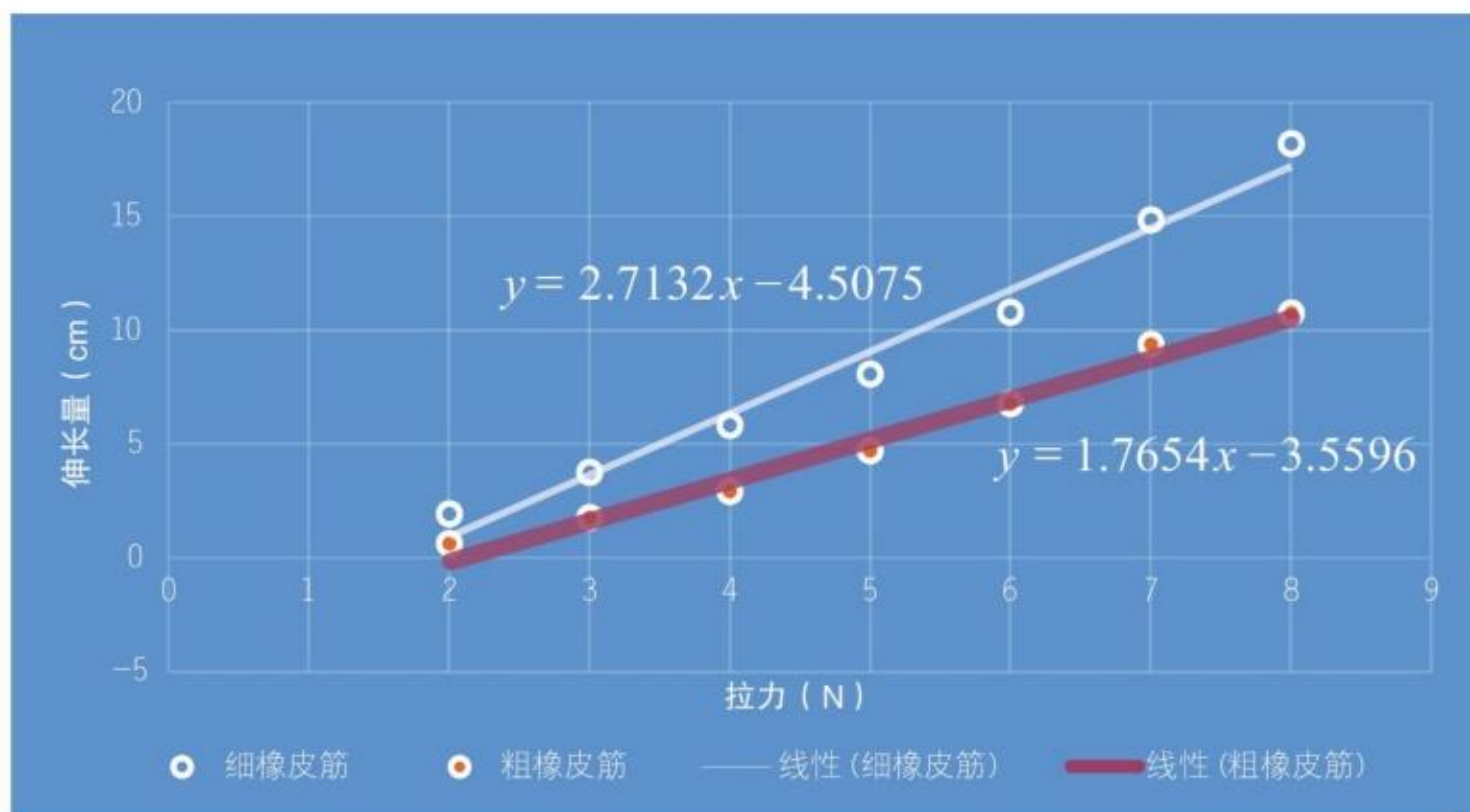
图4-13 不同粗细橡皮筋伸长量与拉力关系
