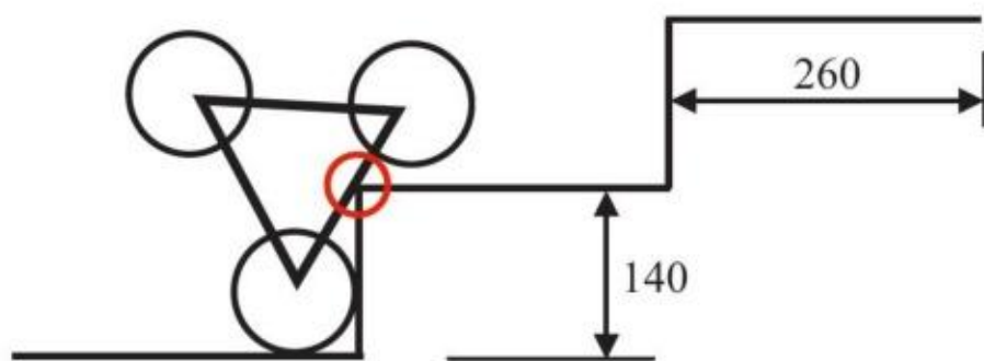
图2-30 车轮设计需要改进
