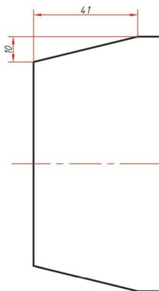
图2-74 循迹小车底板左右下角约束
