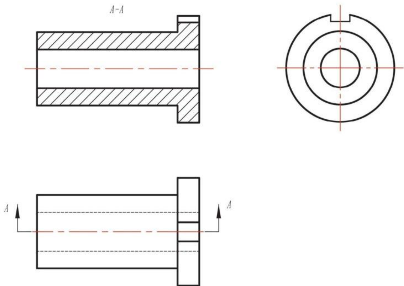
图2-62 零件剖视图
