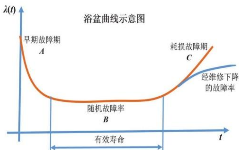
图4-19 典型故障曲线（浴盆曲线）示意图
