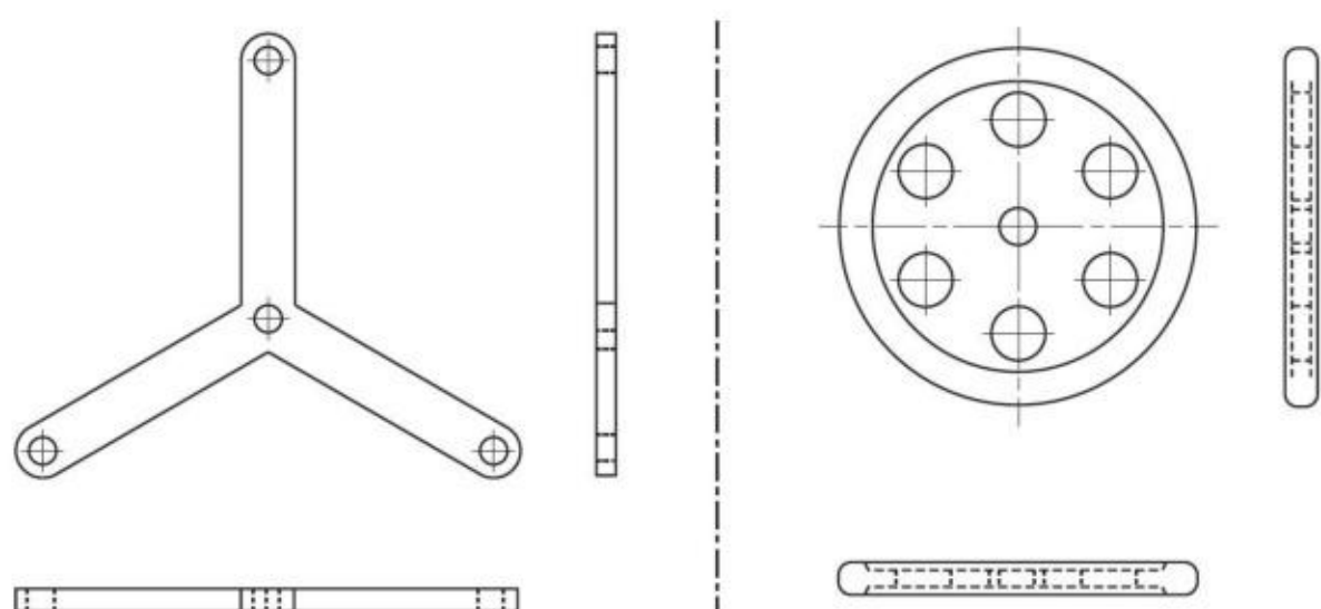
图2-7 计算机辅助绘制的支架和轮子三视图
