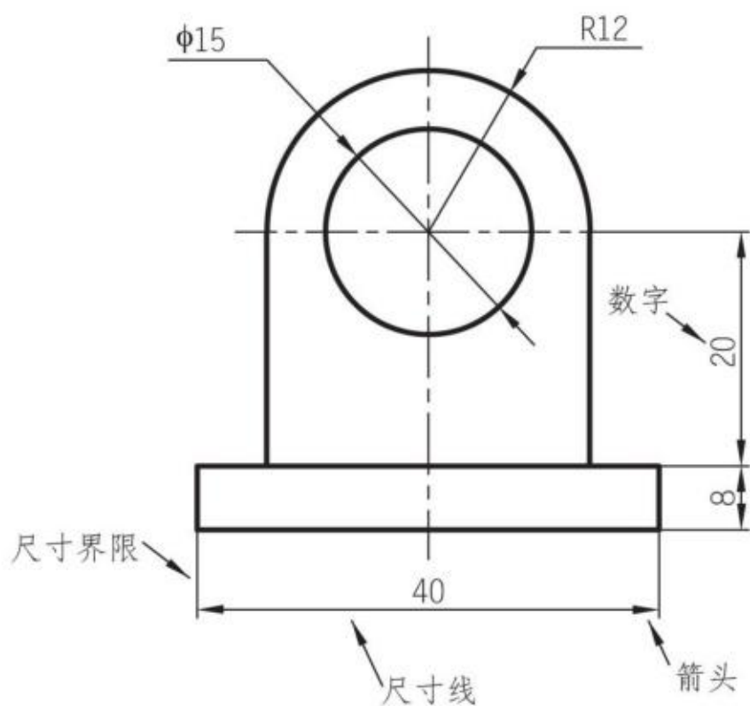
图2-63 尺寸标注
