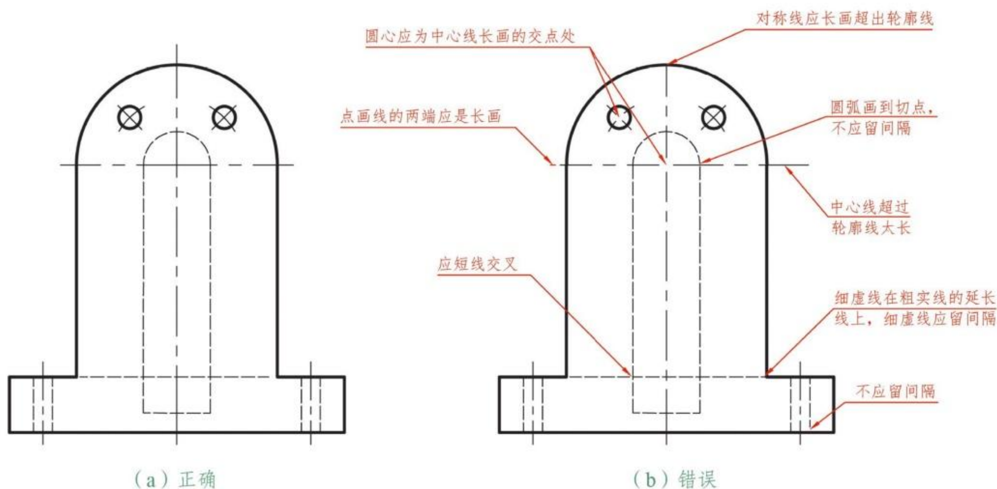
图2-50 图线画法正误对比示例
