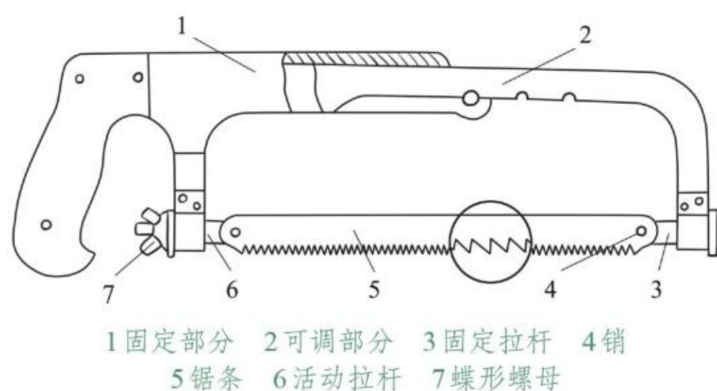
图3-21 可调锯弓式手锯
