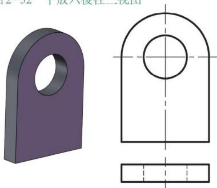
图2-53 组合体视图
