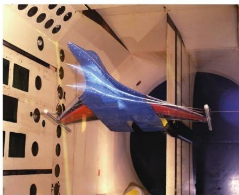
图2-16 飞机风洞试验
