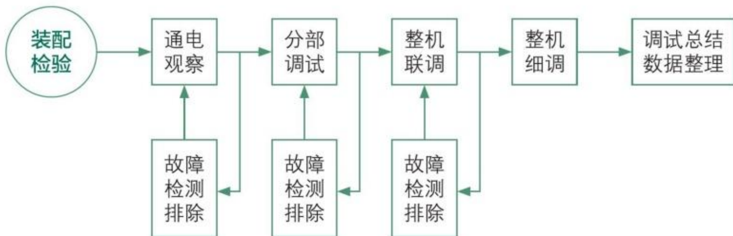
图3-58 样机的整机调试过程
