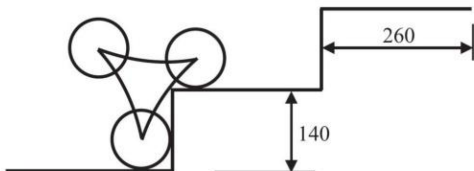
图2-31 改进设计后的车轮
