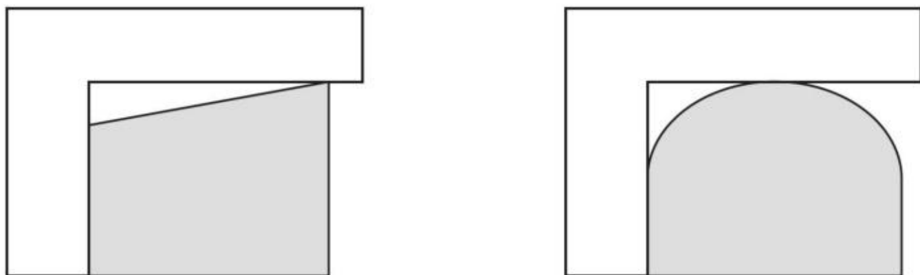
图3-35 不合格锉面
