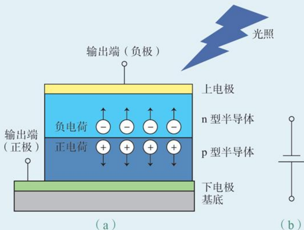
图2-22 太阳能电池结构和等效电路示意图
