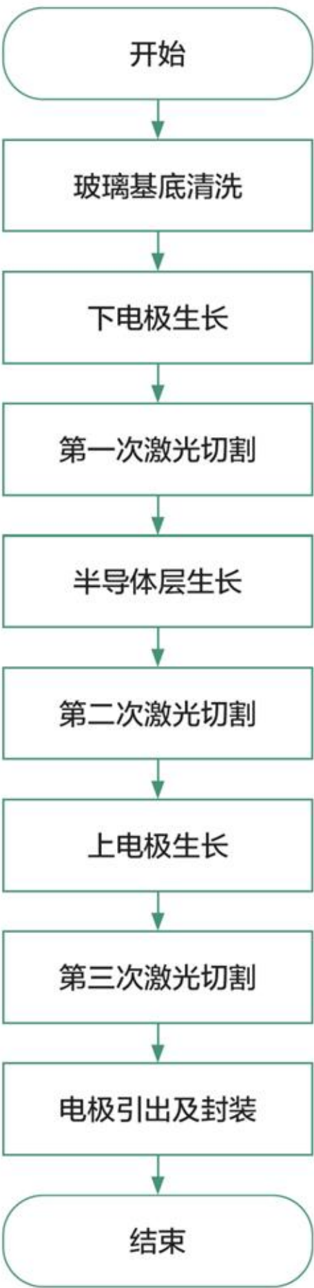
图2-24 多片串联太阳能电池板生产流程图
