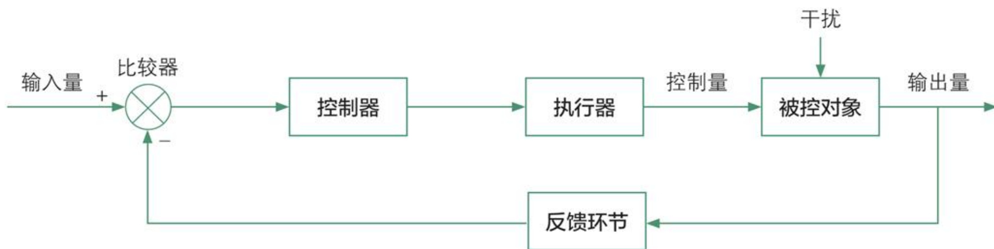
图4-18 闭环控制系统的干扰情况
