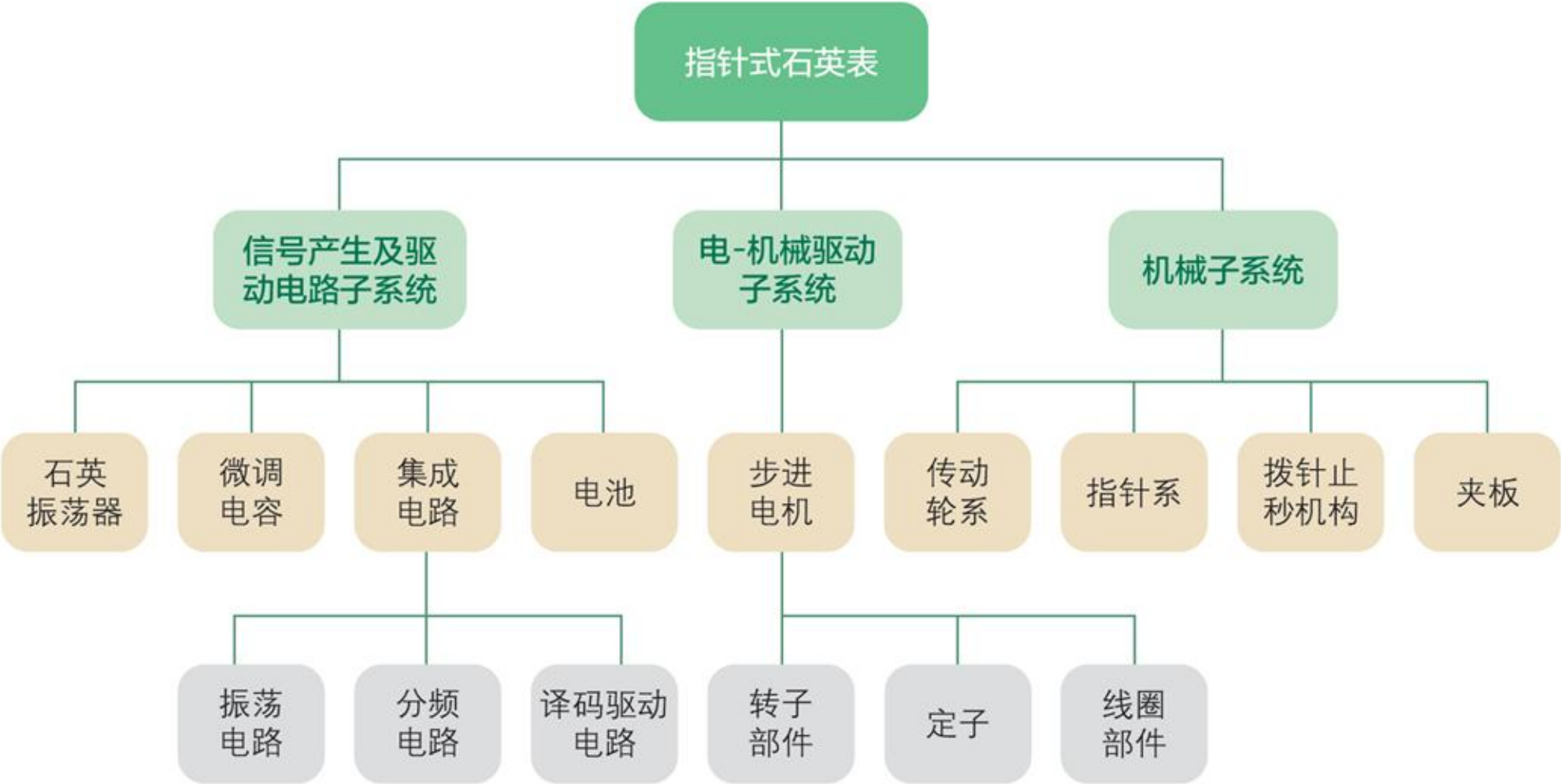
图 3-7 指针式石英表的系统构成
