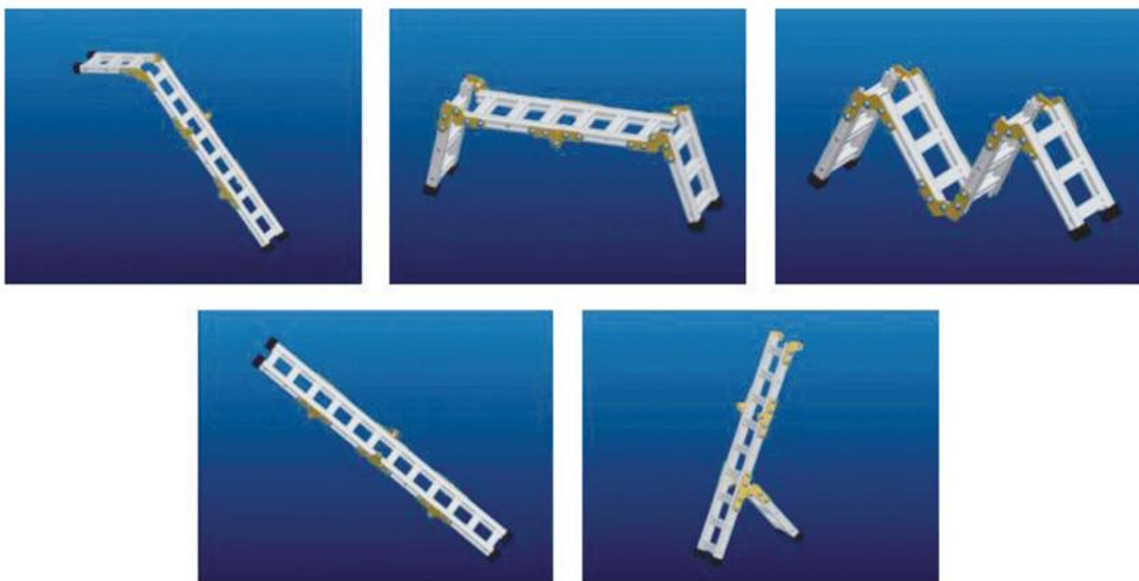
图 1-35 多功能人字梯模型变形图
