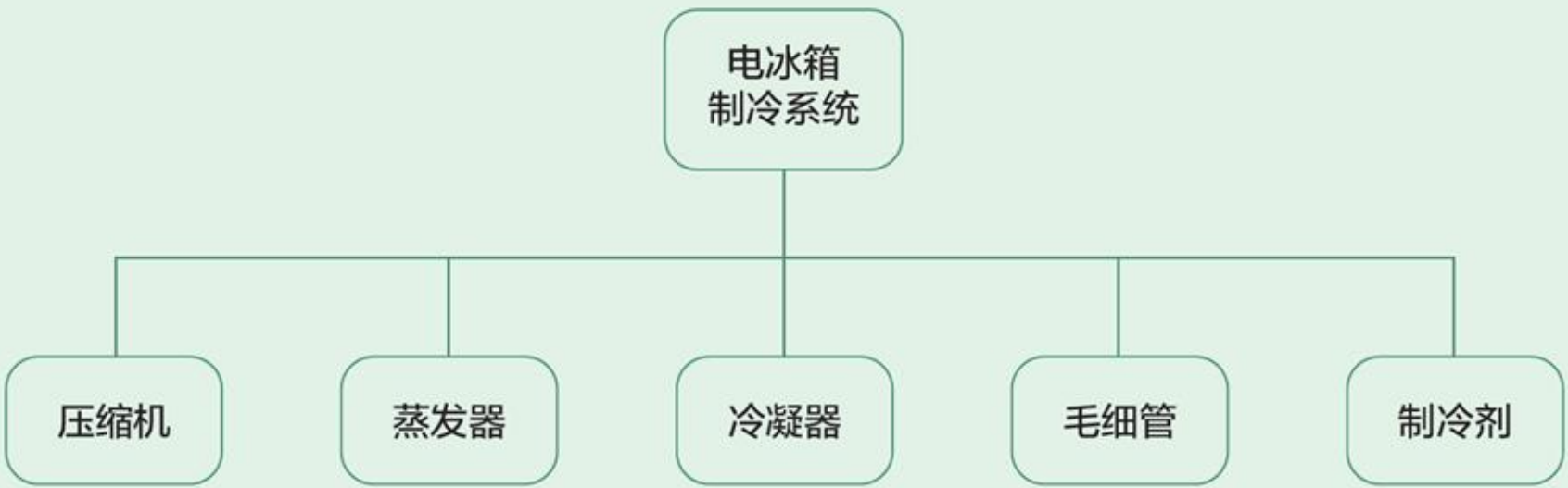
图3-3 电冰箱制冷系统构成
