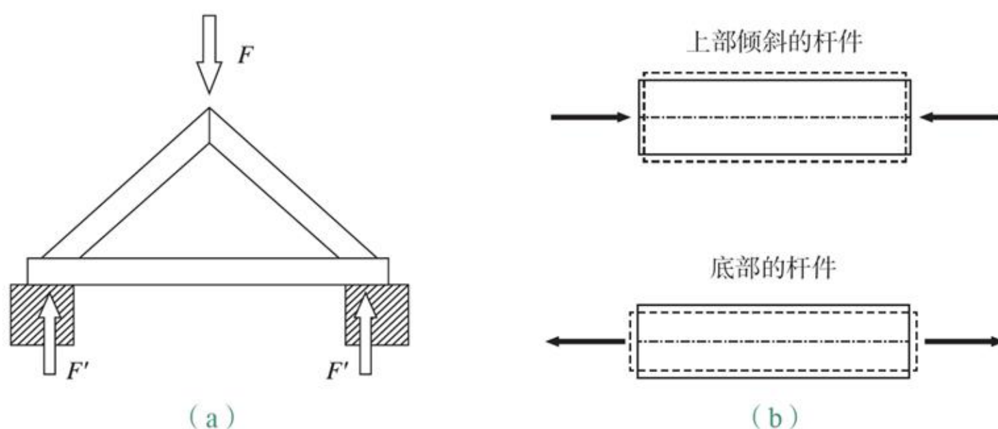
图1-16 三角形桁架受力与形变示意图
