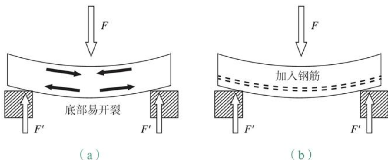
图 1-31 钢筋混凝土梁示意图
