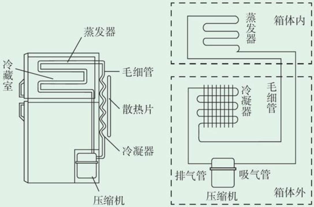
图3-2 电冰箱制冷系统示意图
