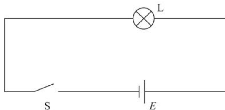
图4-3 台灯模型电路图
