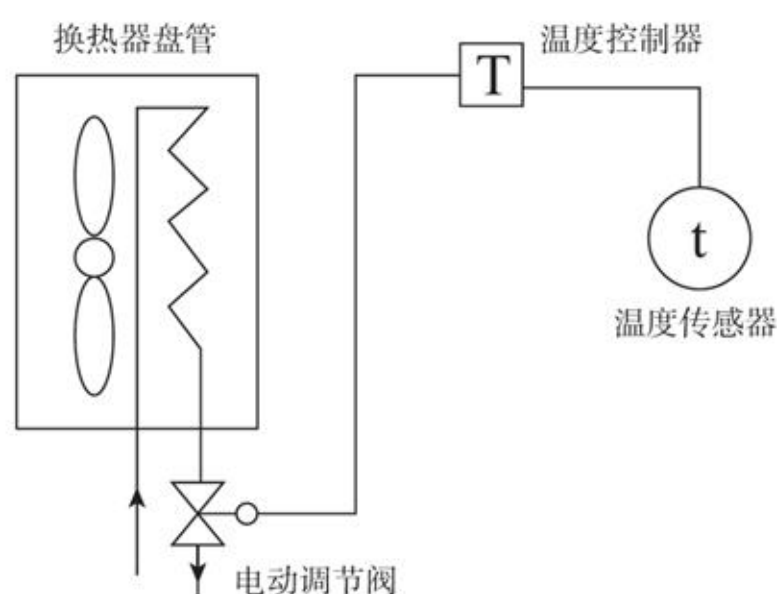
图4-19 空调温度控制系统示意图
