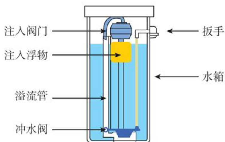
图3-9 水箱注水管系统示意图
