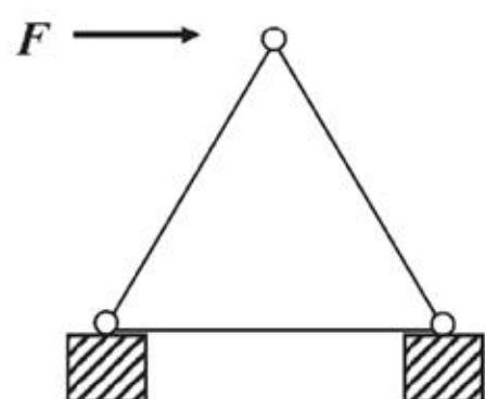
(a) 三角形几何不变体系
