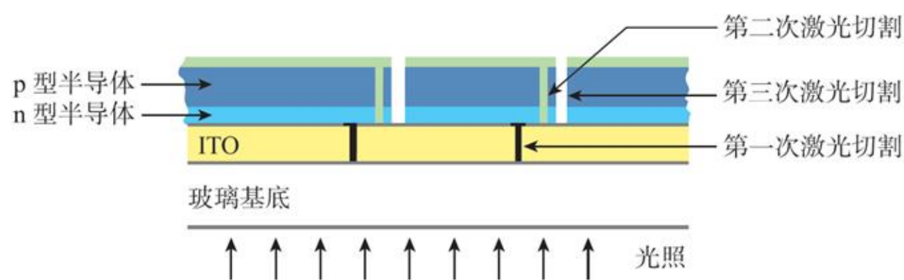
图2-25 三次激光切割的位置示意图
