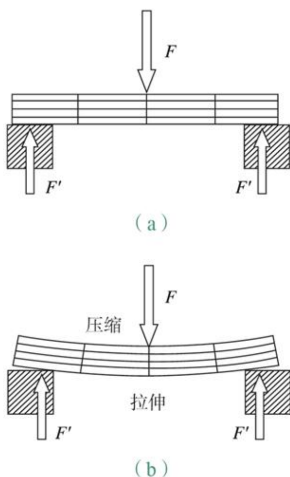
图1-14 梁的受力与形变示意图
