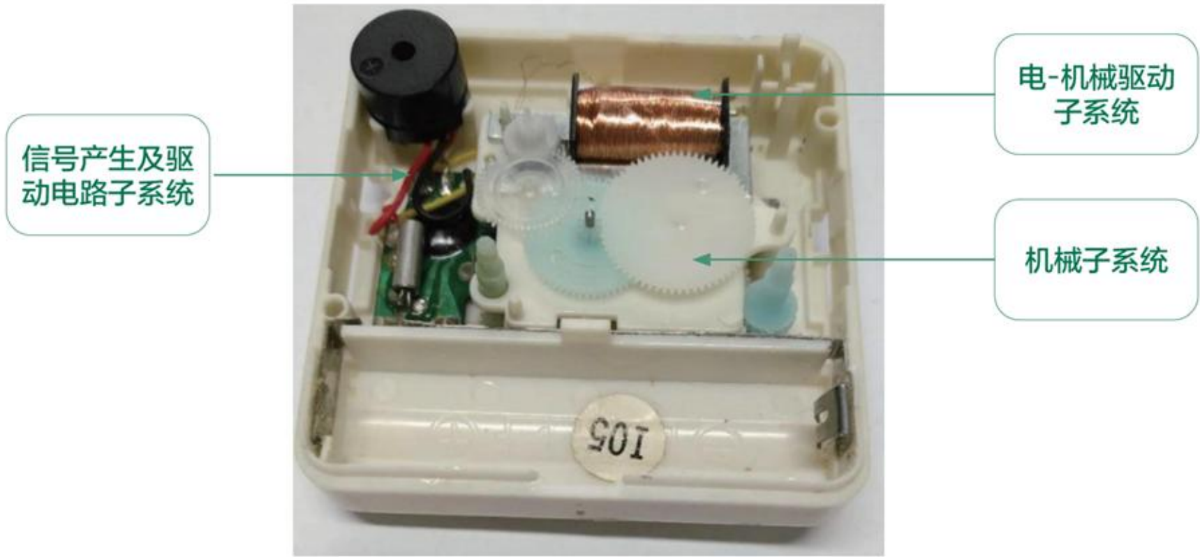
图 3-8 指针式石英表的实物图
