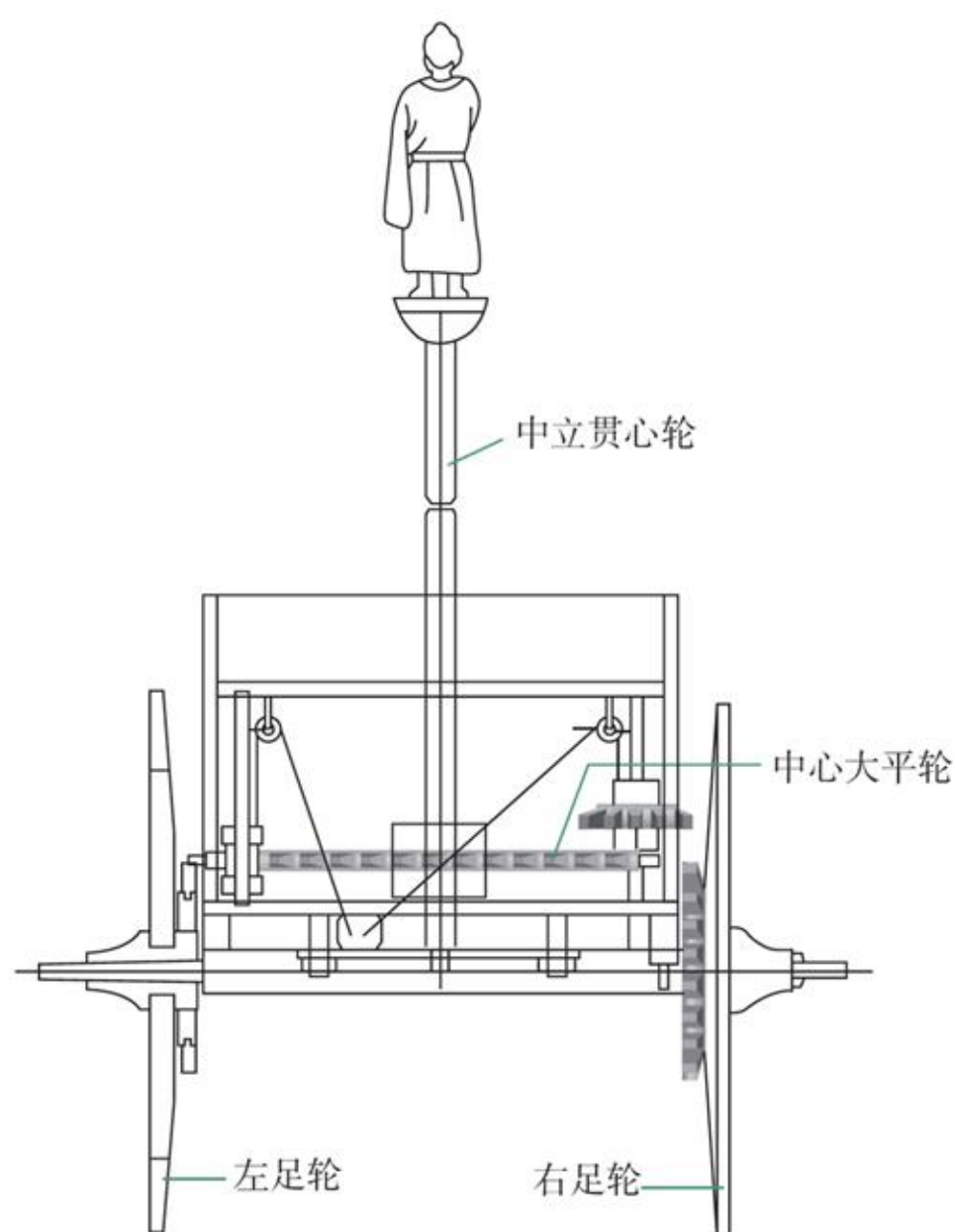
图4-7 一种指南车复原模型结构示意图
