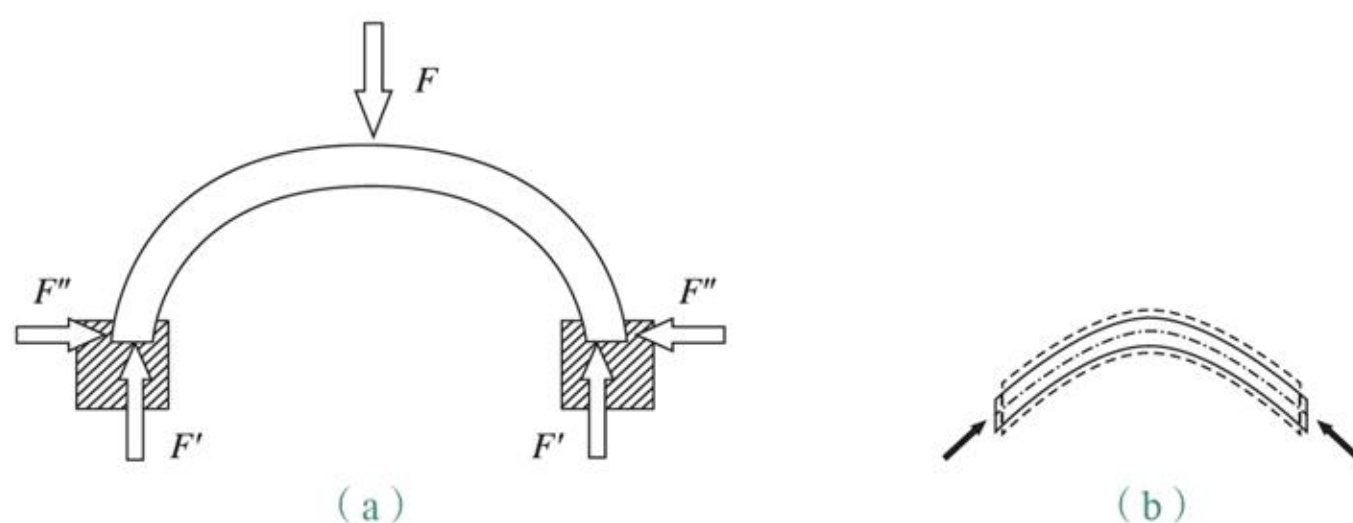
图1-18 弧形拱的受力与形变示意图
