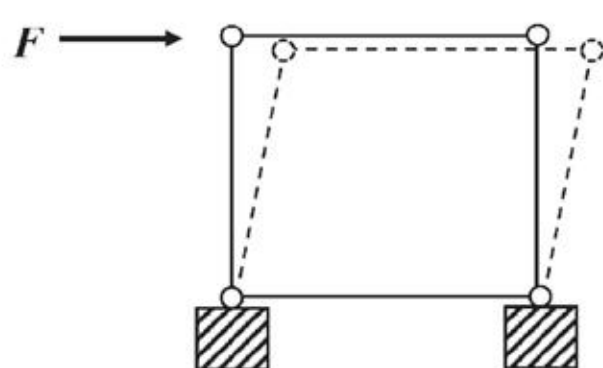
(b) 四边形几何可变体系
