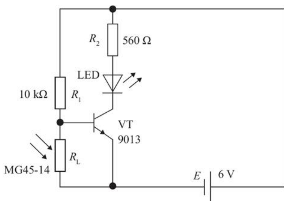
图4-5 路灯模型电路图
