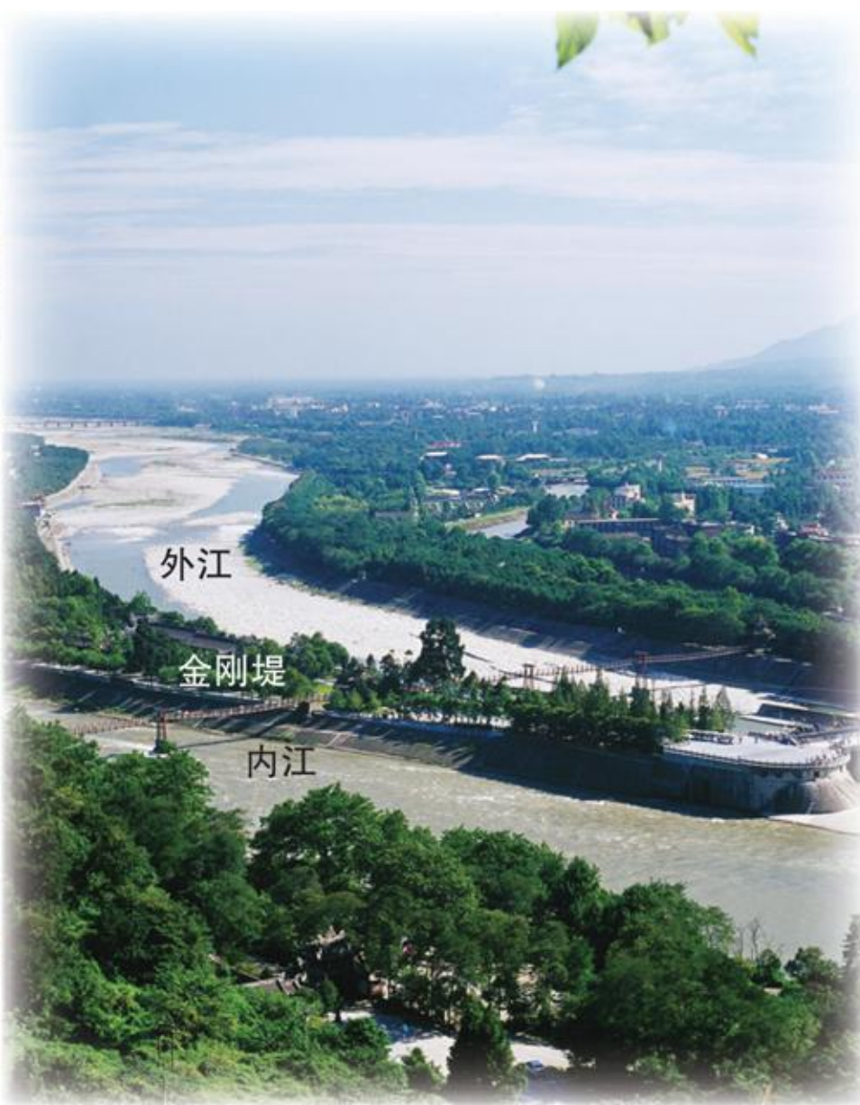
图3-10 都江堰水利工程
