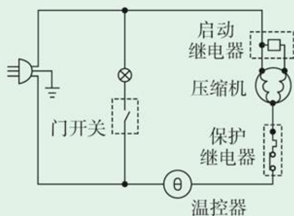
图3-4 电冰箱电气系统示意图
