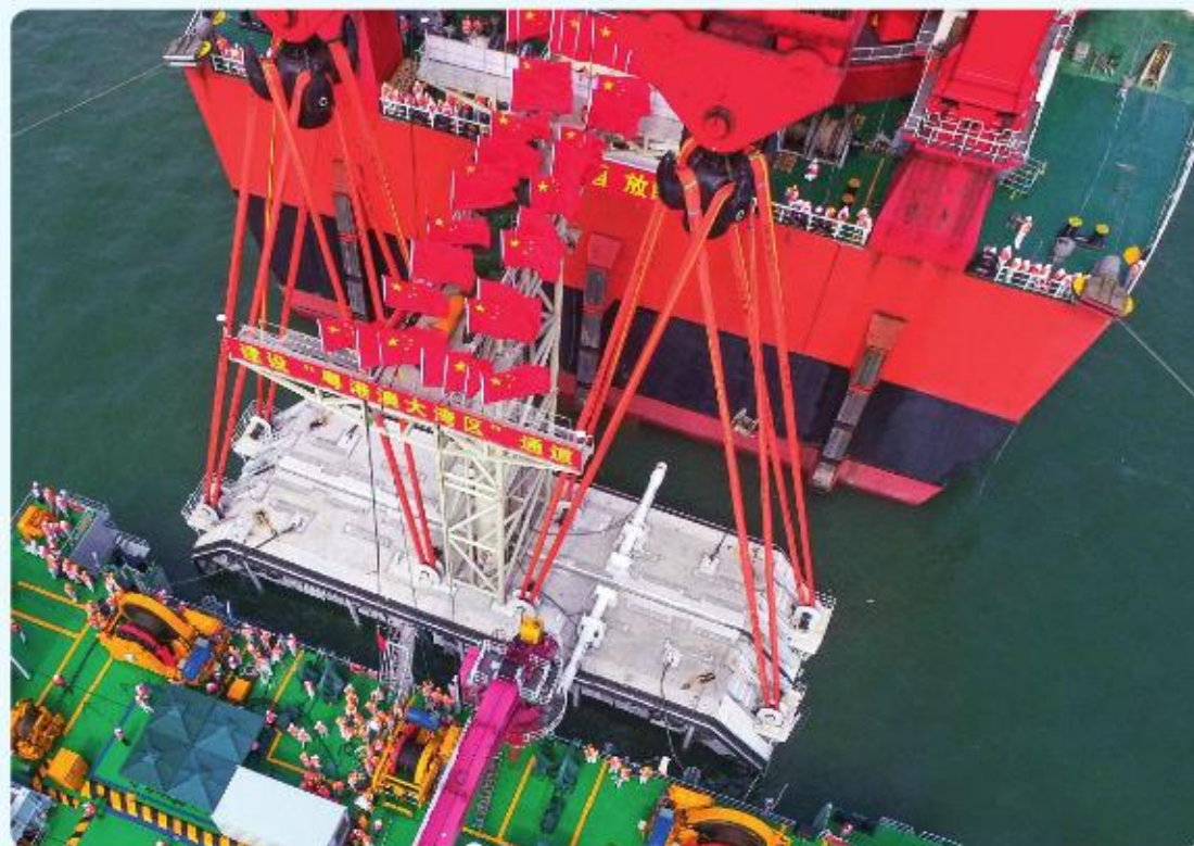
港珠澳大桥岛隧工程海底隧道的最终接头在伶仃洋主航道吊装下沉对接完成
