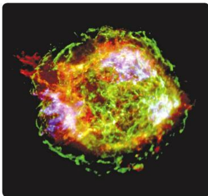
超新星“仙后座A”爆炸形成的壮观美景
