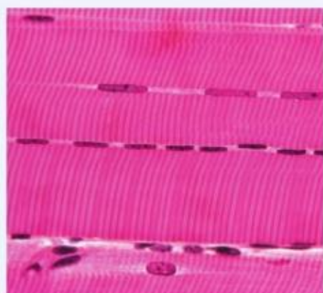
骨骼肌细胞
