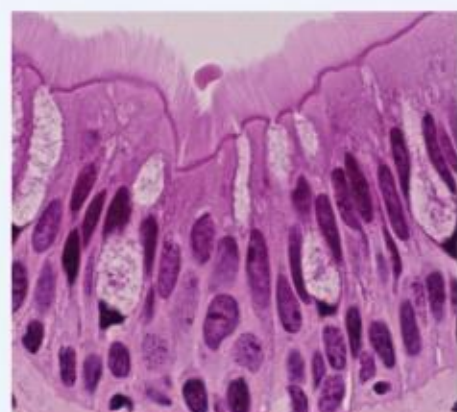
上皮细胞
