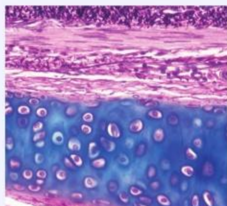
软骨细胞
