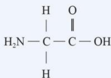
甘氨酸
