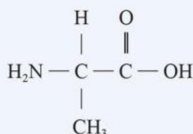
丙氨酸
