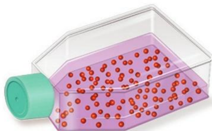
细胞培养
