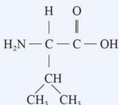
缬氨酸
