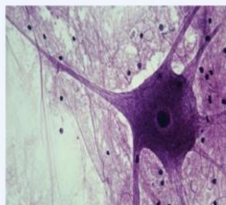
神经细胞
