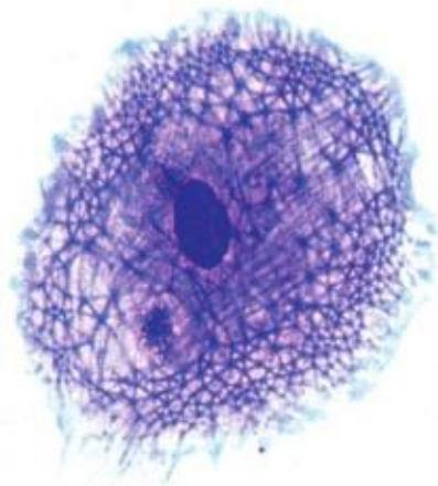
▲ 图 3-7 细胞骨架
