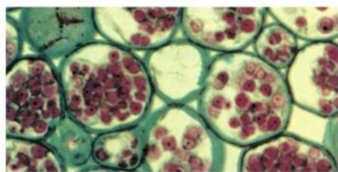
储藏细胞
