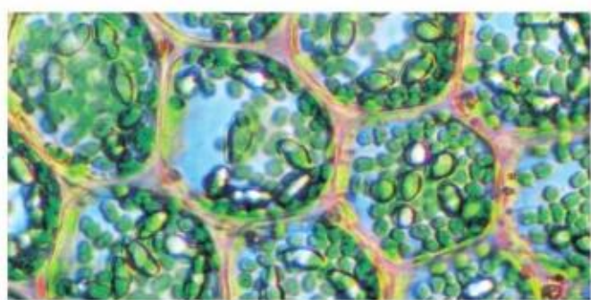
叶肉细胞
