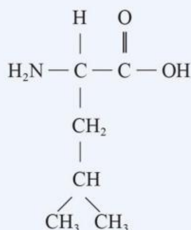
亮氨酸
