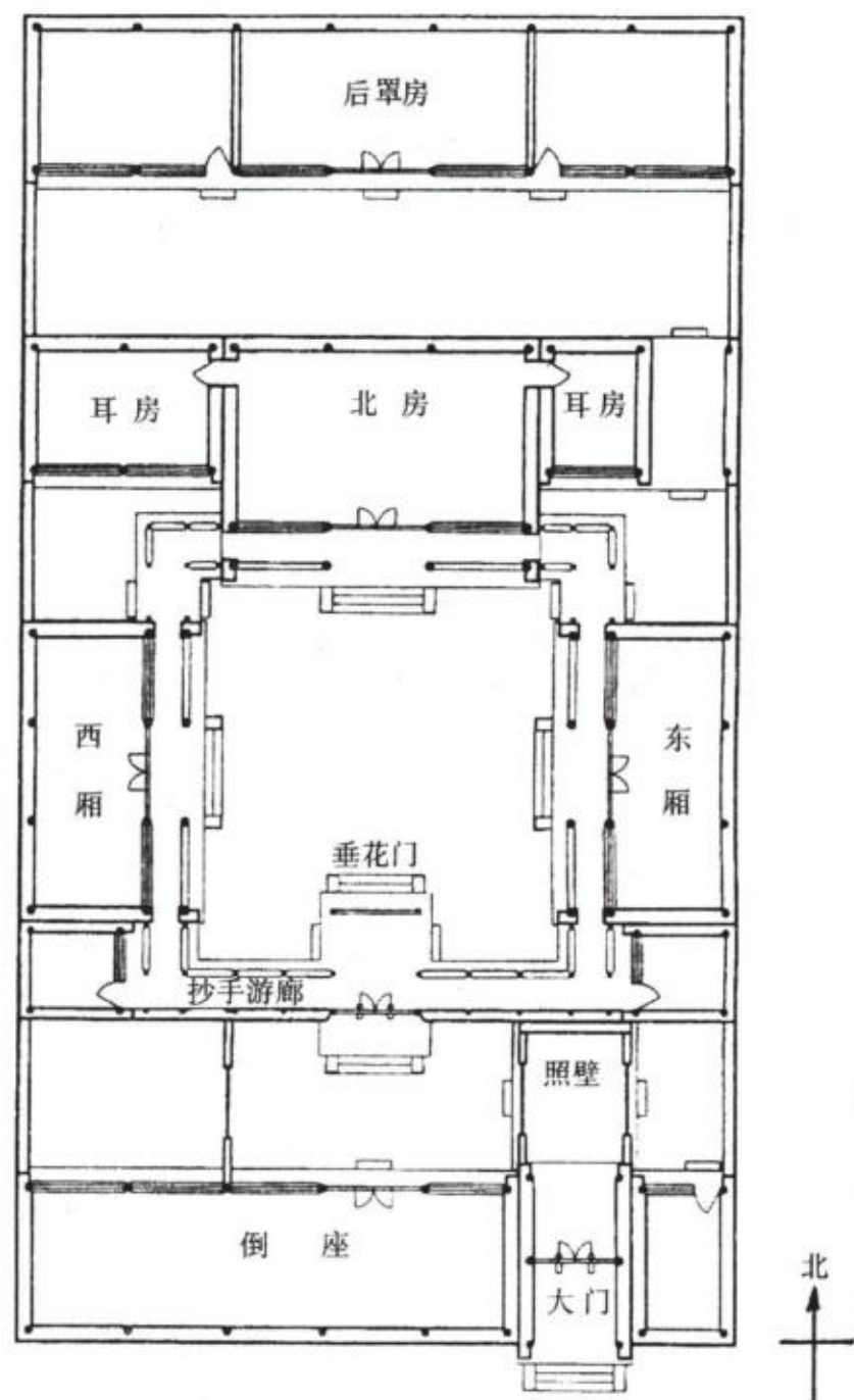
◇北京典型三进院四合院平面图
