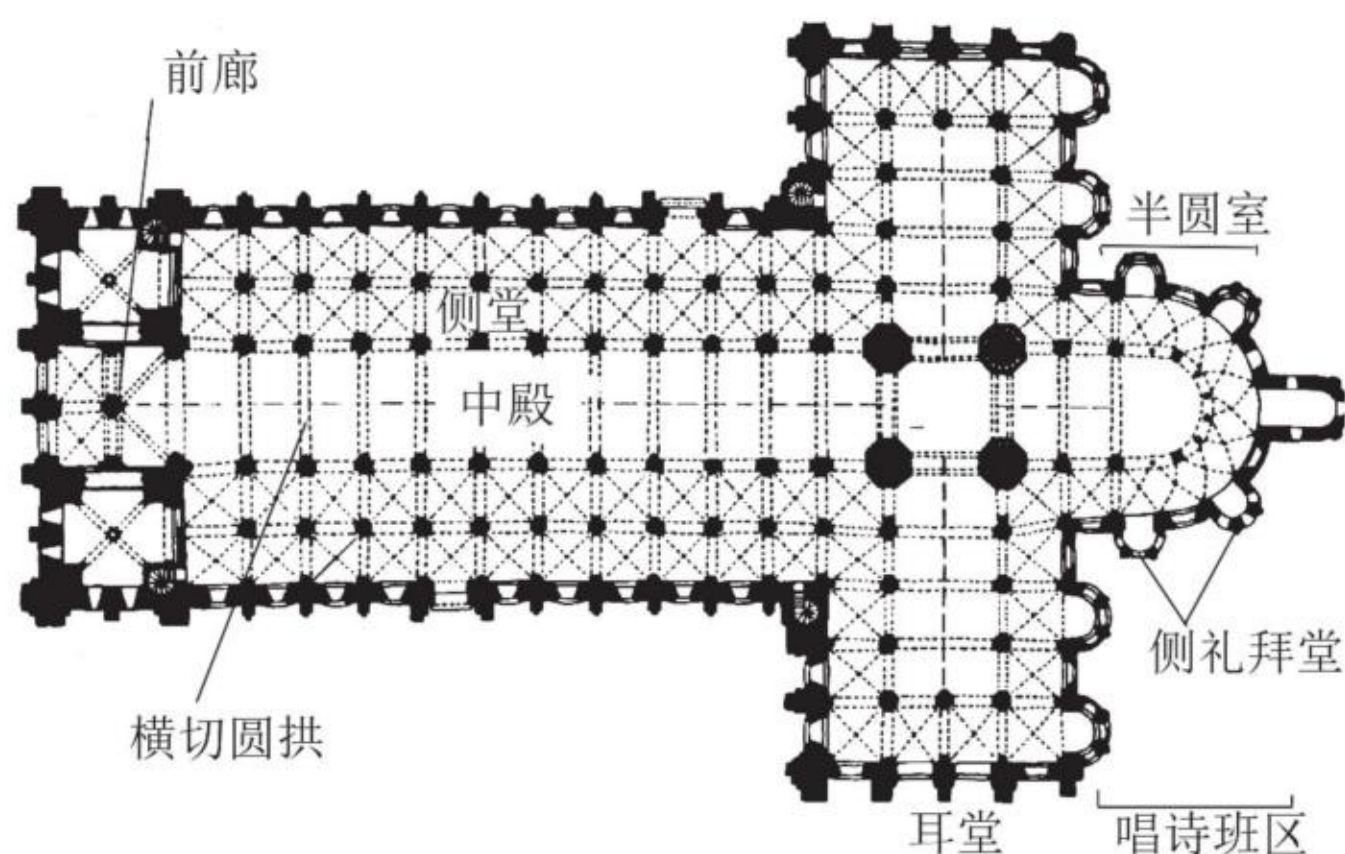
◇ 圣塞尔南教堂平面图
