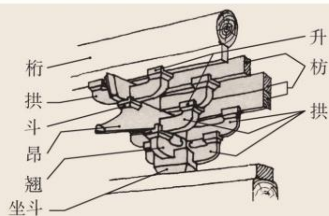
◇ 斗拱结构示意图
