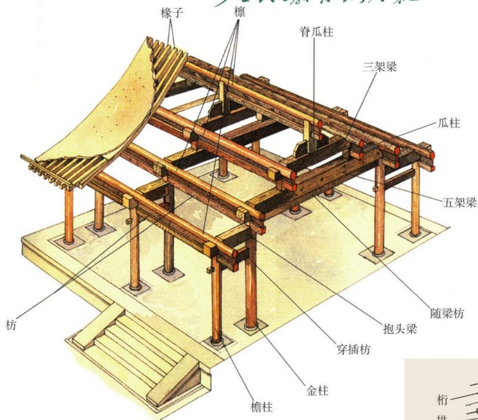
◇ 硬山式木构架结构示意图
