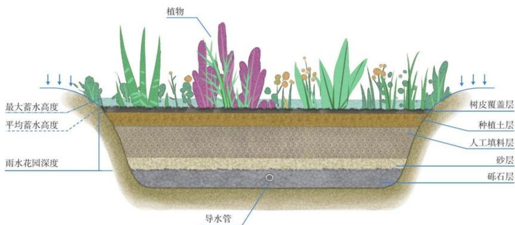
图5.23 典型雨水花园结构示意图
