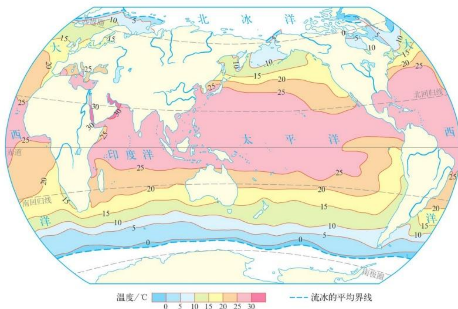
图 3.9 世界大洋 8 月表层海水温度分布
