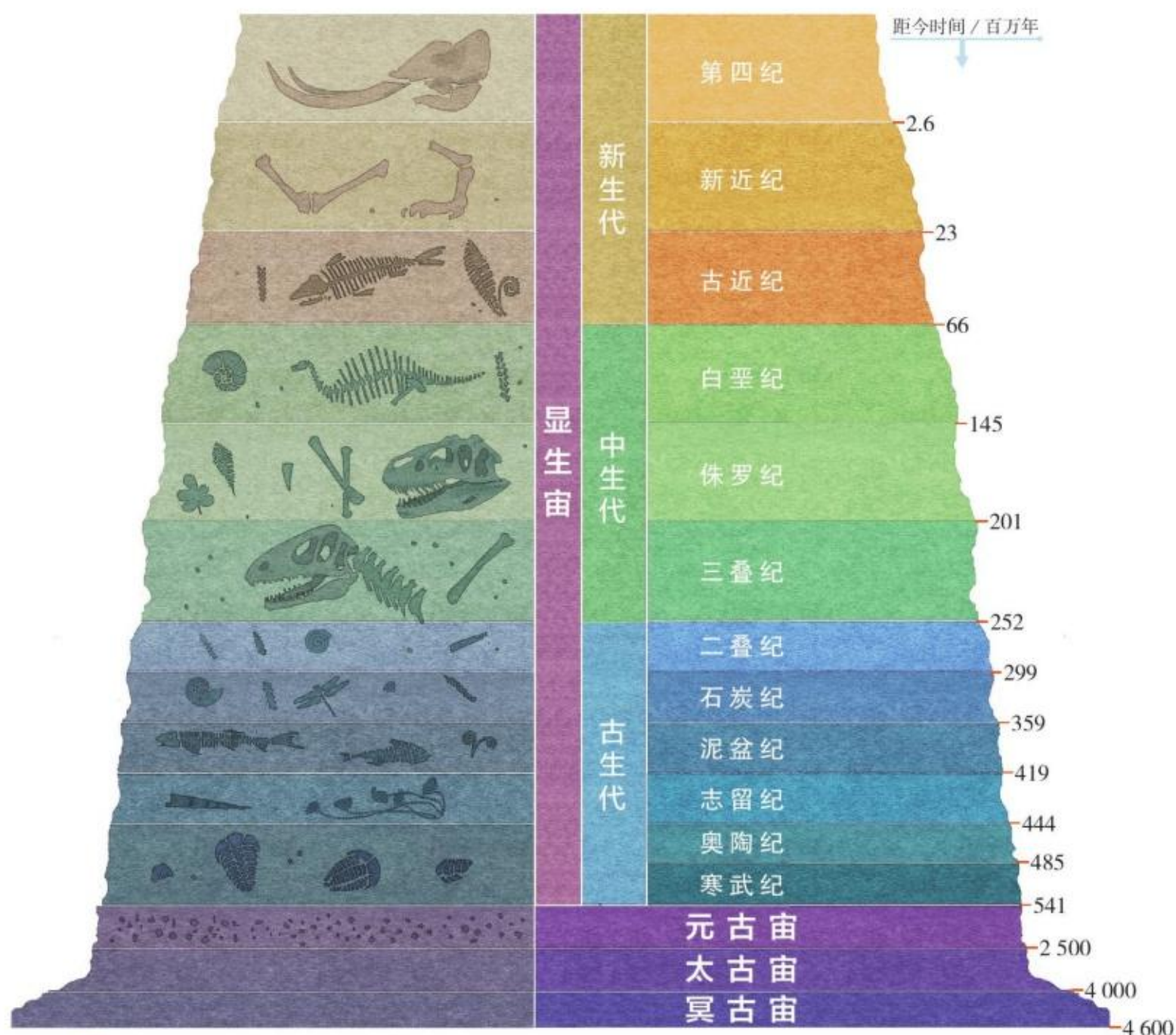
图 1.24 地质年代表示意 (a)
