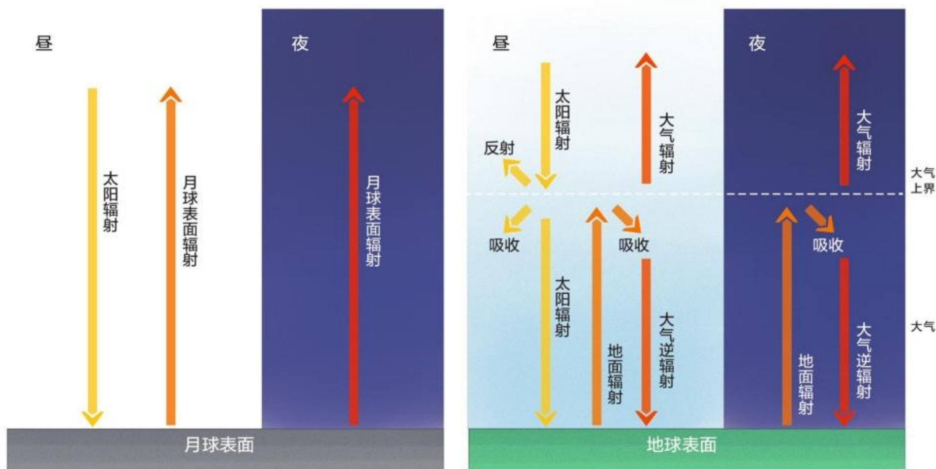
图 2.10 地球和月球表面辐射过程示意
