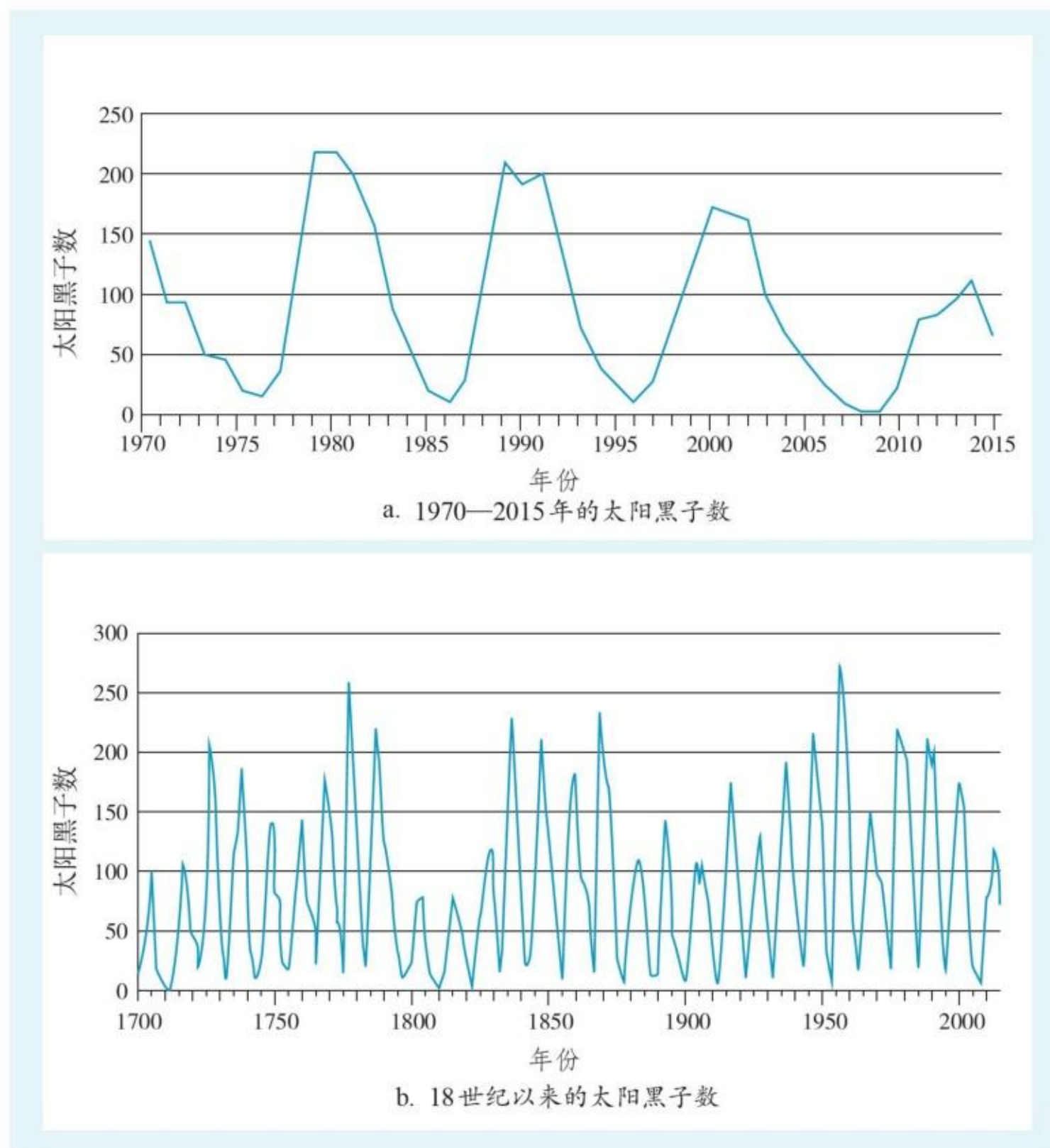
图 1.20 太阳黑子数的变化
