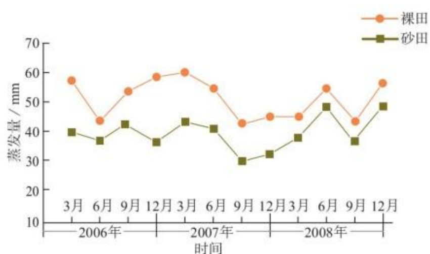
图3.4 砂田和裸田的蒸发量
