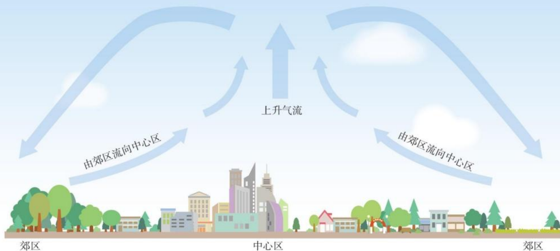
图2.12 城市热岛环流示意
