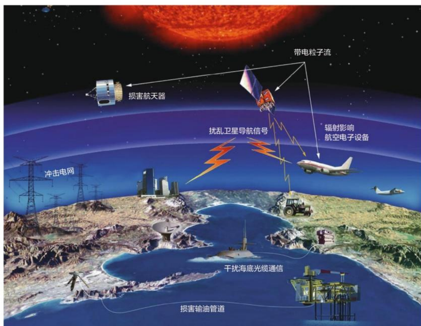
图 1.19 太阳活动强烈时对地球的影响
