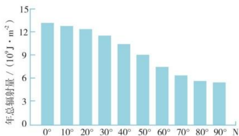
图 1.12 北半球大气上界太阳辐射的分布
