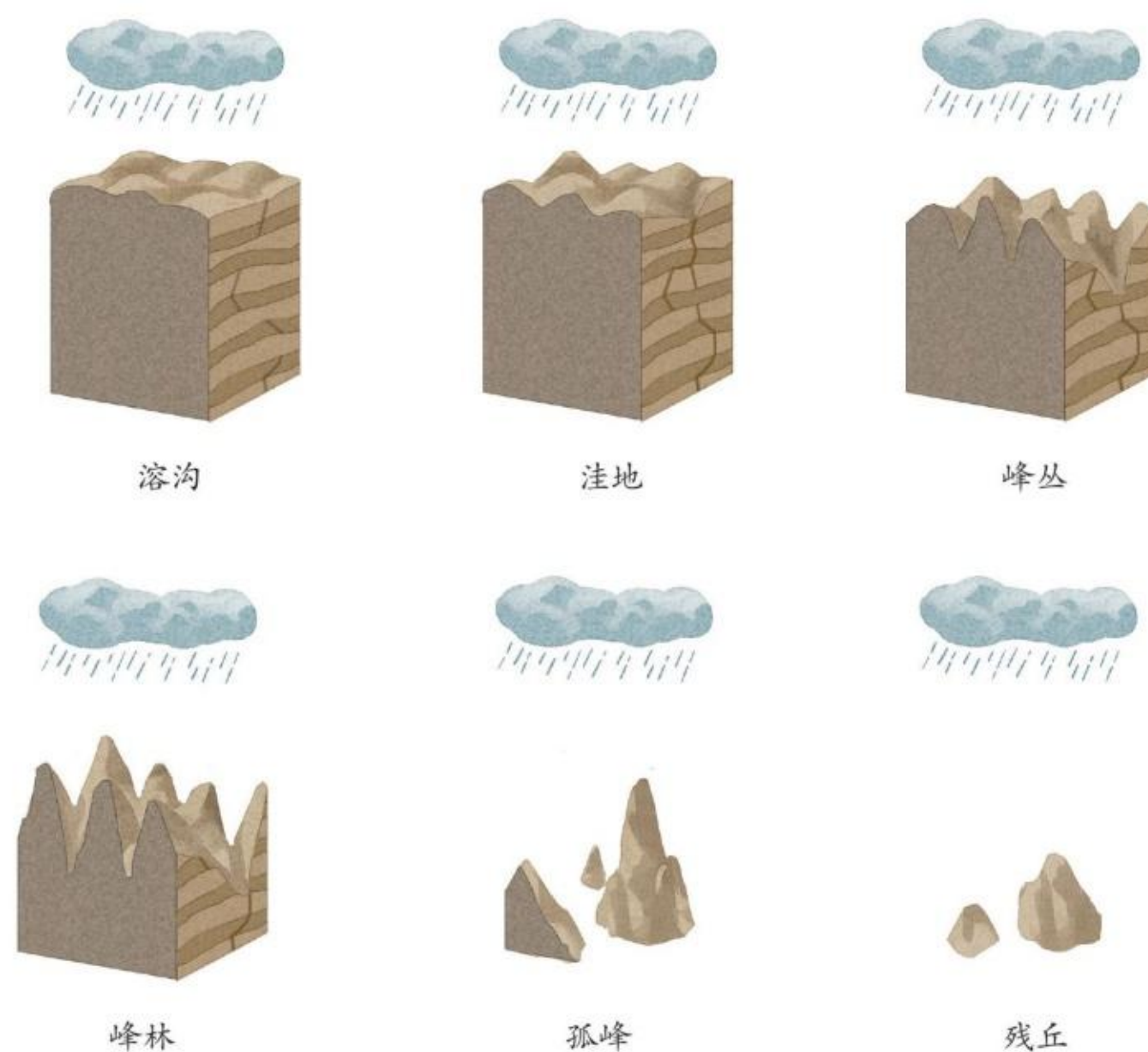
图4.2 地表喀斯特地貌景观演变示意
