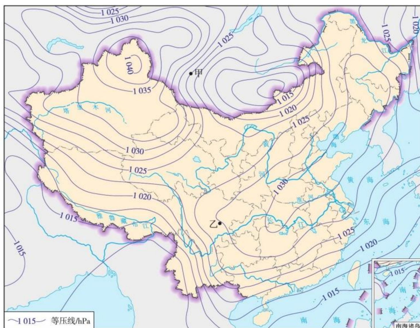
图2.17 海平面气压分布（2016年11月9日6时）
