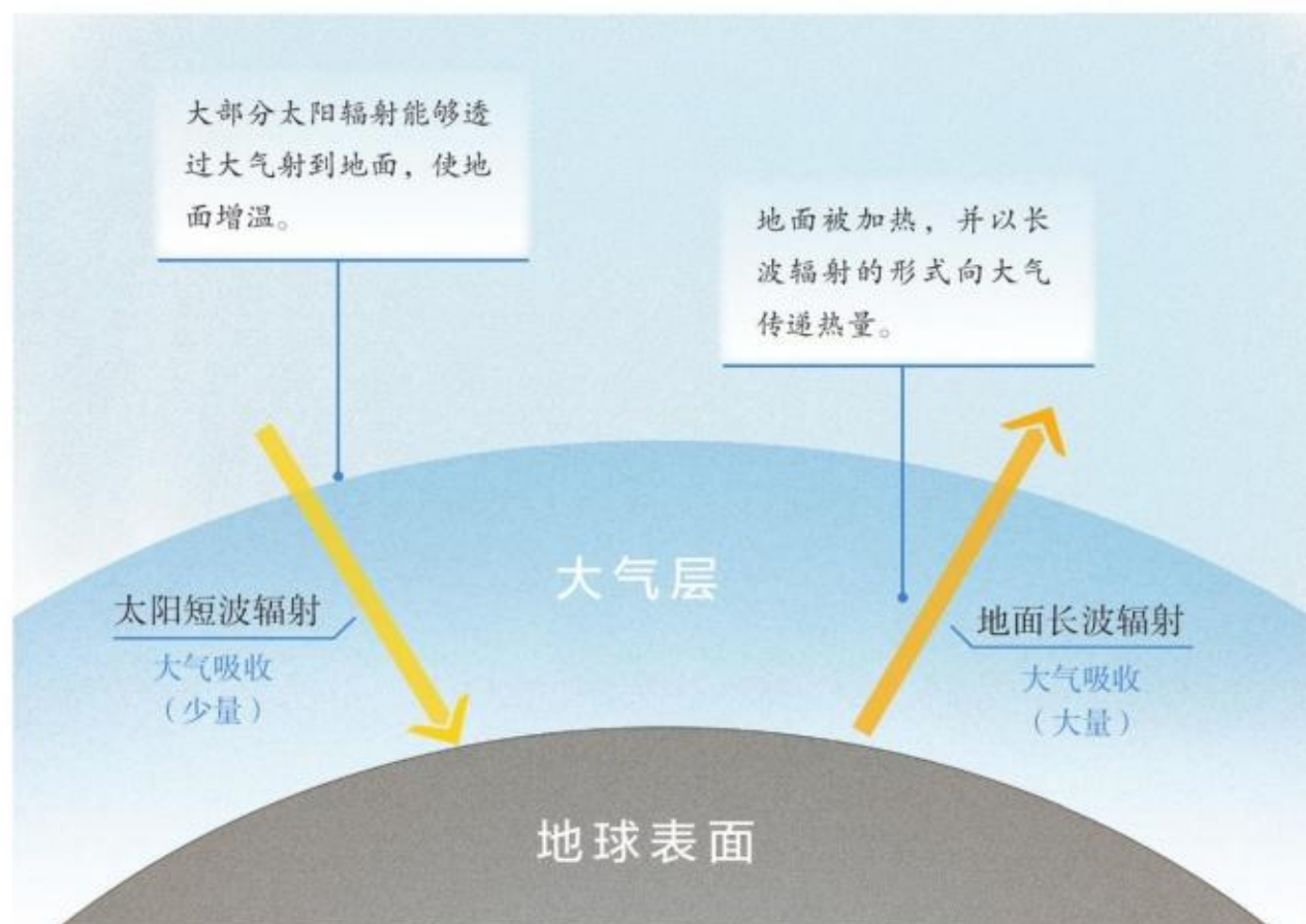
图 2.9 大气的受热过程示意
