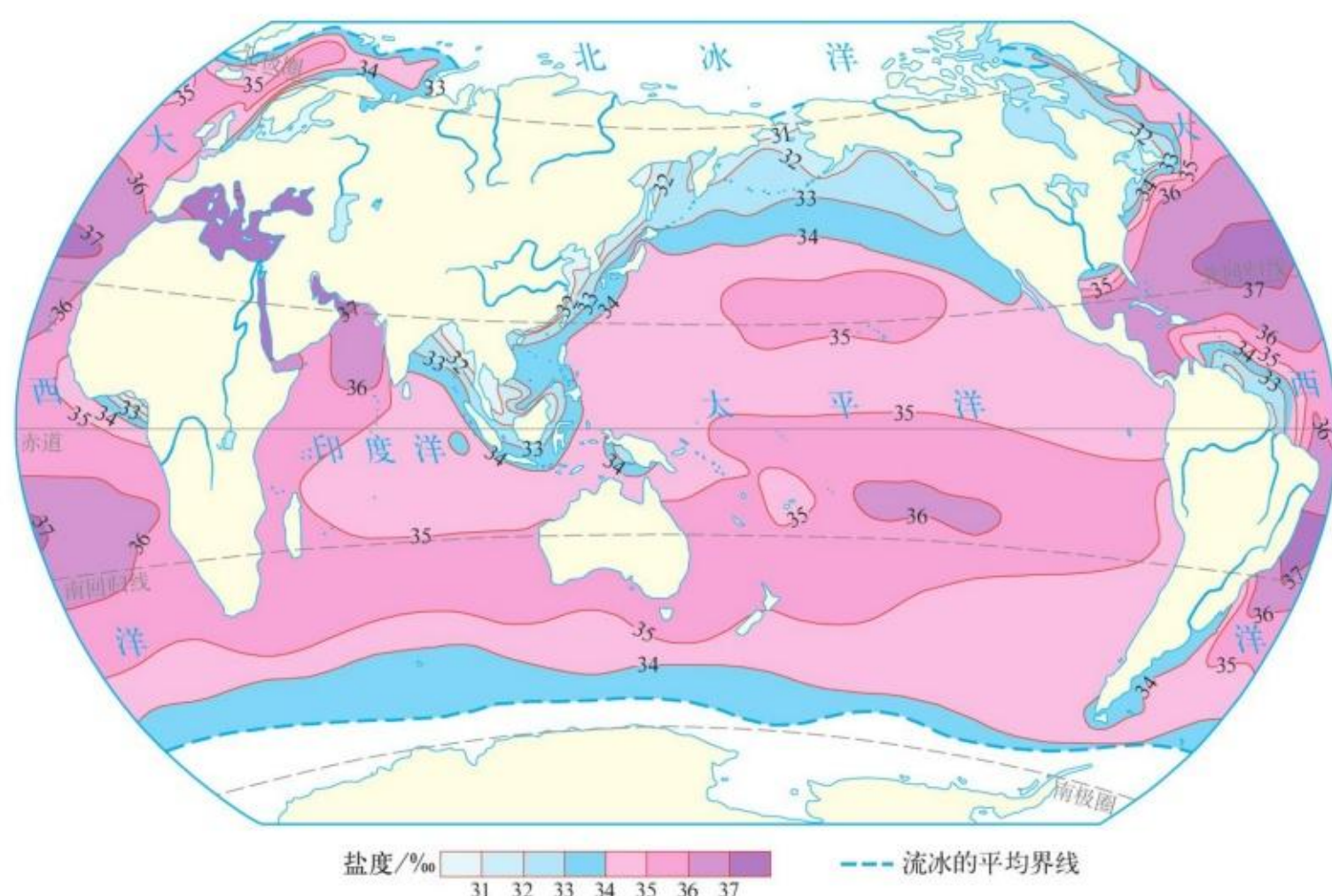
图3.12 世界大洋8月表层海水盐度分布
