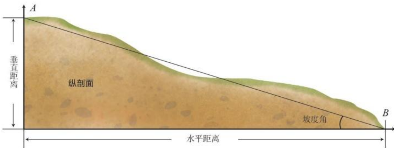
图4.23 坡和坡度角示意
