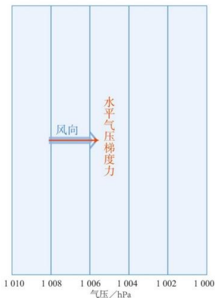
图2.14 在水平气压梯度力作用下的风向
