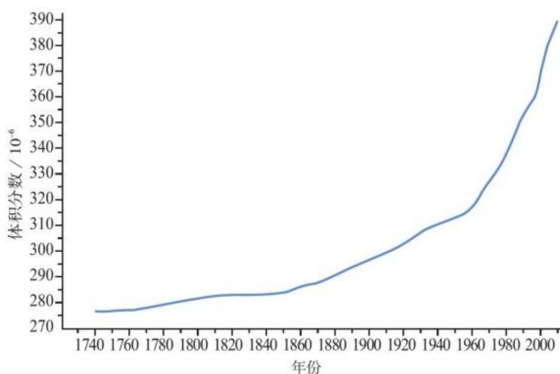
图2.4 二氧化碳体积分数的变化
