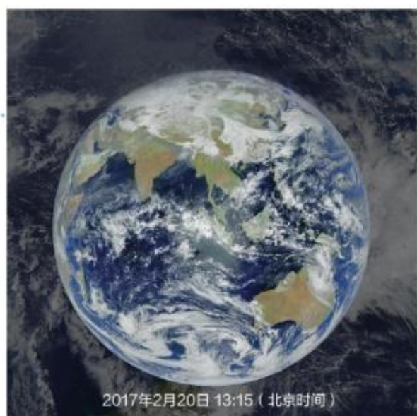
图 1.1 中国“风云四号”气象卫星拍摄的地球
