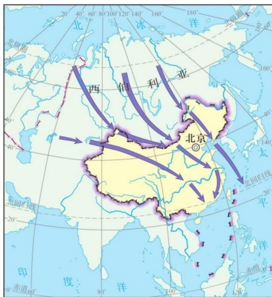
图6.9 侵入我国的寒潮路径示意
