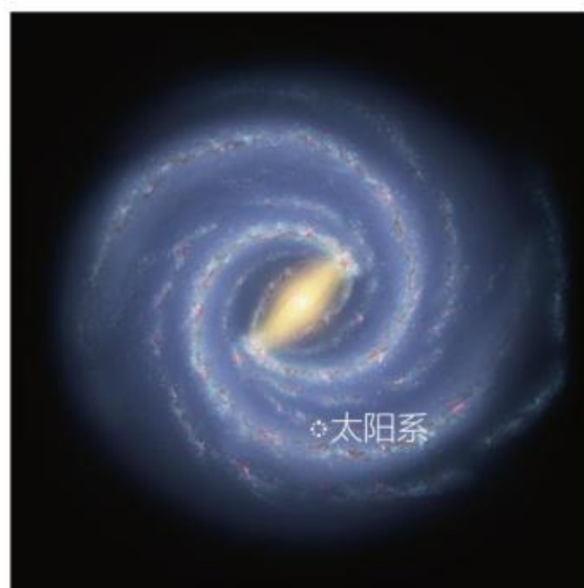
图 1.6 太阳系在银河系中的位置
