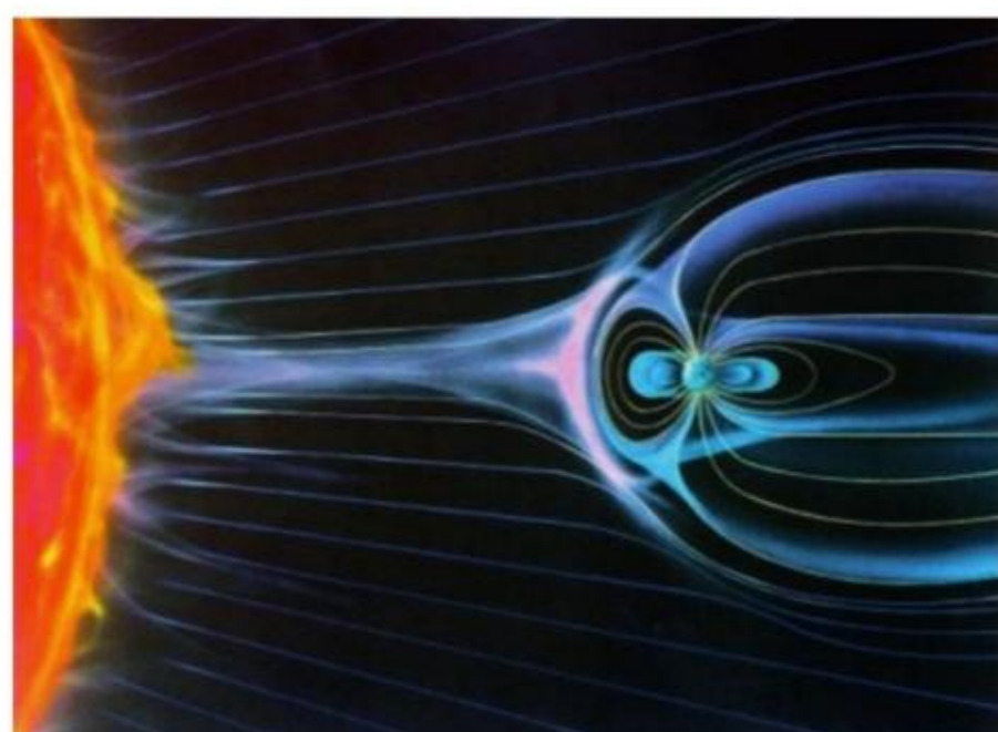
图1.17 吹向地球的太阳风
