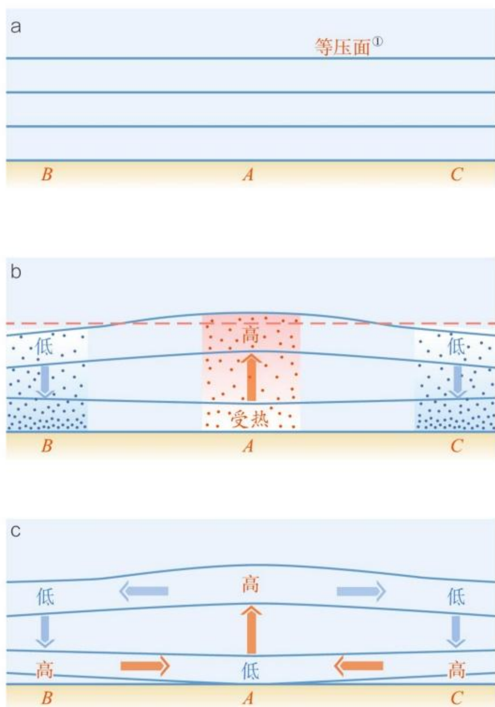
图2.11 热力环流的形成示意
