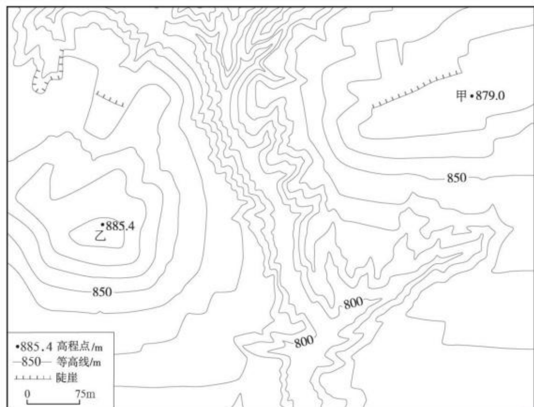
图4.22 黄土高原某地等高线地形示意
