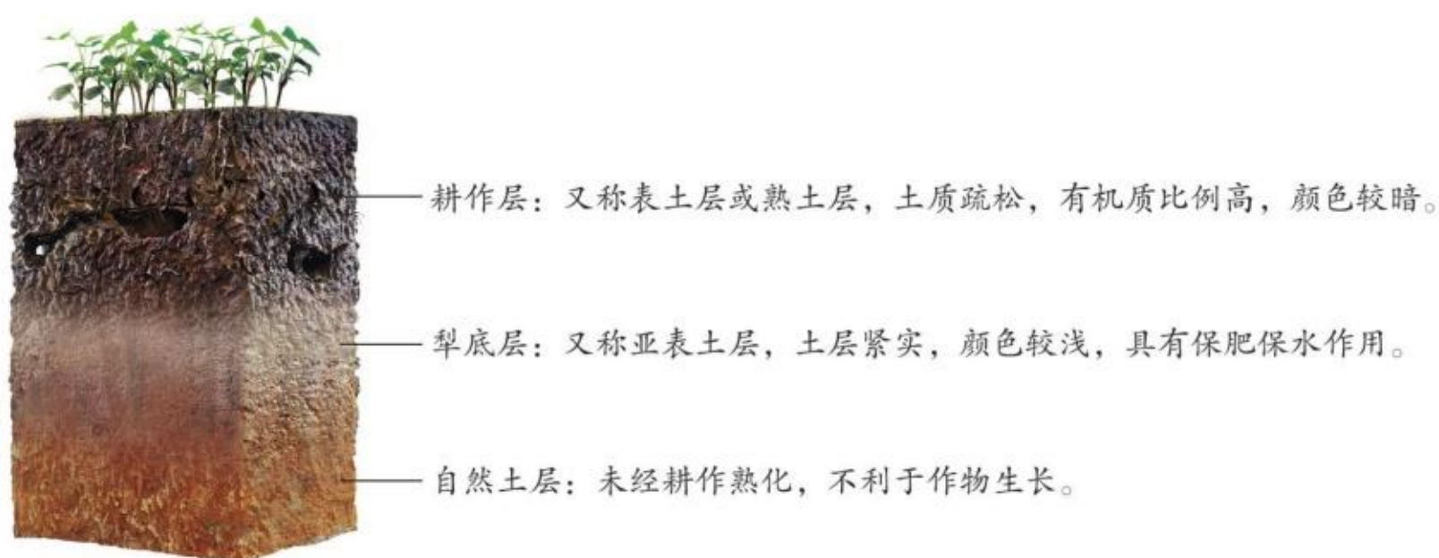
图 5.18 耕作土壤剖面示意及各土层特点
