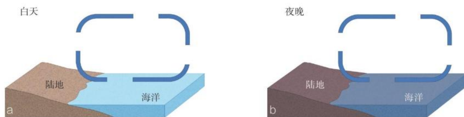
图2.13 海陆间的大气热力环流
