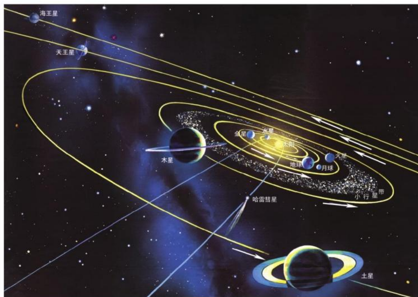
图1.4 太阳系结构示意图
