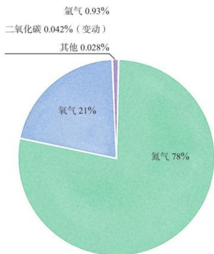
图 2.2 干洁空气成分的体积分数（25千米以下）
