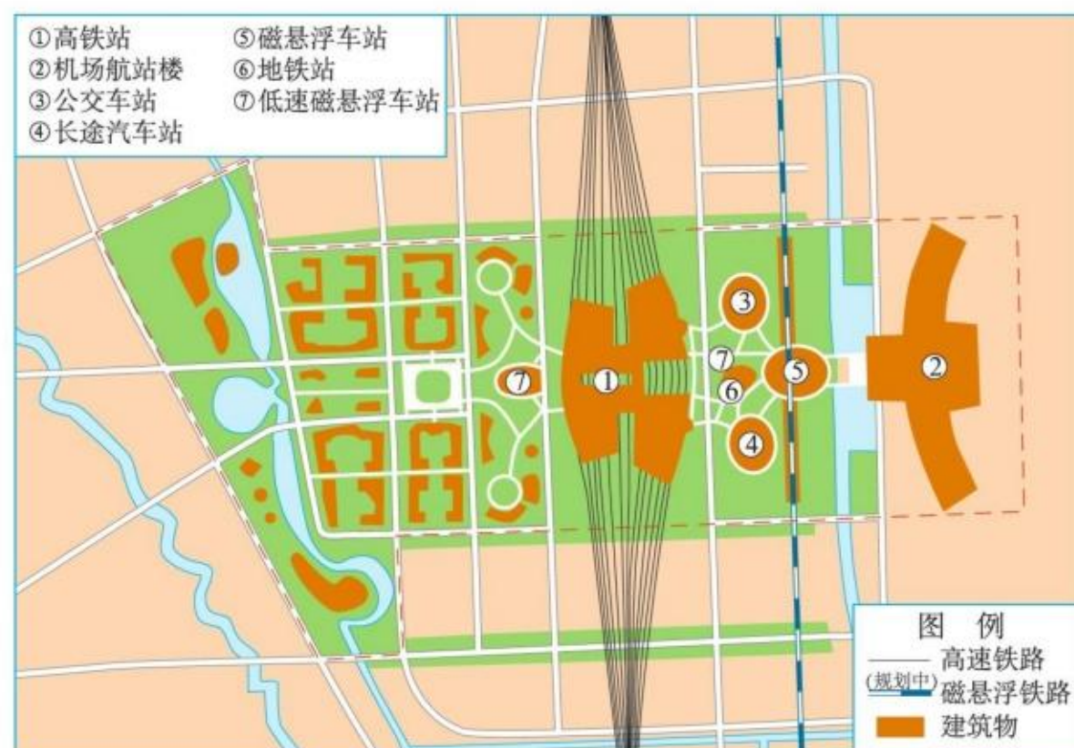
图4.4 上海虹桥综合交通枢纽平面示意
