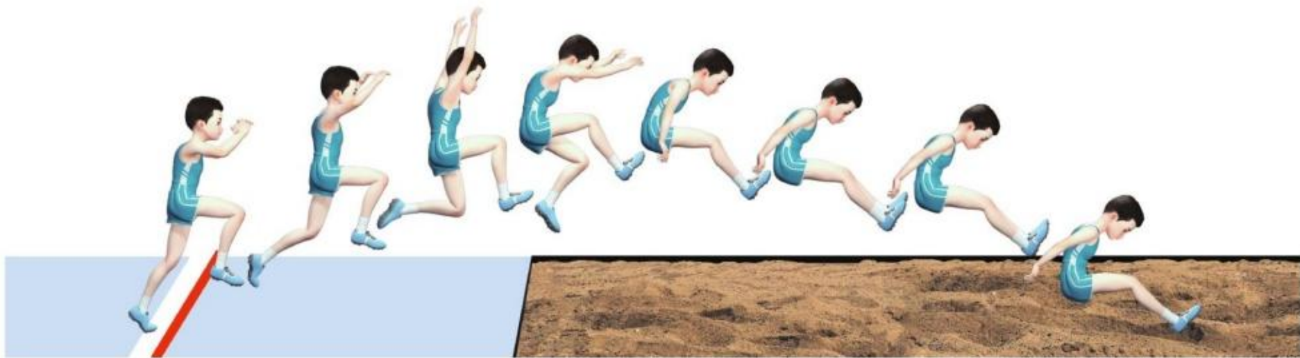
图 4-2-2 蹲踞式跳远
