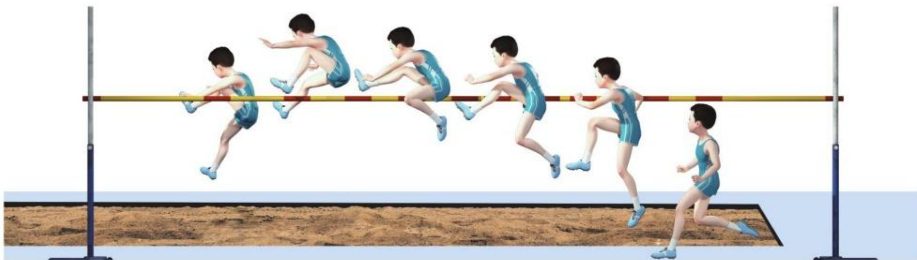
图 4-2-4 跨越式跳高
