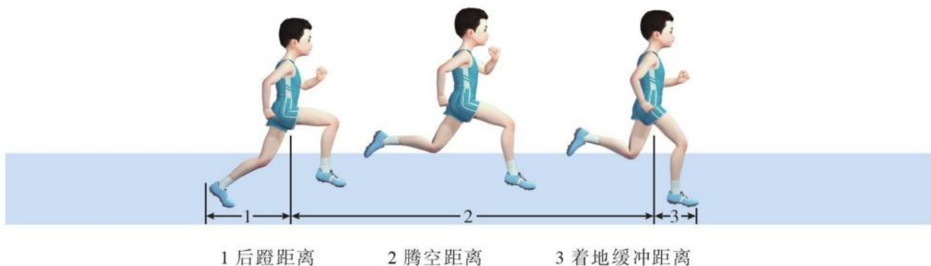
图 3-2-2 步长的组成
