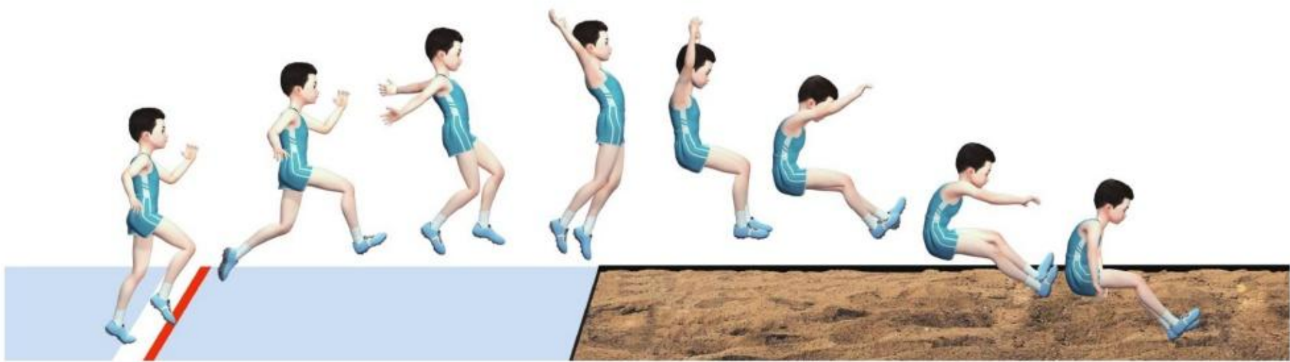
图 4-2-3 挺身式跳远
