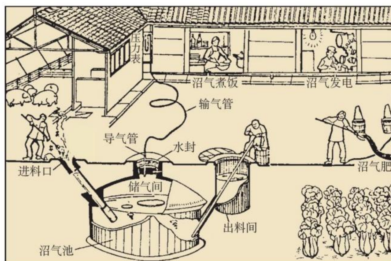
图7-21 沼气的制取和利用示意图
