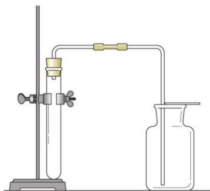
图 6-21 制取二氧化碳的装置
