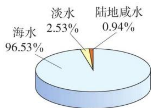
图4-1 地球咸水、淡水的储量比
