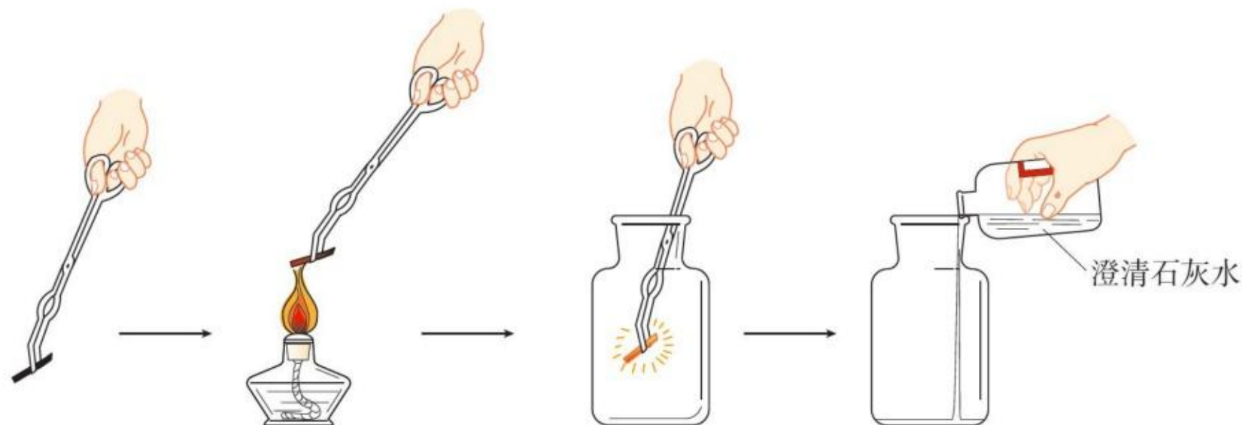
图2-19 木炭在氧气中燃烧实验示意图
