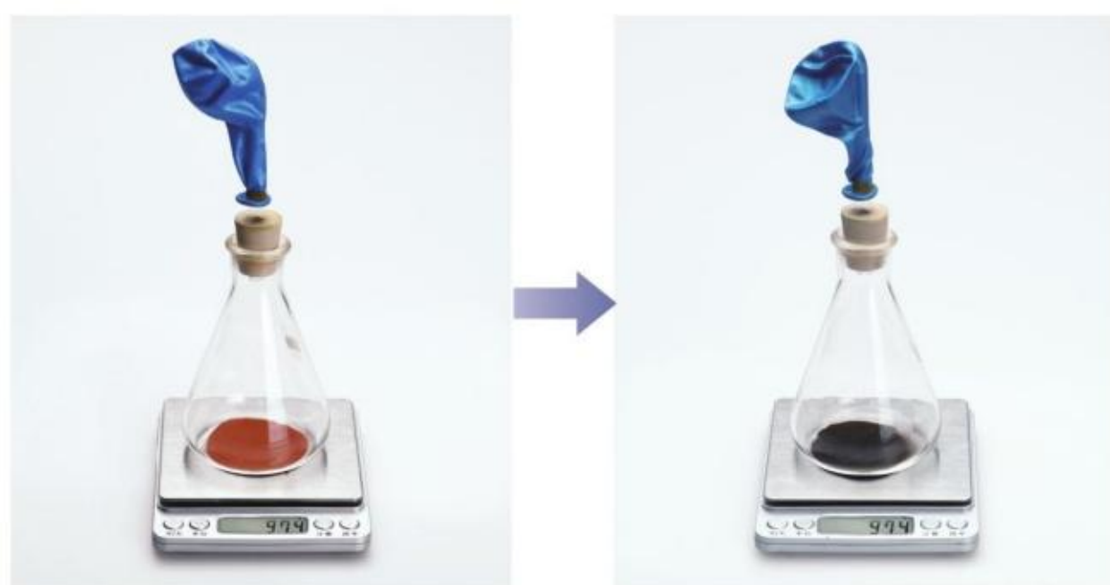
图5-1 铜与氧气反应前后质量的测定
