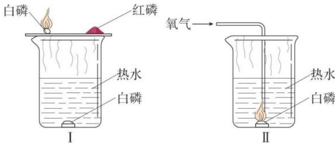
图 7-3 探究燃烧的条件实验示意图
