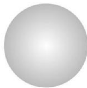
图3-15 道尔顿原子模型示意图
