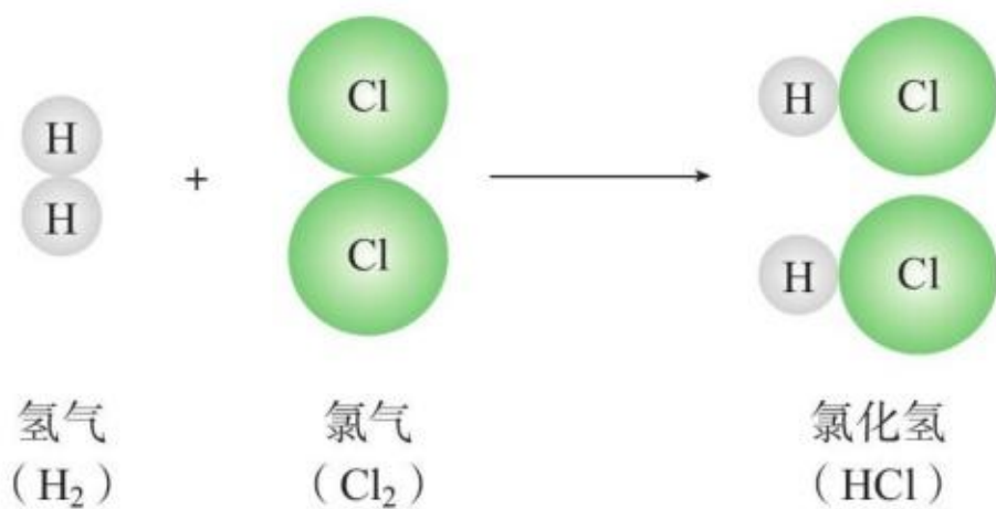
图3-7 氢气与氯气反应的示意图
