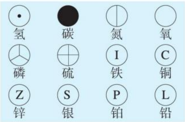
图3-21 道尔顿的元素符号
