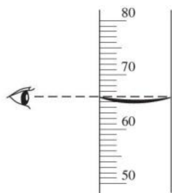
读取量筒内液体的体积
