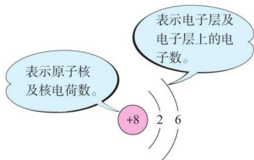
图3-11 氧原子的结构示意图
