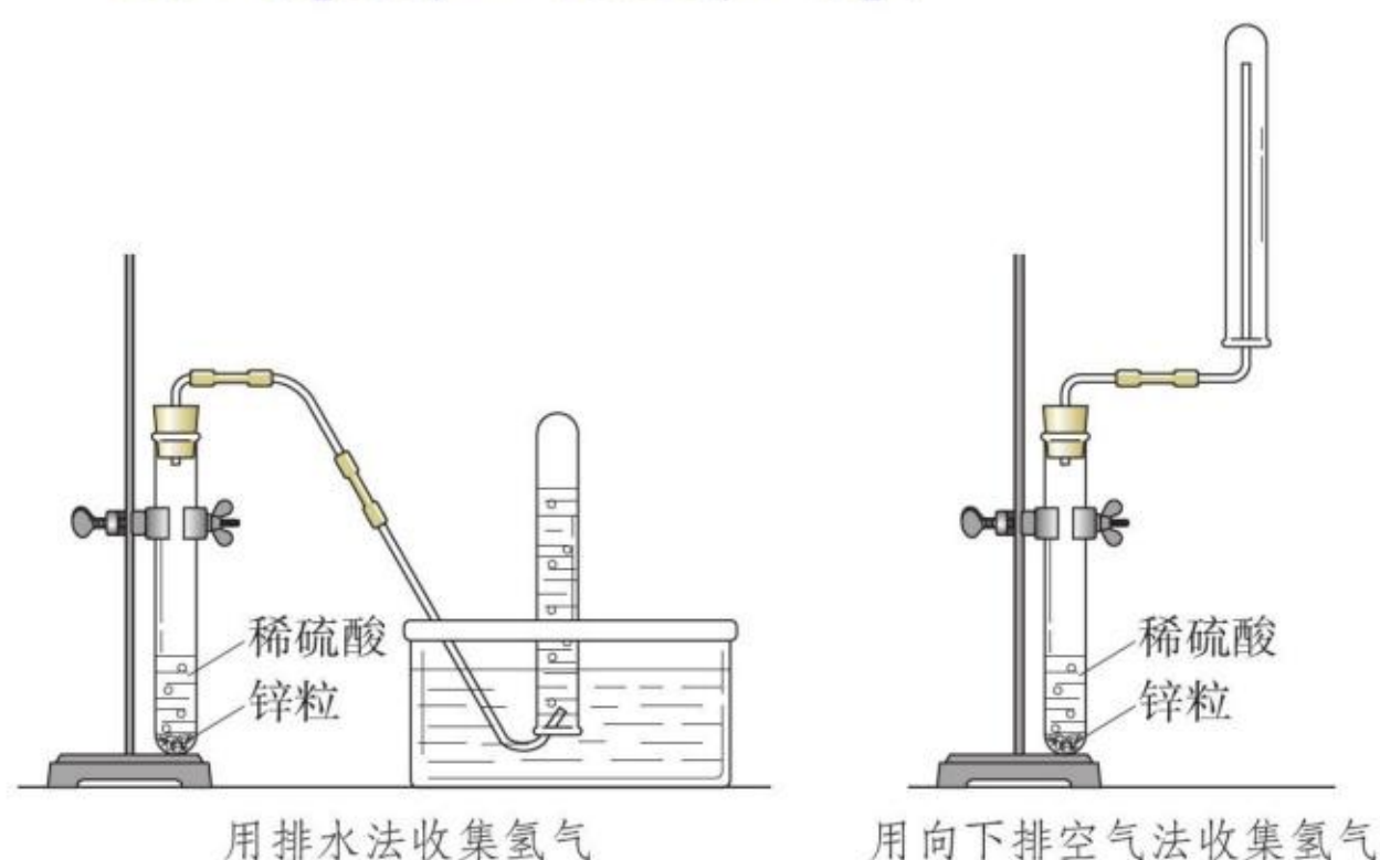
图7-26 实验室里制取氢气的简易装置
