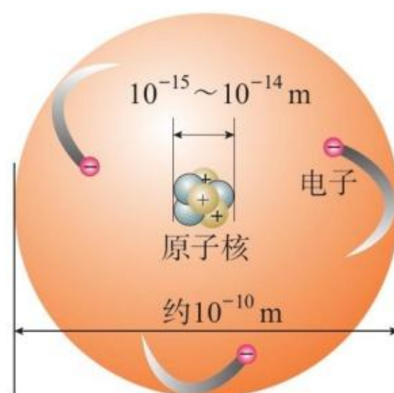
图3-9 原子的构成示意图
