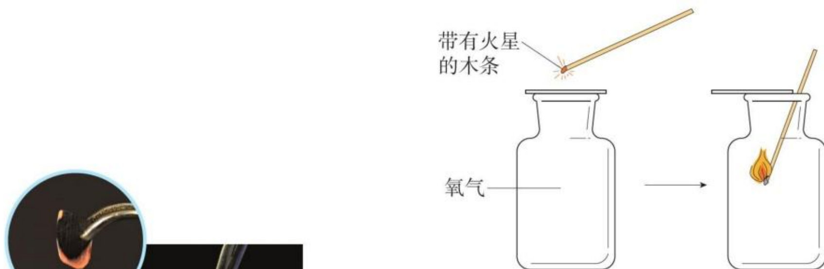
图2-10 氧气可以使带有火星的木条复燃
