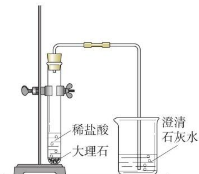
图 1-4 大理石与稀盐酸反应
