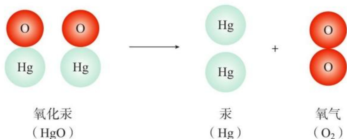
图3-6 氧化汞分子分解示意图
