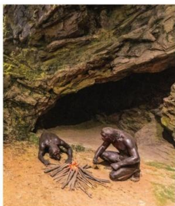
图 7-1 燃烧是人类最早利用的化学反应之一 ①
