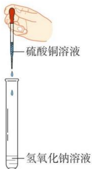
图 1-3 氢氧化钠溶液与硫酸铜溶液反应
