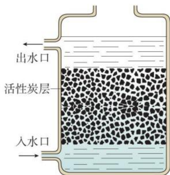
图4-12 活性炭净水器示意图
