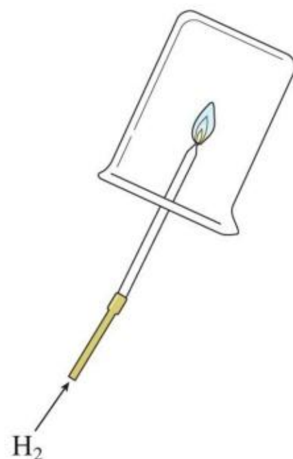
图4-16 氢气在空气里燃烧
