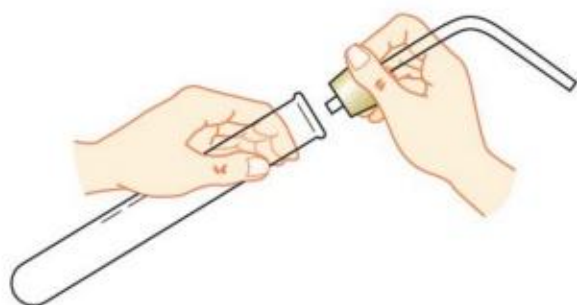
图 1-24 用橡胶塞塞住试管
