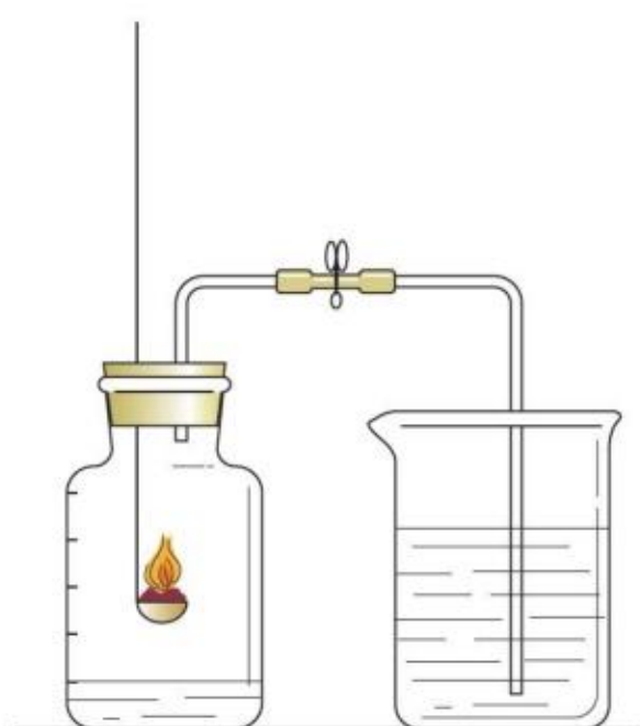
图 2-4 探究空气中氧气含量的装置
