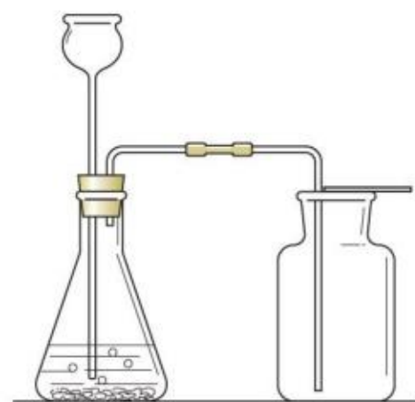
图6-19 实验室里制取二氧化碳的一种装置
