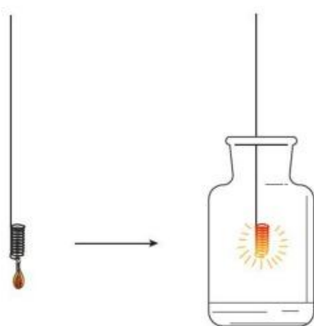
图2-20 铁丝在氧气中燃烧实验示意图
