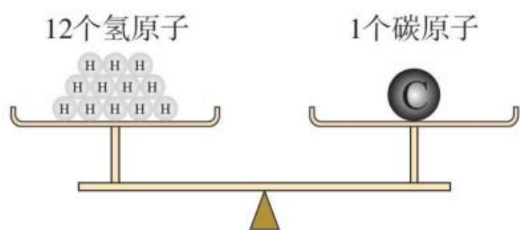
图3-13 相对质量示意图
