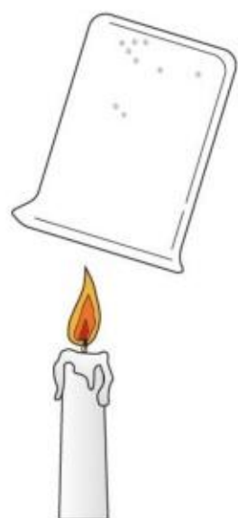
图 1-27 验证蜡烛燃烧的产物
