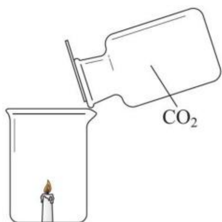
图 6-22 把二氧化碳倒入烧杯
