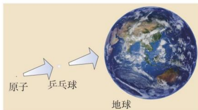
图3-8 原子的体积很小
