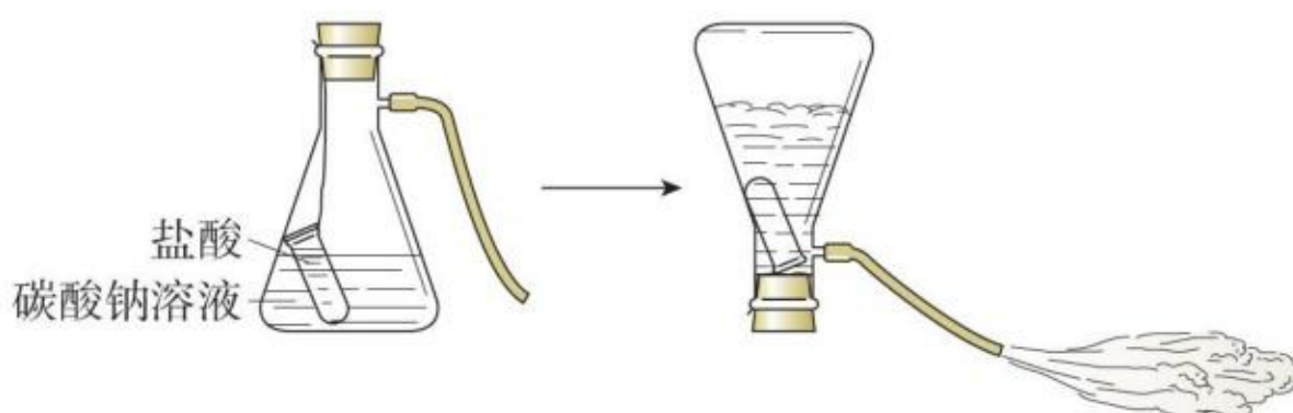
图 7-7 简易灭火器原理示意图
