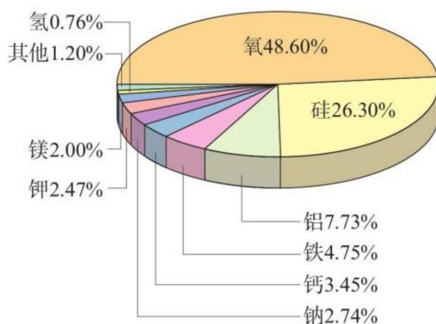
图3-19 地壳中的元素含量（质量分数）
