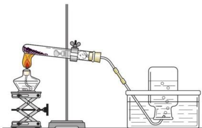
图2-18 高锰酸钾分解制取氧气的装置
