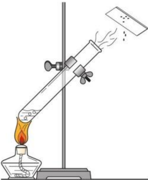
图 1-1 水的沸腾
