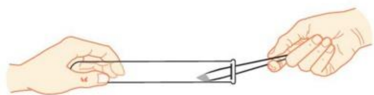
图 1-12 向试管中加入块状试剂
