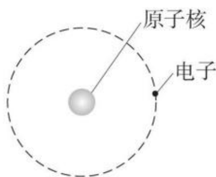
图3-17 卢瑟福原子模型示意图
