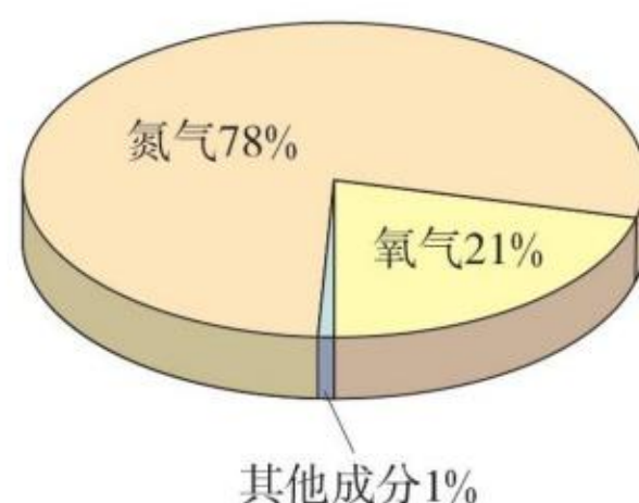
图 2-3 空气成分示意图
