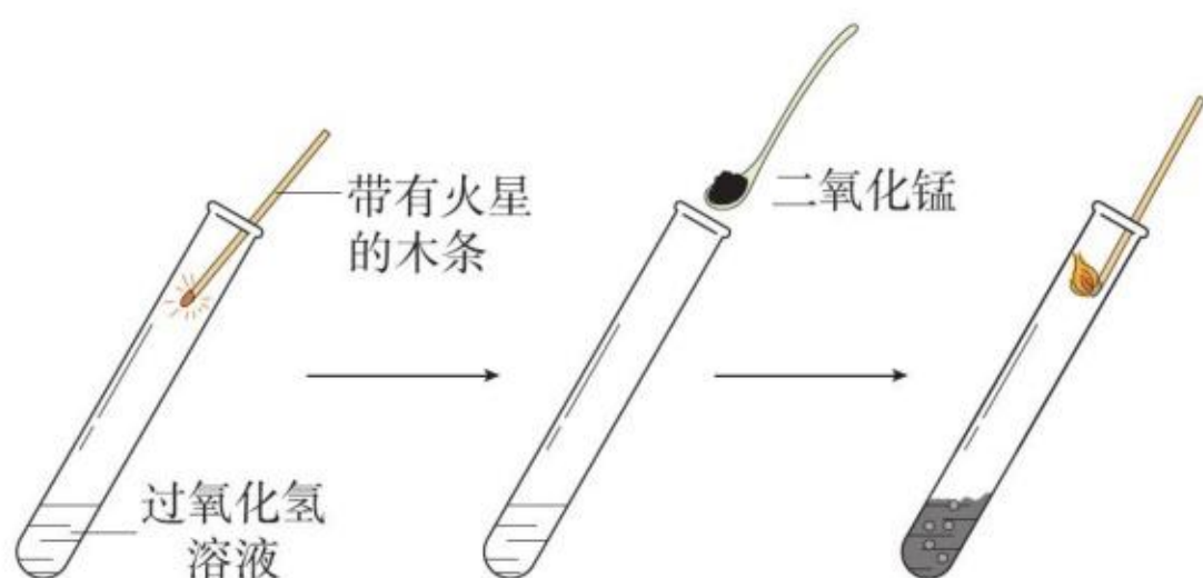
图 2-16 过氧化氢分解实验示意图
