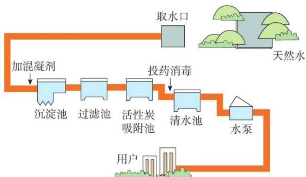
图4-9 自来水厂净水过程示意图
