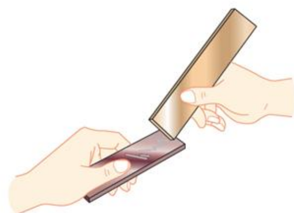
图8-3 比较合金和纯金属的硬度
