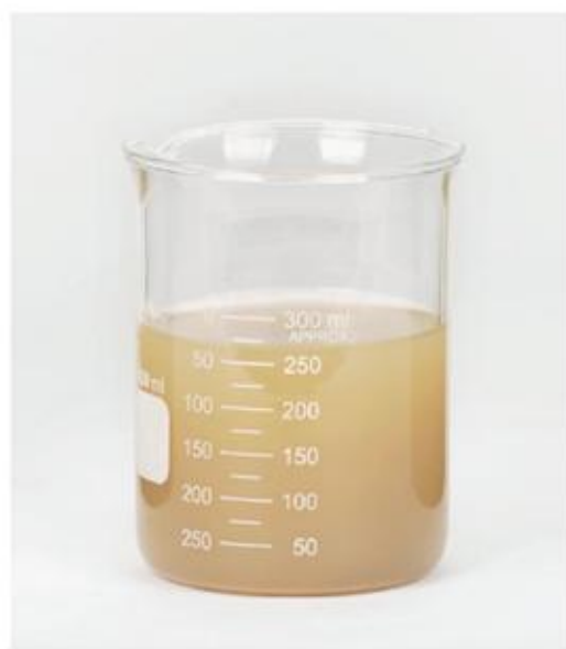
图9-7 悬浊液
