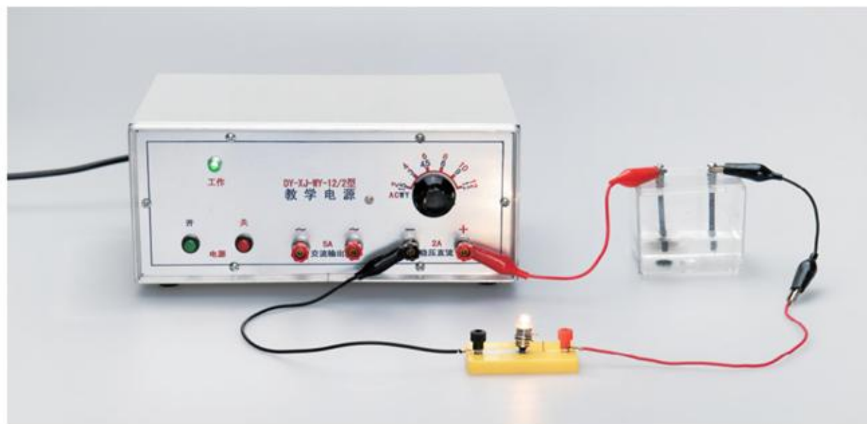
图10-11 试验物质的导电性
