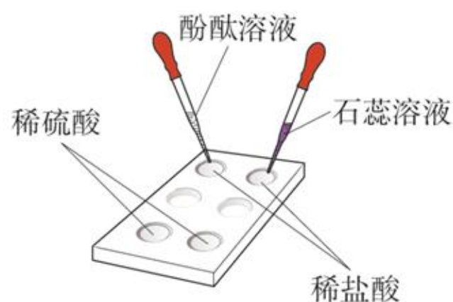
图10-10 酸与指示剂作用
