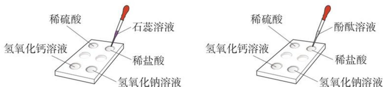
图 10-22 酸、碱与指示剂作用
