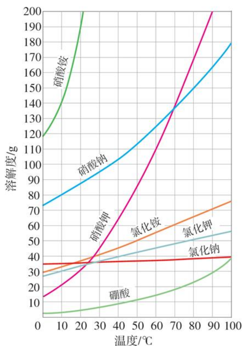
图 9-11 几种固体的溶解度曲线
