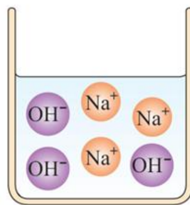
图10-14 NaOH在水中解离出离子示意图
