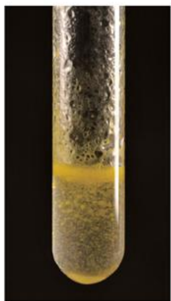
图9-6 乳浊液
