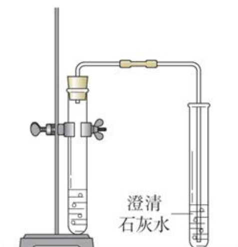
图10-19 碳酸钠与稀盐酸反应的装置
