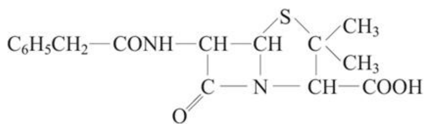
图11-7 青霉素的分子结构
