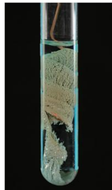
图 8-12 铜与硝酸银溶液的反应
