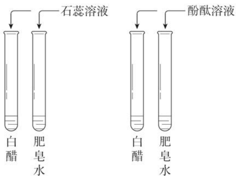
图 10-1 向溶液中加入酸碱指示剂
