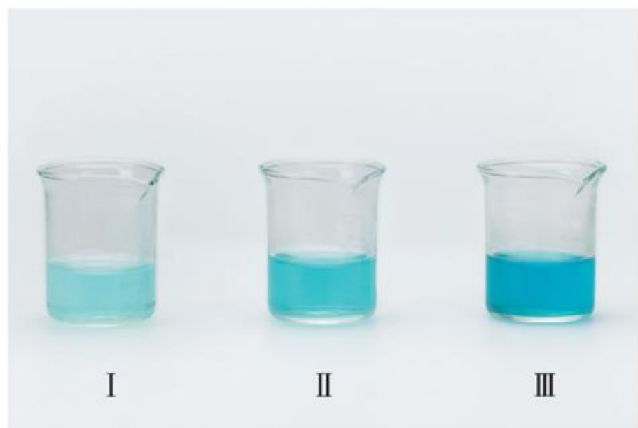
图9-15 三种浓稀程度不同的硫酸铜溶液
