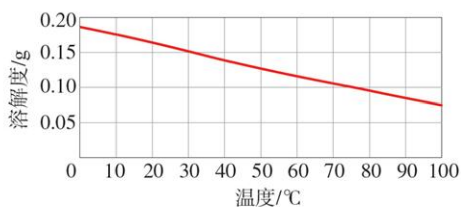
图 9-12 氢氧化钙的溶解度曲线
