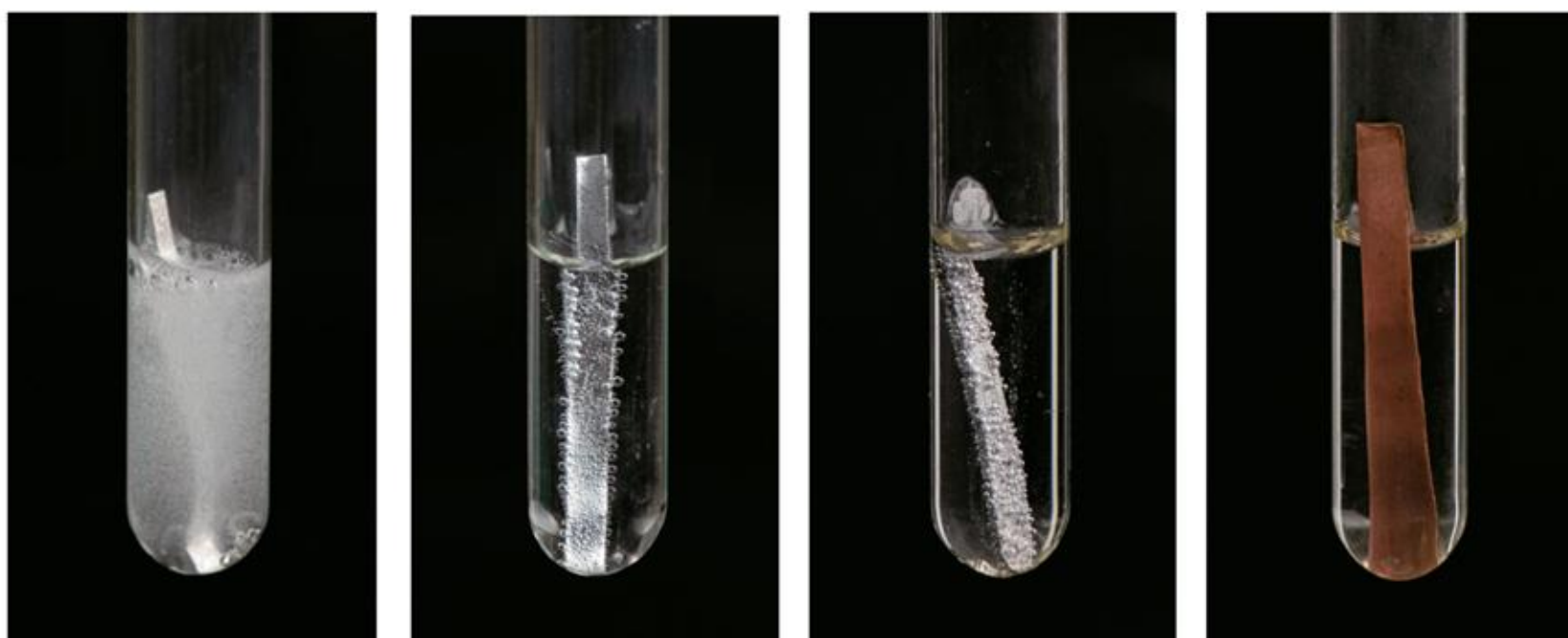
图 8-10 镁、锌、铁、铜分别在稀盐酸中
