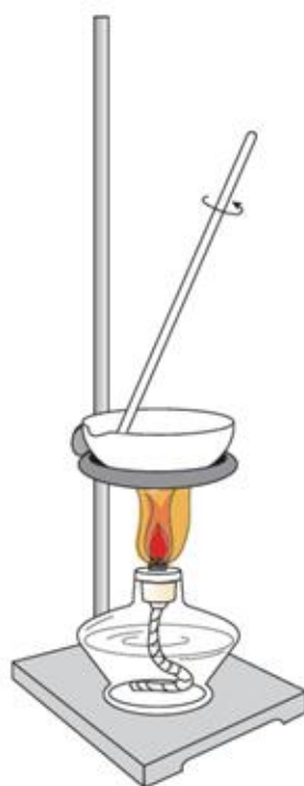
图9-19 蒸发
