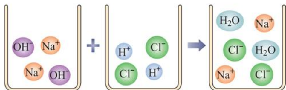
图 10-16 氢氧化钠与盐酸反应示意图
