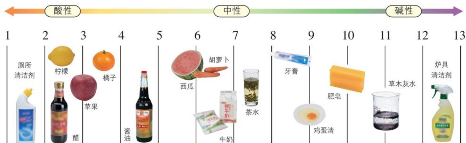
图 10-5 身边一些物质的 pH
