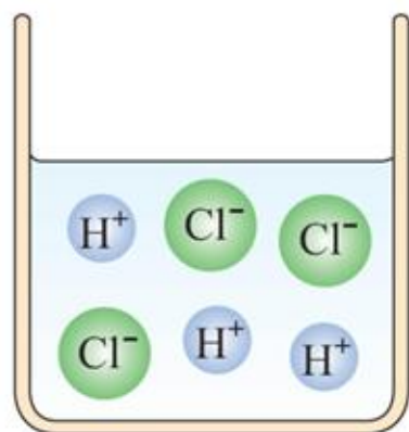
图10-12 HCl在水中解离出离子示意图
