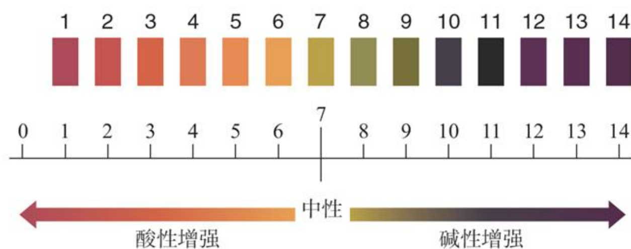
图 10-3 \text{pH} 和溶液的酸碱性
