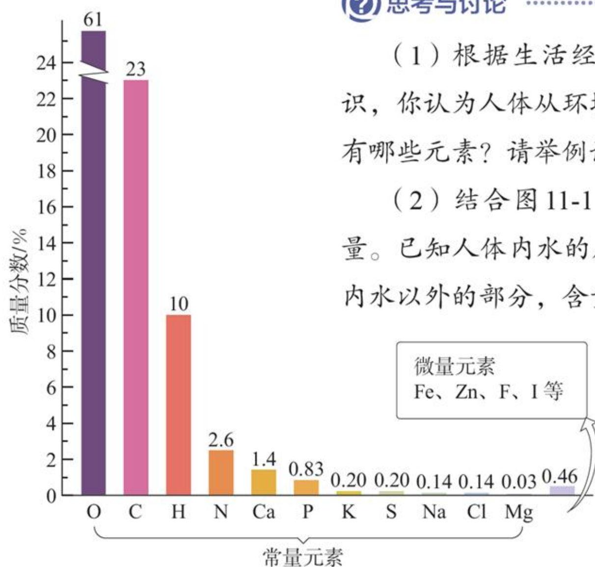
图 11-1 人体中元素的含量
