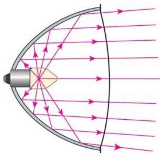
图4.3-7 汽车前灯的反光装置
