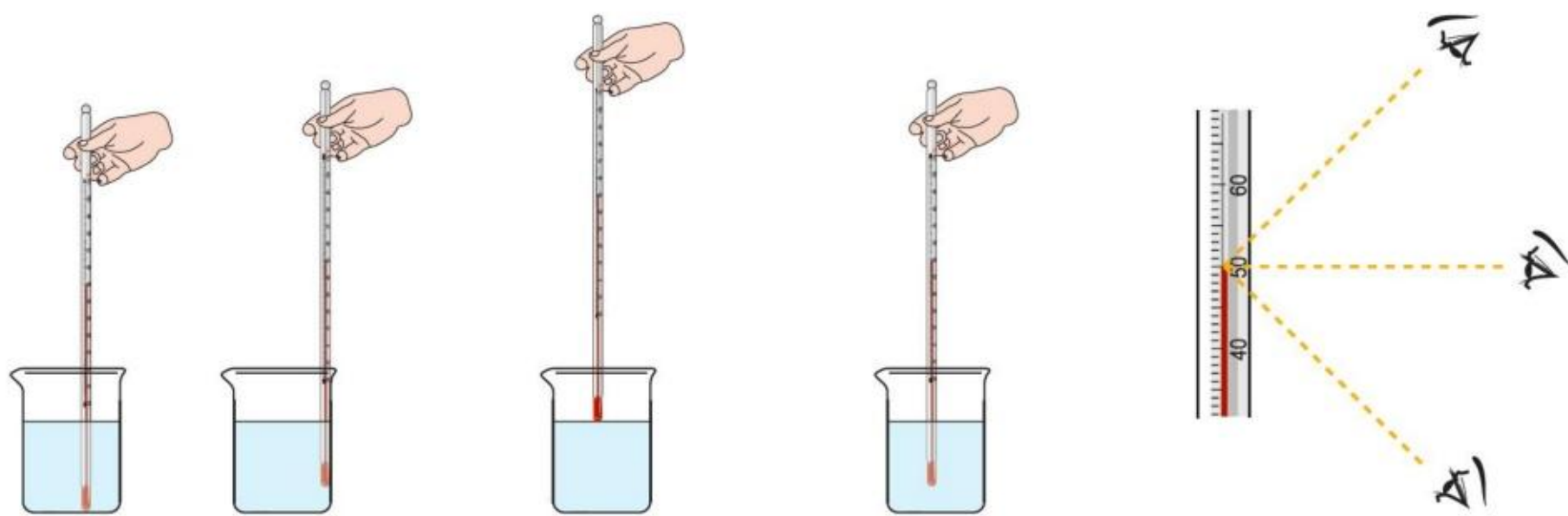
图3.1-4 温度计的使用和读数方法
