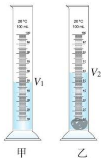
图6.3-3 用量筒测量形状不规则固体的体积
