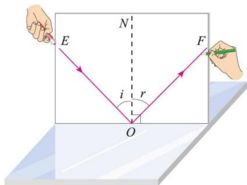
图4.2-3 探究光反射时的规律
