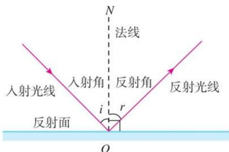
图 4.2-5 光的反射
