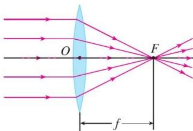
图5.1-7 凸透镜的焦点和焦距
