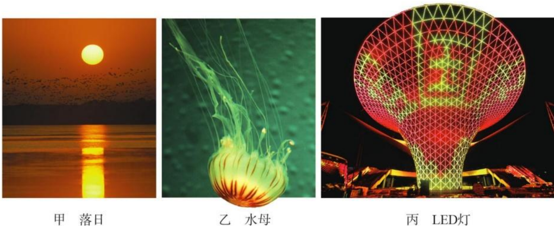
图4.1-1 发光的物体
