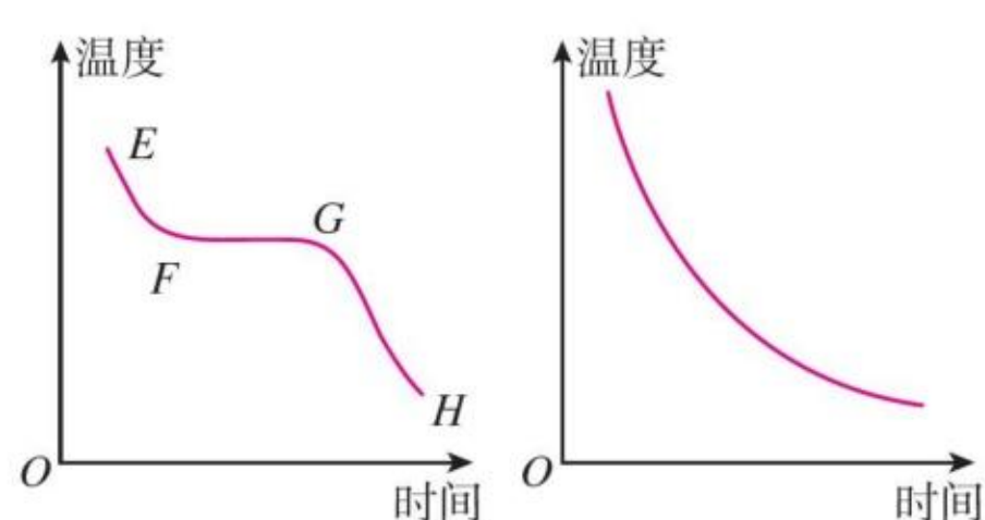
甲 晶体
