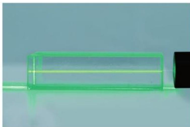
乙 光在玻璃中的传播
