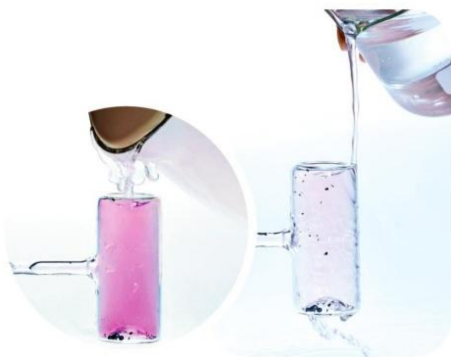
图3.4-1 观察碘的物态变化
