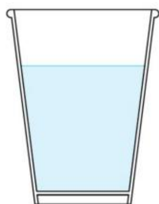
甲 热水
