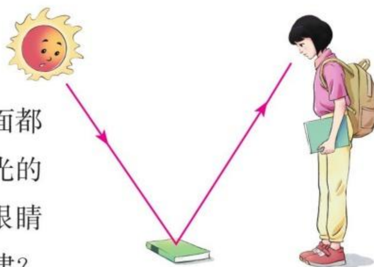
图4.2-2 反射光进入人眼
