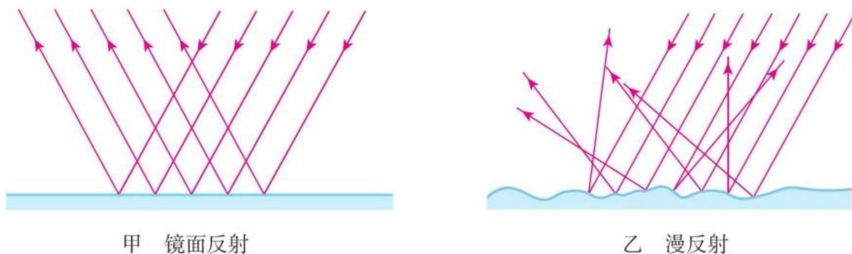
图4.2-7 两种反射
