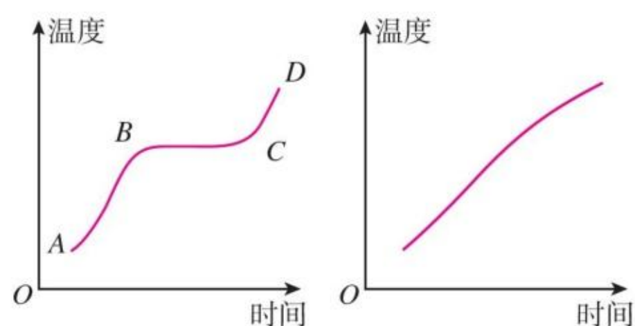
甲 晶体
