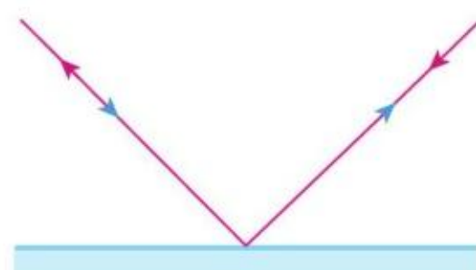
图 4.2-6 光路可逆
