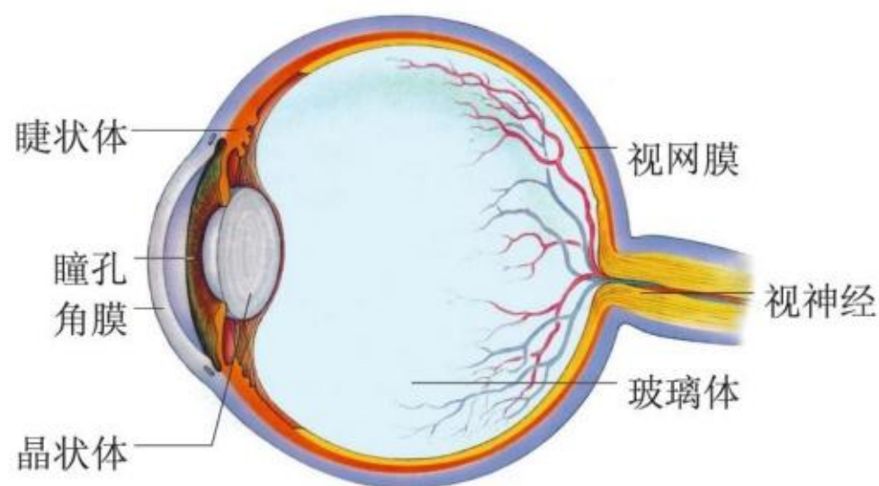
图5.4-1 眼球主要的结构
