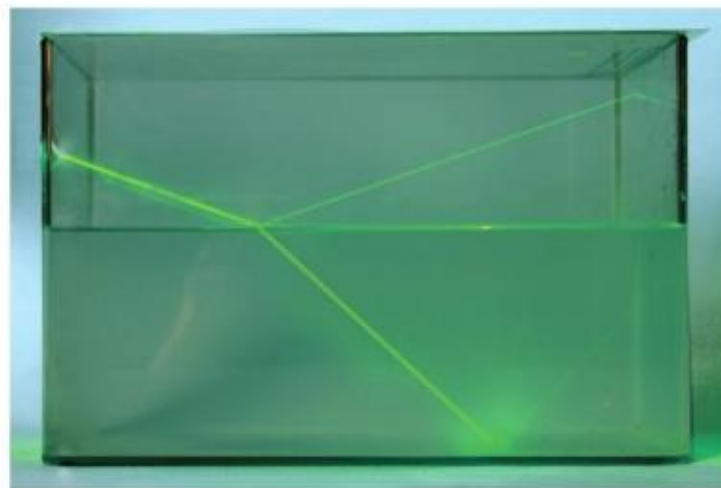
图4.4-2 光斜射入水中时的折射现象
