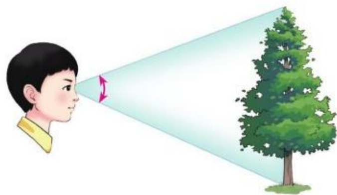
图5.5-3 视角
