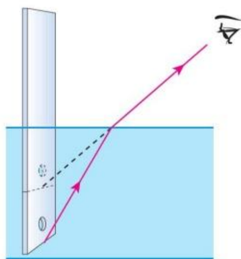
图4.4-4 池水变“浅”了
