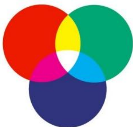
图4.5-3 色光的三原色
