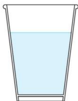
乙 冰水
