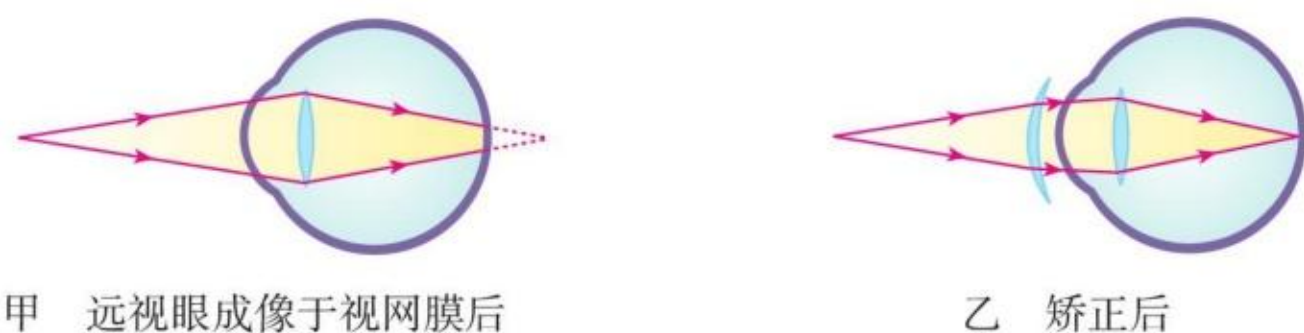
图5.4-4 远视眼及其矫正
