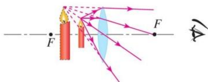
图5.2-8 凸透镜成虚像的情景
