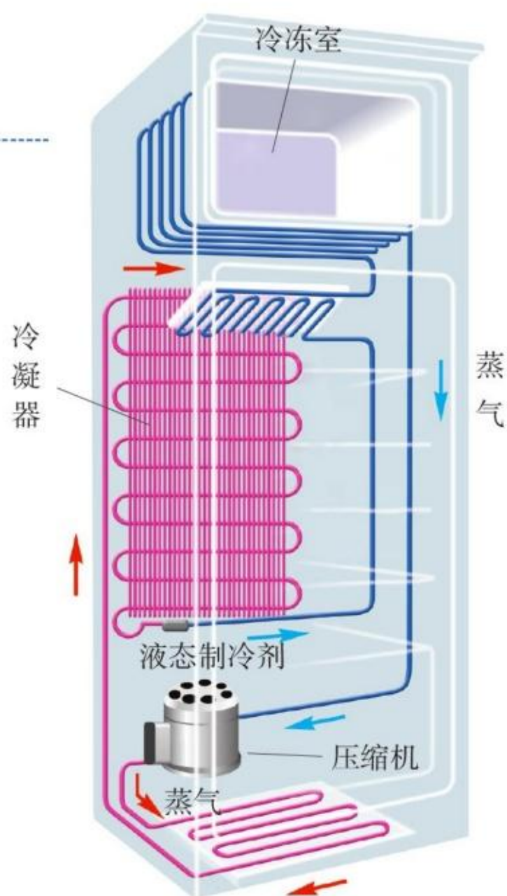
图3.3-7 一种电冰箱的原理图
