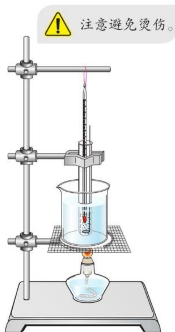
图 3.2-2 观察熔化现象的实验装置
