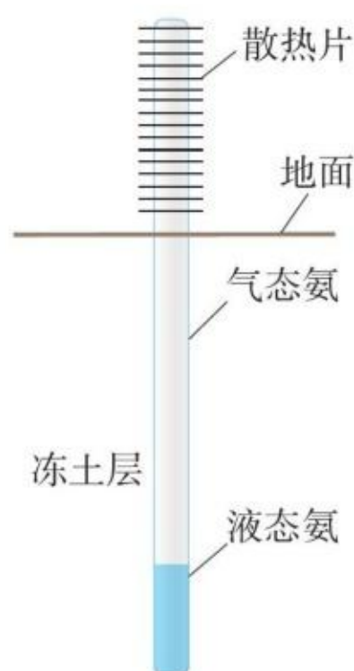
图3.3-9 热棒示意图
