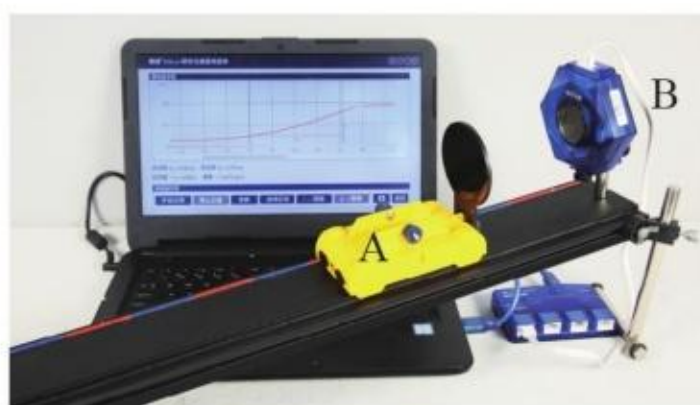
图1.4-3 利用传感器测量物体运动的速度
