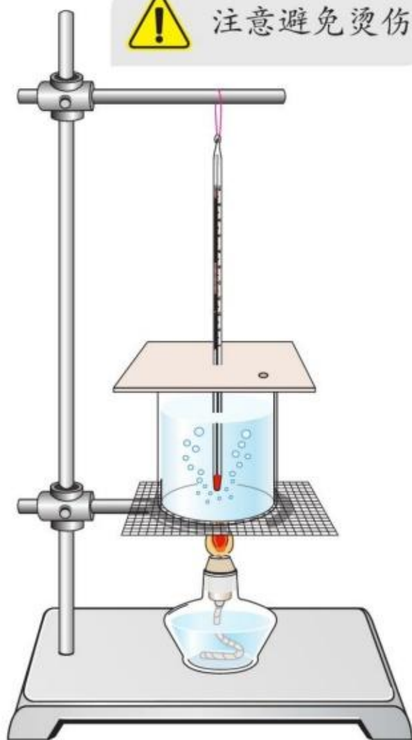
图3.3-2 观察水沸腾的实验装置
