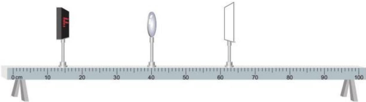
图5.3-2 探究凸透镜成像规律的装置
