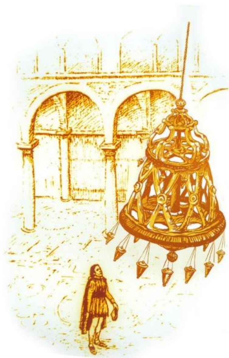
图10 伽利略 (G. Galilei, 1564—1642)
