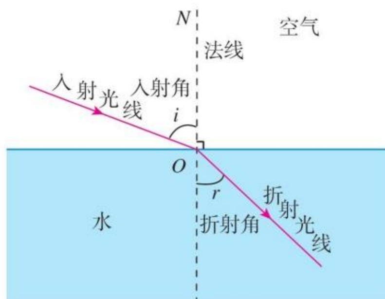
图4.4-3 光的折射
