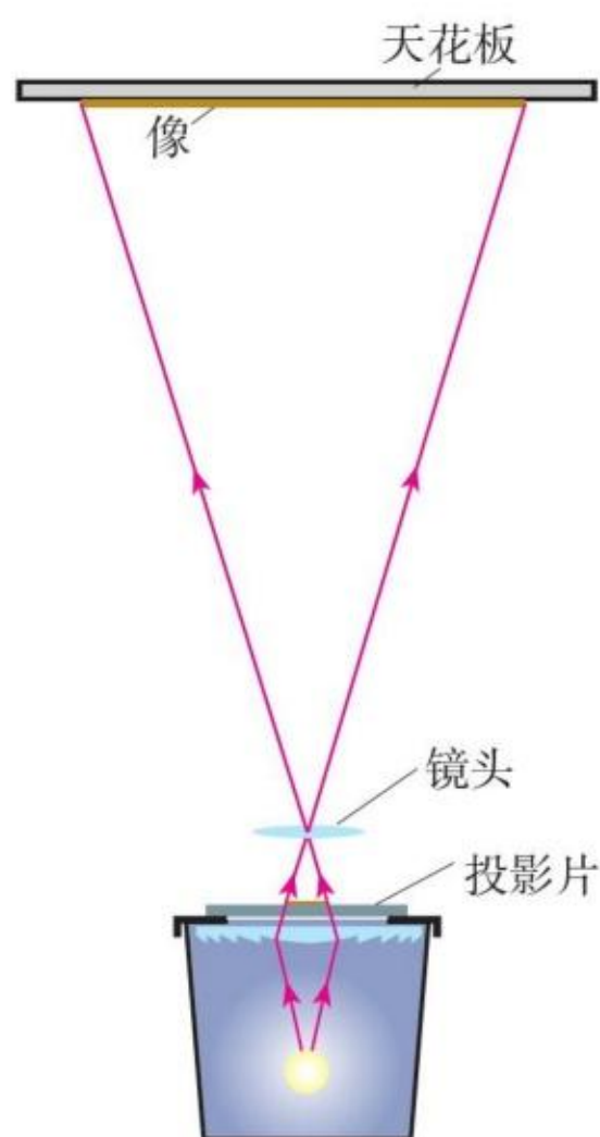
图5.2-4 投影仪成像
