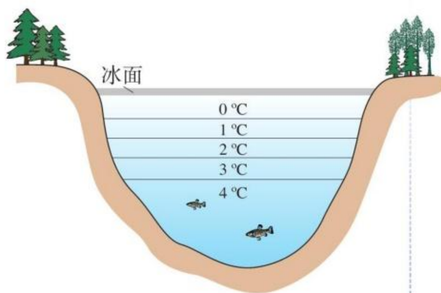
图6.2-3 冬天湖水温度分布示意图
