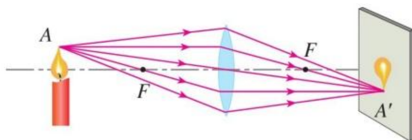
图5.2-7 凸透镜成实像的情景
