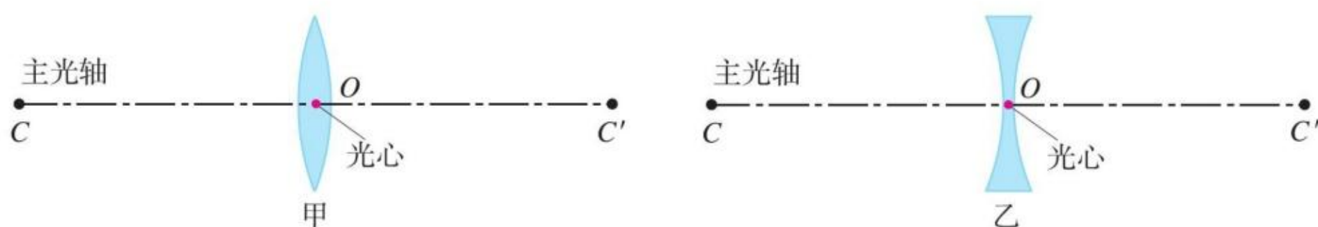
图5.1-3 透镜的主光轴和光心
