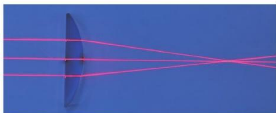
图5.1-5 凸透镜使光会聚
