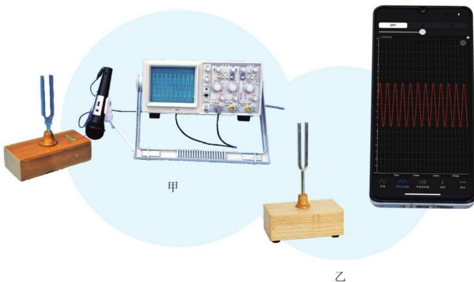
图2.2-3 声音的波形
