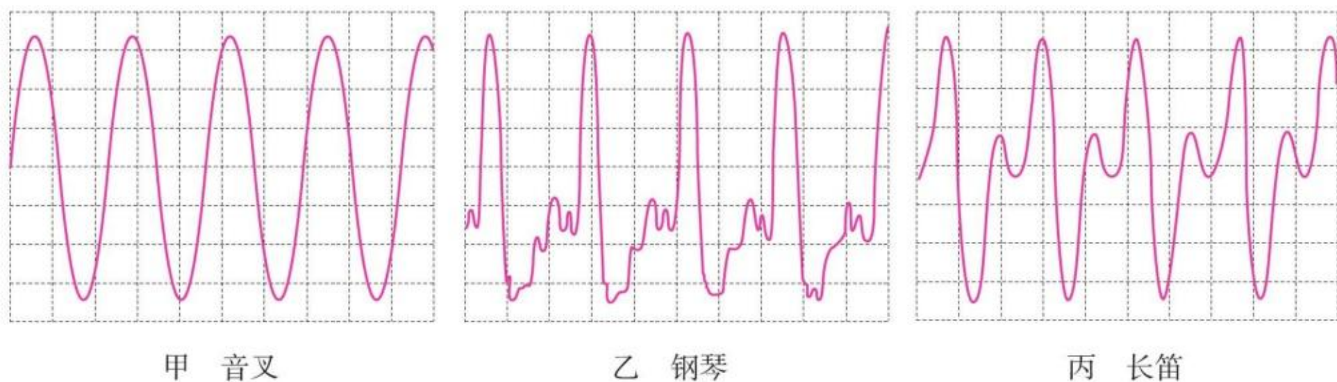
图2.2-5 声音的波形
