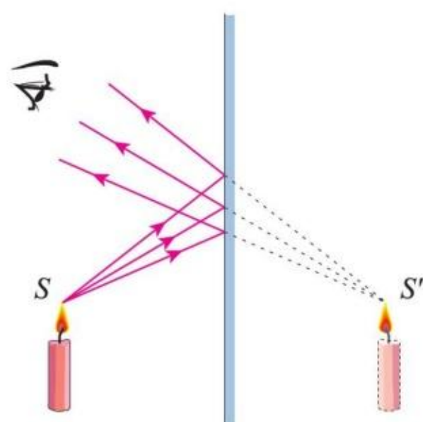
图4.3-3 平面镜中的像是虚像
