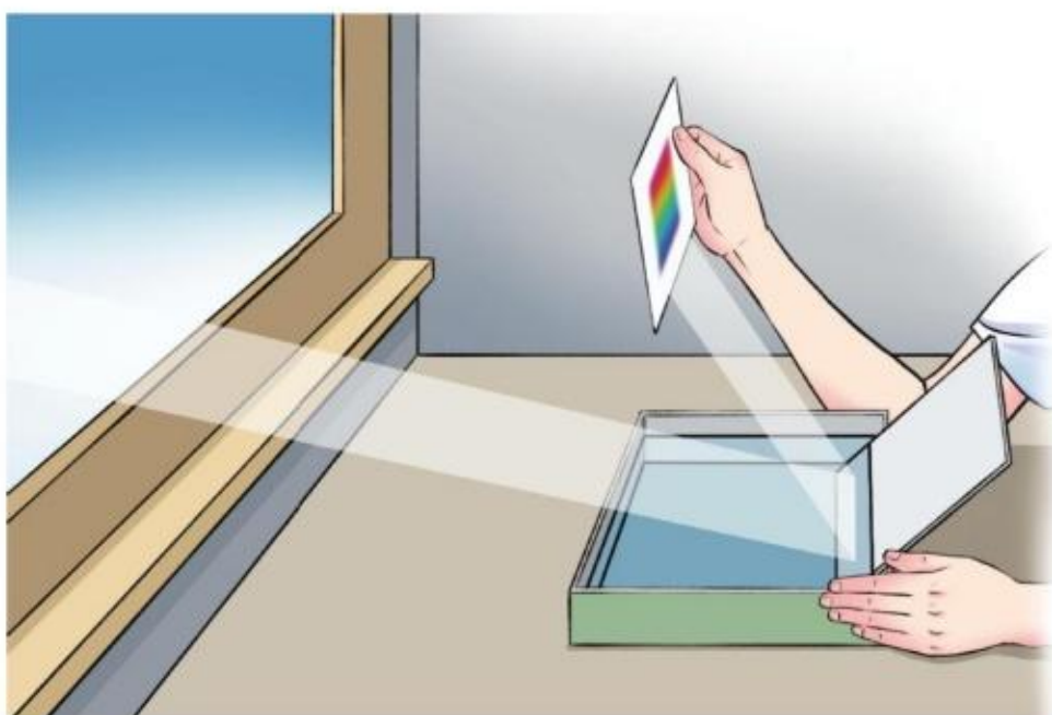
图4.5-2 光的色散实验
