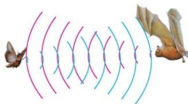
图2.3-3 蝙蝠靠超声波发现昆虫
