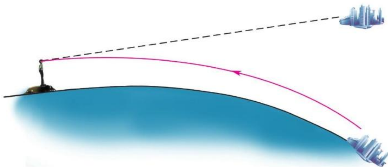
图4.4-6 海市蜃楼的成因
