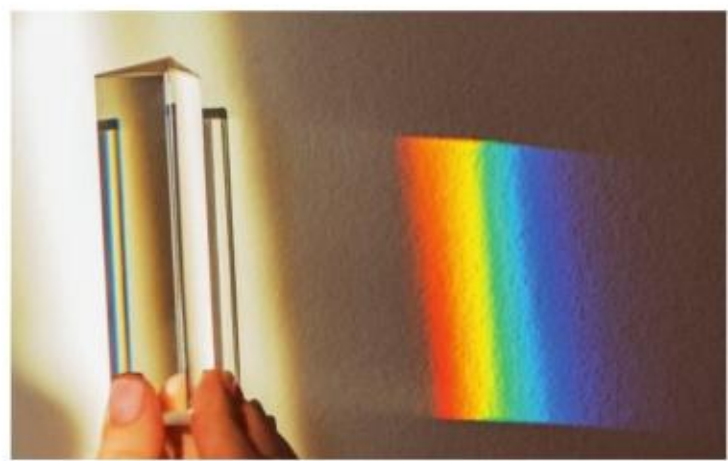
图4.5-1 光的色散
