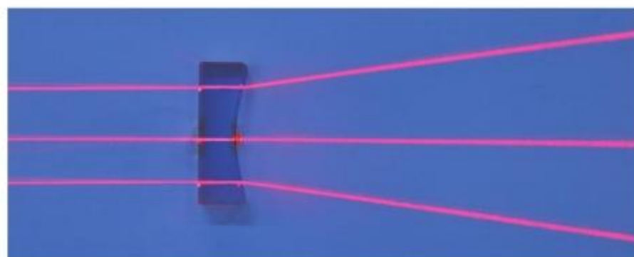
图5.1-6 凹透镜使光发散
