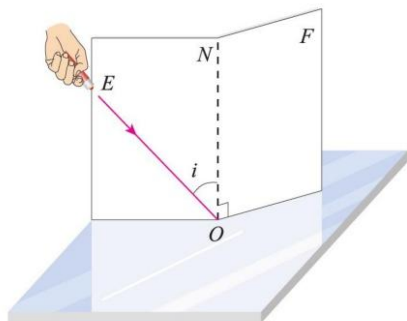
图4.2-4 是否还能看到反射光
