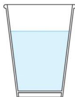
丙 室温水
