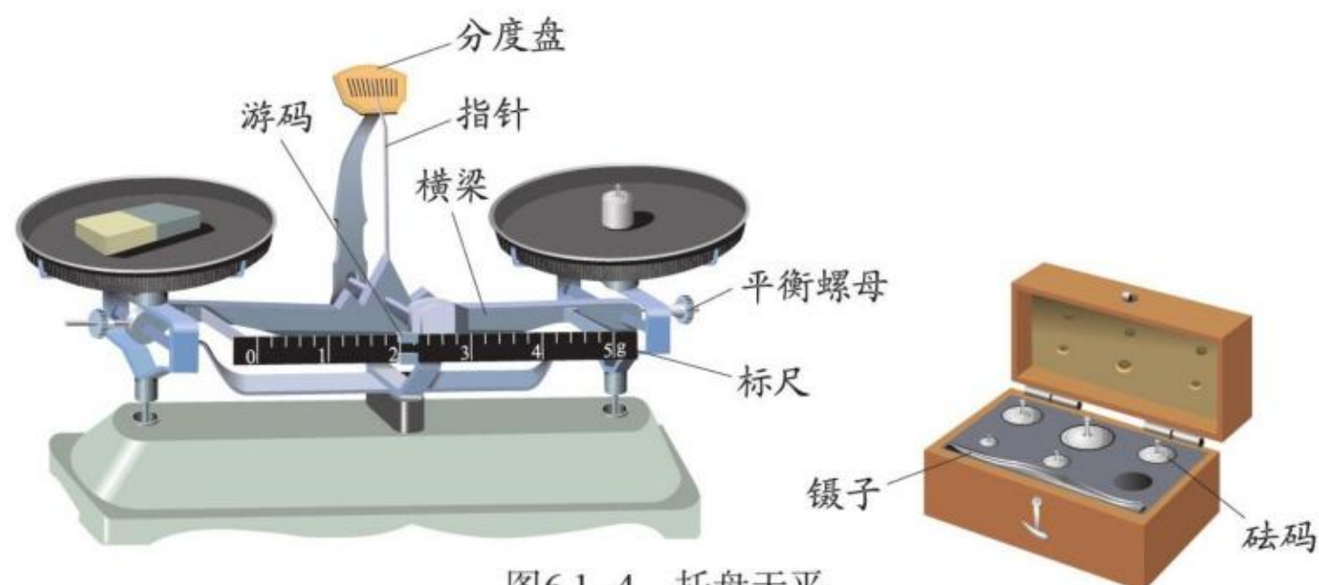
图6.1-4 托盘天平
