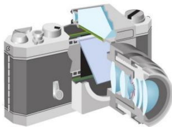
图 5.1-1 照相机镜头剖面图
